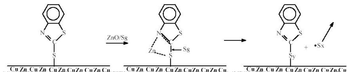
Figura 3.18 – Mecanismo de inserção do S na ligação latão-S [19].
