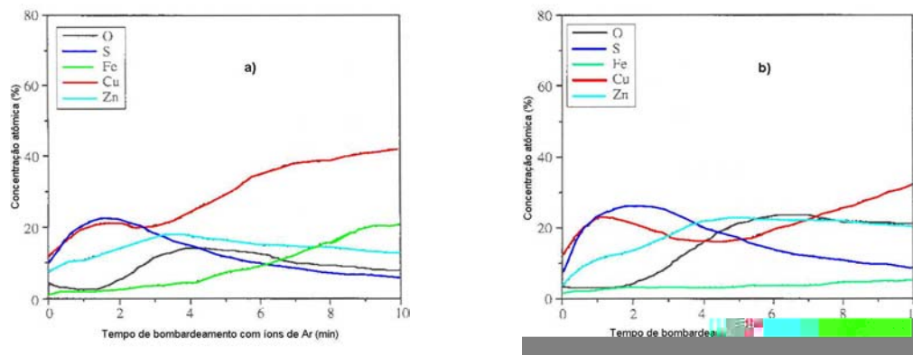
Figura 3.32 – a) AES em perfil de profundidade da superfície de uma corda metálica com deposição de 5 nm de Co no latão (Alto Cobalto), não envelhecida; b) amostra envelhecida 15 dias em umidade. Taxa de remoção equivalente a 9 nm/min [14].
