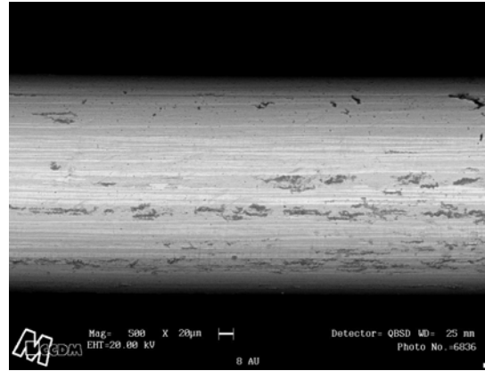
Figura 5.77 – MEV para o Experimento 8 em AU com QSBD.
