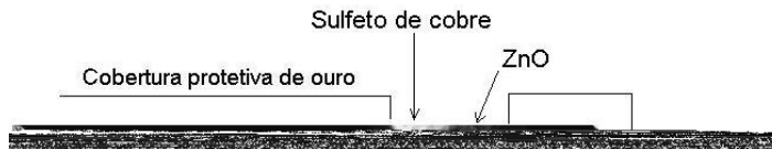
Figura 3.44 – TEM da seção transversal da interface de ligação do latão com o composto com cobalto não envelhecido. Magnificação: 250000x [43].
