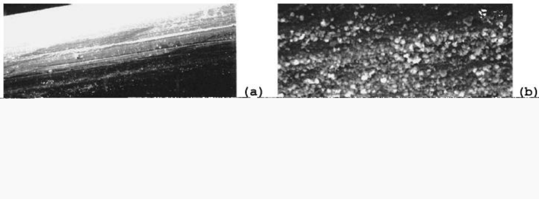
Figura 3.38 – MEV de uma corda metálica latonada sulfetizada em mistura de esqualeno com HMMM e Resorcinol: a) A= 300x; b) A= 4000x [41].
