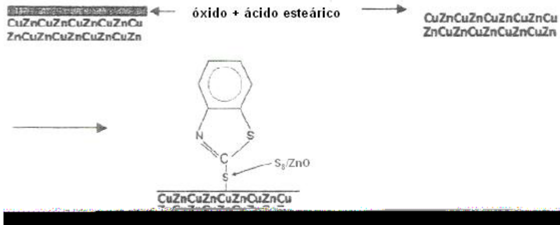
Figura 3.17 – Formação do complexo entre o fragmento do acelerador e o latão [19].
