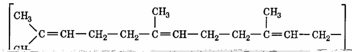
Figura 3.13 – Estrutura molecular do esqualeno [35].
