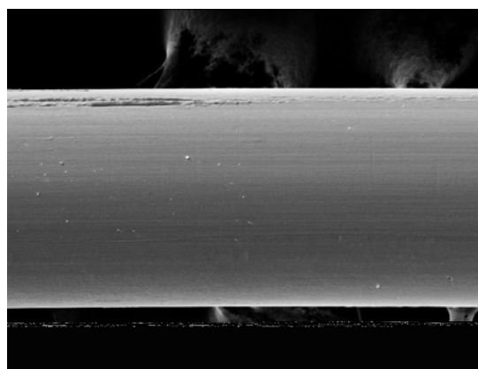
Figura 5.106 – MEV para o Experimento 6 em CC.
