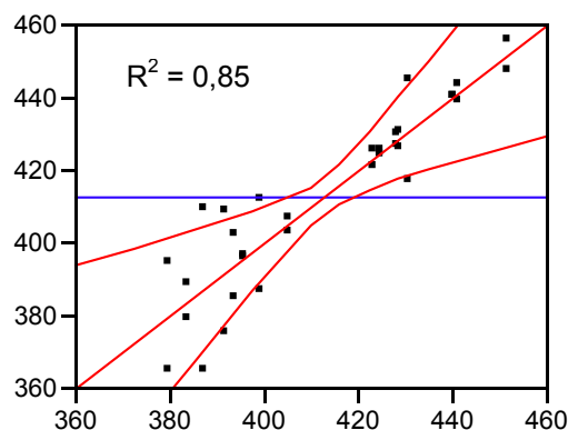
Figura 5.33 – Ajuste dos resultados de Carga para os experimentos envelhecidos em Estufa.
