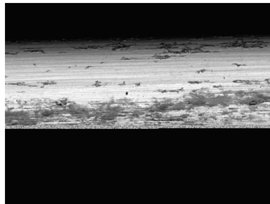
Figura 5.97 – MEV para o Experimento 16 envelhecida em AU com QSBD.
