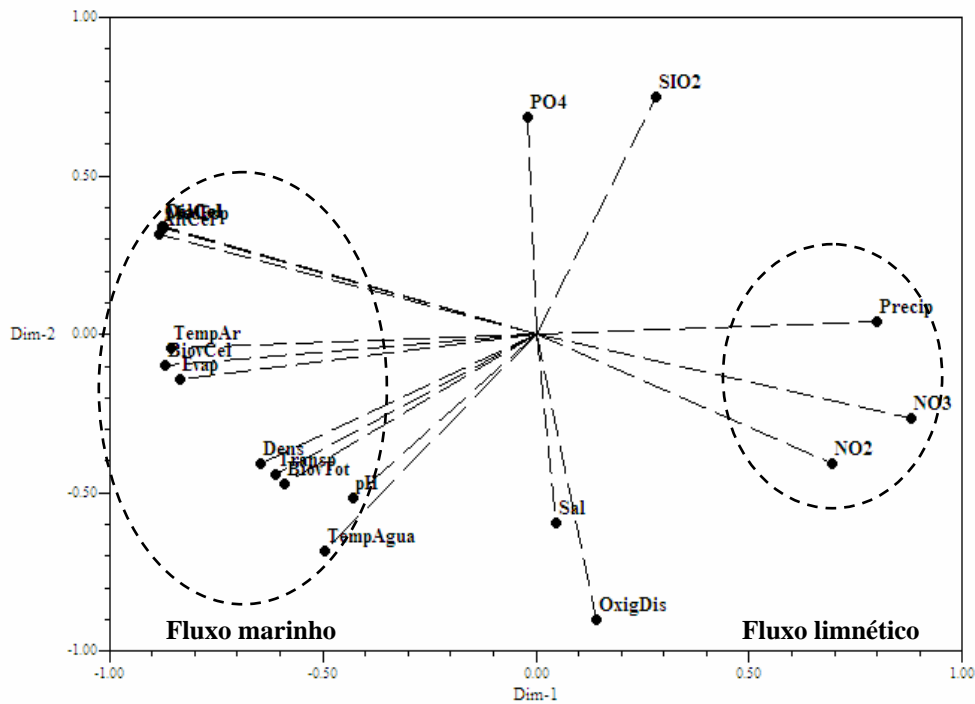
Fig 30- Análise dos Componentes Principais no estuário da bacia do Pina, Recife (PE) no período seco e chuvoso (siglas na tabela 2).
