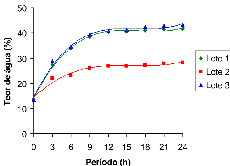
Figura 1 - Curva de hidratação de três lotes de sementes de arroz cv IRGA 417 no período de 24 horas. Santa Maria – RS, 2006.
