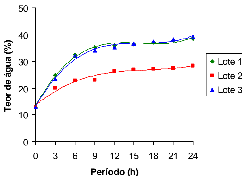
Figura 2 - Curva de hidratação de três lotes de sementes de arroz cv IRGA 422 CL no período de 24 horas. Santa Maria – RS, 2006.
