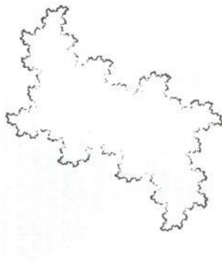
Figura 2.8 Conjunto conectado de Julia para c = 0,1 - 0,6i , usando 20000 pontos selecionados randomicamente.
