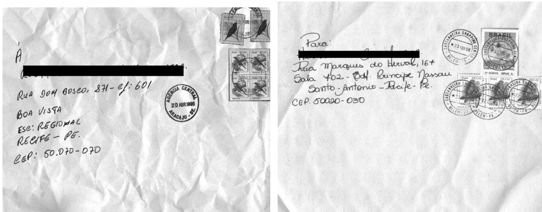
Figura 6.2 Imagens Sintetizadas
