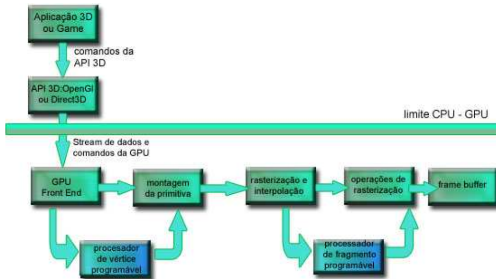
Figura 10 - Pipeline gráfico programável
