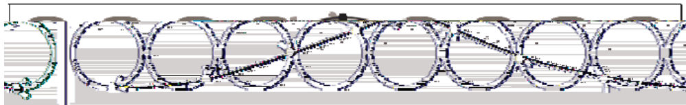
Figura 14 – Posição de uma partícula de água com o movimento da onda
