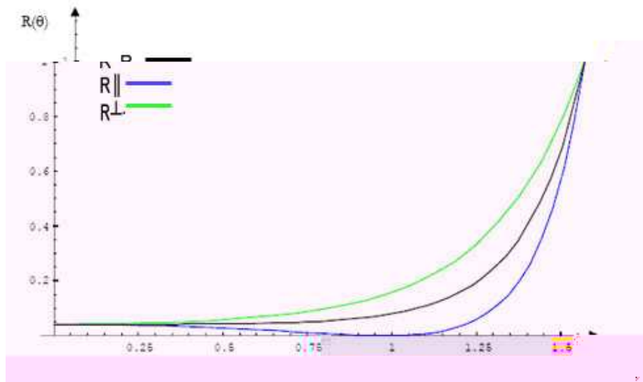
Figura 37 - O gráfico para R , R^\perp e R^\parallel
