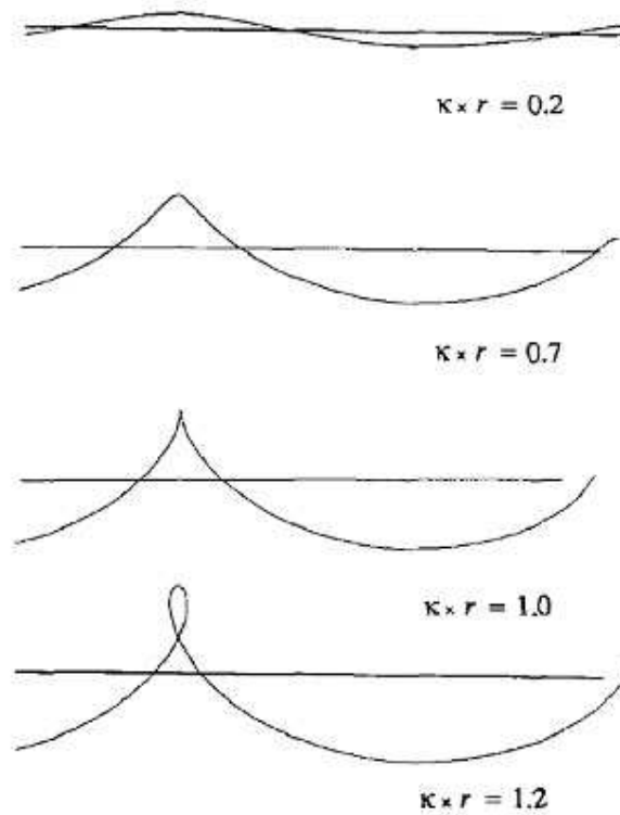
Figura 13 – Formas de onda variando o parâmetro \kappa r .
