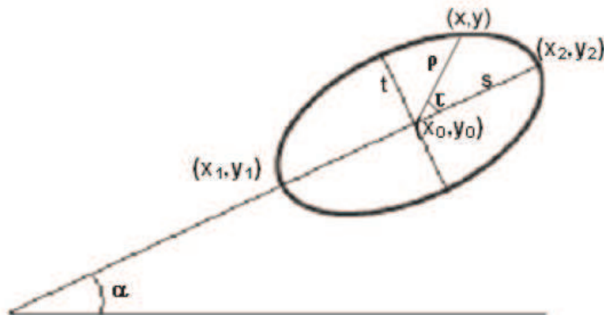
Figura 23 – Considerando a inclinação do fundo do mar na simulação
