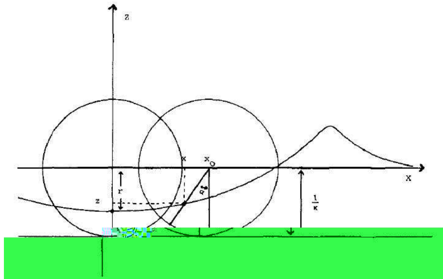
Figura 12 – A trocóiide
