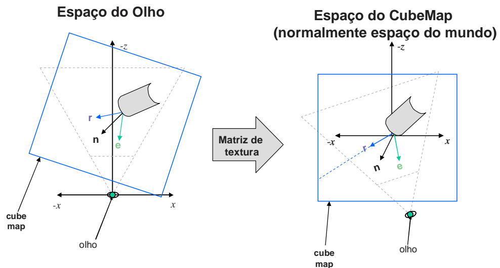
Figura 33 – Diagrama do mapeamento de reflexão
