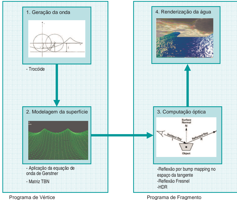
Figura 11 – Estágios do sistema de simulação
