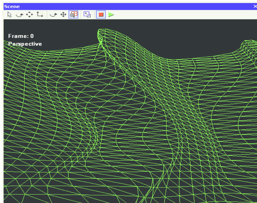
Figura 16 – Acrescentando a influência do vento.
