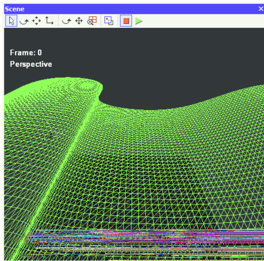
Figura 24 – Onda se quebrando na costa
