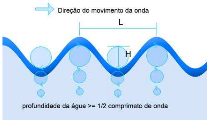
Figura 4 – Ondas de águas profundas
