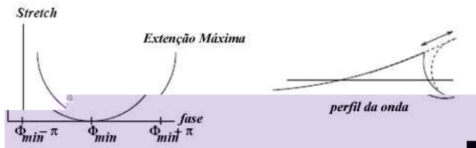
Figura 28 – Função Stretch
