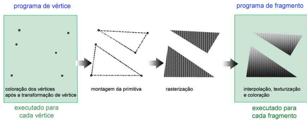
Figura 9 - Pipeline gráfico
