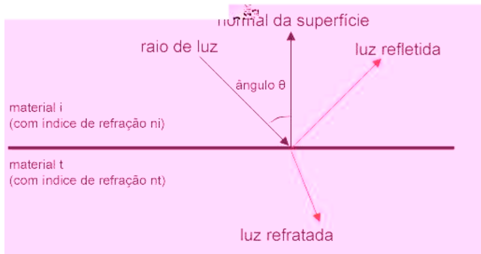
Figura 36 - Raio de luz viajando através de dois meios materiais.
