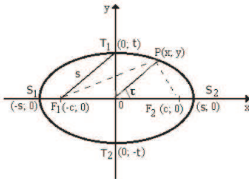
Figura 21 - Elipse
