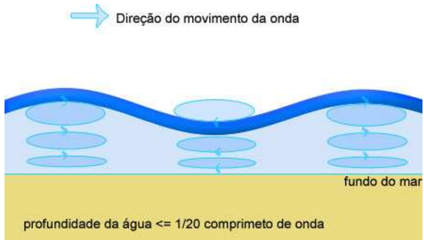
Figura 5 – Ondas de águas rasas
