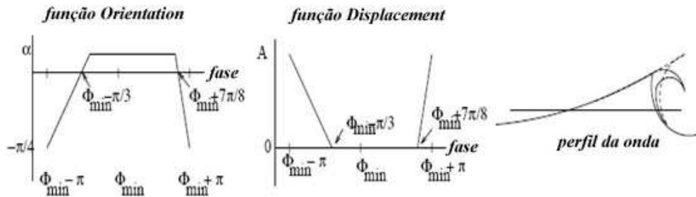
Figura 29 – Quebra da onda
