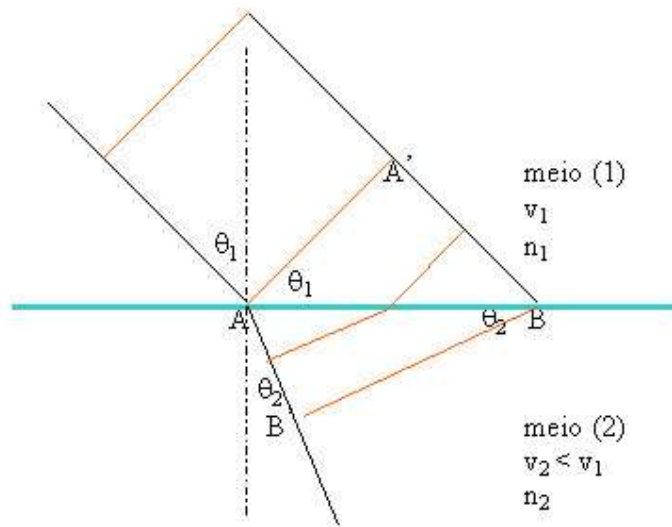
Figura 18 – Frente de onda na refração de acordo com a lei de Snell.
