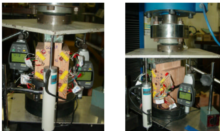
FIGURA 3.12 – Esquema dos Ensaios com Célula de Carga, Tarugo de Distribuição da Força, Medidores de Deslocamentos e Corpos-de-Prova Posicionados na Máquina Universal de Ensaio
