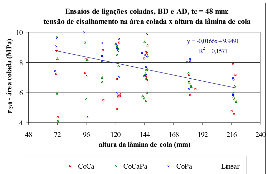
FIGURA 4.44 – Gráfico Tensão Média de Cisalhamento na Área Colada x Altura da Lâmina Adesiva, LCP, Madeira BD e AD, t_c = 48 mm
