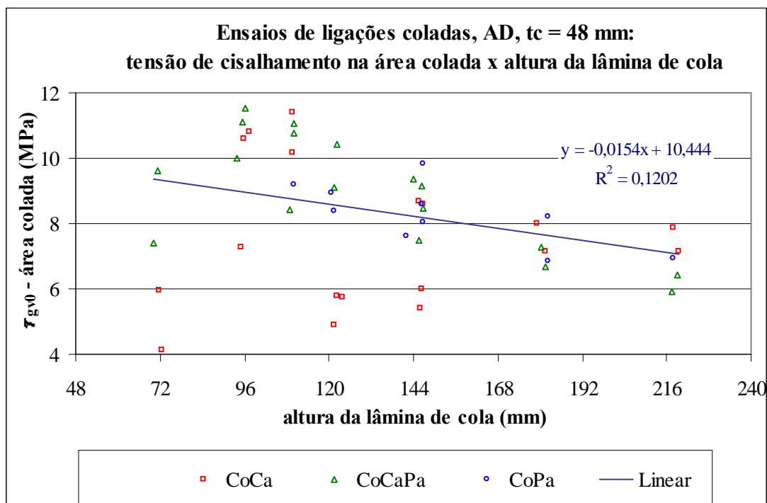
FIGURA 4.40 – Gráfico Tensão Média de Cisalhamento na Área Colada x Altura da Lâmina Adesiva, LCP, Madeira AD, t_c = 48 mm
