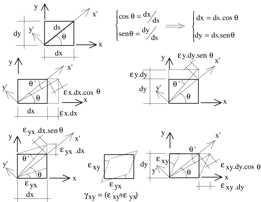
FIGURA 2.28 – Relações Geométricas entre Deformações em Elemento Infinitesimal
