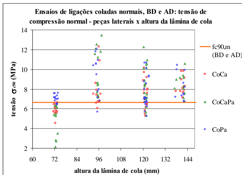
FIGURA 4.61 – Tensão de Compressão Normal Média nas Peças Laterais em Função da Altura da Lâmina Adesiva, Madeira BD e AD
