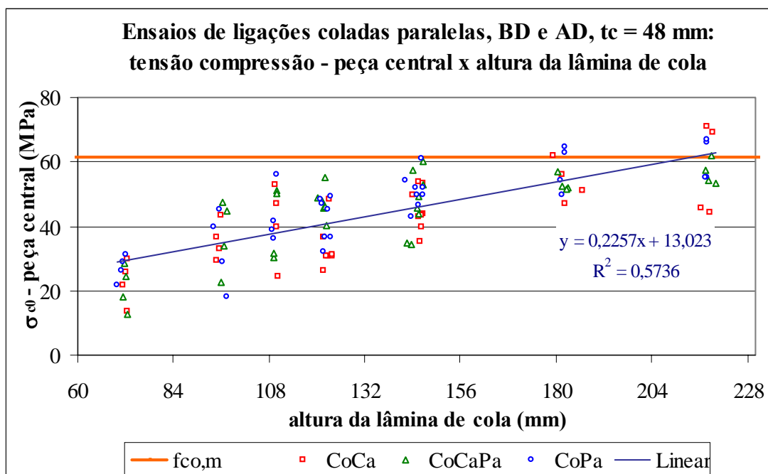
FIGURA 4.42 – Gráfico Tensão Média de Compressão da Peça Central x Altura da Lâmina Adesiva e Correspondente Retas de Correlação, LCP, Madeira BD e AD, t_c = 48 mm
