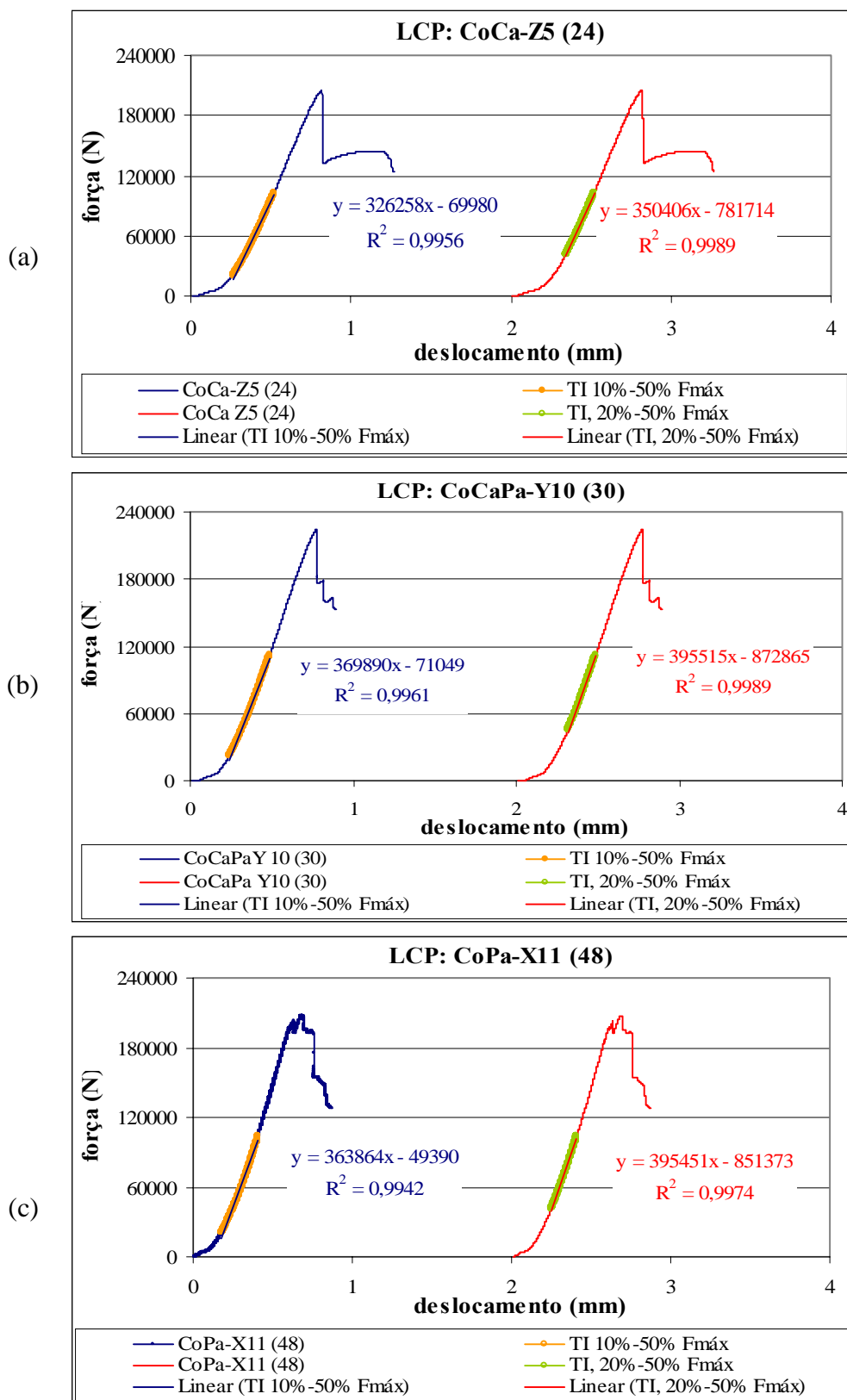
FIGURA B.1 - Gráficos Força x Deslocamento, LCP: a) CoCa Z5, t_c = 24 mm;
