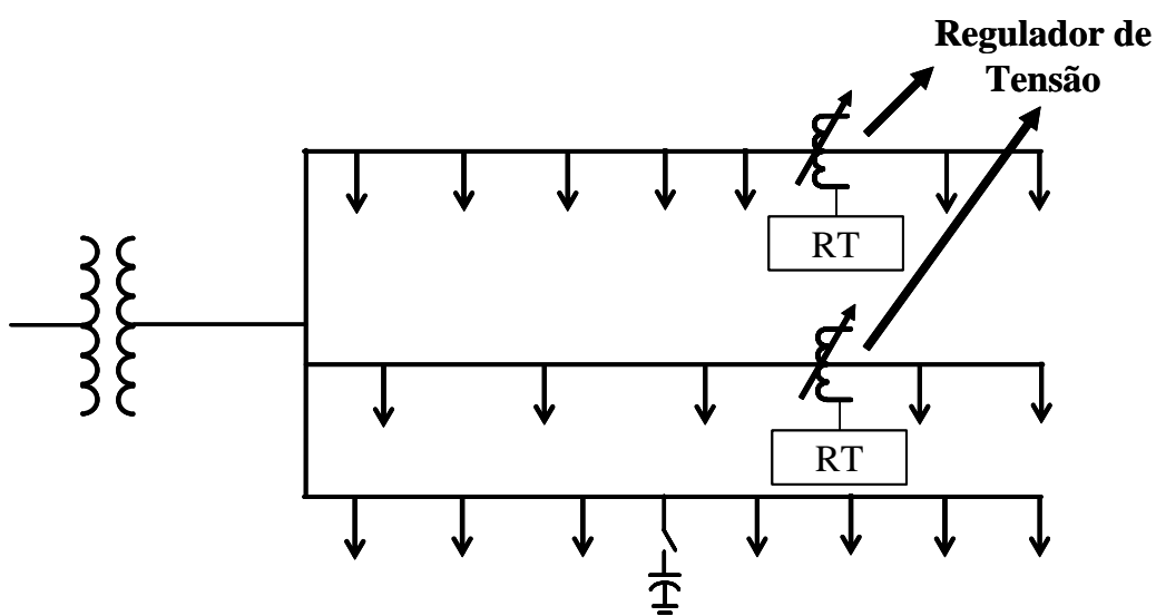
Figura 2.6 - Reguladores de tensão instalados ao longo dos alimentadores.
