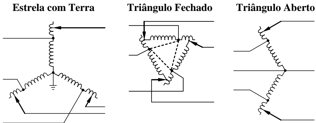
Figura 2.8 – Conexões trifásicas para o autotransformador.
