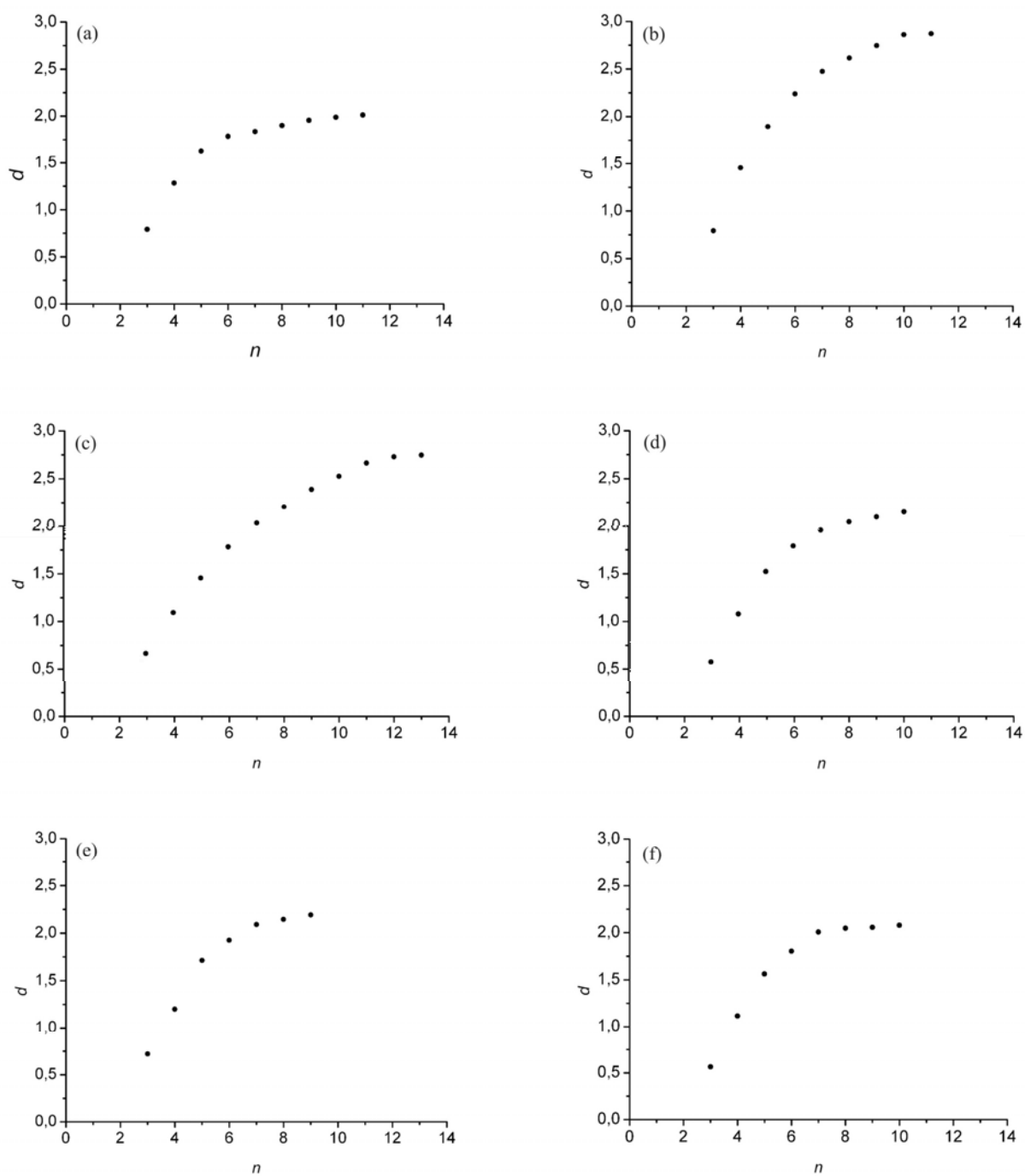
Figura 14 – Comportamento da dimensão embutida, d , para o fluxo de CO 2 , sendo: (a) fevereiro de 2001. (b) junho e julho de 2002. (c) fevereiro de 2003. (d) julho de 2005. (e) janeiro e fevereiro de 2006. (f) agosto de 2006.
