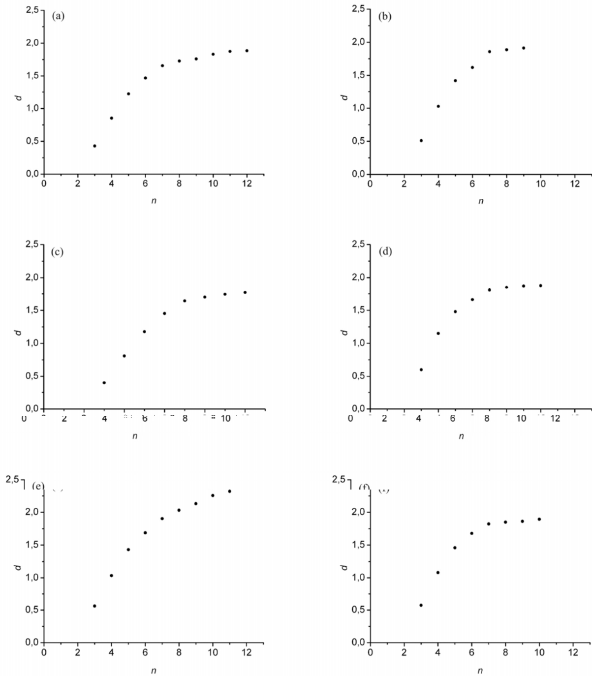
Figura 15 – Comportamento da dimensão embutida, d , para o fluxo de calor latente, sendo: (a) fevereiro de 2001. (b) junho e julho de 2002. (c) fevereiro de 2003. (d) julho de 2005. (e) janeiro e fevereiro de 2006. (f) agosto de 2006.
