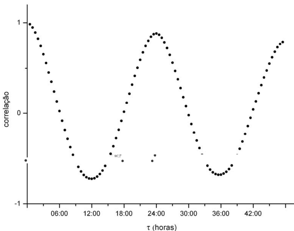
Figura 23 – Comportamento da correlação entre a série temporal do período de julho e julho de 2002 para temperatura e a mesma série defasada em \tau .
