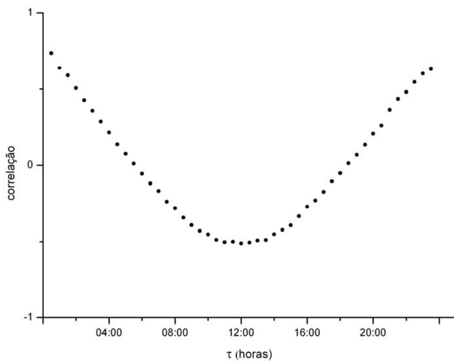
Figura 8 - Comportamento da correlação entre a serie temporal do mês fevereiro de 2001 para o fluxo de CO 2 e a mesma série defasada em \tau .
