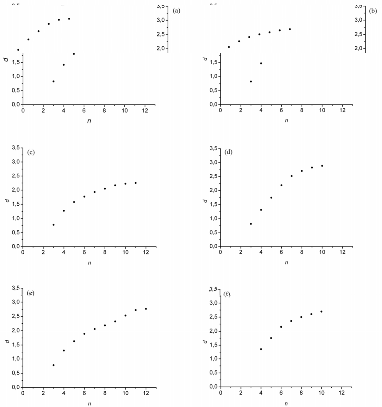
Figura 13 Comportamento da dimensão embutida, d , para concentração de H_2O , sendo: (a) fevereiro de 2001. (b) junho e julho de 2002. (c) fevereiro de 2003. (d) julho de 2005. (e) janeiro e fevereiro de 2006. (f) agosto de 2006.
