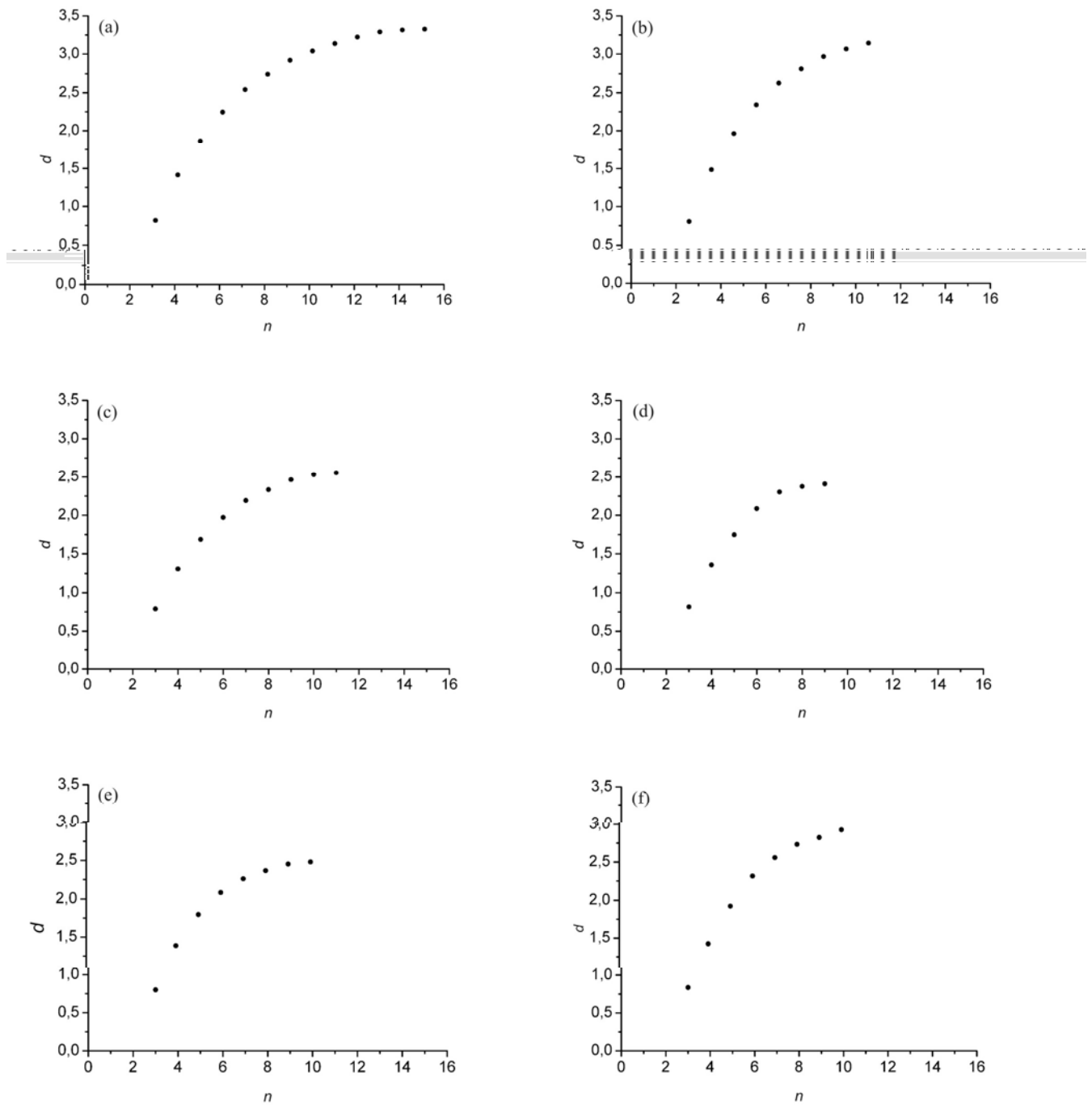
Figura 18 – Comportamento da dimensão embutida, d , para a velocidade do vento, sendo: (a) fevereiro de 2001. (b) junho e julho de 2002. (c) fevereiro de 2003. (d) julho de 2005. (e) janeiro e fevereiro de 2006. (f) agosto de 2006.
