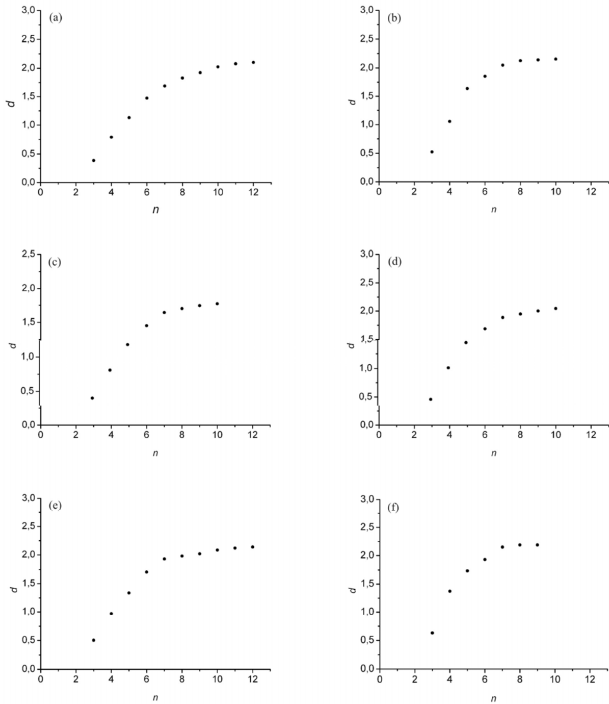
Figura 16 – comportamento da dimensão embutida para o fluxo de calor sensível, sendo: (a) fevereiro de 2001. (b) junho e julho de 2002. (c) fevereiro de 2003. (d) julho de 2005. (e) janeiro e fevereiro de 2006. (f) agosto de 2006.
