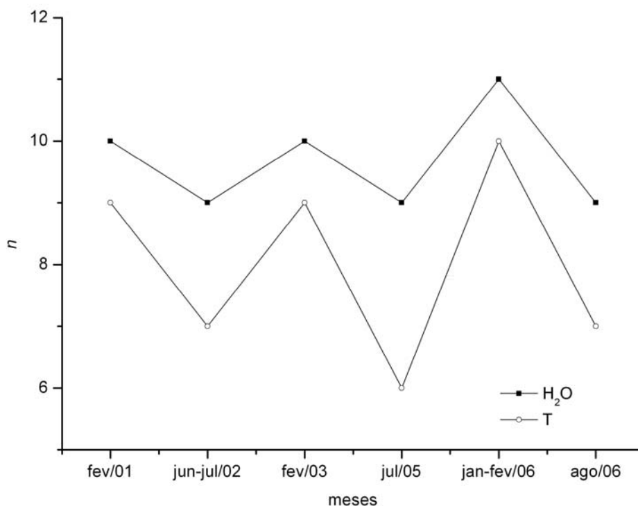
Figura 25 – Tendência sazonal da dimensionalidade mínima para a concentração H_2O e temperatura.
