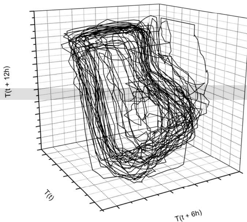
Figura 22 - Atrator da temperatura.
