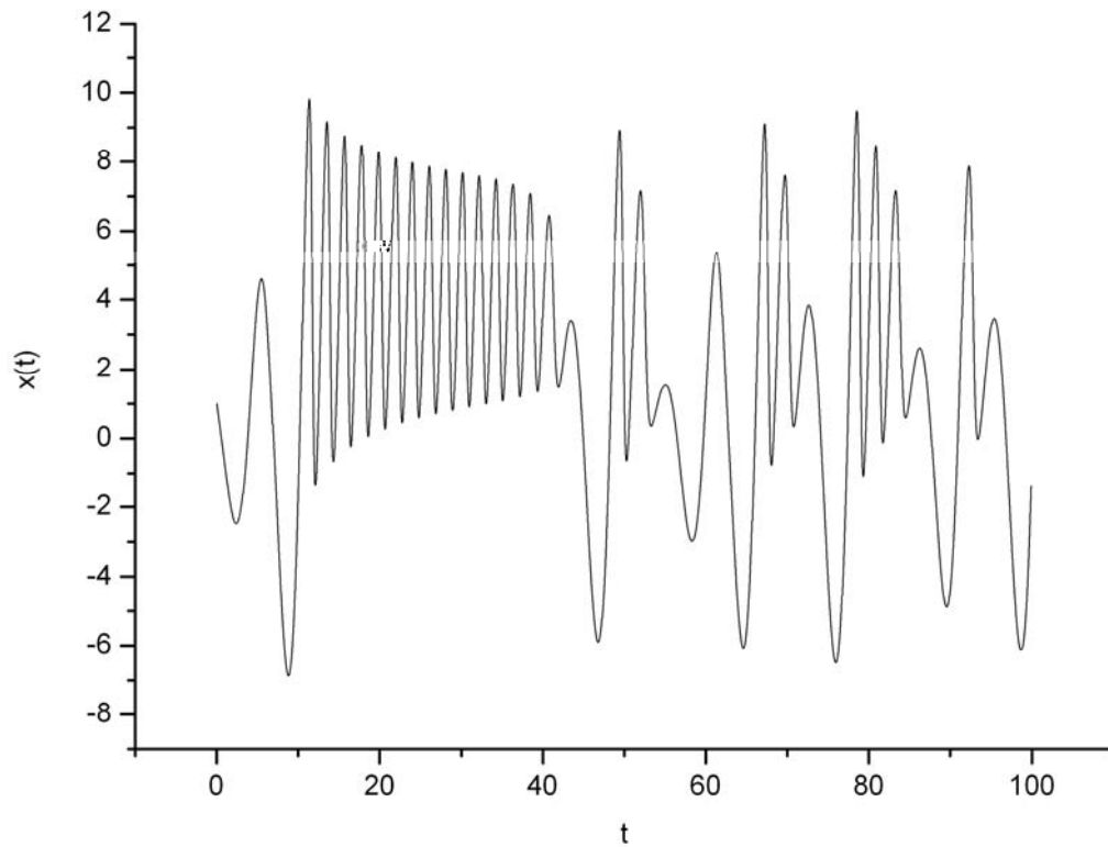
Figura 5 – Solução da componente x(t) das equações de Otto Rössler.
