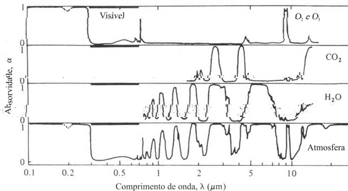
Figura 2 – Absorvidade dos principais componentes da atmosfera.
