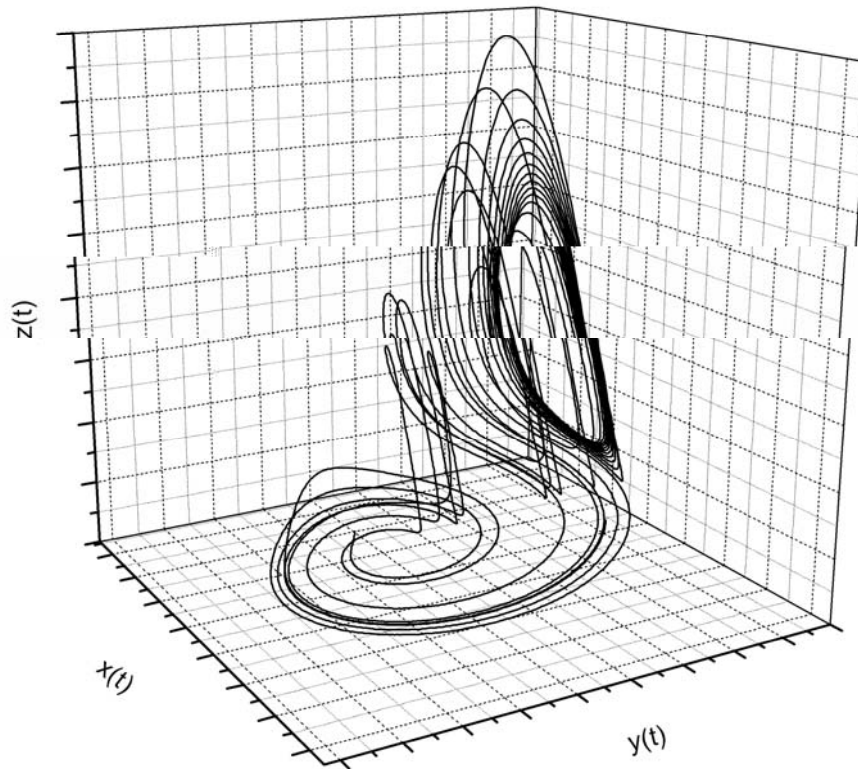
Figura 4 – Atrator caótico obtido por integração numérica do modelo de Rössler, com \sigma = 0,32 , \omega = 0,3 e \beta = 4,5 .
