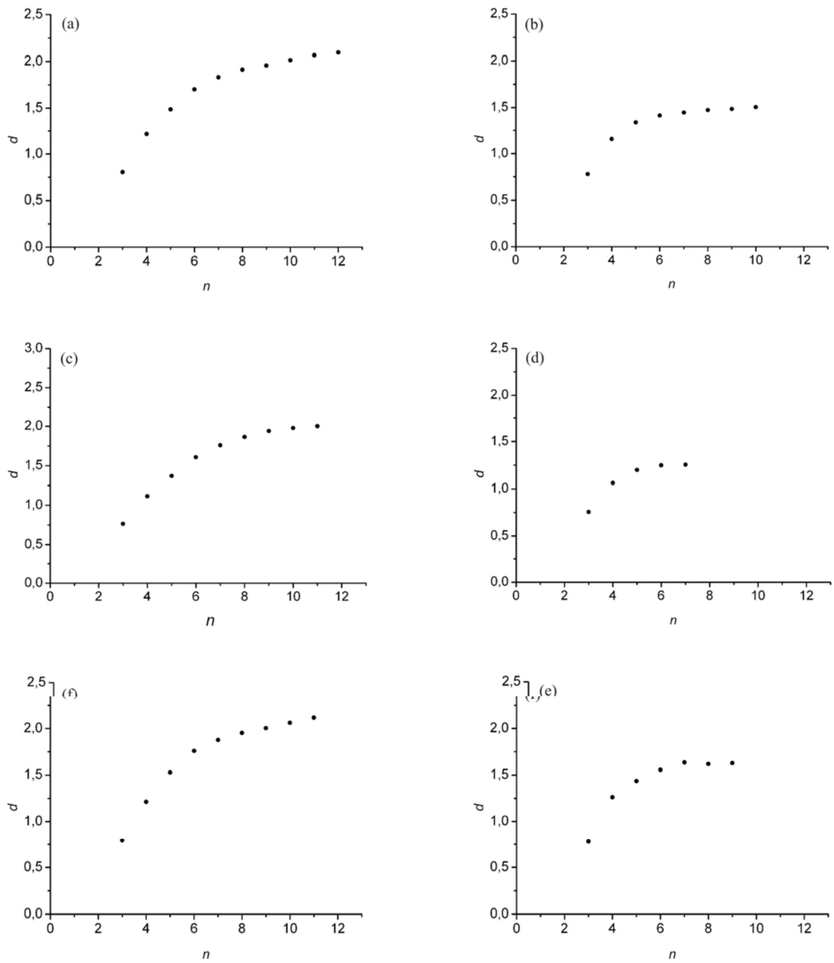
Figura 17 – Comportamento da dimensão embutida, d , para a temperatura, sendo: (a) fevereiro de 2001. (b) junho e julho de 2002. (c) fevereiro de 2003. (d) julho de 2005. (e) janeiro e fevereiro de 2006. (f) agosto de 2006.
