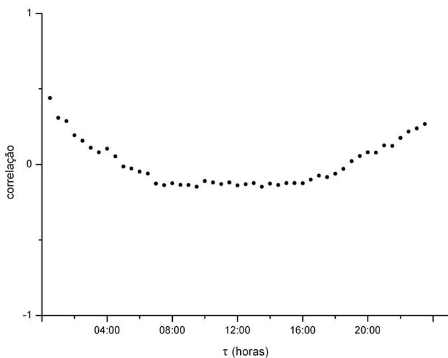
Figura 9 - Comportamento da correlação entre a serie temporal do período de julho e julho de 2002 para o fluxo de CO 2 e a mesma série defasada em \tau .
