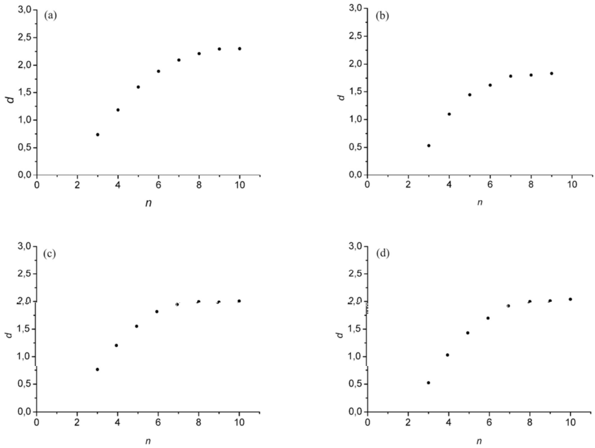
Figura 19 – Comportamento da dimensão embutida, d , para velocidade de fricção, sendo: (a) fevereiro de 2001. (b) julho de 2005. (c) janeiro e fevereiro de 2006. (d) agosto de 2006.
