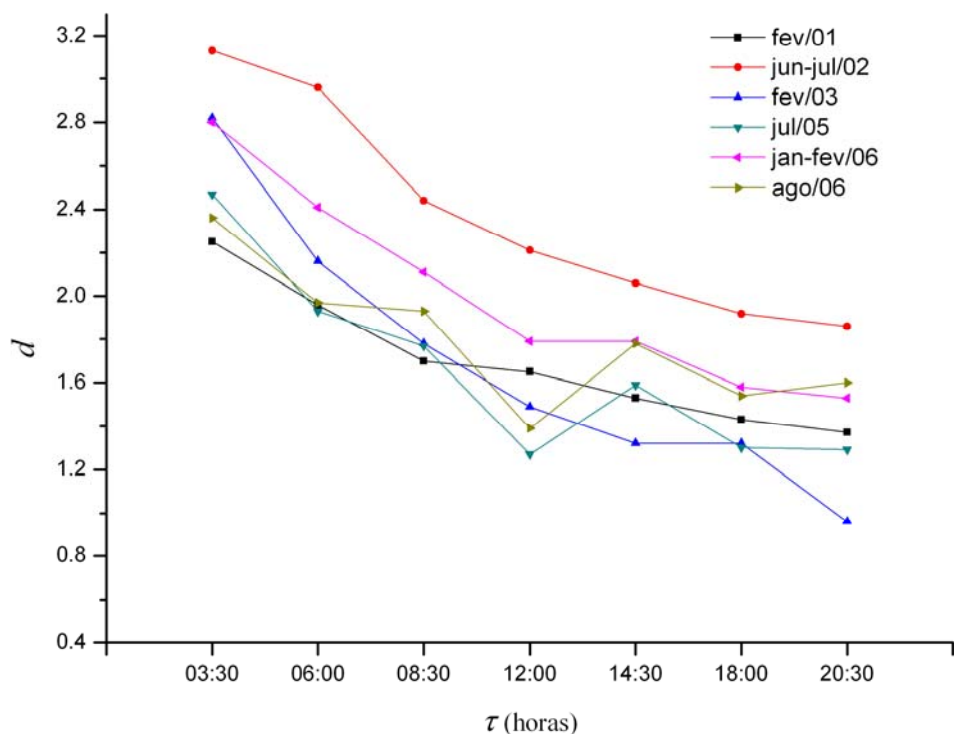
Figura 20 – Comportamento da dimensionalidade dos atratores de fluxo de CO 2 a defasagem temporal ( \tau ) para os meses de fevereiro de 2001, junho e julho de 2002, fevereiro de 2003, julho de 2005, janeiro e fevereiro de 2006, e agosto de 2006.
