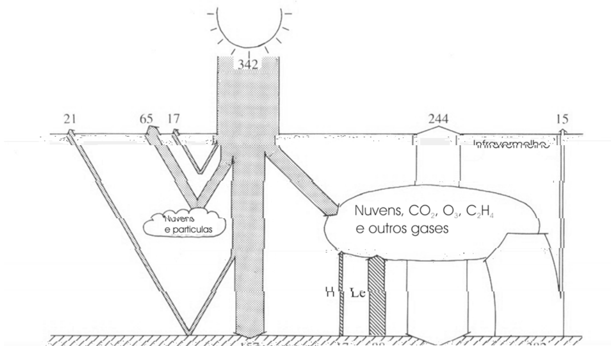
Figura 3 – Balanço de energia.
