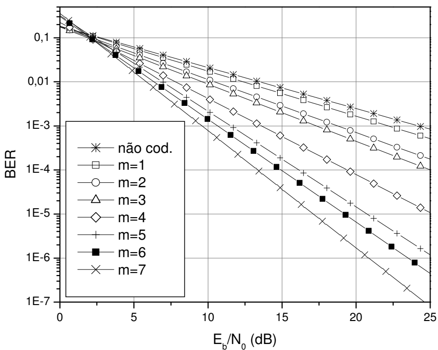
Figura 3.7: Taxa de erro de bit para dados codificados em canal Rayleigh
