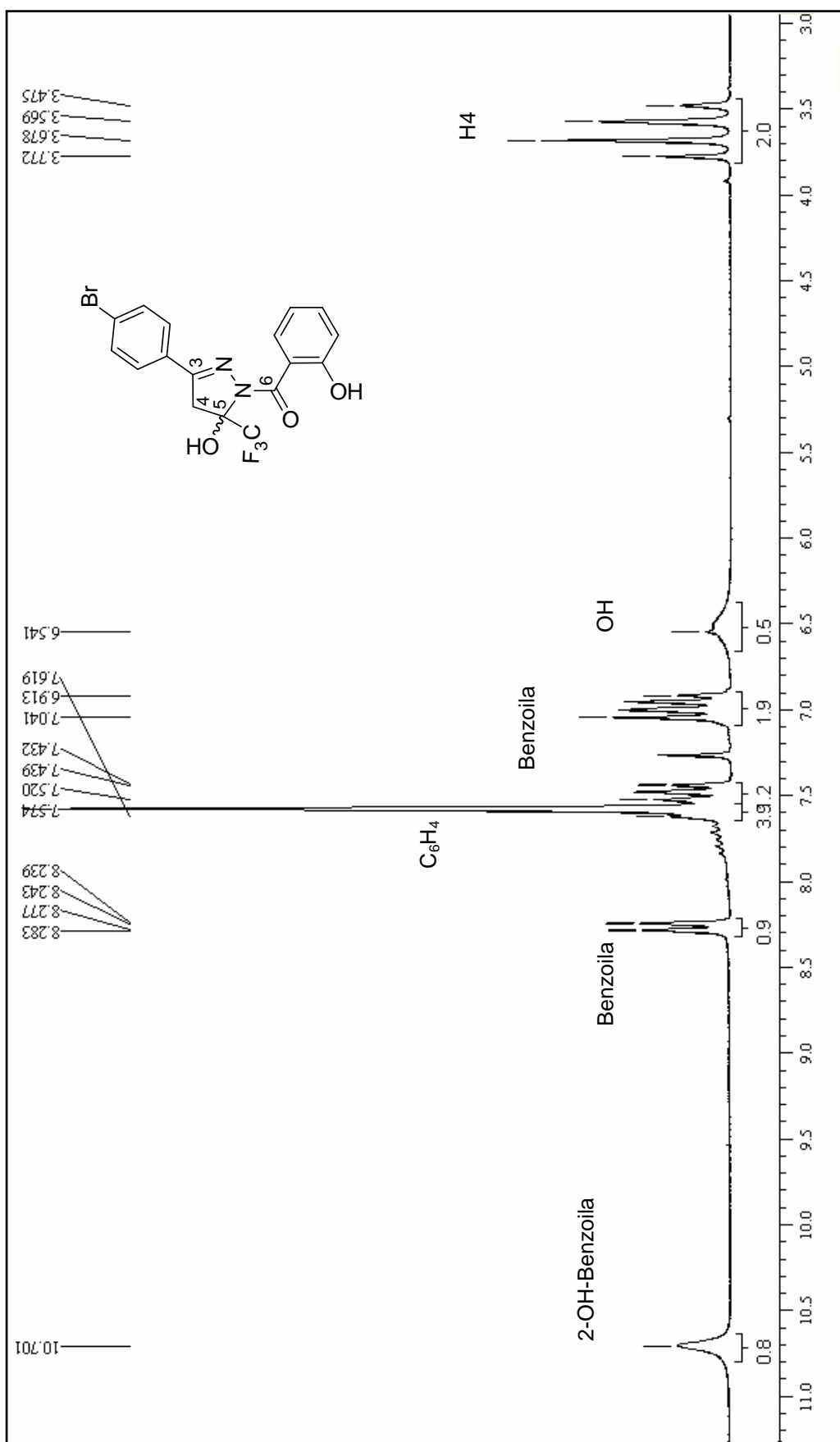
Figura 52. Espectro de RMN de ^1\text{H} do 3-(4-bromofenil)-5-hidróxi-5-trifluormetil-4,5-diidro-1H-1-(2-hidroxibenzoil)pirazol ( 7d ) em \text{CDCl}_3 .
