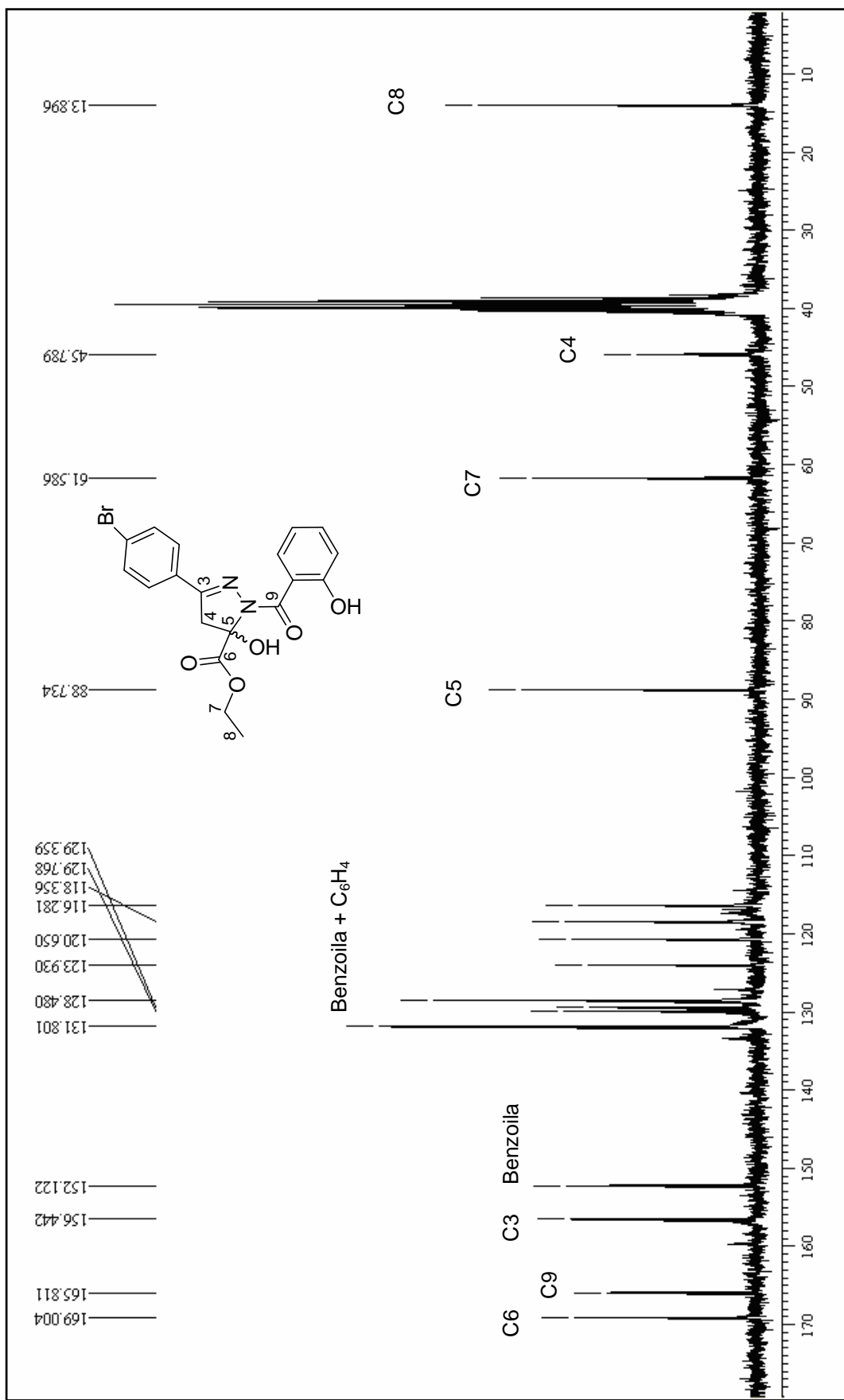
Figura 41. Espectro de RMN de ^{13}\text{C} do 5-etilcarboxilato-(4-bromofenil)-5-hidróxi-1-(2-hidróxi-benzil)-4,5-diidro-1 H -pirazol (6d) em \text{DMSO-d}_6 .
