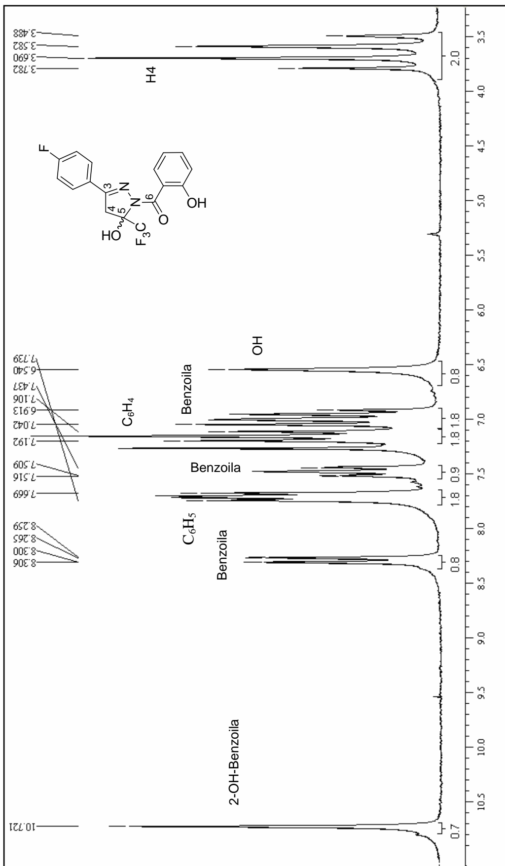
Figura 54. Espectro de RMN de ^1\text{H} do 3-(4-fluorfenil)-5-hidróxi-4,5-diidro-1H-1-(2-hidróxi-benzóil)pirazol ( 7e ) em \text{CDCl}_3 .
