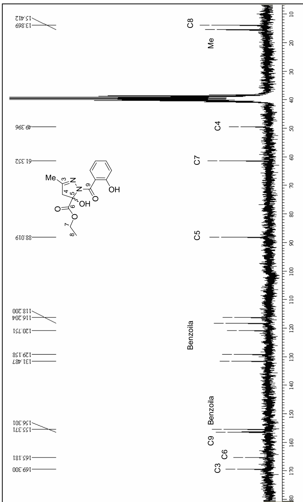
Figura 35. Espectro de RMN de 13 C do 5-etilcarboxilato-5-hidroxi-3-metil-1-(2-hidroxi-benzoi)-4,5-dihidro-1H-pirazol (6a) em DMSO-d 6 .
