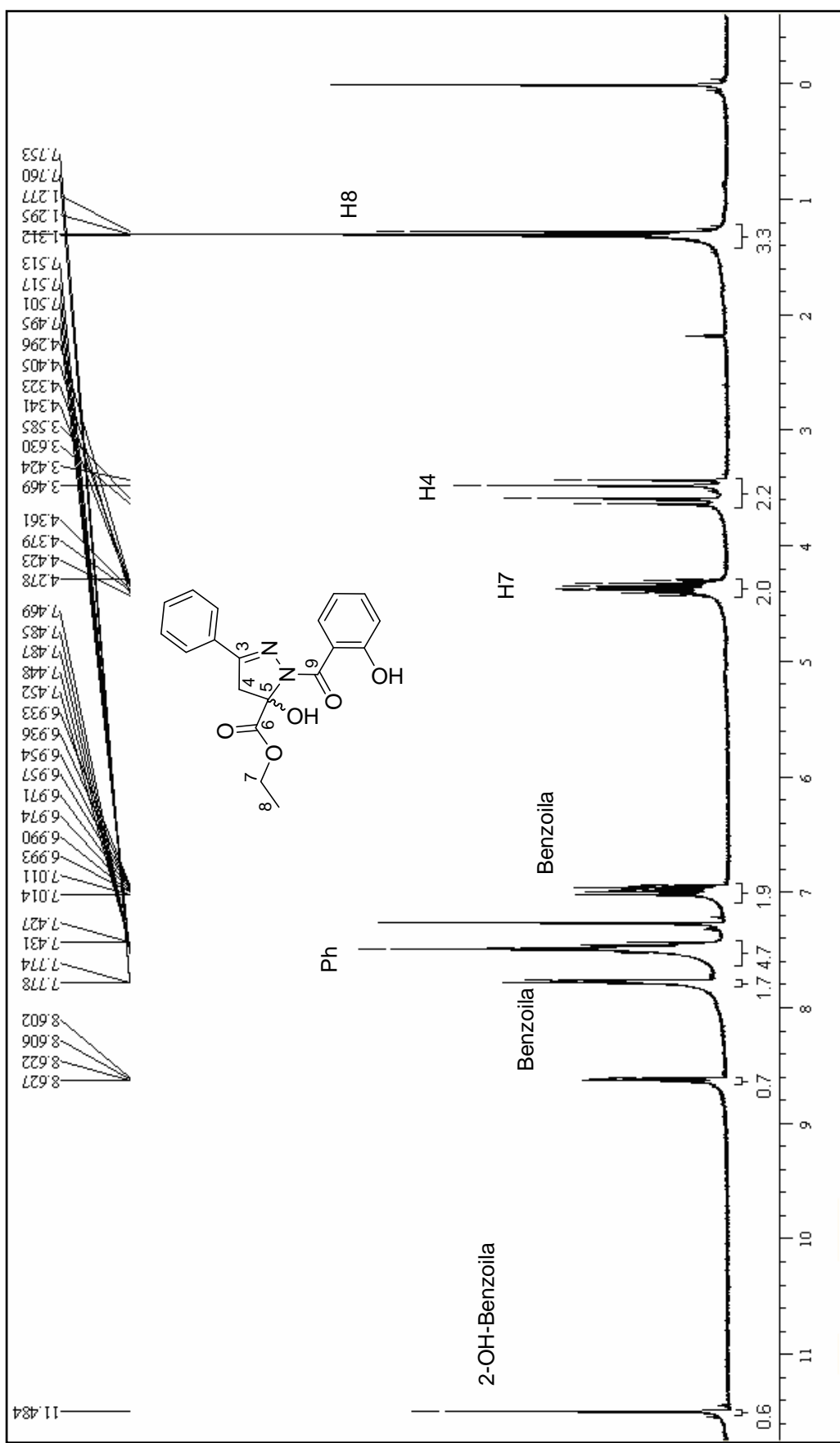
Figura 36. Espectro de RMN de ^1\text{H} do 5-etilcarboxilato-5-hidroxi-3-fenil-1-(2-hidroxi-benzoil)-4,5-didro-1H-pirazol ( 6b ) em \text{CDCl}_3 .
