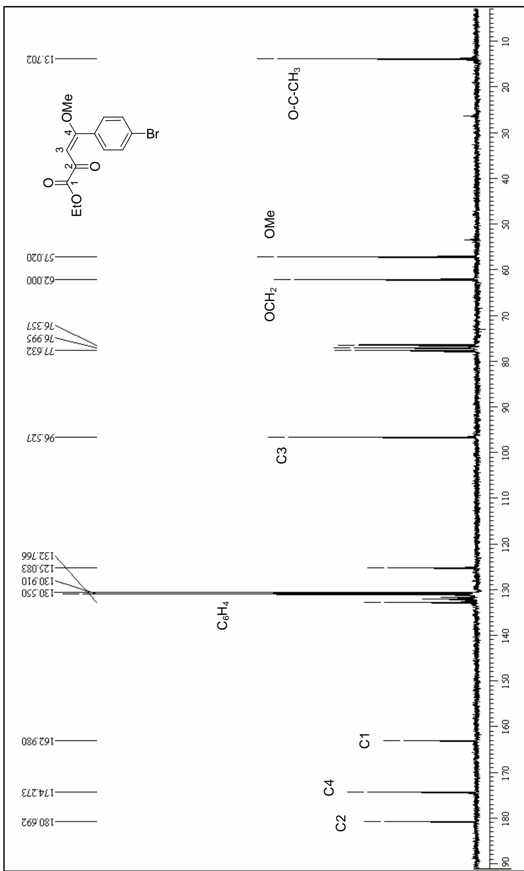
Figura 29. Espectro de RMN de ^{13}\text{C} do (E)-4-(4-bromofenil)-4-metóxi-2-oxo-3-butenolato de etila (2d) em \text{CDCl}_3 .
