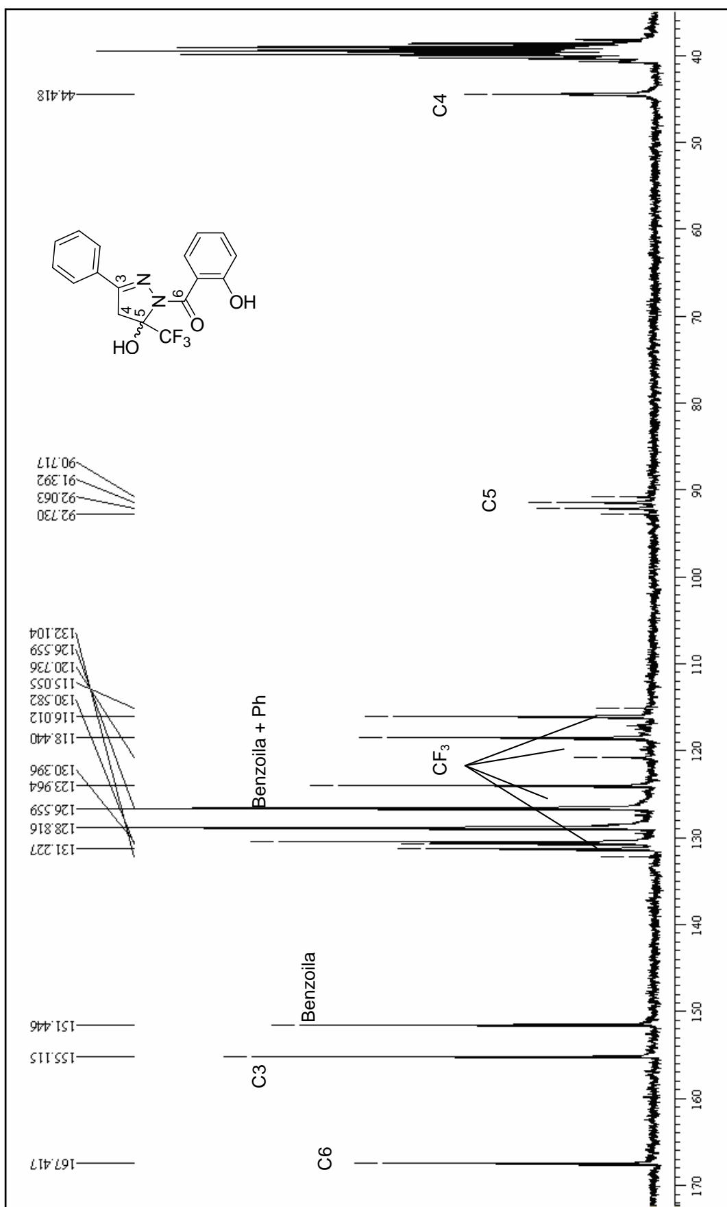
Figura 49. Espectro de RMN de ^{13}\text{C} do 5-hidróxi-3-fenil-5-trifluormetil-4,5-diidro-1H-1-(2-hidroxibenzoil)pirazol ( 7b ) em \text{DMSO-d}_6 .
