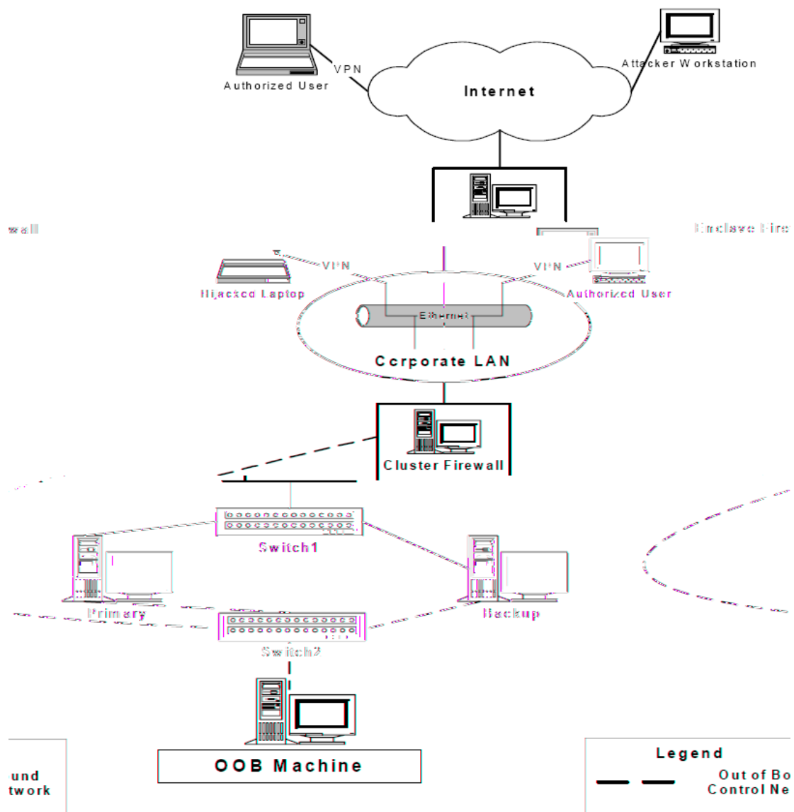
Figura 3.3 – Arquitetura do sistema HACQIT [Reynolds 2003]
