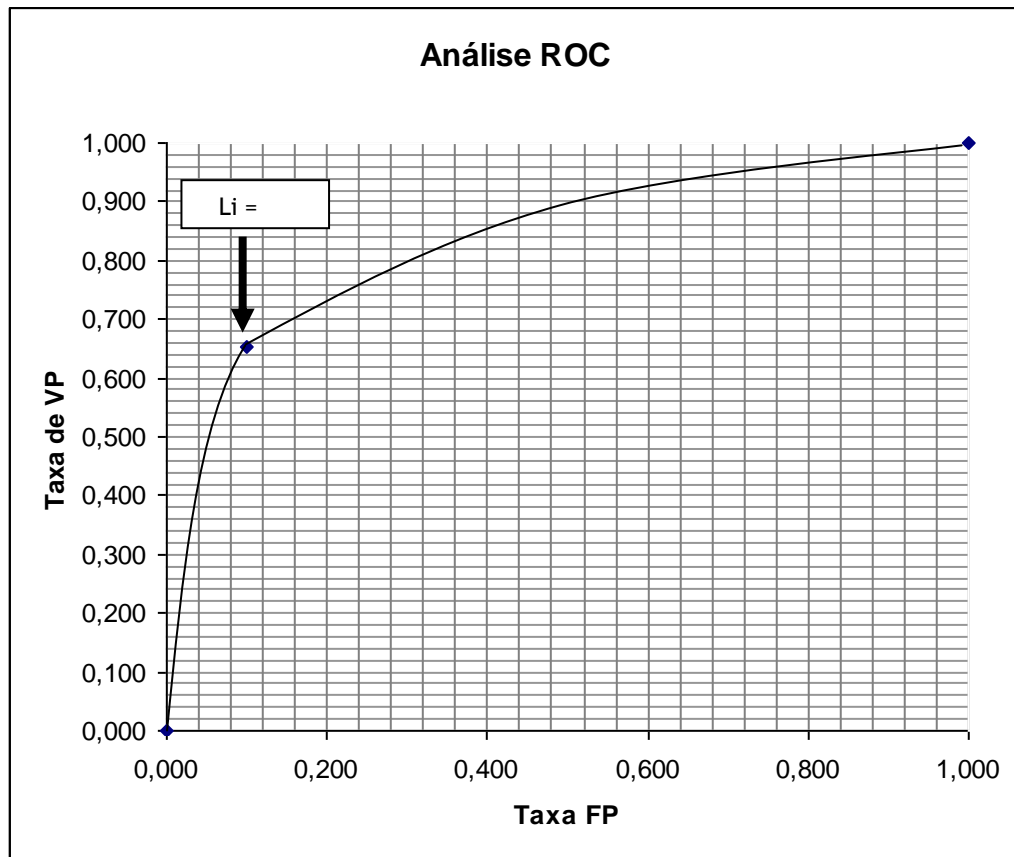
Figura E.1 – Traçado da Curva ROC - HoneyBOT
