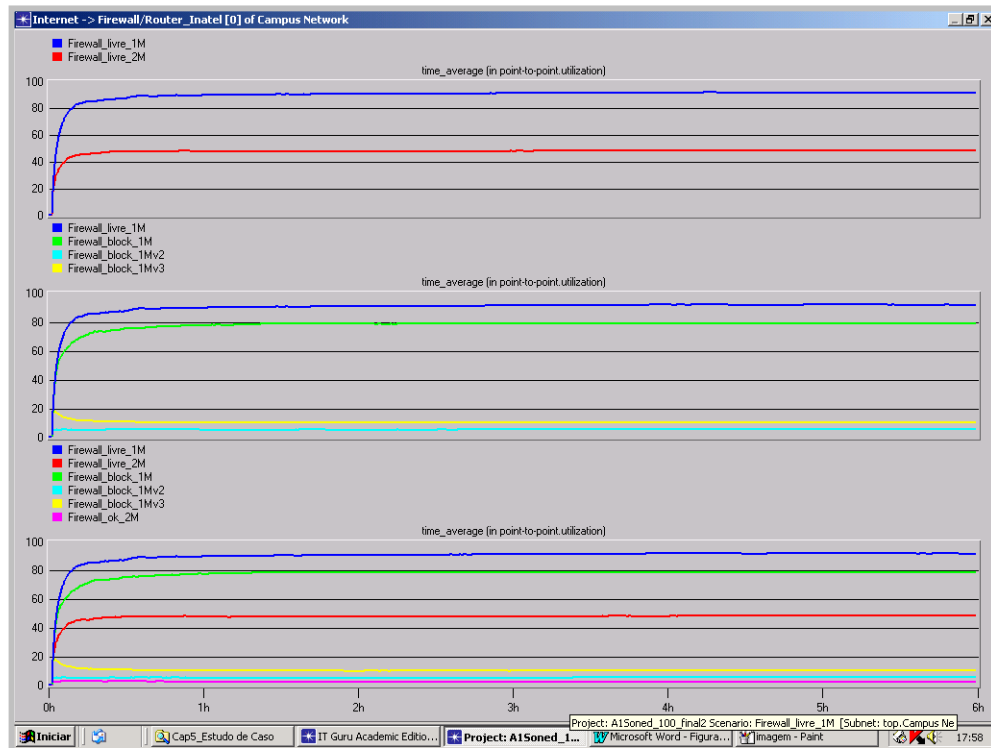
Figura C.22 - Enlace Internet→Firewall/Router_INATEL.
