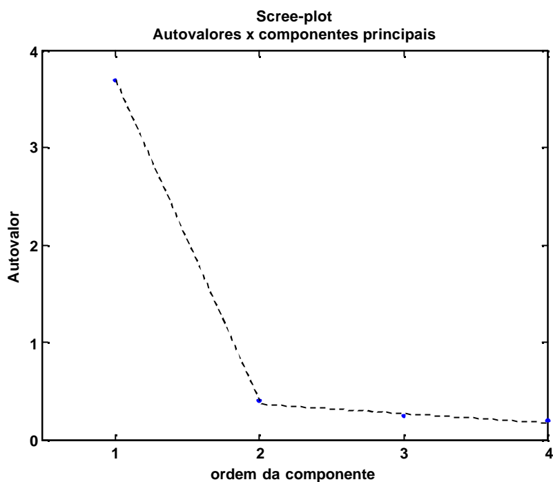
Figura 5.2 - O scree-plot mostra as componentes principais seguindo a tendência de estabilidade, aproximação de zero, dos autovalores \hat{\lambda}_i para um vetor aleatório X .
