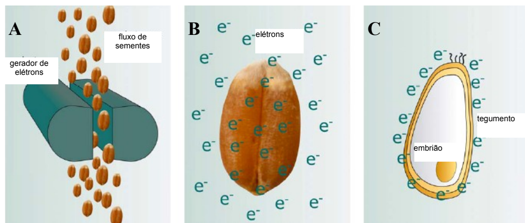
Figura 2. Sequência de tratamento com elétrons de baixa energia; (A) fluxo de sementes passando pelo gerador de elétrons, (B) camada externa (tegumento) da semente tratada com elétrons (C) semente tratada sem dano ao embrião (modificado de e - ventus , 2005).
