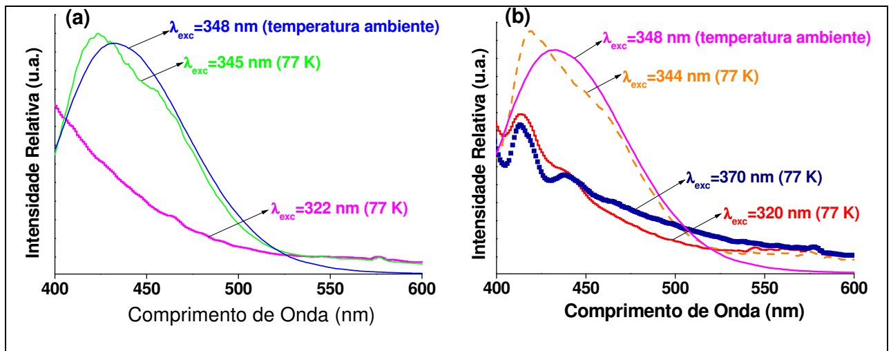
Figura 47: Espectros de emissão (diferentes \lambda_{exc} , de acordo com os espectros de excitação) do composto Gd_2SiO_5:Ce(1,0\%) sintetizados pelos métodos (a) sol-gel convencional e (b) sol-gel modificado usando PVA como polímero precursor, a temperatura ambiente e a 77 K.
