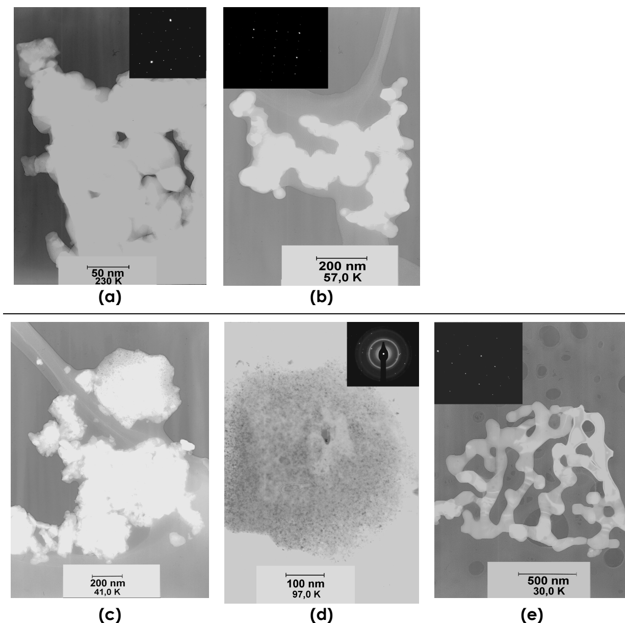
Figura 45: MET, imagens de campo claro e escuro (somente (d)), dos compostos \text{Lu}_2\text{SiO}_5:\text{Tm}(1,0\%) , (a) e (b), e \text{Y}_2\text{SiO}_5:\text{Tm}(1,0\%) (c) a (e), calcinados a 1100^\circ\text{C} . (a), (c) e (d) são fotos dos compostos obtidos pelo método sol-gel convencional e (b), e (e) pelo método sol-gel modificado usando PVA como polímero precursor. Os quadros superiores representam a difração de elétrons de uma área selecionada (SAED- selected area diffraction).
