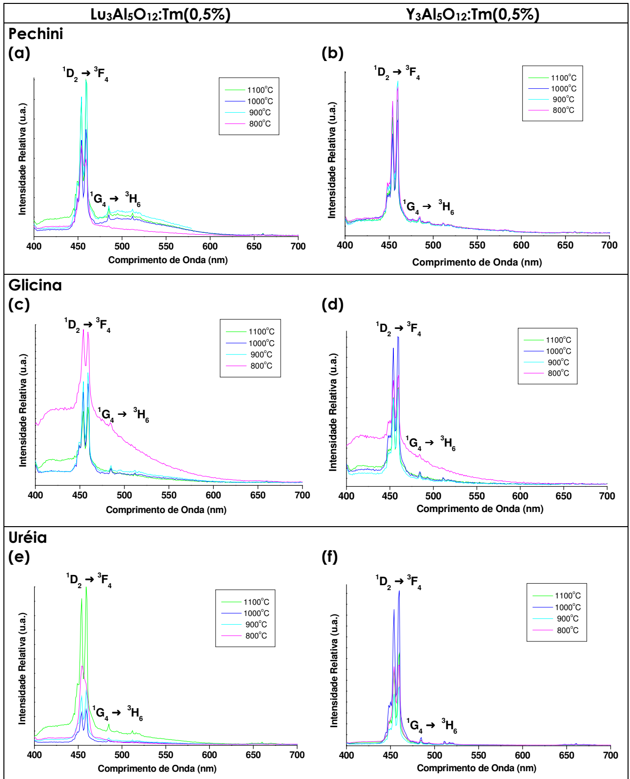
Figura 28: Espectros de emissão do íon \text{Tm}^{3+} ( \lambda_{\text{ex}} = 355 \text{ nm} ) das amostras \text{Lu}_3\text{Al}_5\text{O}_{12}:\text{Tm}(0,5\%) ((a), (c) e (e)) e \text{Y}_3\text{Al}_5\text{O}_{12}:\text{Tm}(0,5\%) ((b), (d) e (f)) preparadas através dos métodos Pechini ou combustão e calcinadas de 800 a 1100°C. f_{\text{ex}} = f_{\text{em}} que resultam em largura de banda a \frac{1}{2} altura = 1 nm; temperatura ambiente.
