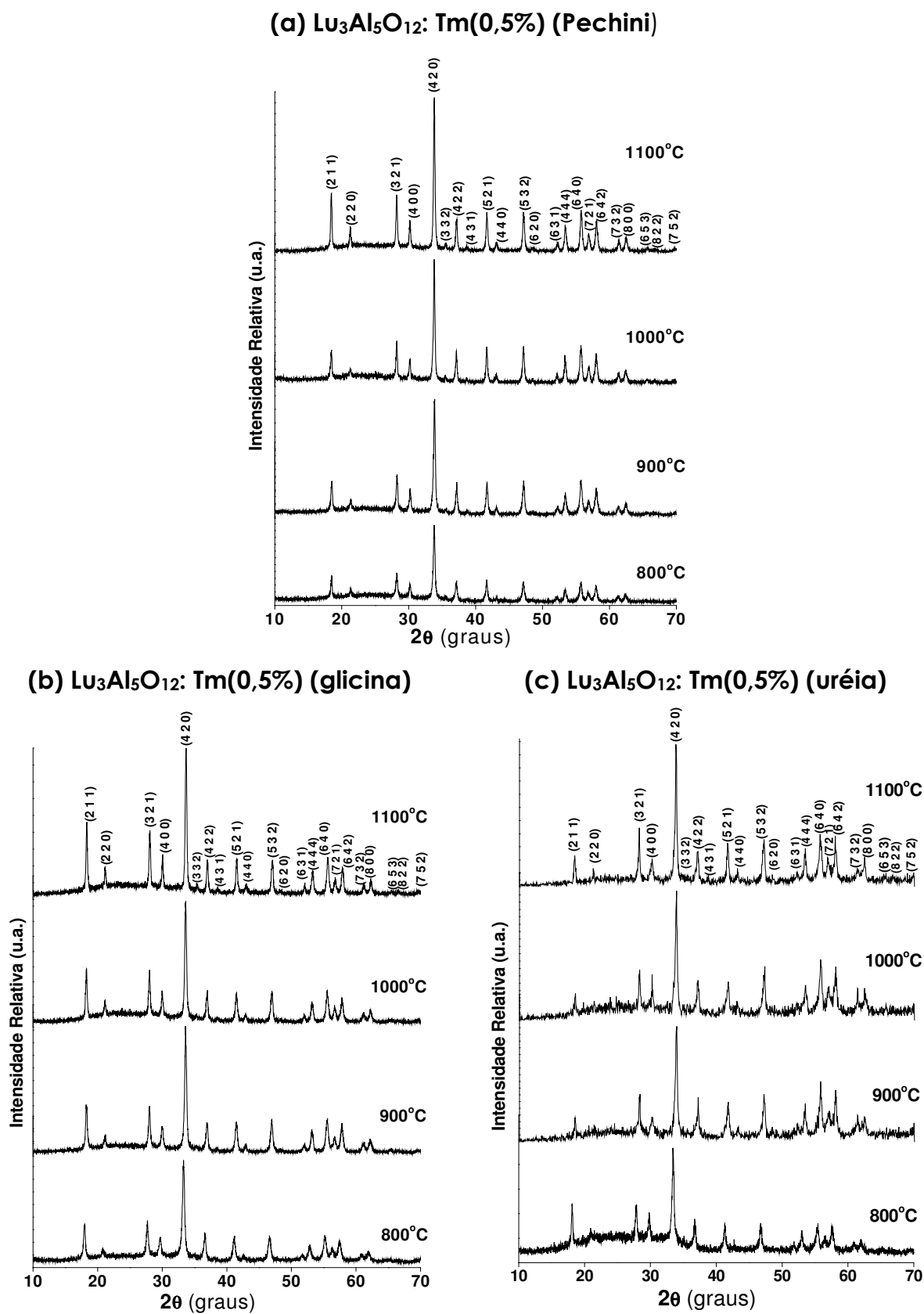
Figura 15: Difratogramas de raios X do pó do composto \text{Lu}_3\text{Al}_5\text{O}_{12}:\text{Tm}(0,5\%) preparado pelos métodos Pechini (a) e combustão com glicina (b) ou uréia (c) , calcinado nas temperaturas de 800 a 1100°C.
