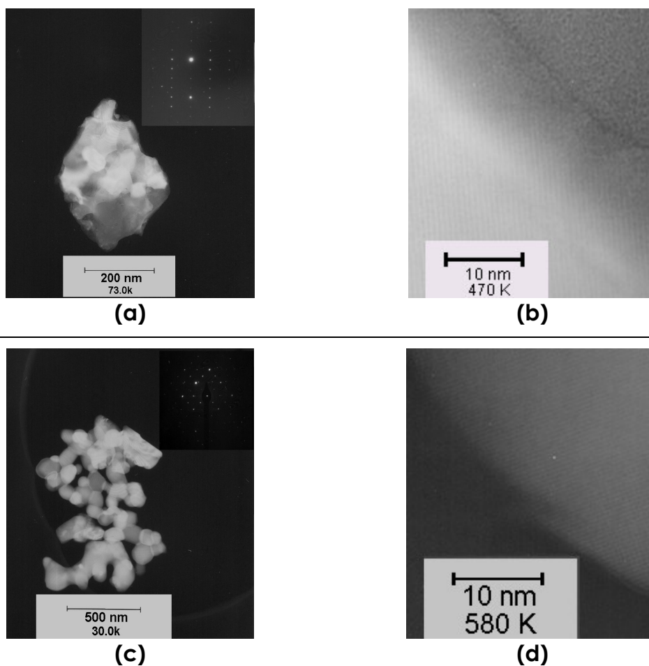
Figura 42: MET, imagens de campo claro, dos compostos Gd_2SiO_5:Ce(1,0\%) sintetizados (calcinaados à 1100^\circ C ): (a) e (b) pelo método sol-gel convencional; (c) e (d) pelo método sol-gel modificado usando um polímero precursor. (b) e (d) representam uma visão detalhada de MET em alta resolução com 470 e 580 K de magnitude, respectivamente. Em (a) e (c) , os quadros superiores à direita representam a difração de elétrons de uma área selecionada (SAED-selected area diffraction).
