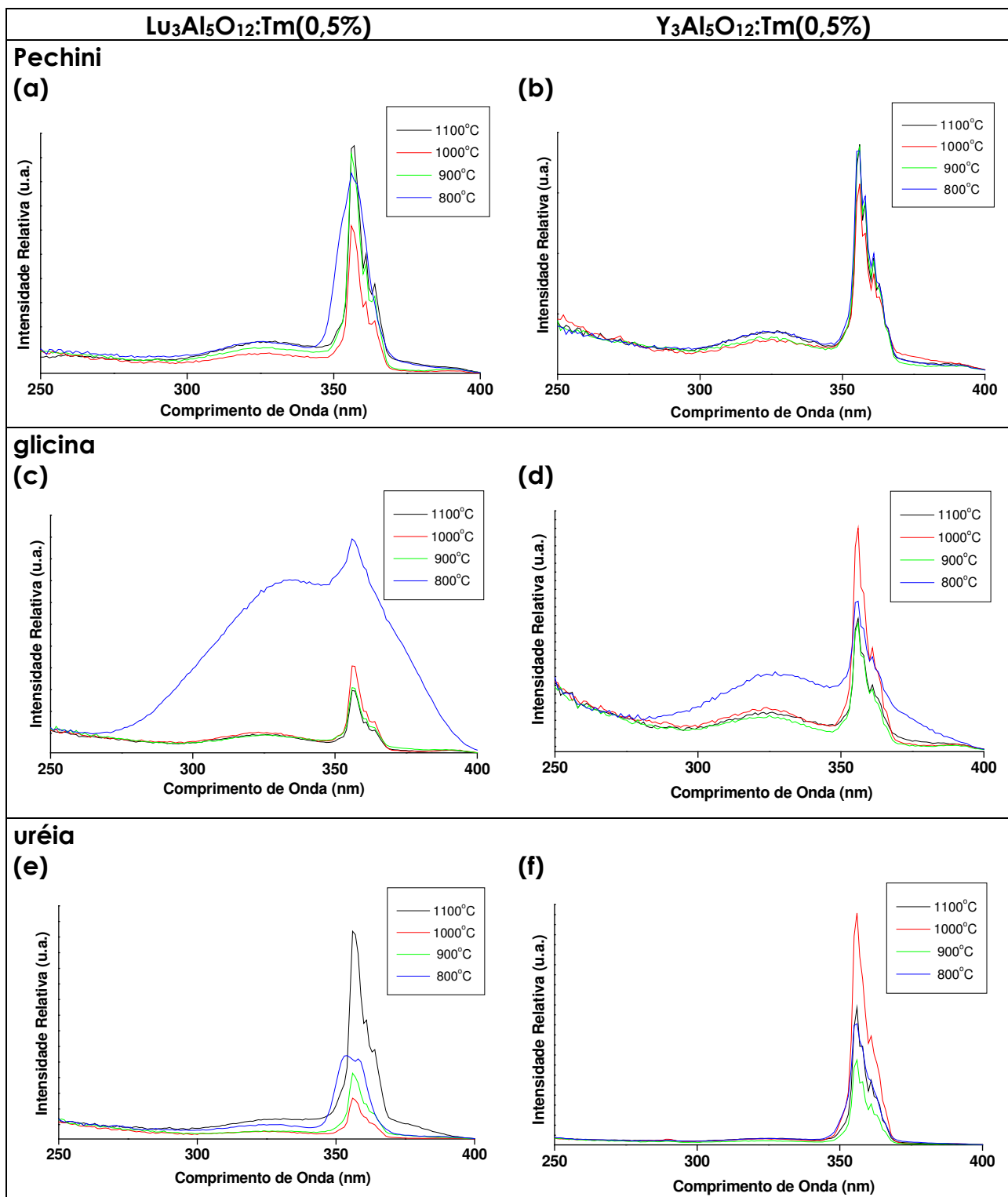
Figura 27: Espectros de excitação ( \lambda_{em} = 460 nm) corrigidos das amostras \text{Lu}_3\text{Al}_5\text{O}_{12}:\text{Tm}(0,5\%) ((a), (c) e (e)) e \text{Y}_3\text{Al}_5\text{O}_{12}:\text{Tm}(0,5\%) ((b), (d) e (f)) preparadas através dos métodos Pechini e combustão e calcinadas de 800 a 1100°C. f_{ex} = f_{em} que resultam em largura de banda a \frac{1}{2} altura = 1 nm; temperatura ambiente.
