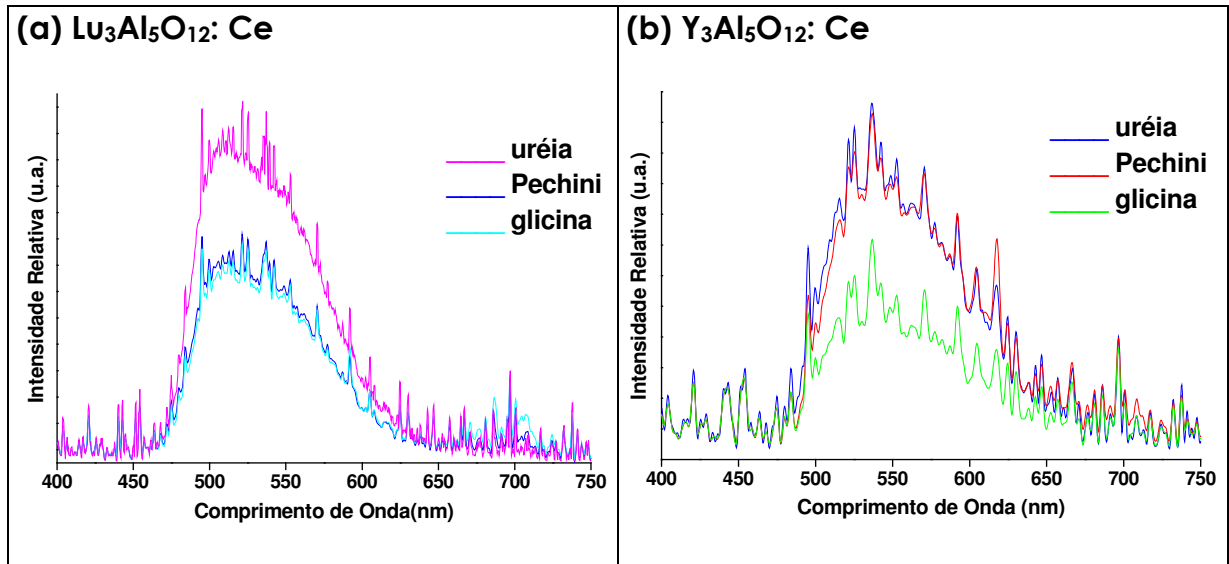
Figura 57: Espectros de emissão do íon Ce 3+ nas matrizes Lu 3 Al 5 O 12 e Y 3 Al 5 O 12 , sob excitação de raios X (radiação K \alpha -Cu, 8.050 keV, 40 kV). Compostos preparados por Pechini ou combustão, calcinados a 1100°C.
