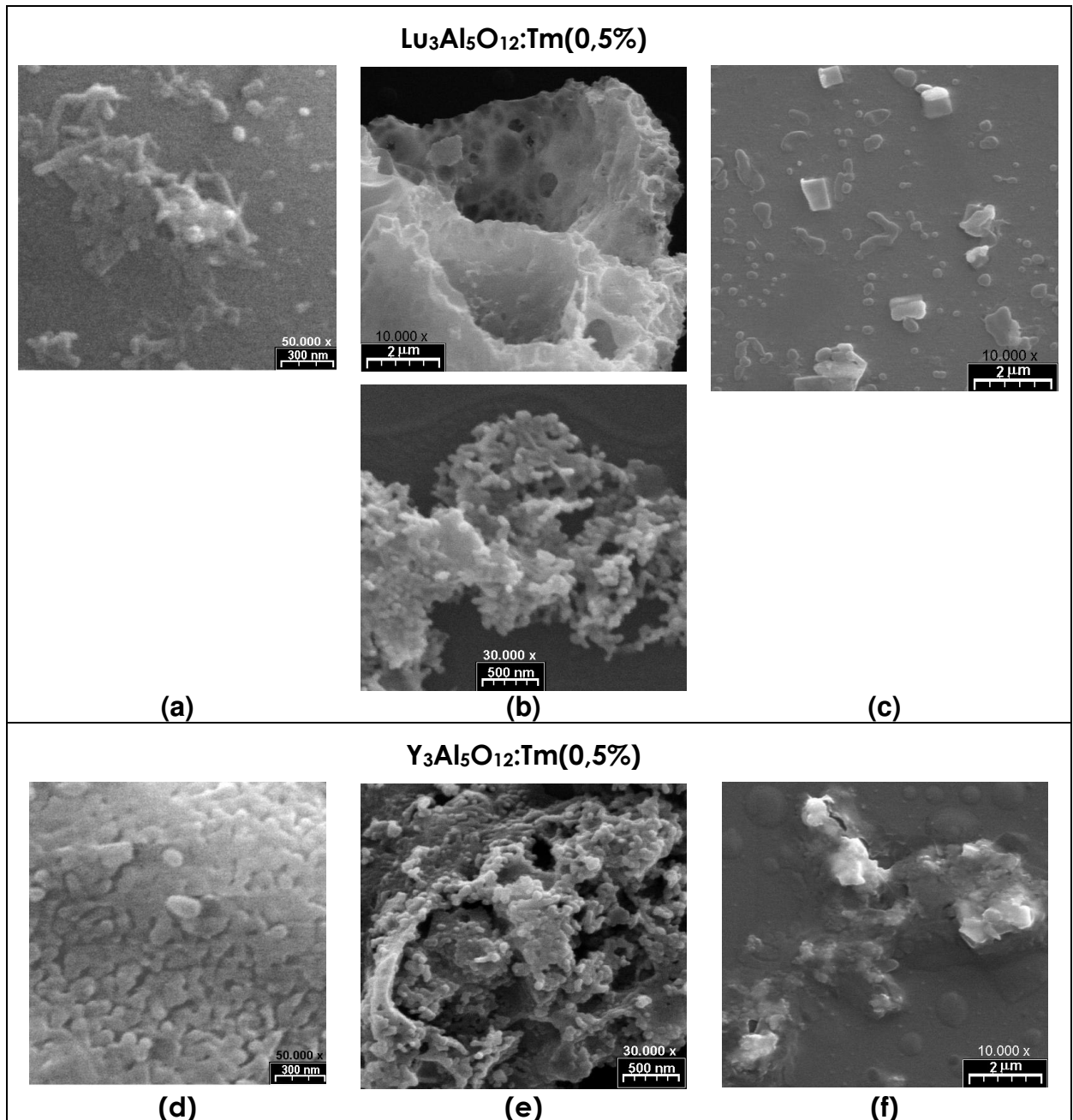
Figura 19: MEV de amostras de aluminatos de lutécio ou ítrio dopadas com cério obtidas após calcinação a 1100°C. Lu 3 Al 5 O 12 :Tm(0,5%): preparado por (a) Pechini; (b) combustão com glicina e com (c) uréia. Y 3 Al 5 O 12 :Tm(0,5%): preparado por (d) Pechini; (e) combustão com glicina e com (f) uréia.
