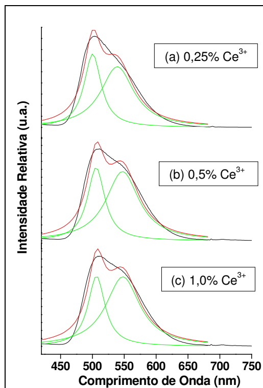
Figura 25: Curvas de emissão do \text{Ce}^{3+} na amostra \text{Lu}_3\text{Al}_5\text{O}_{12} , preparadas pelo método Pechini, dopadas com 0,25, 0,5 e 1,0% de \text{Ce}^{3+} analisadas através do programa ORIGIN 5.0 ® . (—) experimental; (—) decomposição utilizando modelo Lorentziano; e (—) ajuste final calculado.
