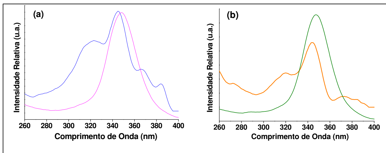
Figura 46: Espectros de excitação ( \lambda_{\text{em}} = 429 \text{ nm} ) do \text{Gd}_2\text{SiO}_5:\text{Ce}(1,0\%) sintetizado pelos métodos (a) sol-gel convencional e (b) sol-gel modificado usando PVA como polímero precursor. (—) e (—) a temperatura ambiente; (—) e (—) a 77 K.
