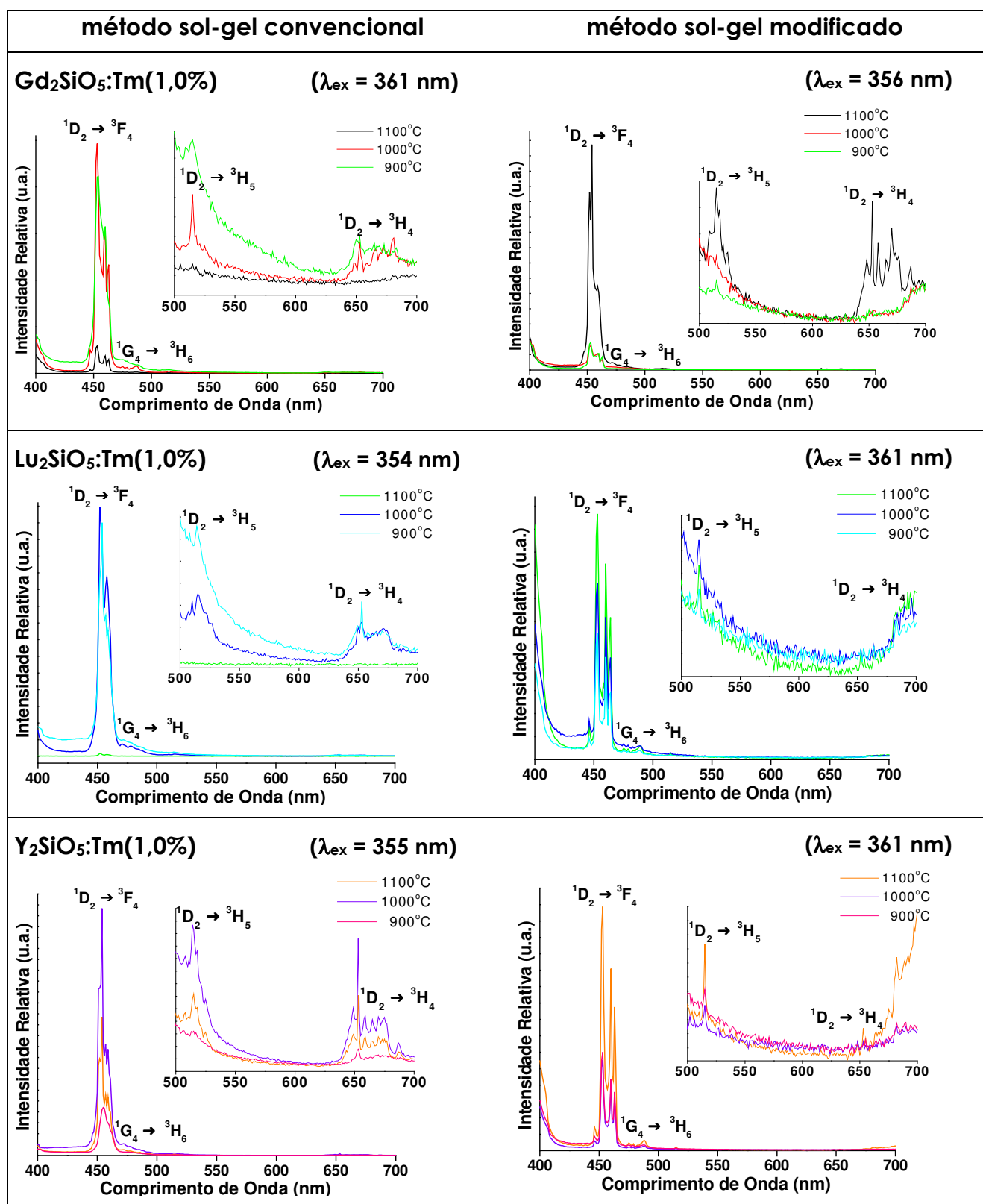
Figura 54: Espectros de emissão das amostras Gd 2 SiO 5 :Tm(1,0%), (a) e (b); Lu 2 SiO 5 :Tm(1,0%), (c) e (d); Y 2 SiO 5 :Tm(1,0%),(e) e (f), sintetizados pelos métodos sol-gel convencional (a), (c) e (e) e sol-gel modificado usando PVA como polímero precursor (b), (d) e (f), calcinadas de 900 a 1100°C. f_{ex} = f_{em} que resultam em largura de banda de emissão de 1 nm; 25°C .
