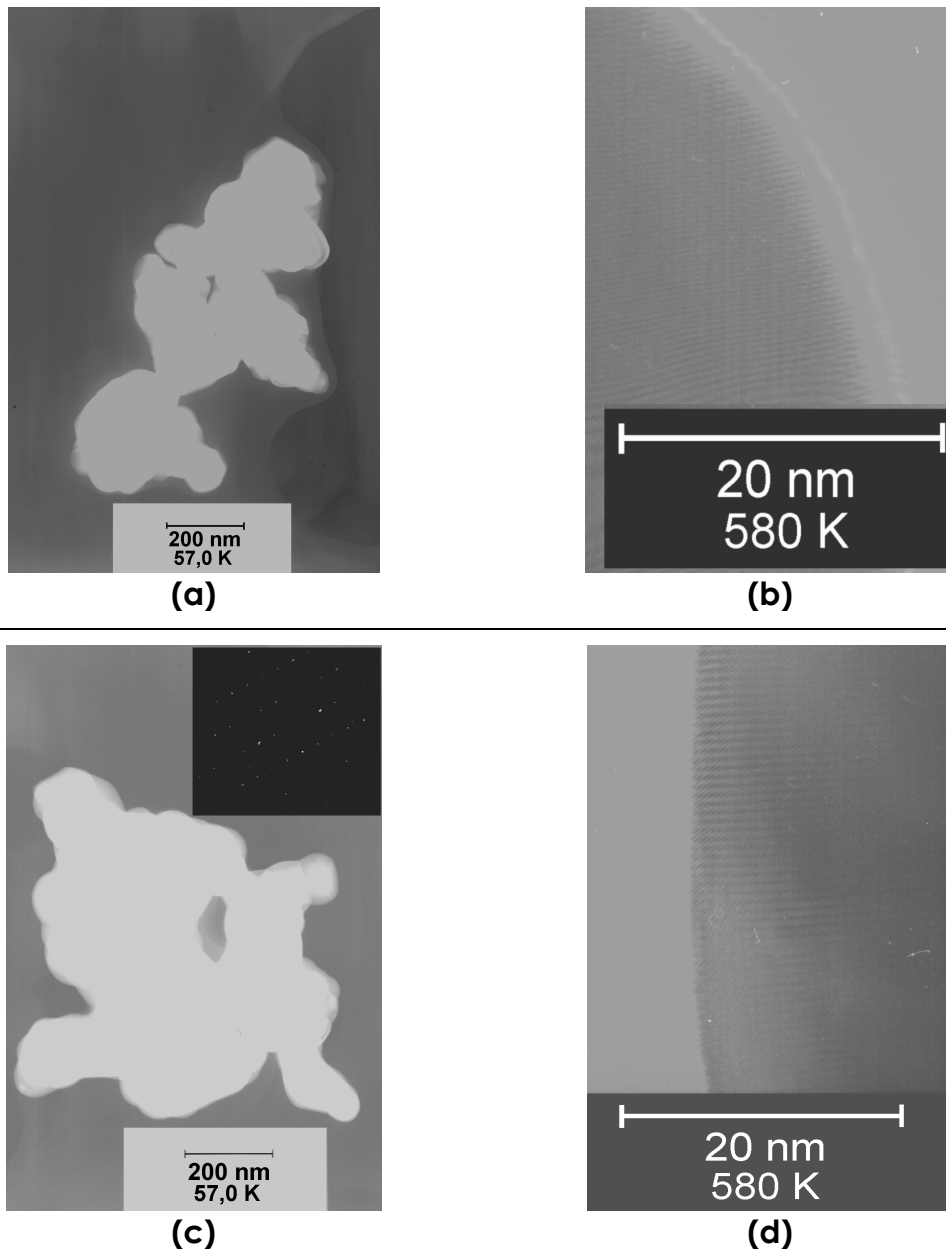
Figura 44: MET, imagens de campo claro, dos compostos Gd_2SiO_5:Tm(1,0\%) sintetizados: (a) e (b) pelo método sol-gel convencional; (c) e (d) pelo método sol-gel modificado usando um polímero precursor. Amostras calcinadas à 1100^\circ C . (b) e (d) representam uma visão detalhada de MET em alta resolução com 580 K de magnitude. Em (c) , o quadro superior à direita representa a difração de elétrons de uma área selecionada (SAED- selected area diffraction).
