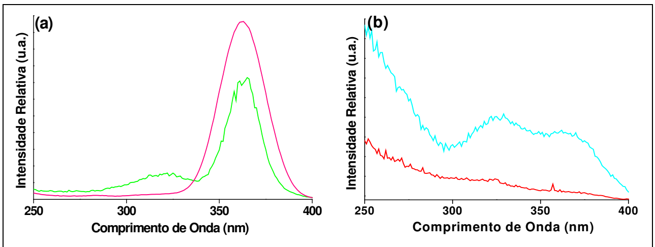
Figura 49: Espectros de excitação ( \lambda_{em} = 442 nm) do \text{Y}_2\text{SiO}_5:\text{Ce}(1,0\%) sintetizado pelos métodos (a) sol-gel convencional e (b) sol-gel modificado usando PVA como polímero precursor, a temperatura ambiente. (—) e (—) a temperatura ambiente; (—) e (—) a 77 K.
