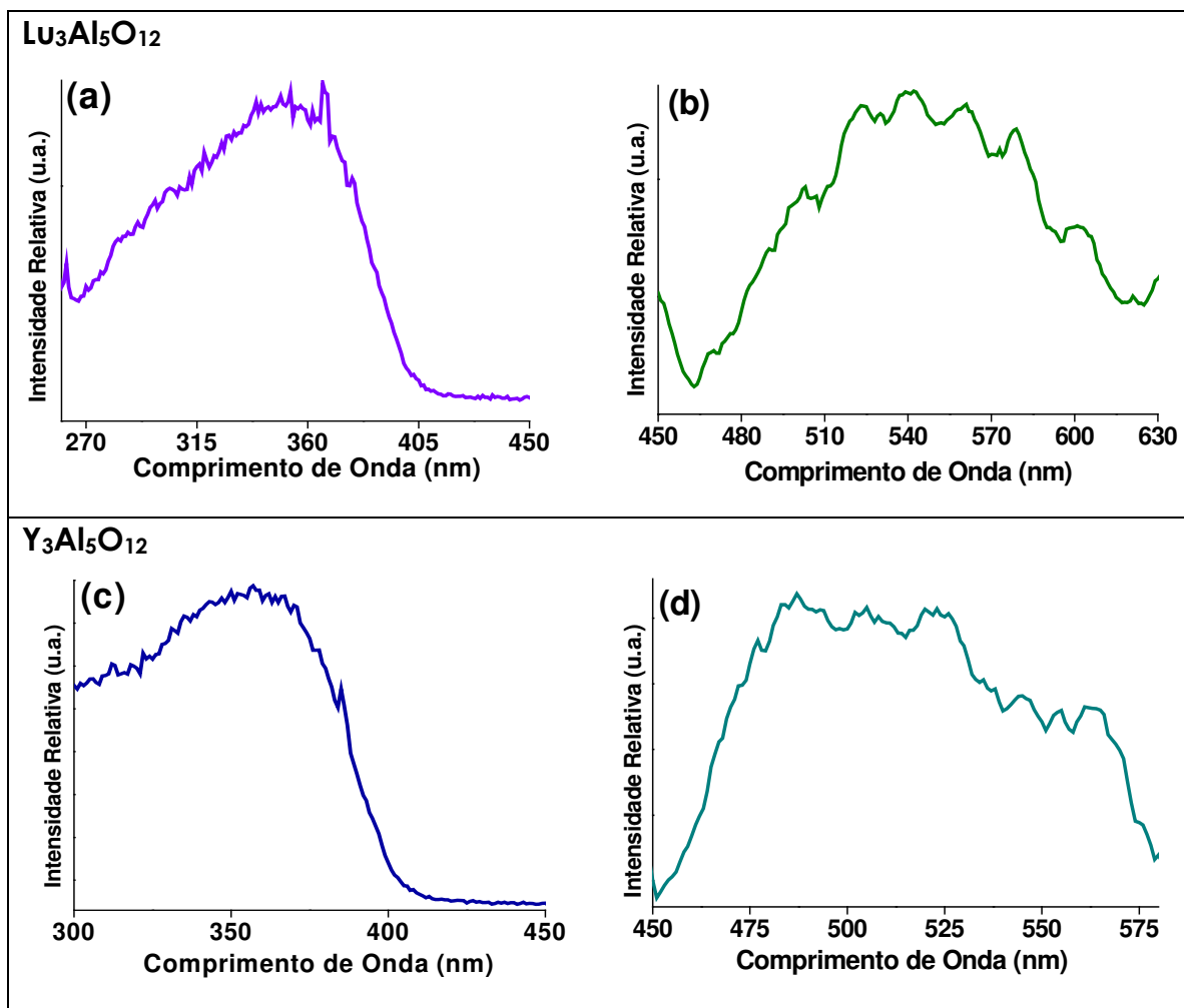
Figura 24: Espectros de excitação e emissão das matrizes sem dopantes, sintetizadas pelo método Pechini e calcinadas a 1000°C. (a) e (c) , espectros de excitação, respectivamente para \text{Lu}_3\text{Al}_5\text{O}_{12} , \lambda_{\text{em}} = 540 nm, e \text{Y}_3\text{Al}_5\text{O}_{12} , \lambda_{\text{em}} = 490 nm. (b) e (d) , espectros de emissão, respectivamente para \text{Lu}_3\text{Al}_5\text{O}_{12} , \lambda_{\text{ex}} = 352 nm, e \text{Y}_3\text{Al}_5\text{O}_{12} , \lambda_{\text{ex}} = 357 nm. f_{\text{ex}} = f_{\text{em}} que resultam em largura de banda a \frac{1}{2} altura = 1 nm; temperatura ambiente.
