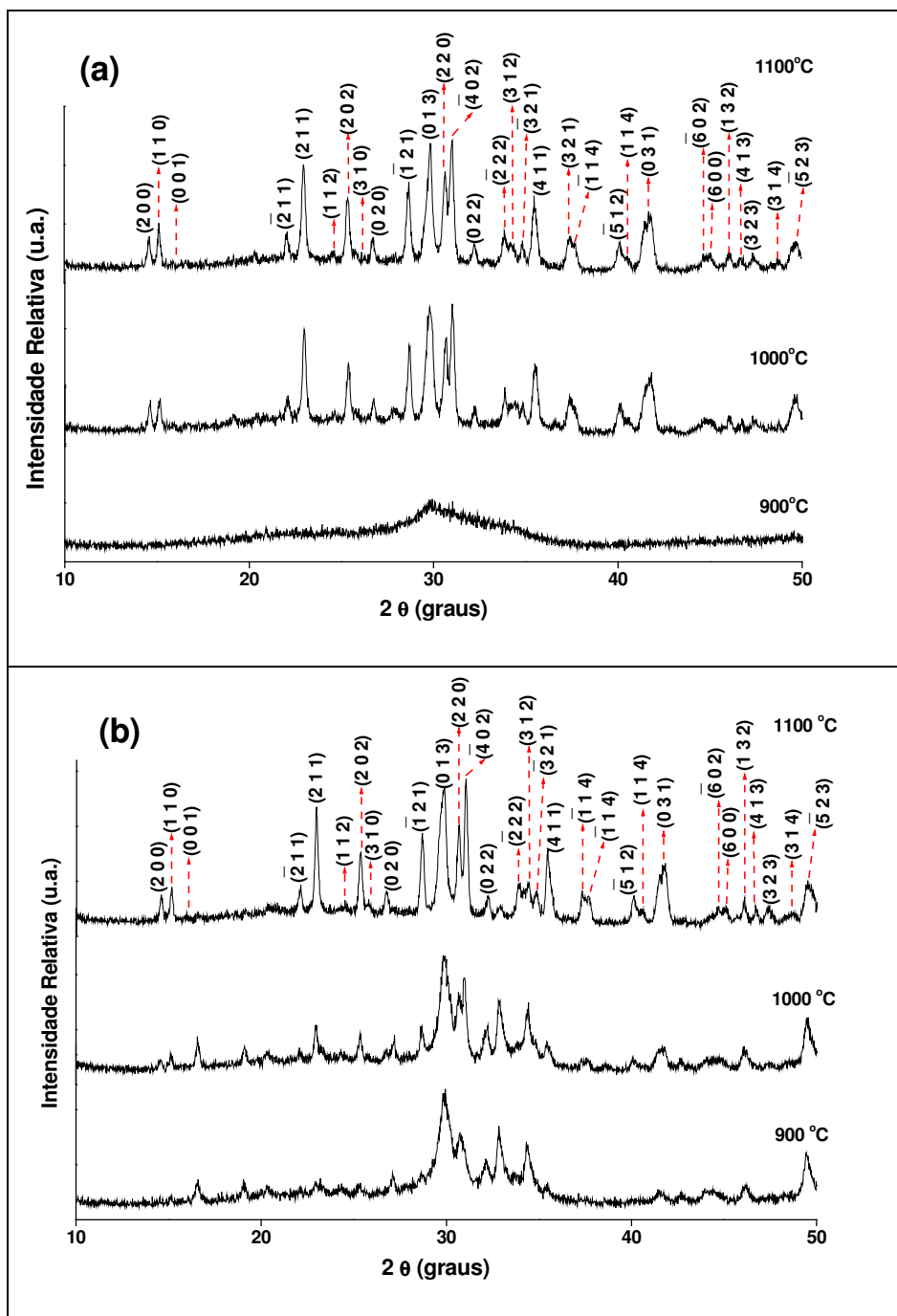
Figura 35: Difratomogramas de raios X das amostras \text{Lu}_2\text{SiO}_5:\text{Ce}(1,0\%) sintetizadas pelos métodos (a) sol-gel convencional e (b) sol-gel modificado usando PVA como polímero precursor e calcinadas nas diferentes temperaturas.
