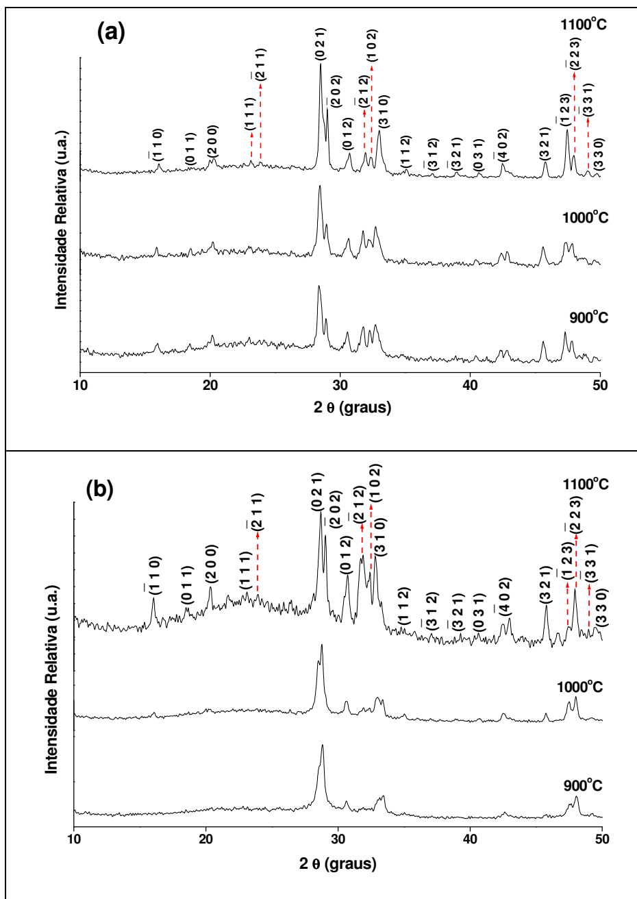
Figura 33: Difratogramas de raios X das amostras Gd_2SiO_5:Ce(1,0\%) sintetizadas pelos métodos (a) sol-gel convencional e (b) sol-gel modificado usando PVA como polímero precursor e calcinadas nas diferentes temperaturas.
