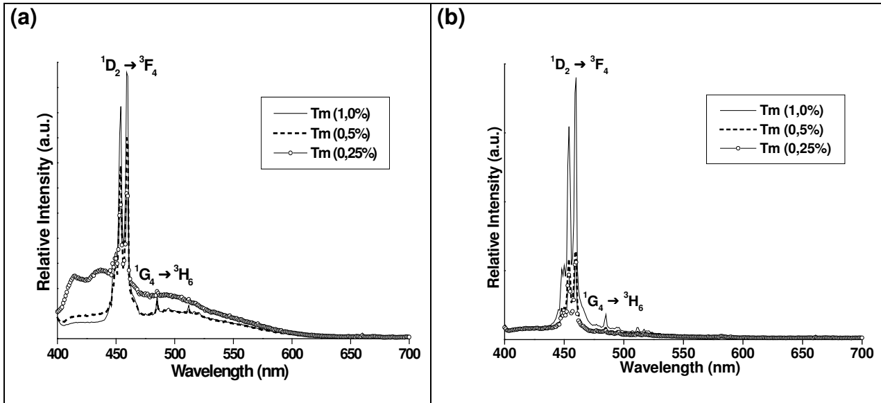
Figura 31: Espectros de emissão ( \lambda_{\text{exc}} = 356 \text{ nm} ), a temperatura ambiente: amostras (a) \text{Lu}_3\text{Al}_5\text{O}_{12}:\text{Tm} e (b) \text{Y}_3\text{Al}_5\text{O}_{12}:\text{Tm} , preparadas por Pechini e calcinadas a 1100^\circ\text{C} .
