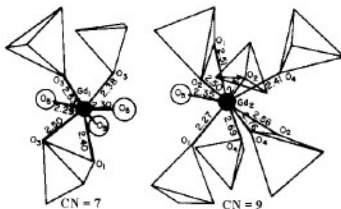
Figura 34: Sítios cristalográficos do \text{Gd}_2\text{SiO}_5 monoclínico, grupo espacial P2_1/c , e correspondentes distâncias atômicas. Os íons \text{Gd}^{3+} , em ambos sítios Gd(1) e Gd(2), são representados por um círculo cheio no centro da estrutura. \text{O}_1 , \text{O}_2 , \text{O}_3 e \text{O}_4 são íons \text{O}^{2-} ligados a grupos silicatos tetraédricos e \text{O}_5 são íons \text{O}^{2-} isolados [13; 73].
