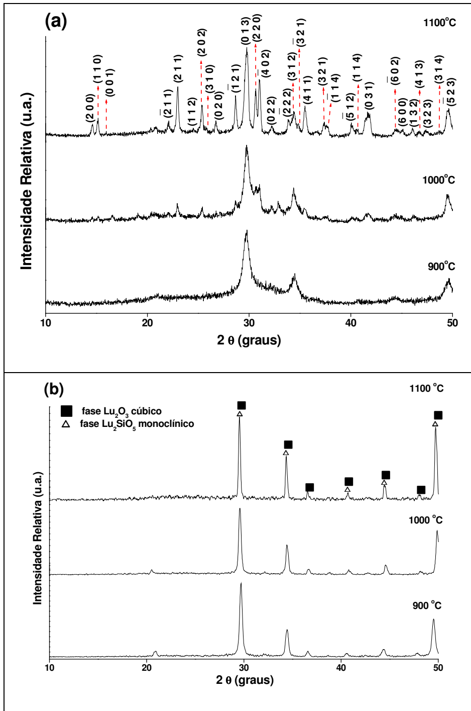
Figura 38: Difratogramas de raios X das amostras \text{Lu}_2\text{SiO}_5:\text{Tm}(1,0\%) sintetizadas pelos métodos (a) sol-gel convencional e (b) sol-gel modificado usando PVA como polímero precursor e calcinadas nas diferentes temperaturas.
