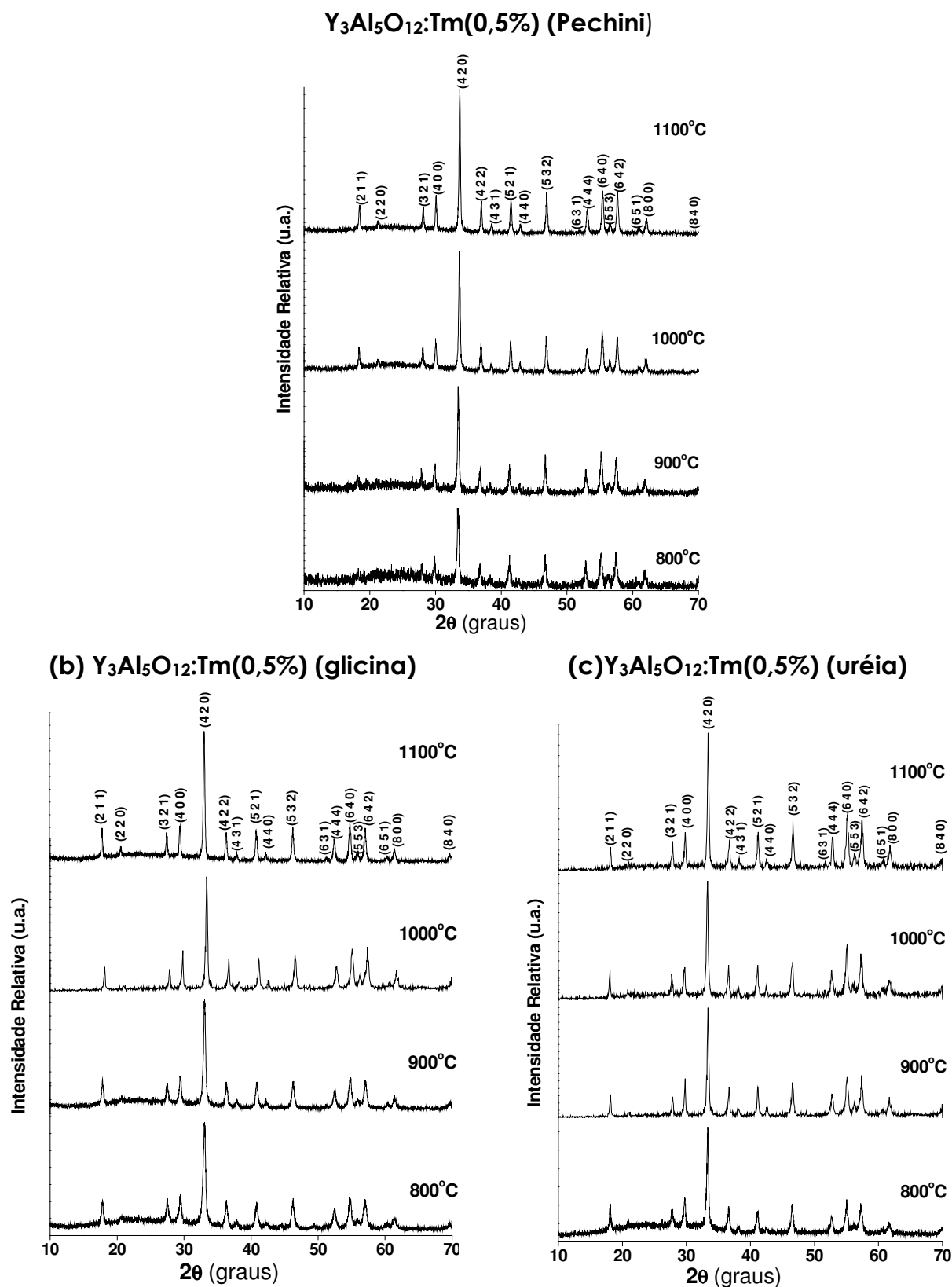
Figura 16: Difractogramas de raios X do pó do composto Y 3 Al 5 O 12 :Tm(0,5%) sintetizado por Pechini (a) e por combustão com glicina (b) ou uréia (c) , calcinado a temperaturas entre 800 e 1100°C.
