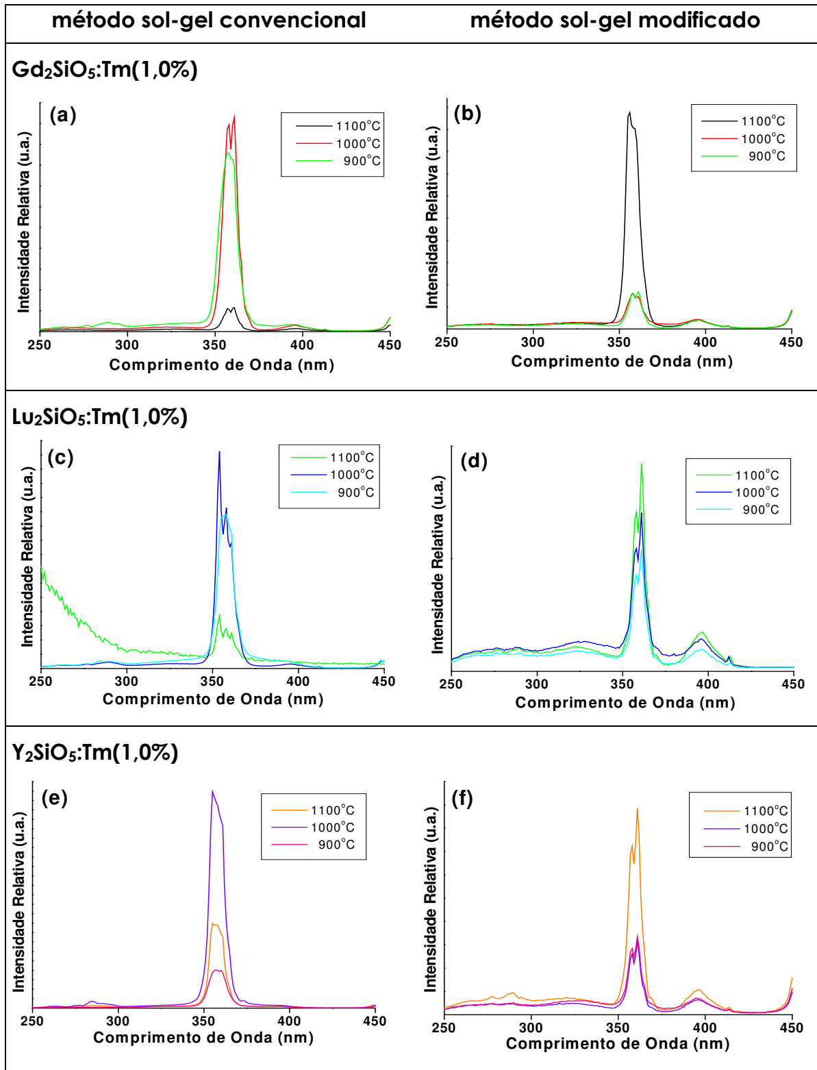
Figura 53: Espectros de excitação corrigidos ( \lambda_{em} = 453 nm) das amostras Gd 2 SiO 5 :Tm(1,0%), (a) e (b); Lu 2 SiO 5 :Tm(1,0%), (c) e (d); Y 2 SiO 5 :Tm(1,0%), (e) e (f), sintetizados pelos métodos sol-gel convencional (a), (c) e (e) e sol-gel modificado usando PVA como polímero precursor (b), (d) e (f), calcinadas de 900 a 1100°C. f_{ex} = f_{em} que resultam em largura de banda de excitação de 1 nm; temperatura ambiente.
