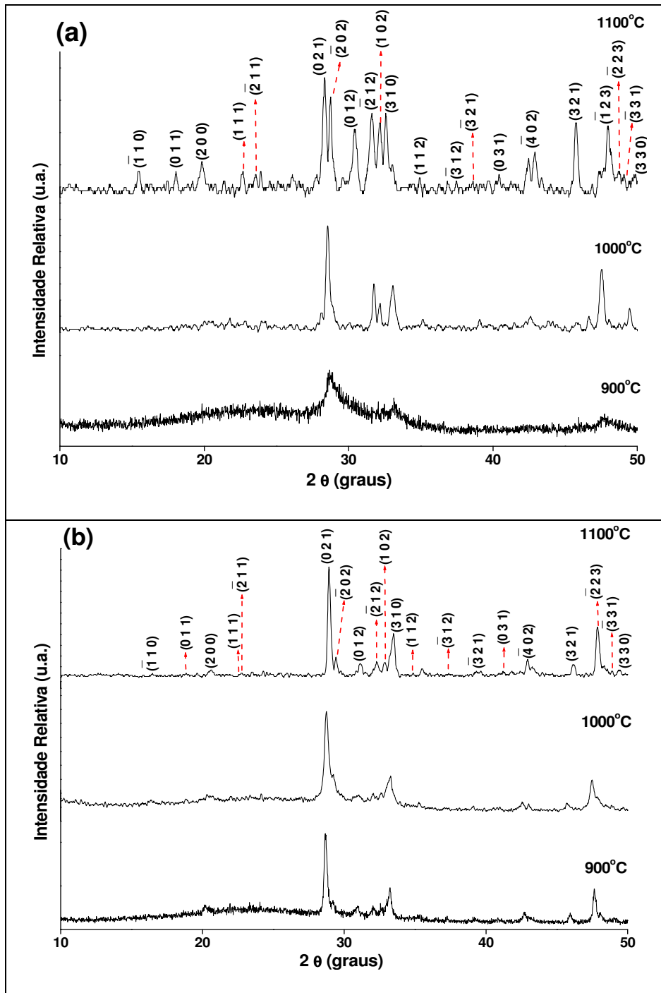
Figura 37: Difratoogramas de raios X das amostras Gd_2SiO_5:Tm(1,0\%) sintetizadas pelos métodos (a) sol-gel convencional e (b) sol-gel modificado usando PVA como polímero precursor e calcinadas nas diferentes temperaturas.
