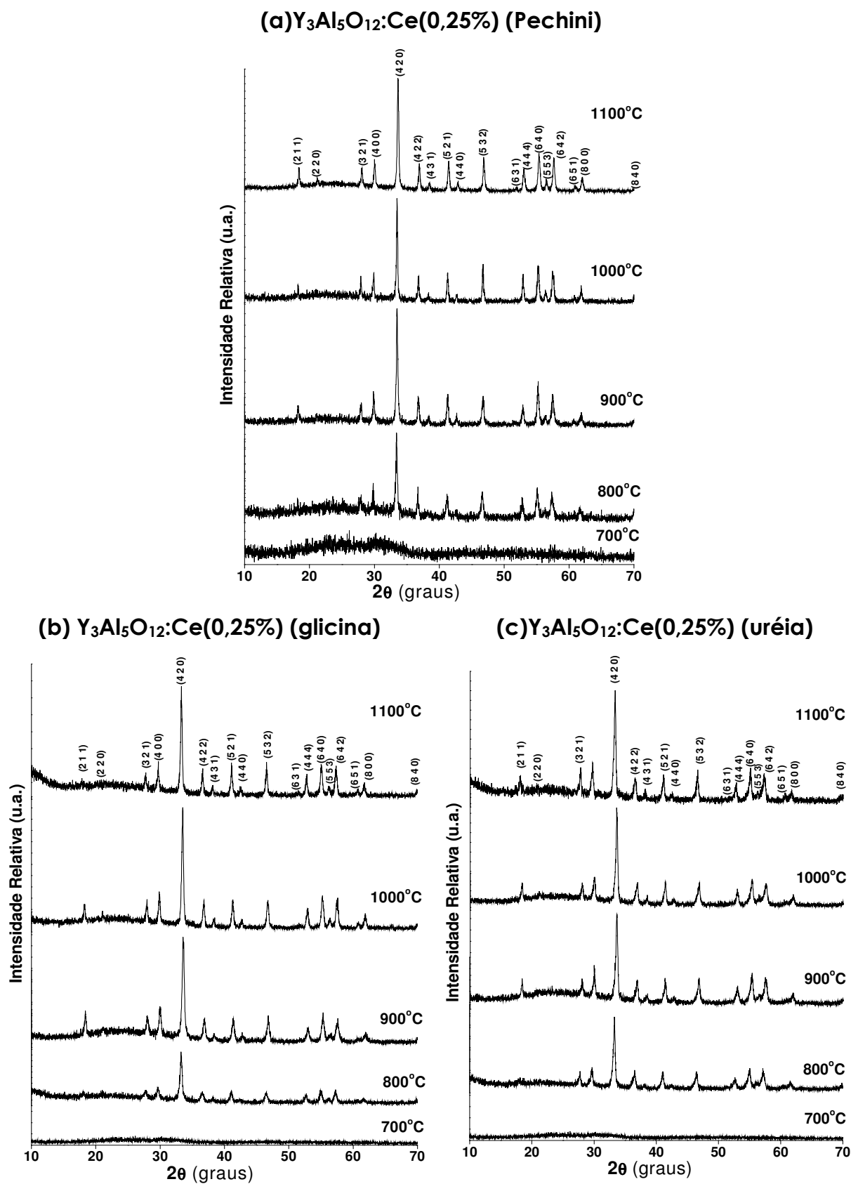
Figura 14: Difratogramas de raios X do pó da amostra Y_3Al_5O_{12}:Ce(0,25\%) preparada pelos métodos Pechini (a) e combustão com glicina (b) ou uréia (c) , calcinadas a temperaturas entre 700 e 1100°C.
