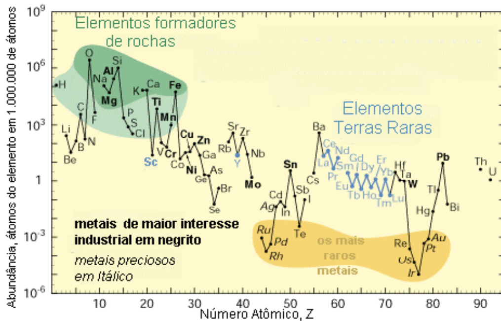
Figura 1: Abundância dos elementos químicos na crosta terrestre em função do número atômico [4].
