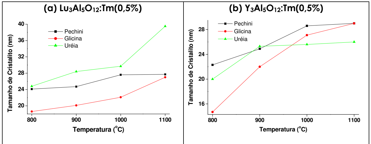
Figura 17: Tamanho médio de cristalito versus temperatura de aquecimento da amostra para (a) \text{Lu}_3\text{Al}_5\text{O}_{12}:\text{Tm}(0,5\%) e (b) \text{Y}_3\text{Al}_5\text{O}_{12}:\text{Tm}(0,5\%) .
