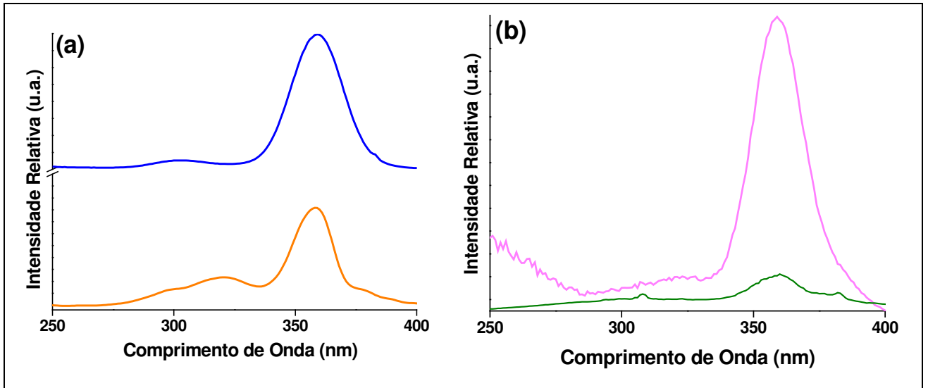
Figura 48: Espectros de excitação ( \lambda_{em} = 419 nm) do \text{Lu}_2\text{SiO}_5:\text{Ce}(1,0\%) sintetizado pelos métodos (a) sol-gel convencional e (b) sol-gel modificado usando PVA como polímero precursor, a temperatura ambiente. (—) e (—) a temperatura ambiente; (—) e (—) a 77 K.
