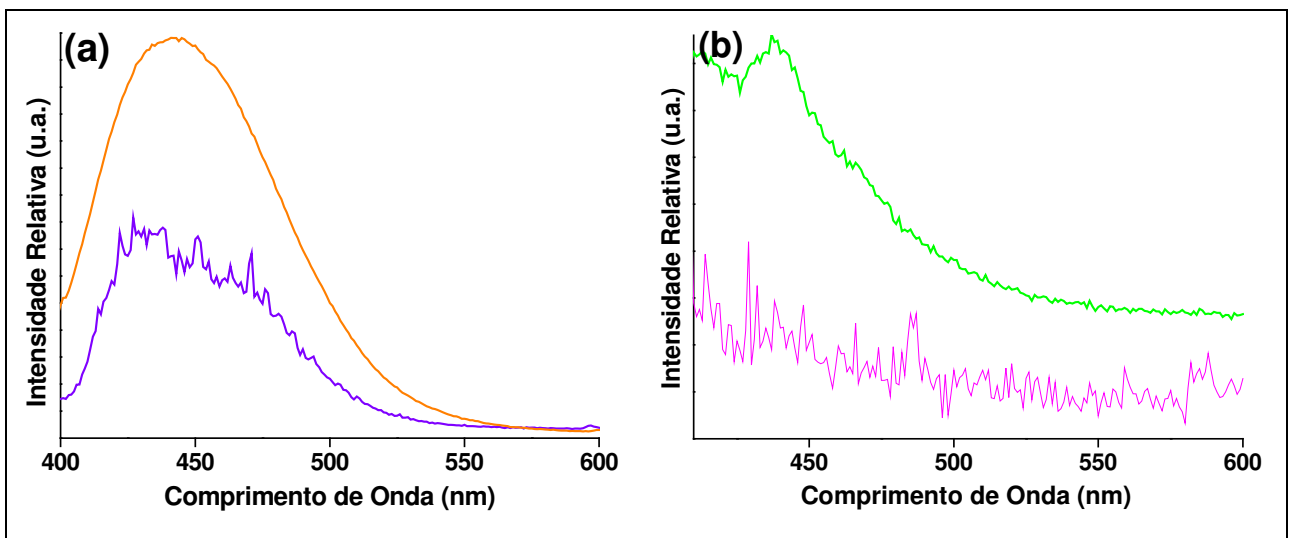
Figura 51: Espectros de emissão ( \lambda_{exc}= 365 nm) do composto \text{Y}_2\text{SiO}_5:\text{Ce}(1,0\%) sintetizado pelos métodos (a) sol-gel convencional e (b) sol-gel modificado usando PVA como polímero precursor. (—) e (—) a temperatura ambiente; (—) e (—) a 77 K.
