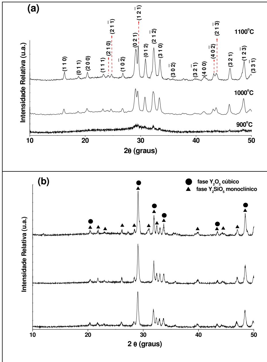
Figura 36: Difratoogramas de raios X das amostras Y_2SiO_5:Ce(1,0\%) sintetizadas pelos métodos (a) sol-gel convencional e (b) sol-gel modificado usando PVA como polímero precursor e calcinadas nas diferentes temperaturas.
