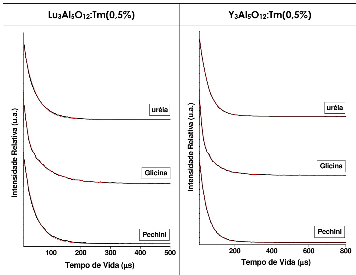
Figura 32: Curvas de decaimento, (—) experimental e (---) calculada, do singlete D_2 referente à transição ^1D_2 \rightarrow ^3F_4 do Tm^{3+} nos compostos Lu_3Al_5O_{12}:Tm(0,5\%) e Y_3Al_5O_{12}:Tm(0,5\%) ; \lambda_{ex} = 355 nm e \lambda_{em} = 460 nm; temperatura ambiente.
