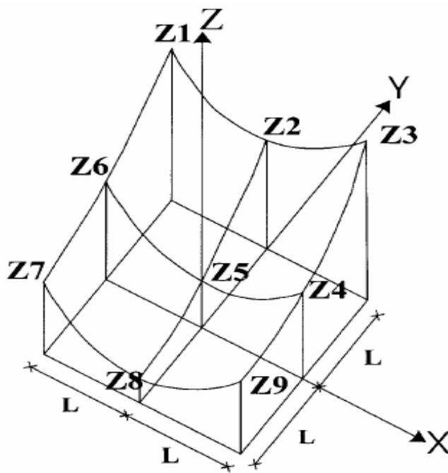
Figura 2. Submatriz de elevação, empregada nos cálculos de variáveis topográficas do terreno (Zevenbergen & Törnén, 1987).
