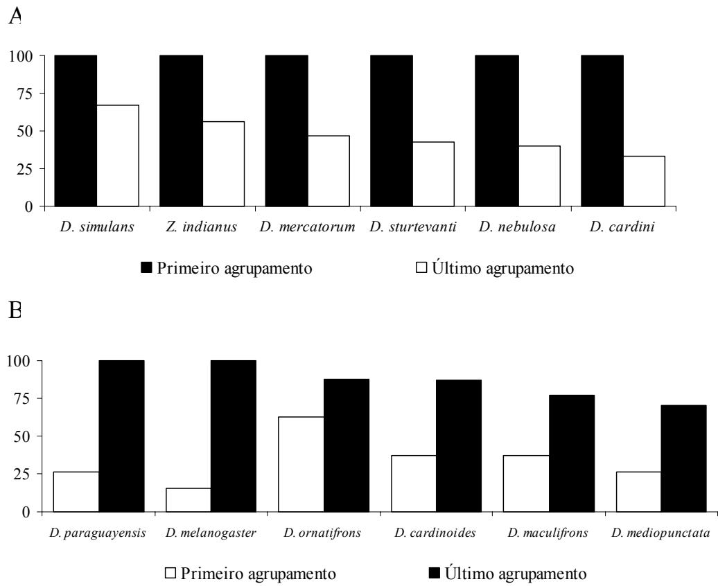
Figura 3 – Valor indicador (%) obtido para o primeiro e último agrupamento de tipos de habitats das espécies que reagiram ao agrupamento hierárquico que separou os tipos de habitats. A. espécies com maior IndVal (%) no primeiro agrupamento (amplamente distribuídas); B. aquelas com maior IndVal (%) no último agrupamento (restritas).
