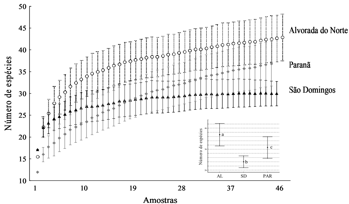
Figura 1 – Curva de acumulação (Jackknife 1) para cada área, mostrando também as médias diferentes das últimas amostras de cada uma delas. AL , Alvorada do Norte; SD , São Domingos; PAR , Paranã. Letras diferentes indicam diferença significativa.
