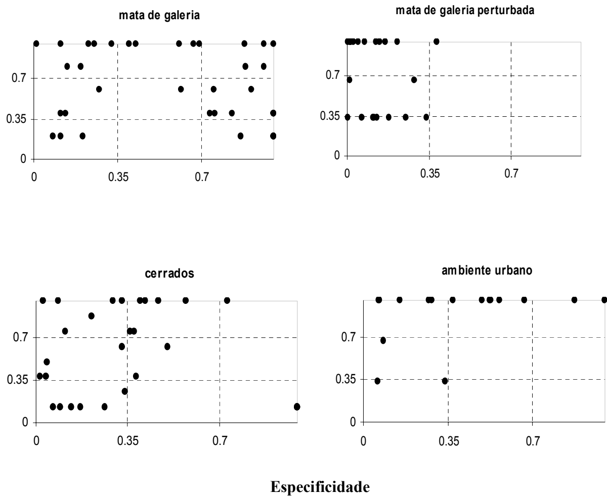
Figura 4 - Relação entre os dois componentes do IndVal (especificidade e fidelidade) para as espécies das assembléias de drosofilídeos, em cada tipo de hábitat.
