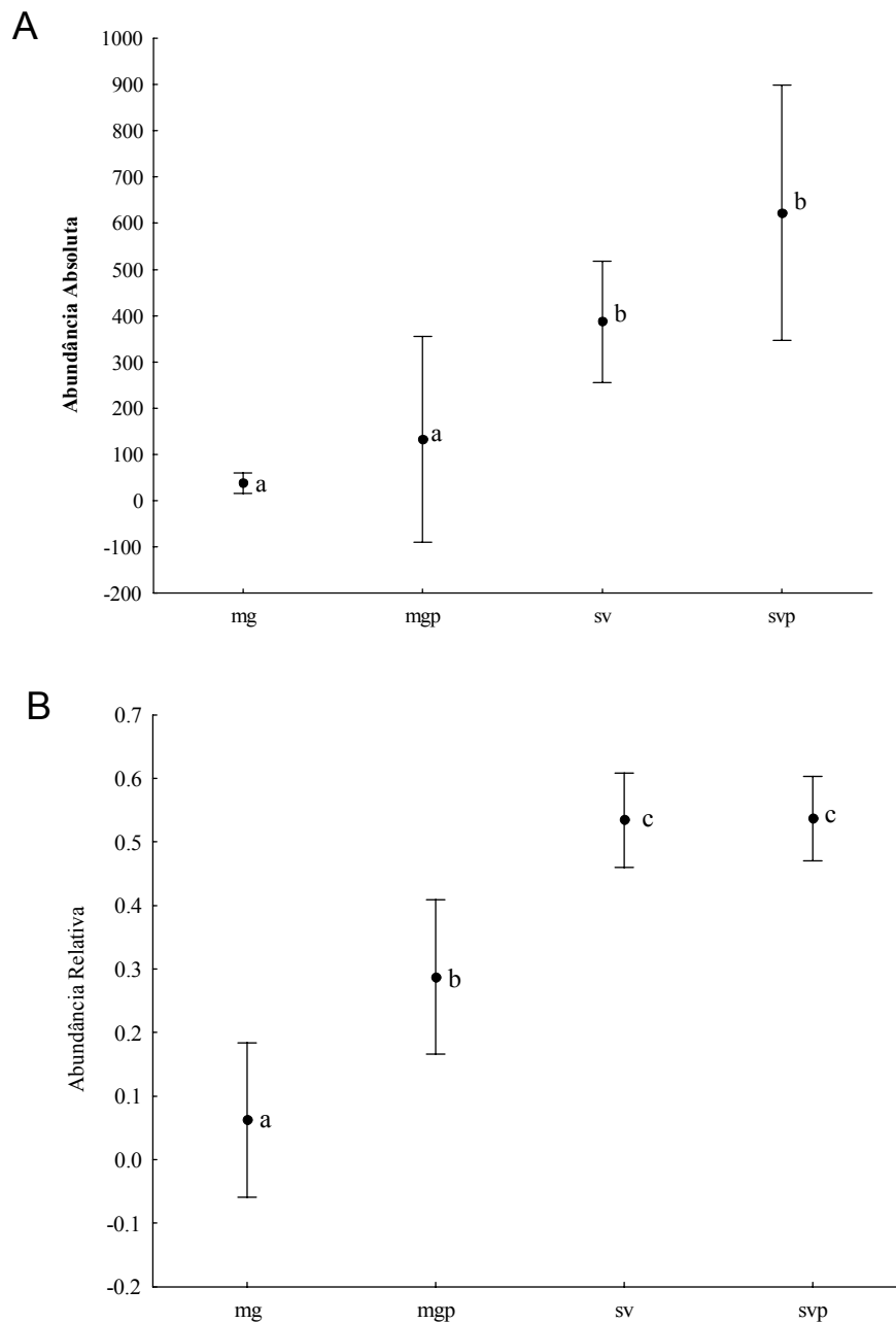
Figura 3 – Médias da abundância absoluta (A) e relativa (B) das espécies exóticas nas matas de galeria não perturbadas (mg), nas matas de galeria perturbadas (mgp), nas savanas não perturbadas (sv) e nas savanas perturbadas (svp). Letras diferentes indicam diferença significativa.
