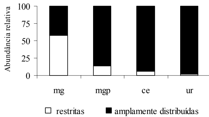
Figura 2 – Diferenças na composição das assembléias de drosofilídeos entre os tipos de habitats estudados, mostrando a abundância relativa das espécies neotropicais e exóticas (A), bem como das espécies restritas e das amplamente distribuídas (B). mg. mata de galeria não perturbada; mgp. mata de galeria perturbada; ce. cerrados; ur. ambiente urbano
