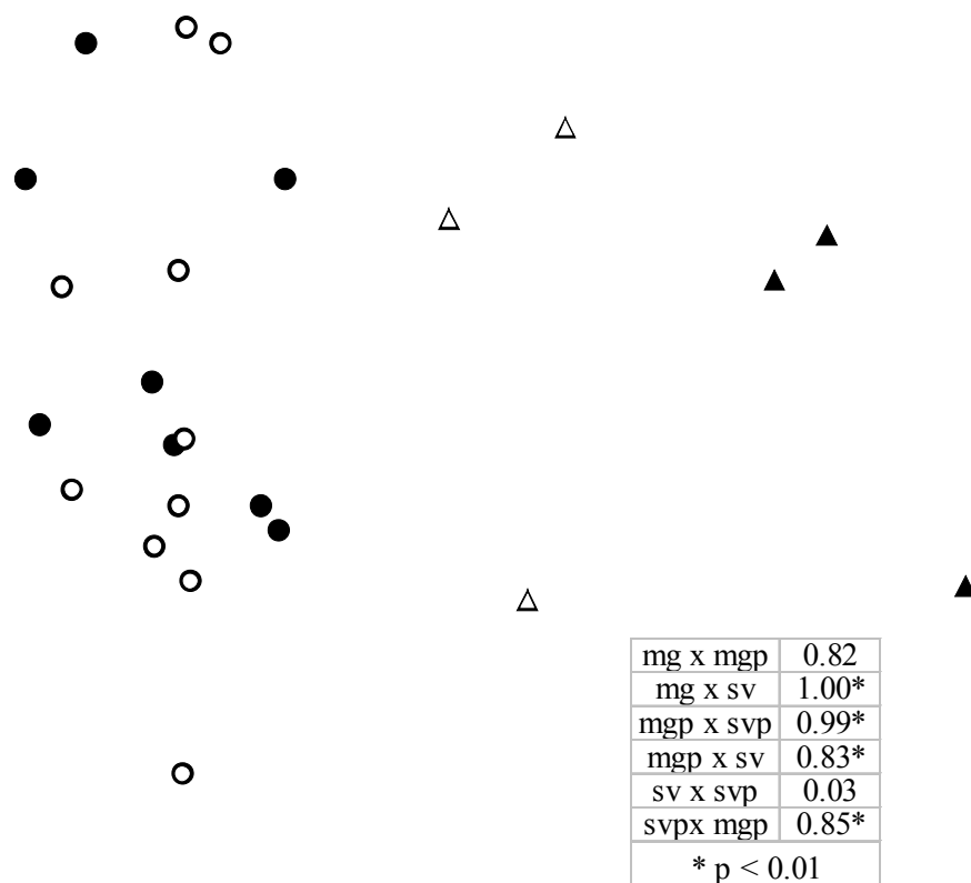
Figura 4 – Ordenação propiciada pela Análise Multidimensional não-Métrica (nMDS) baseada nas abundâncias de drosofilídeos, mostrando a similaridade relativa entre as amostras procedentes de: ▲. matas de galeria não perturbadas; △. matas de galeria perturbadas; ●. savanas não perturbadas; ○ savanas perturbadas. (R global = 0.55; p < 0.001 ; stress = 0.14).
