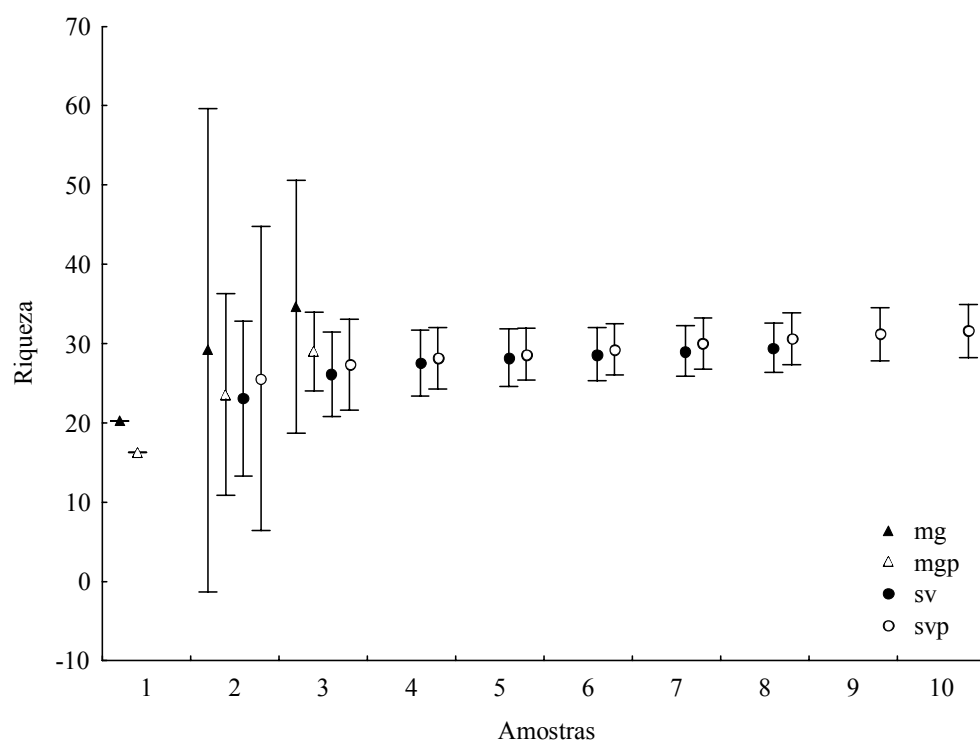
Figura 2 – comparação entre as curvas de acumulação (Jackknife 1) de espécies de drosofilídeos em mata de galeria não perturbada (mg), mata de galeria perturbada (mgp), savanas não perturbadas (sv), savanas perturbadas (svp).
