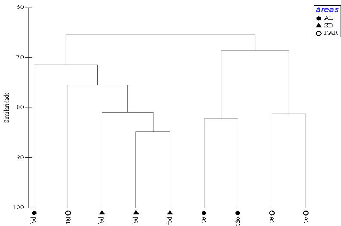
Figura 3 – Relações de similaridade entre as assembléias de drosofilídeos nos habitats analisados. AL , Alvorada do Norte; SD , São Domingos; PAR , Paranã. fed , floresta tropical estacional decidual; mg mata de galeria; ce , cerrado sentido restrito; cão , cerradão.
