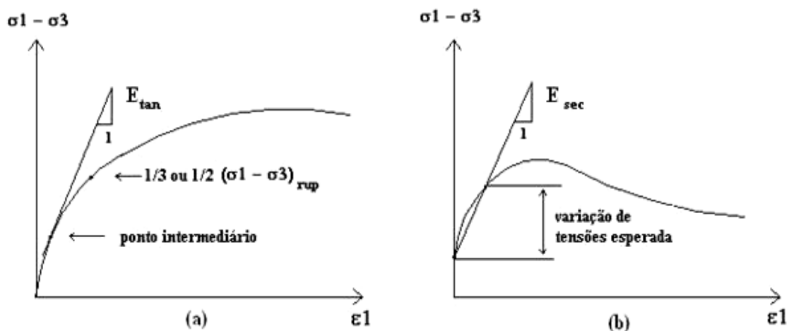
Figura 2.3 - Gráficos comportamento \sigma \times \epsilon para determinação do módulo de elasticidade longitudinal E_s , (a) Módulo Tangente e (b) Módulo Secante
