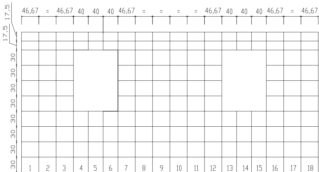
Figura 4.1 – Parede P1-X
