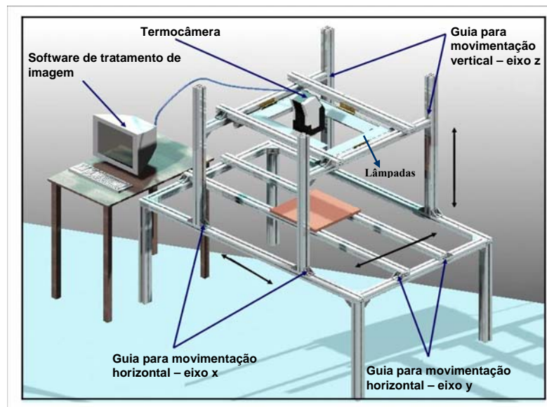
Figura 3.12 – Esquema da bancada de testes
