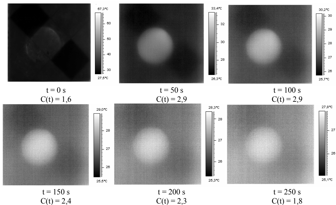
Figura 4.18 – Termografia pulsada – amostra P3 ( 2,4 \times 10^4 \text{ J} e d = 0,50 \text{ m} )
