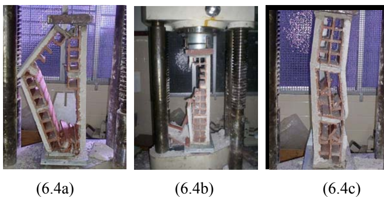
Figura 6.4 - Formas de ruptura dos prismas com revestimento de 2 cm
