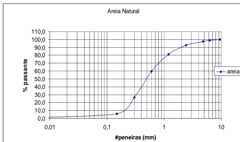
Figura 5.1 – Gráfico da curva granulométrica da areia
