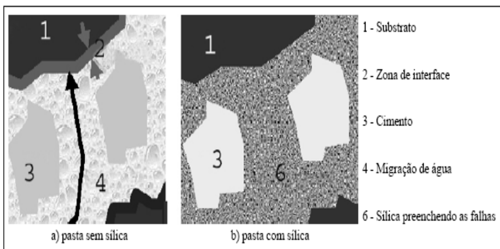
Figura 2.4 – Zona de interface pasta/substrato, SILVA & LIBÓRIO (2003)
