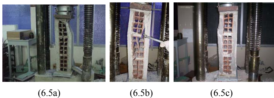
Figura 6.5 - Formas de ruptura dos prismas com revestimento de 3 cm
