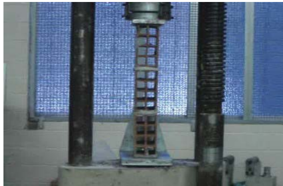
Figura 6.6 (a) – Prisma nu antes da ruptura
