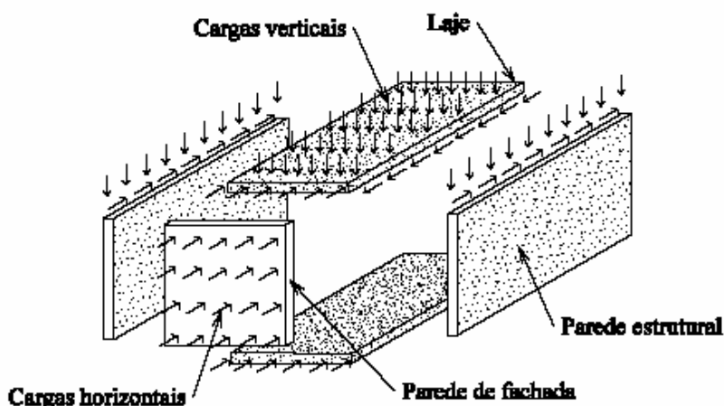
Figura 2.19 – Distribuição de cargas em um prédio de alvenaria estrutural, GOMES (2001)
