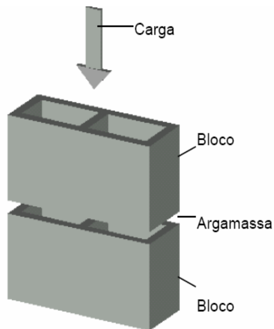
Figura 2.17 (a) – Prisma com blocos estruturais
