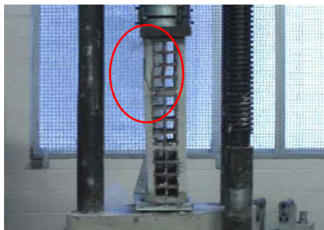
Figura 6.9 (b) – Prisma com 2 cm de revestimento no instante 1 posterior à ruptura
