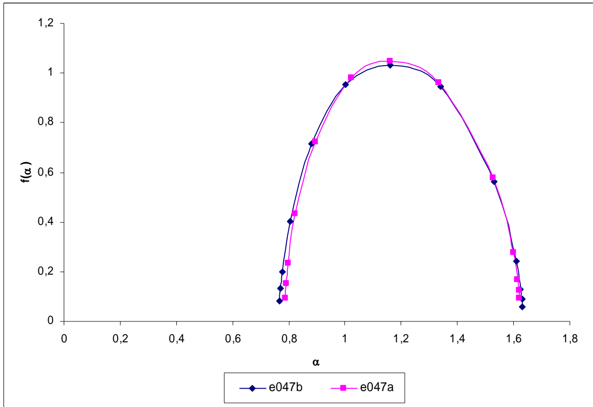
Figura 5.6- Espectros de singularidades para o paciente e047 antes e após medicação, obtida pela técnica MF-DFA
