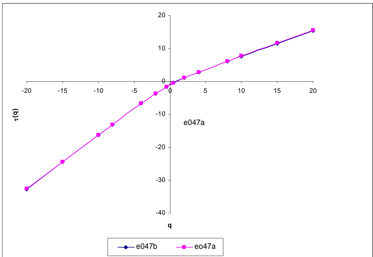
Figura 5.5 (a) e (b) – Dependência do expoente generalizado de Hurst com q para as séries correspondentes ao paciente e047 antes e após medicação, utilizada para tal a técnica MF-DFA
