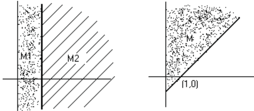
Figura 4.2: Subsemigrupos totais do grupo Aff^+
