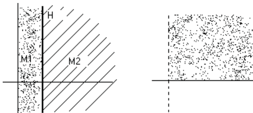
Figura 4.3: Subsemigrupos maximais do grupo Aff^+
