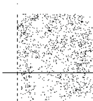
Figura 4.1: Representação geométrica do grupo afim.
