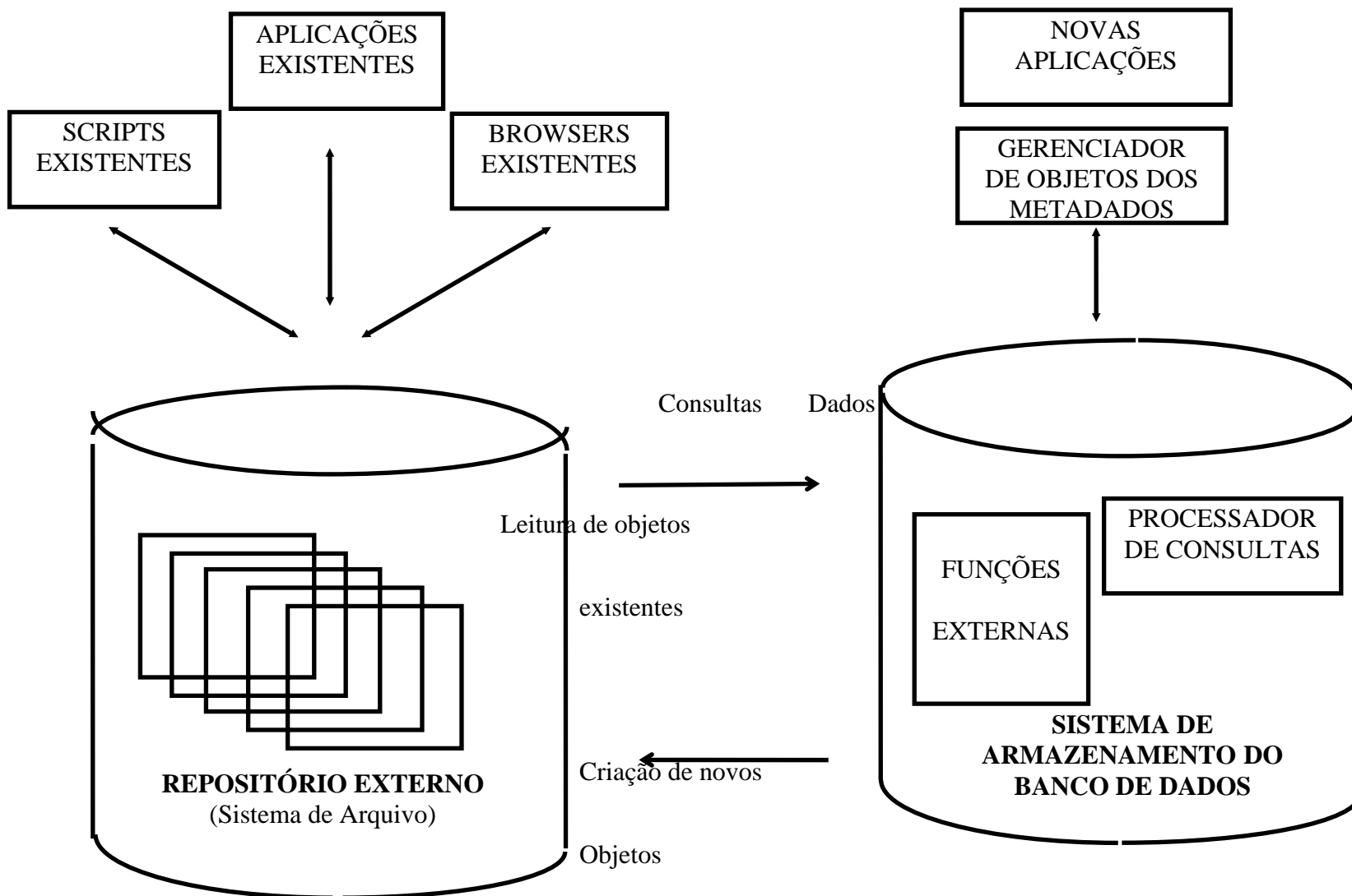
Figura 4: Solução de arquitetura para o sistema aberto para armazenamento de objetos abstratos e acesso a metadados geográficos digitais.
