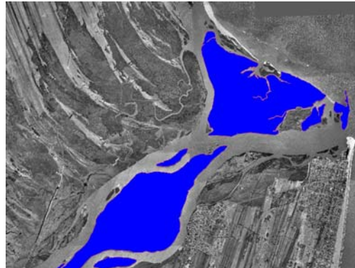
Figura 25: Imagem de algumas ilhas vetorizadas (editadas por VASCONCELOS, 2005).
