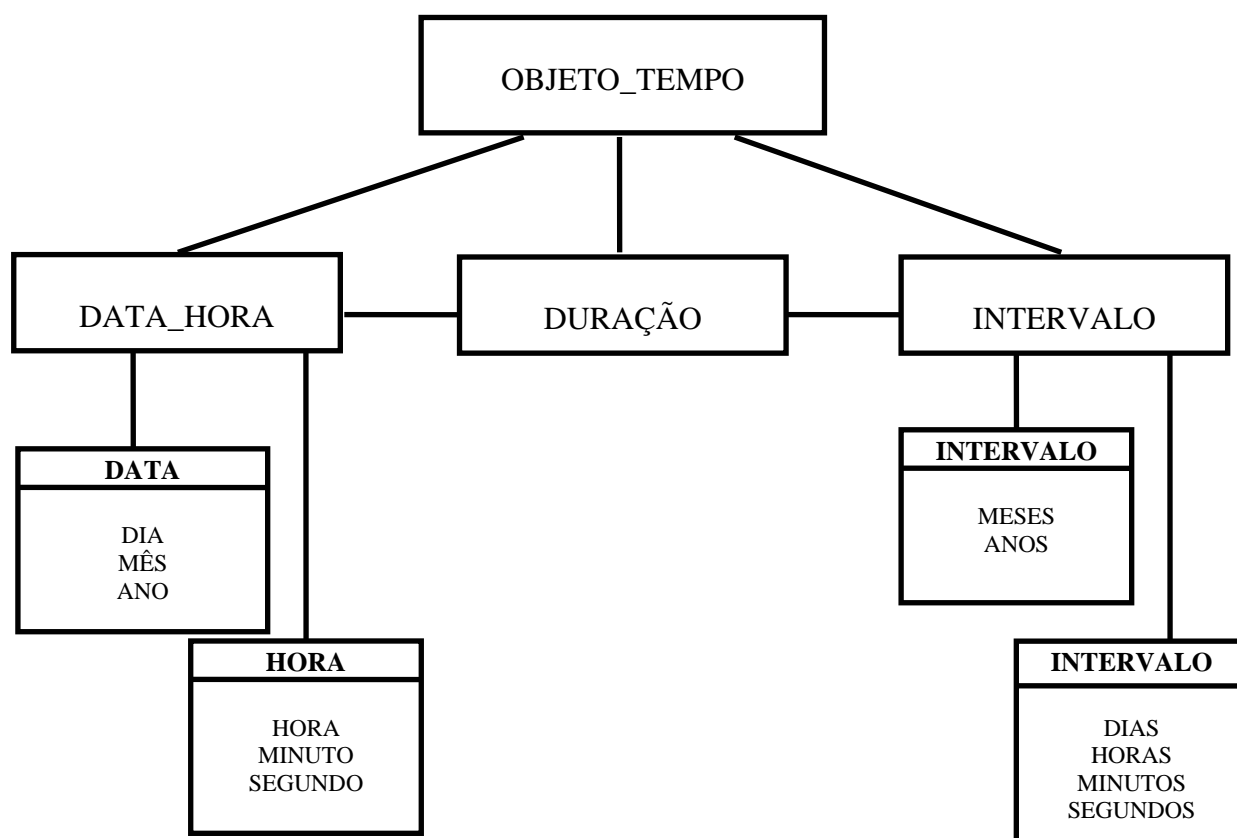
Figura 6: Estrutura de classes de tempo no contexto do SAIF.
