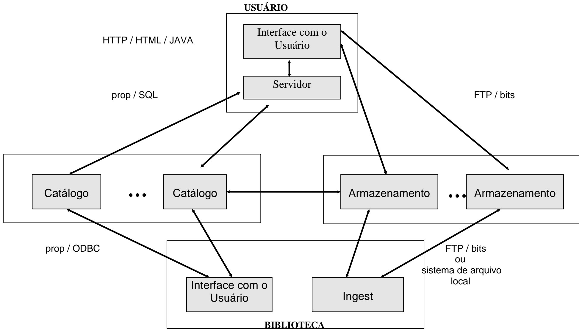
Figura 5: Arquitetura geral da Biblioteca Digital Alexandria.
