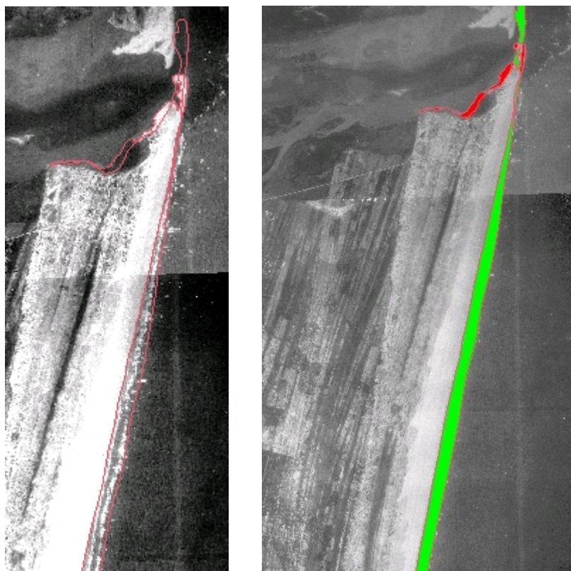
Figuras 38: Evolução da linha de costa entre 1954 e 1974 (vermelho=erosão; verde=progradação).
