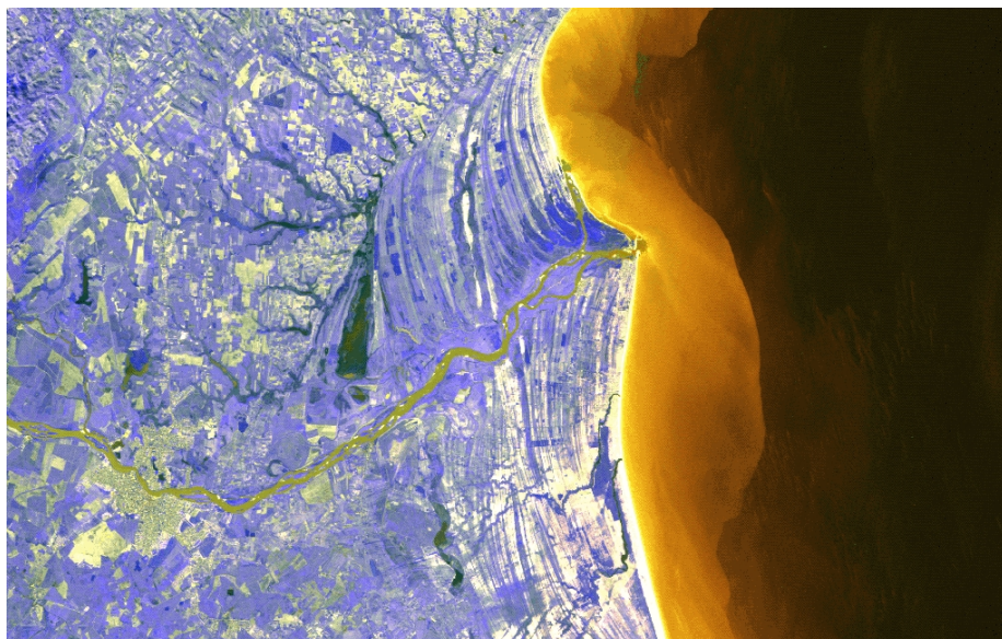
Figura 20: Recorte de imagem CBERS (RGB243), data: 16/07/2004.
