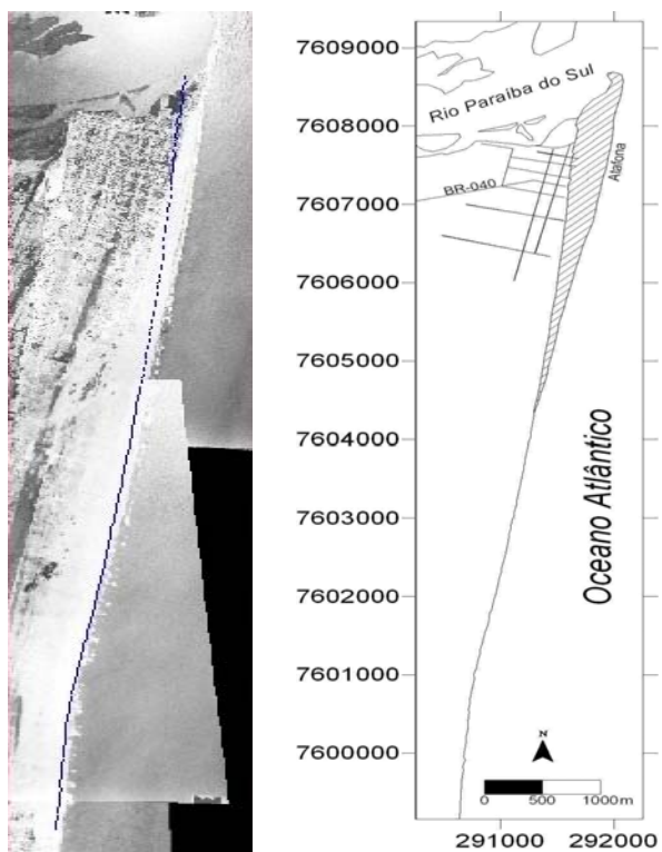
Figuras 32 e 33: Área erodida entre 1964/2004.
