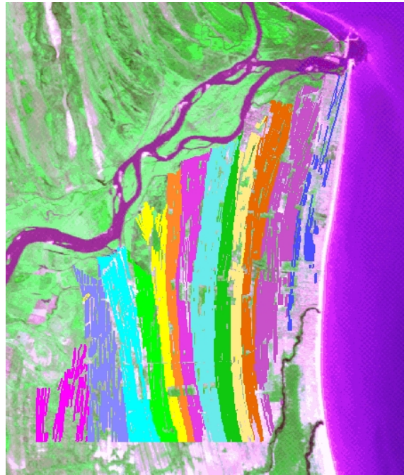
Figura 19: Treze sistemas de discordâncias (apresentados por cores distintas) compostos pelas cristas de praia preservadas na parte meridional da planície deltaica do rio Paraíba do Sul. Pano de fundo composição colorida CBERS RGB342, data: 16/07/2004.
