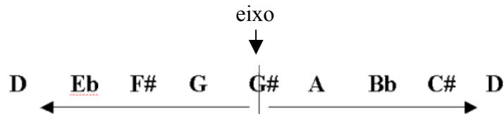
Exemplo 2b: Escala com nota agregada e simetria intervalar com eixo no G#
