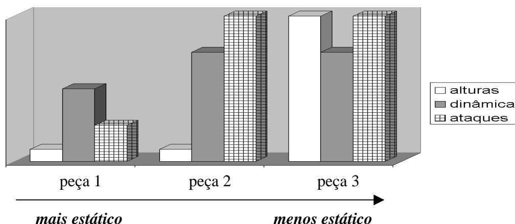
Figura 4: Variações de dinâmica, alturas e incidência de ataques
