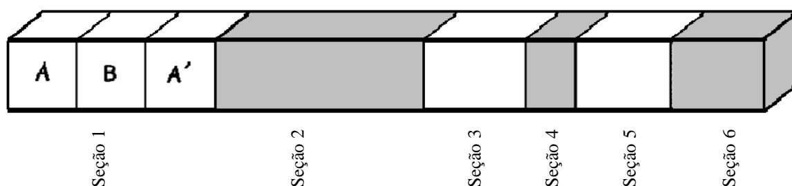
Figura 2: Estrutura formal da peça “Como Enlouquecer Um Trovador”
