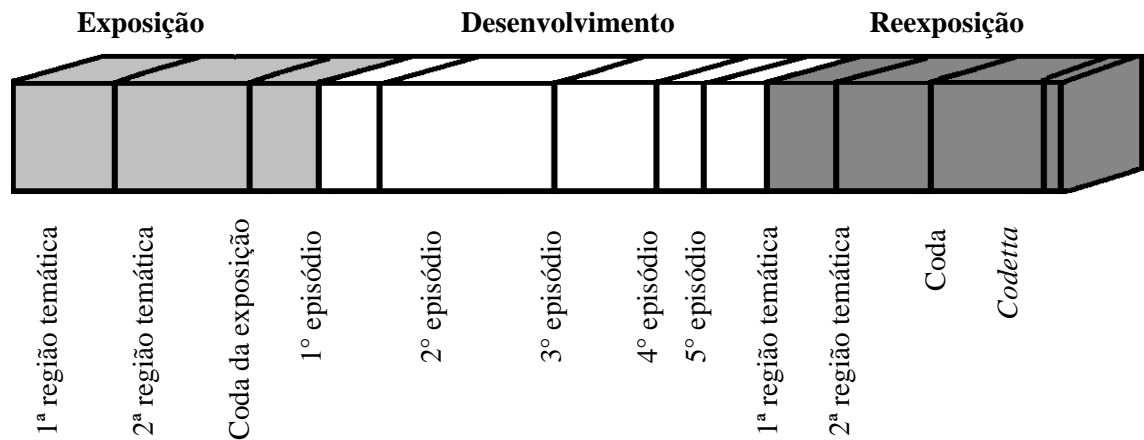
Figura 3: Estrutura formal de “Peça Para Cães Famintos”
