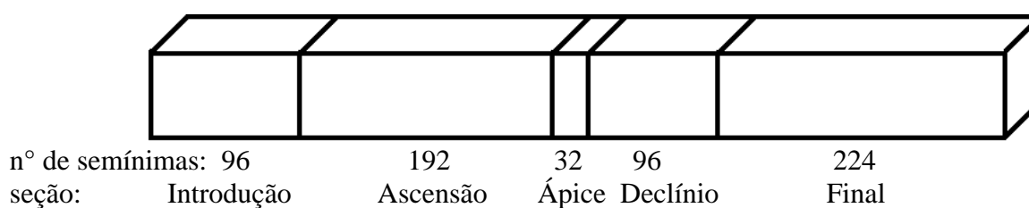
Figura 1: Estrutura formal original de “Nocaute!”
