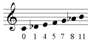
Exemplo 1a: Conjunto de sete notas formado pelas alturas C, Db, E, F, G, Ab e B
