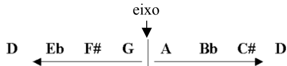
Exemplo 2a: Escala original com simetria intervalar com o eixo entre o G e A
