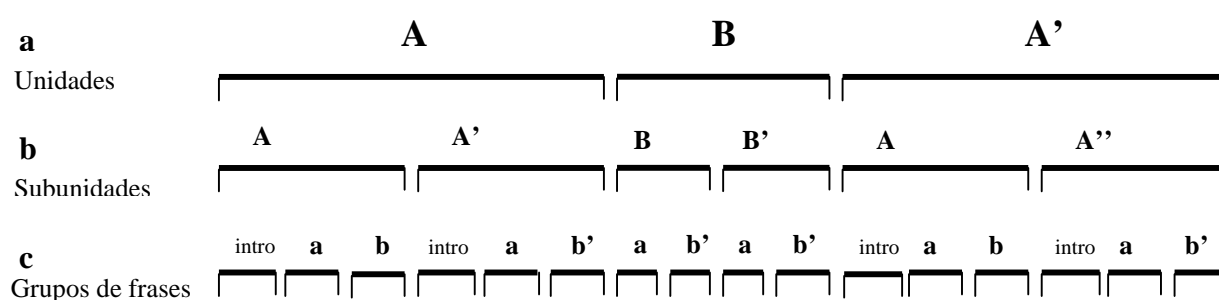
Exemplo 7 a, b e c: Subdivisões da primeira seção formal de “Como Enlouquecer Um Trovador”
