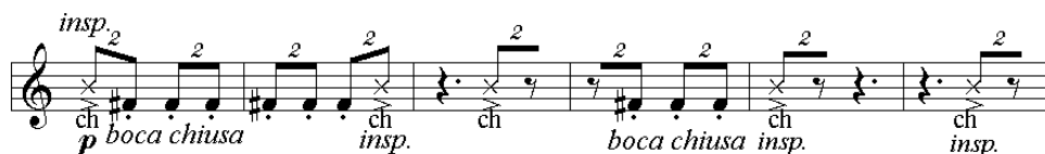
Exemplo 10: Grupo de notas no [363]
