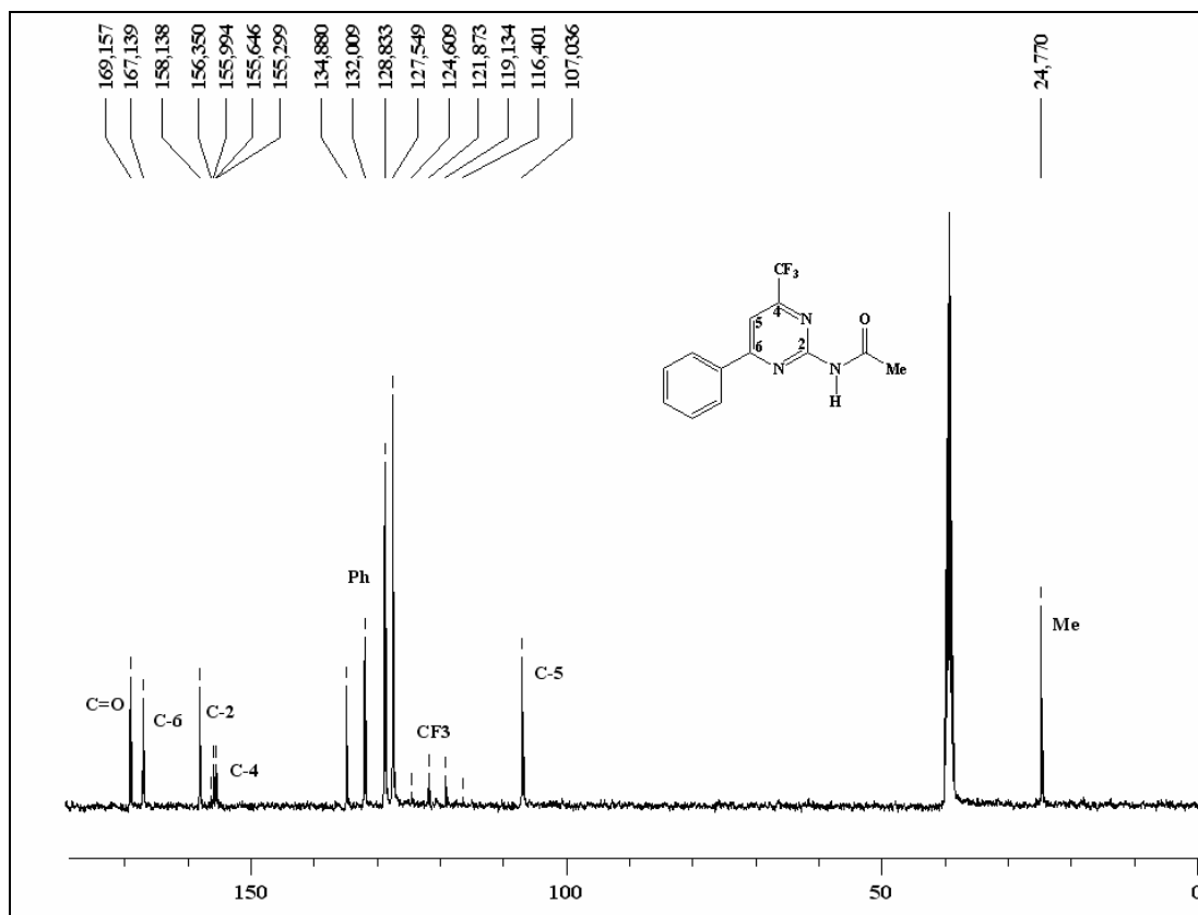
Figura 04 – Espectro de RMN ^{13}\text{C} \{^1\text{H}\} a 100 MHz do composto 4-trifluormetil-6-fenil-2-acetilaminopirimidina 6b , registrado em \text{DMSO-d}_6 .
