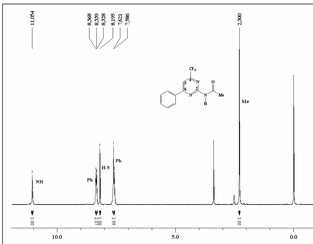
Figura 03 – Espectro de RMN ^1\text{H} a 50 MHz do composto 4-trifluormetil-6-fenil-2-acetilaminopirimidina 6b , registrado em DMSO- d_6 .
