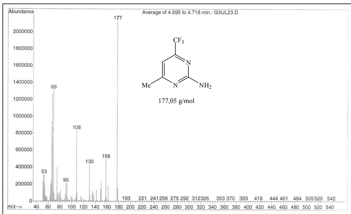
Figura 69 – Espectro de Massas do composto 4-trifluormetil-6-metil-2-aminopirimidina 8a .
