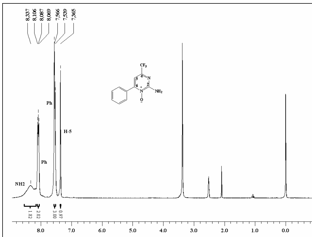
Figura 12 – Espectro de RMN ^1\text{H} a 50 MHz do composto 4-trifluormetil-6-fenil-2-aminopirimidina- N^1 -óxido 11b , registrado em \text{DMSO-d}_6 .
