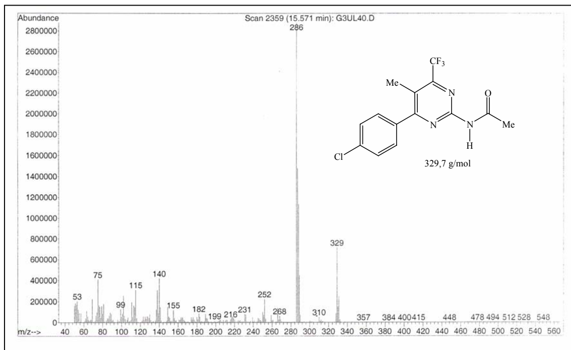
Figura 55 – Espectro de Massas do composto 4-trifluorometil-5-metil-6-(4-clorofenil)-2-acetilaminopirimidina 6i .
