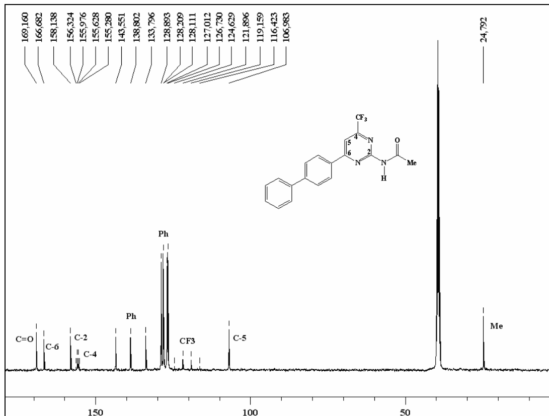
Figura 30 – Espectro de RMN 1 H a 50 MHz e RMN 13 C { 1 H} a 100 MHz do composto 4-trifluormetil-6-(bifenil)-2-acetilaminopirimidina 6k , registrado em DMSO-d 6 .
