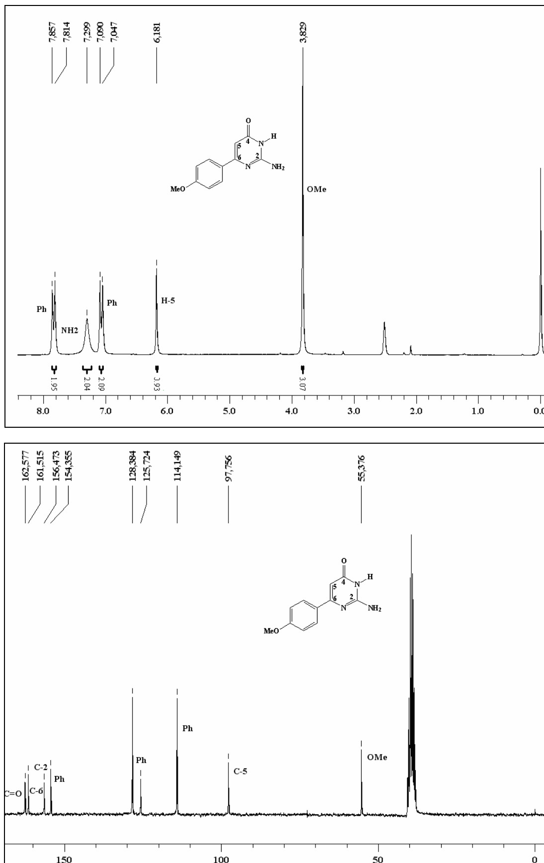
Figura 46 – Espectro de RMN ^1\text{H} a 50 MHz e RMN ^{13}\text{C} \{^1\text{H}\} a 100 MHz do composto 6-(4-metoxifenil)-2-amino-4(3H)-pirimidinona 9g , registrado em \text{DMSO-d}_6 .
