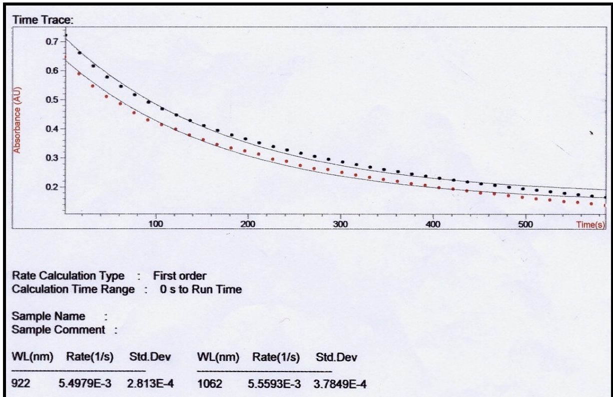
Figura 23: gráfico do ensaio de cinética do corante Q-Switch (absorbância x tempo).
