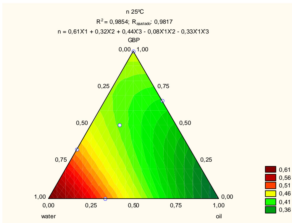
FIGURA 27 – DIAGRAMA TERNÁRIO DA SUPERFÍCIE DE RESPOSTA DO MODELO QUADRÁTICO RELATIVO AO ÍNDICE DE COMPORTAMENTO (n) NA TEMPERATURA DE 25°C
