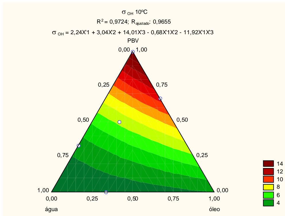
FIGURA 28 – DIAGRAMA TERNÁRIO DA SUPERFÍCIE DE RESPOSTA DO MODELO QUADRÁTICO RELATIVO À TENSÃO INICIAL ( \sigma_{OH} ) NA TEMPERATURA DE 10°C.
