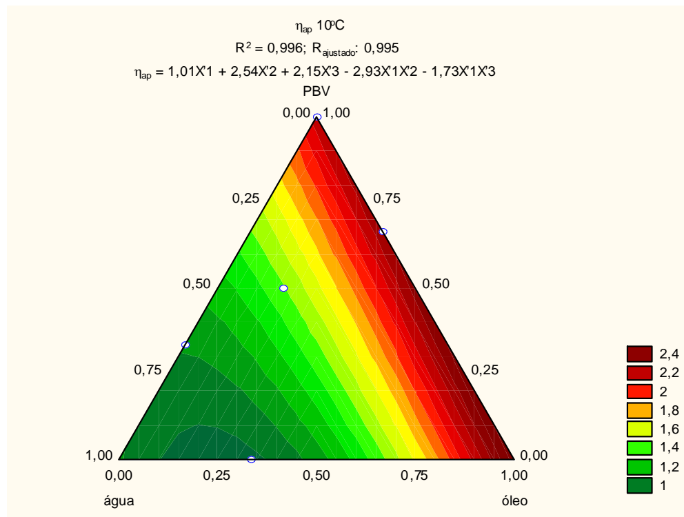
FIGURA 34 – DIAGRAMA TERNÁRIO DA SUPERFÍCIE DE RESPOSTA DO MODELO QUADRÁTICO RELATIVO À VISCOSIDADE APARENTE ( \eta_{ap} ) NA TEMPERATURA DE 10°C
