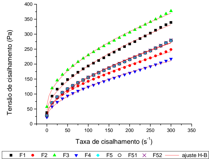
FIGURA 39 – REOGRAMAS AJUSTADOS PELO MODELO DE HERSCHEL-BULKLEY (H-B) PARA AS FORMULAÇÕES A 25°C
