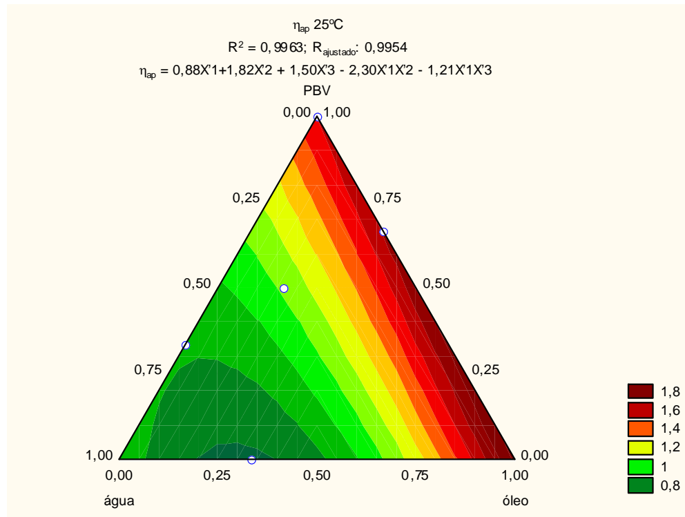
FIGURA 35 – DIAGRAMA TERNÁRIO DA SUPERFÍCIE DE RESPOSTA DO MODELO QUADRÁTICO RELATIVO À VISCOSIDADE APARENTE ( \eta_{ap} ) NA TEMPERATURA DE 25°C
