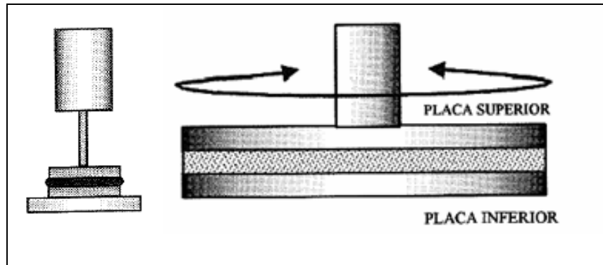
FIGURA 11 – ESQUEMA REPRESENTATIVO DO REÔMETRO PLACA –PLACA
