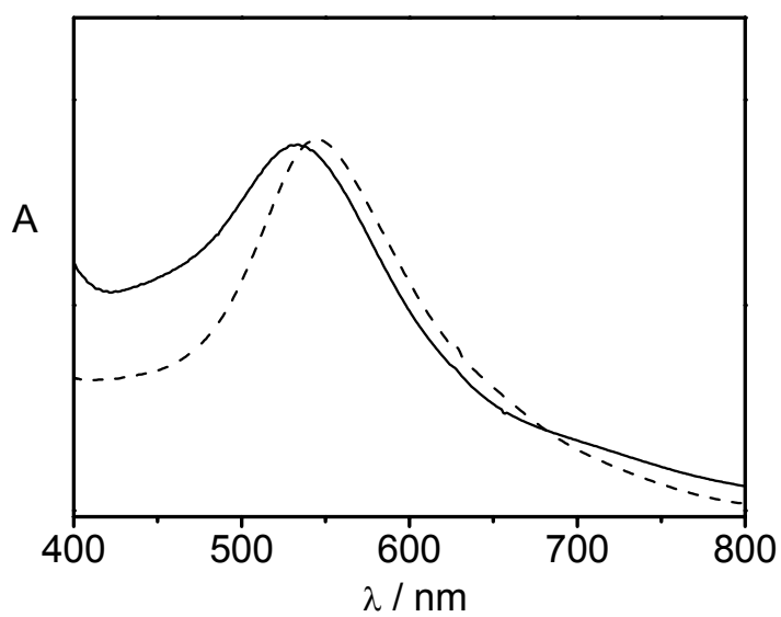
Figura 26. Espectro de absorção da calda de calafate (—) e do fotoanodo sensibilizado pelo mesmo (---).
