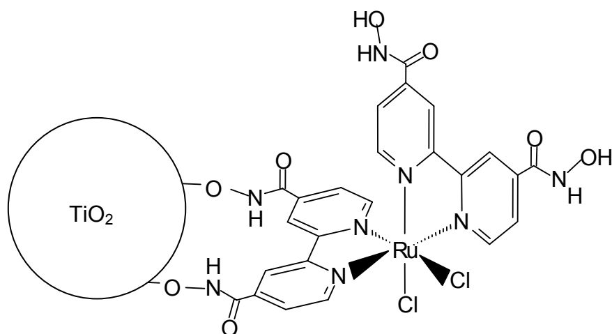
Figura 18. Esquema da adsorção química do composto cis -[Cl 2 Ru(dobH 2 ) 2 ] à superfície do TiO 2 .
