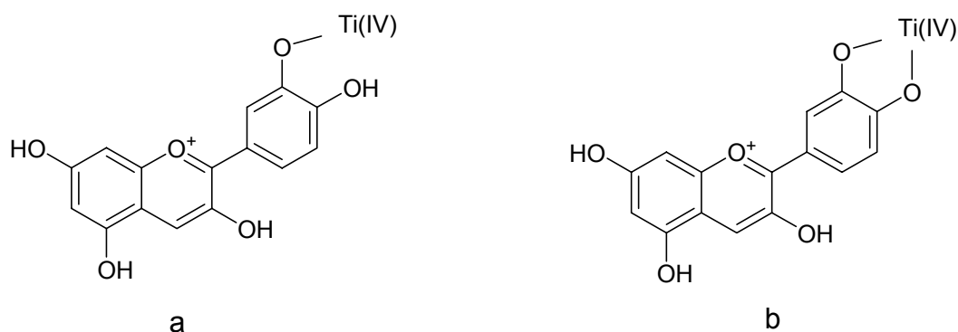
Figura 31. Representação da adsorção da cianidina ao TiO 2 através da condensação de um grupo OH (a) e através do efeito quelato (b).
