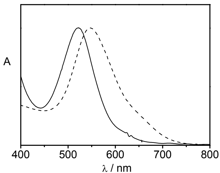
Figura 29. Espectro de absorção do extrato etanólico de jambolão (—) e do fotoanodo sensibilizado pelo mesmo (---).
