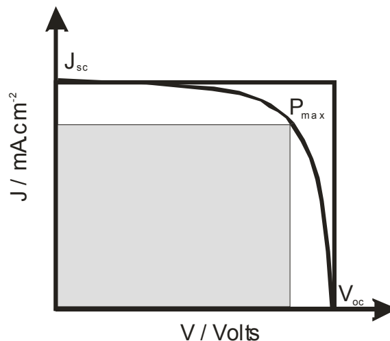
Figura 8. Representação de uma curva-corrente potencial e os pontos onde são obtidos os parâmetros fotoeletroquímicos
