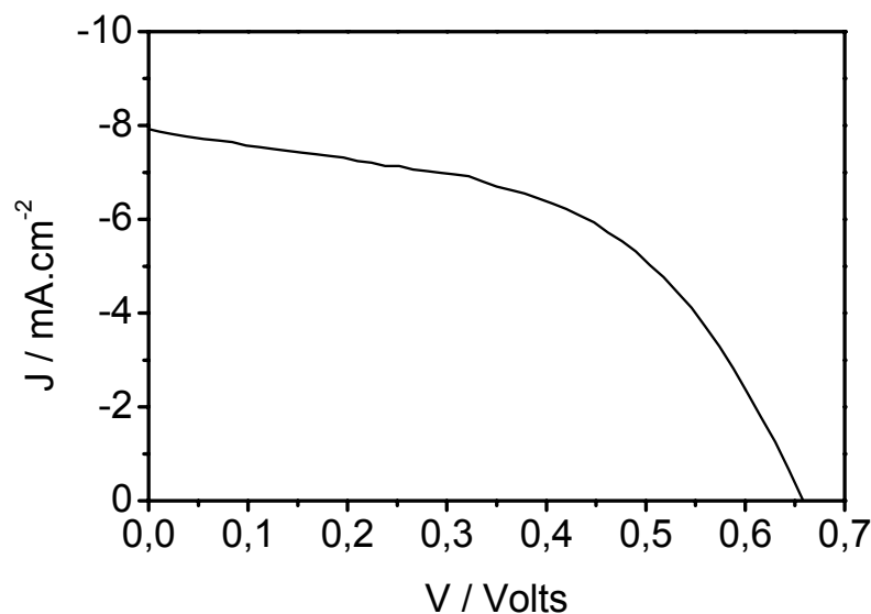
Figura 15. Curva corrente-potencial obtida com uma célula solar sensibilizada pelo corante cis - [(\text{H}_3\text{BCN})_2\text{Ru}(\text{dcbH}_2)_2] .
