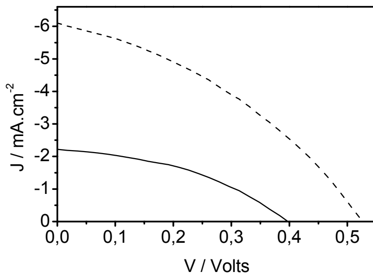
Figura 32. Curva corrente-potencial obtida com uma célula solar sensibilizada pela calda de calafate (—) e pelo extrato aquoso do fruto (---).
