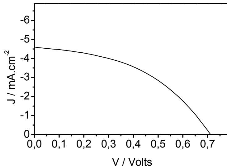
Figura 23. Curva corrente-potencial obtida com uma célula solar sensibilizada pelo corante cis - [(\text{SCN})_2\text{Ru}(\text{dobH}_2)_2] .
