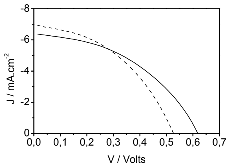
Figura 34. Curva corrente-potencial obtida com uma célula solar sensibilizada pelo extrato etanólico (—) e aquoso (---) de jambolão.
