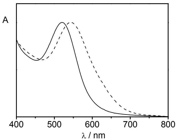
Figura 24. Espectro de absorção do extrato aquoso de jaboticaba (—) e do fotoanodo sensibilizado pelo mesmo (---).
