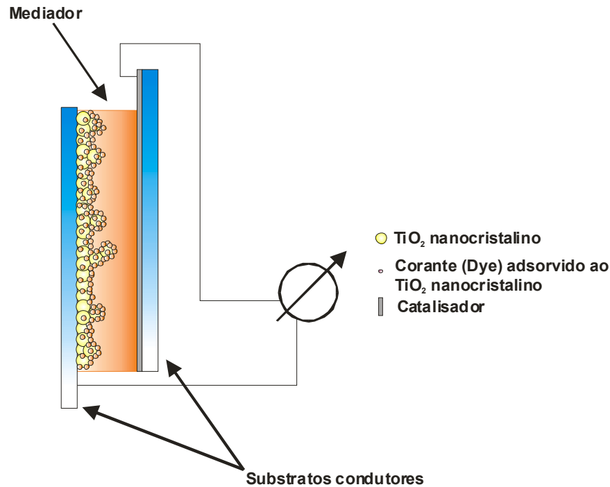
Figura 7. Representação esquemática de uma Dye-Cell ® .
