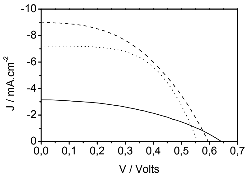
Figura 33. Curva corrente-potencial obtida com uma célula solar sensibilizada pelo extrato de jaboticaba em meio etanólico (—), aquoso (---) e o obtido com água quente (· ·).
