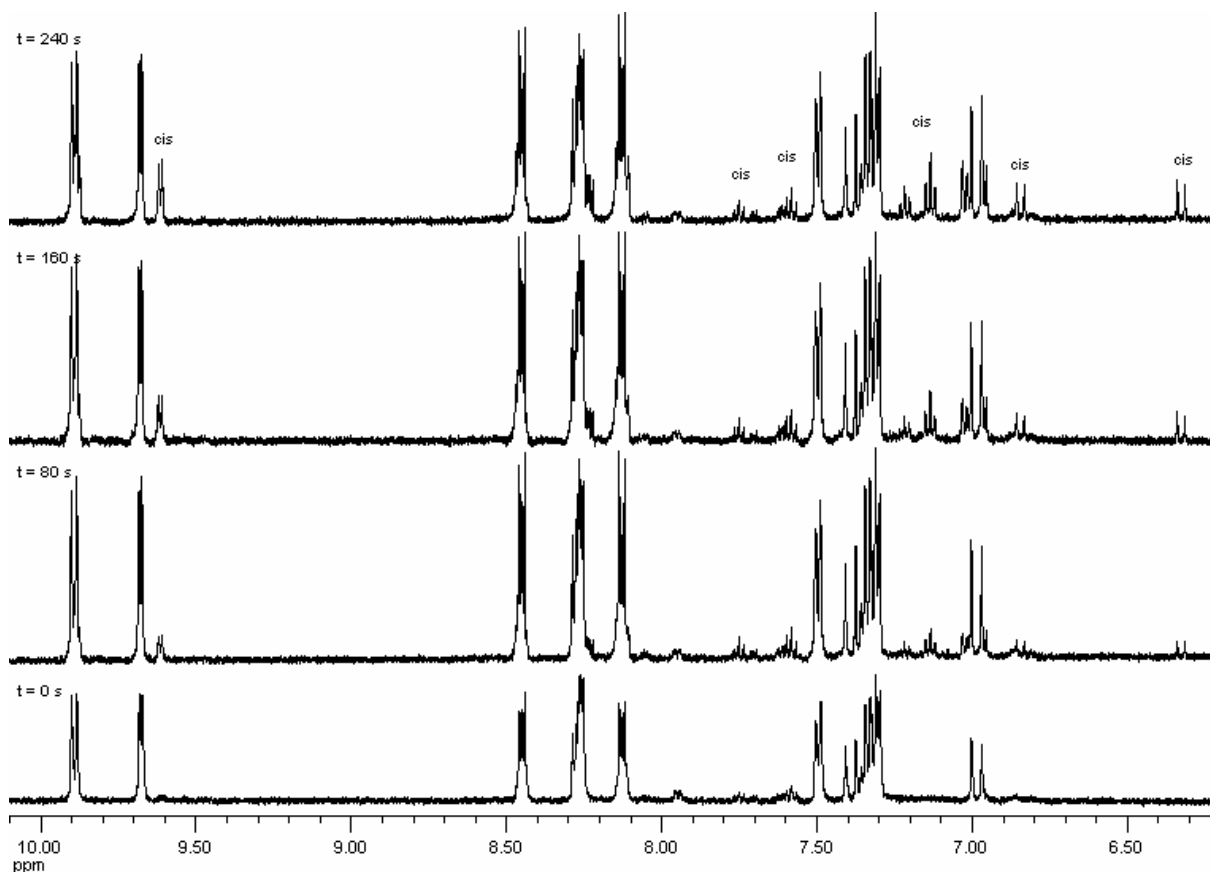
Figura 51. Variação no espectro de ^1\text{H} RMN do composto \text{fac-}[\text{Re}(\text{CO})_3(\text{dppz})(\text{trans-stpy})]^+ em \text{CD}_3\text{CN} após 80, 160 e 240 s sob irradiação em 404 nm. (500 MHz, T = 298\text{ K} )
