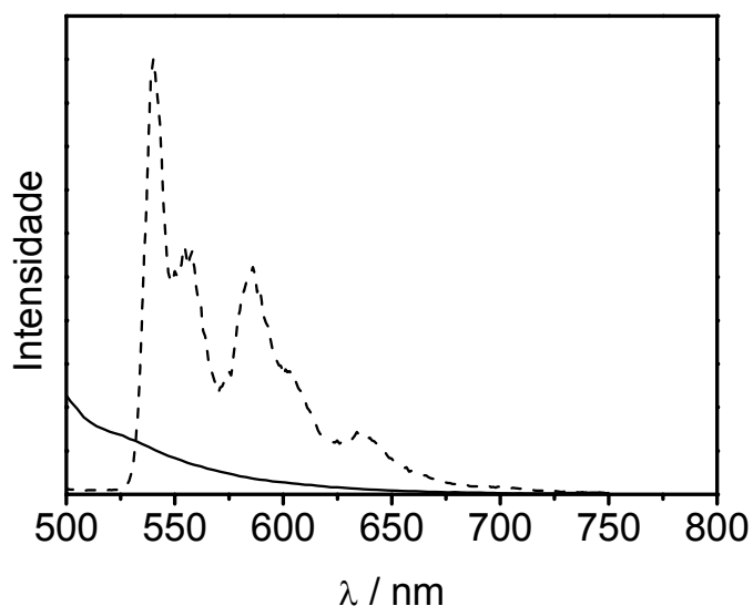
Figura 63. Espectros de emissão do dipirido[3,2-a:2',3'-c]fenazina em EPA a 298 K (—) e a 77 K (---). ( \lambda_{\text{ex}} = 340 \text{ nm} ; \nu = 1 \text{ nm}\cdot\text{s}^{-1} )
