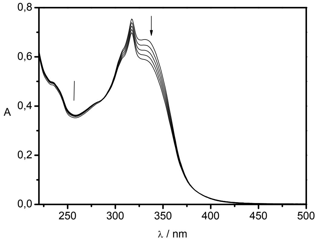
Figura 46. Variações espectrais em função do tempo de irradiação a 404 nm da solução 163 \mu\text{mol}\cdot\text{L}^{-1} do complexo \text{fac-}[\text{Re}(\text{CO})_3(\text{Me}_2\text{bpy})(\text{trans-stpy})]^+ em acetonitrila. ( T = 300 \text{ K} , \Delta t = 60 \text{ s} )
