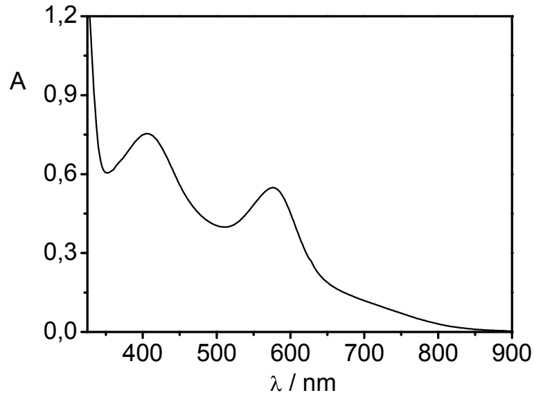
Figura 17. Espectro eletrônico de uma solução do composto cis -[Cl 2 Ru(dobH 2 ) 2 ] em DMF.
