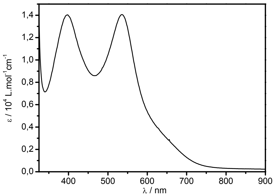
Figura 11. Espectro eletrônico da solução etanólica do cis -[(SCN) 2 Ru(dcbH 2 ) 2 ].
