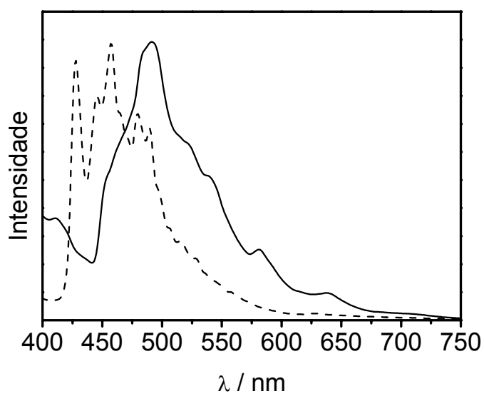
Figura 60. Espectros de emissão dos compostos fac-[Re(CO)_3(bpy)(cis-stpy)]^+ ( \lambda_{ex} = 350 nm) (—) e do ligante bpy ( \lambda_{ex} = 285 nm) (---) em EPA a 77 K. ( \nu = 1 nm·s -1 )
