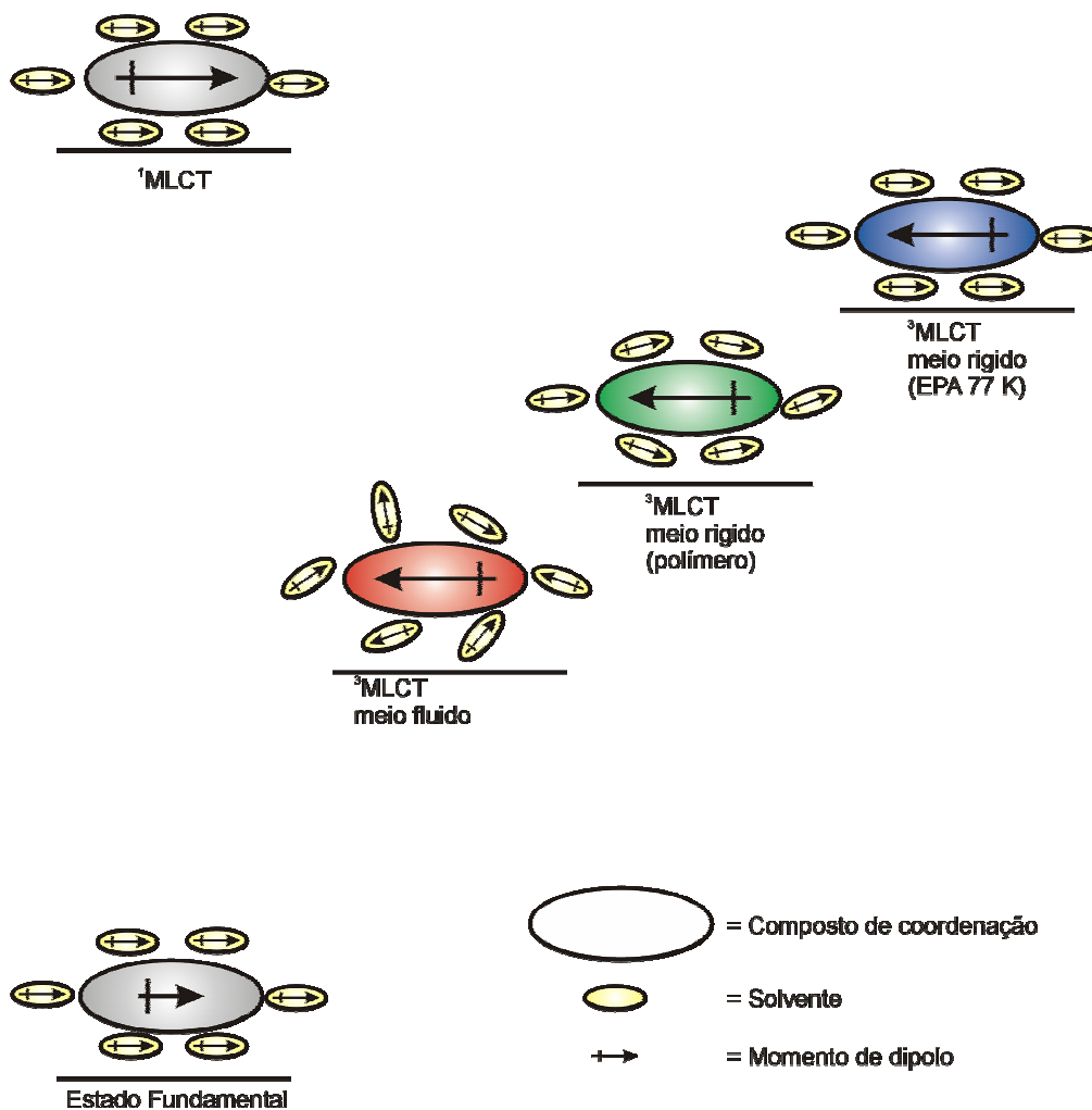
Figura 58. Representação esquemática da orientação do solvente ao redor da espécie no estado fundamental, no estado excitado ^1\text{MLCT} e em diversos meios para o estado ^3\text{MLCT} .
