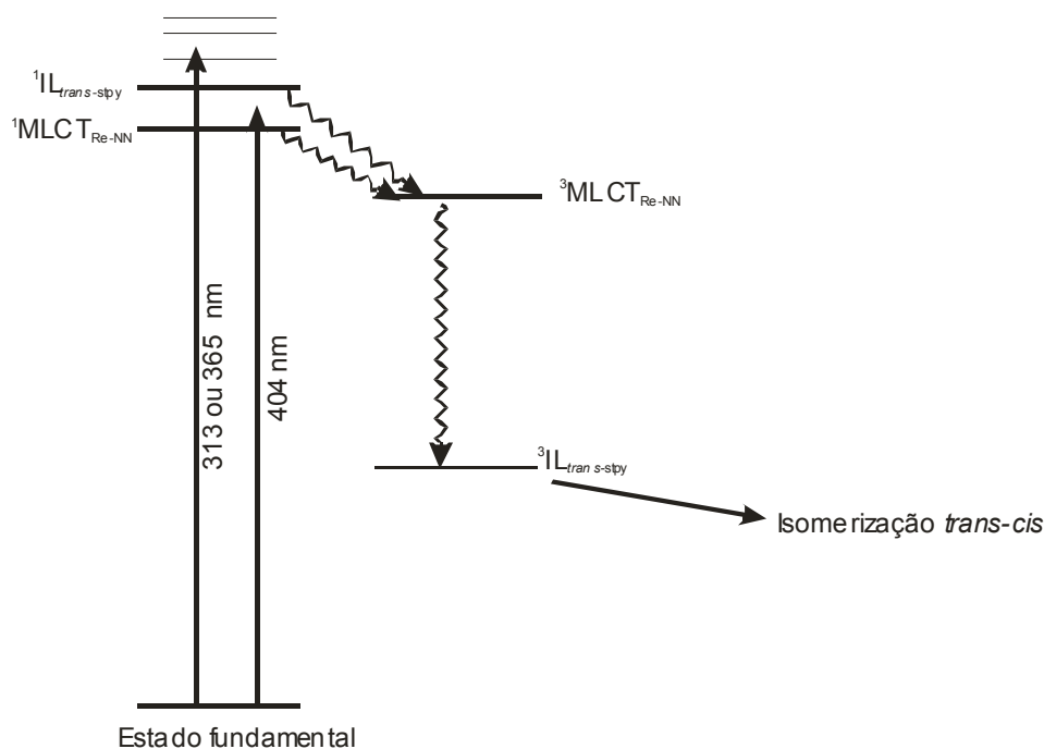
Figura 42. Diagrama de energia proposto para a população do nível de energia responsável pela isomerização trans-cis dos compostos fac-[Re(CO)_3(NN)(trans-stpy)]^+ .
