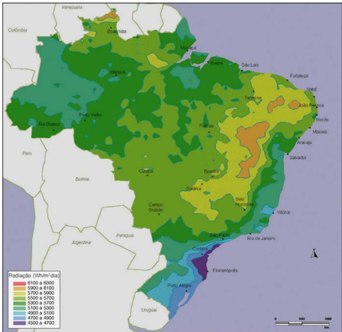
Figura 5. Mapa nacional mostrando a distribuição da radiação solar no Brasil [13].
