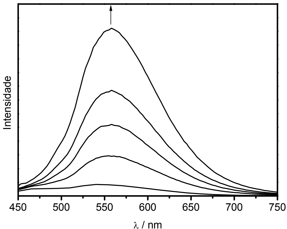
Figura 53. Aumentos do espectro de emissão em função do tempo de irradiação do composto fac-[Re(CO)_3(bpy)(trans-stpy)]^+ em acetonitrila. ( \lambda_{irr} = 365 nm, \lambda_{ex} = 410 nm, t_{irr} = 0, 10, 20, 30 e 50 min)
