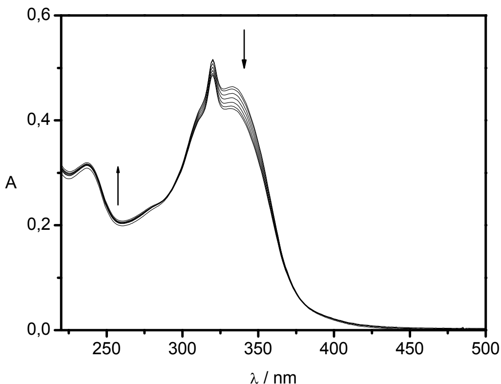
Figura 41. Variações espectrais em função do tempo de irradiação a 404 nm da solução 128 \mu\text{mol}\cdot\text{L}^{-1} do complexo \text{fac-}[\text{Re}(\text{CO})_3(\text{bpy})(\text{trans-stpy})]^+ em acetonitrila. ( T = 300 \text{ K} , \Delta t = 20 \text{ s} )
