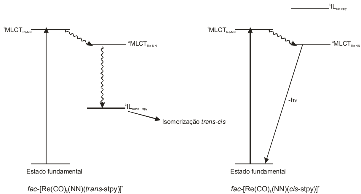
Figura 54. Diagrama simplificado de energia para os compostos fac -[Re(CO) 3 (NN)( trans -stpy)] + e fac -[Re(CO) 3 (NN)( cis -stpy)] + .
