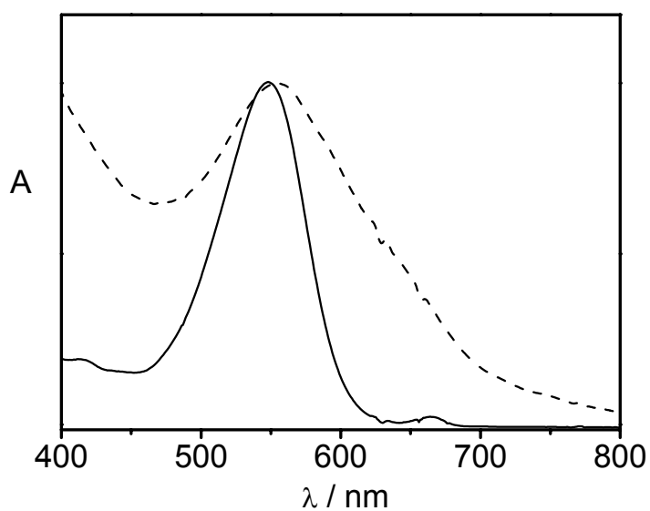
Figura 30. Espectro de absorção do extrato etanólico de maria-preta (—) e do fotoanodo sensibilizado pelo mesmo (---).
