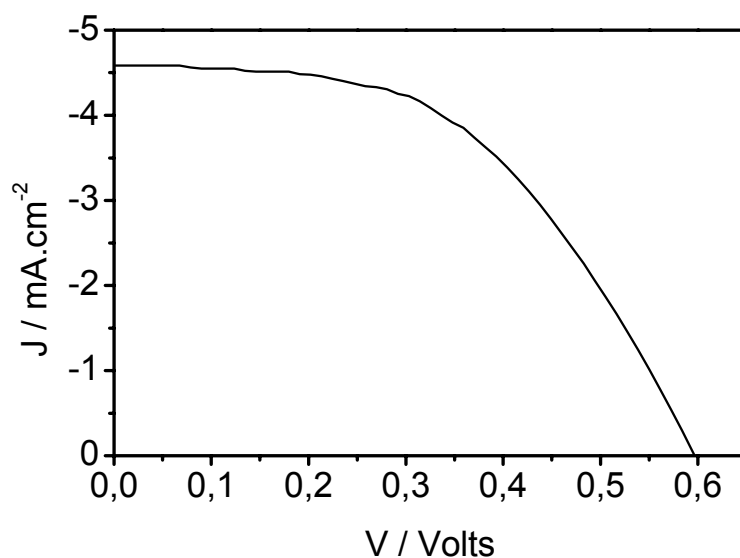
Figura 19. Curva corrente-potencial obtida com uma célula solar sensibilizada pelo corante cis -[Cl 2 Ru(dobH 2 ) 2 ].
