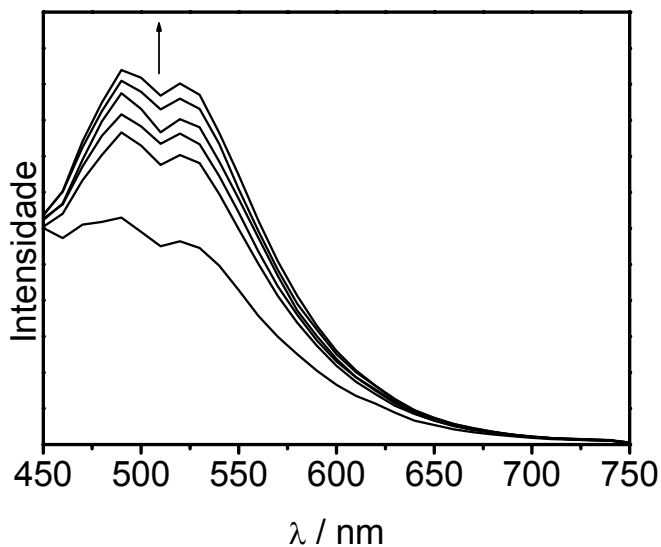
Figura 56. Espectros de emissão do filme contendo o fac-[Re(CO)_3(bpy)(trans-stpy)]^+ em PMMA sob irradiação a 365 nm. ( T=298\text{ K} , \nu=10\text{ nm}\cdot\text{s}^{-1} , \Delta t=60\text{ s} )
