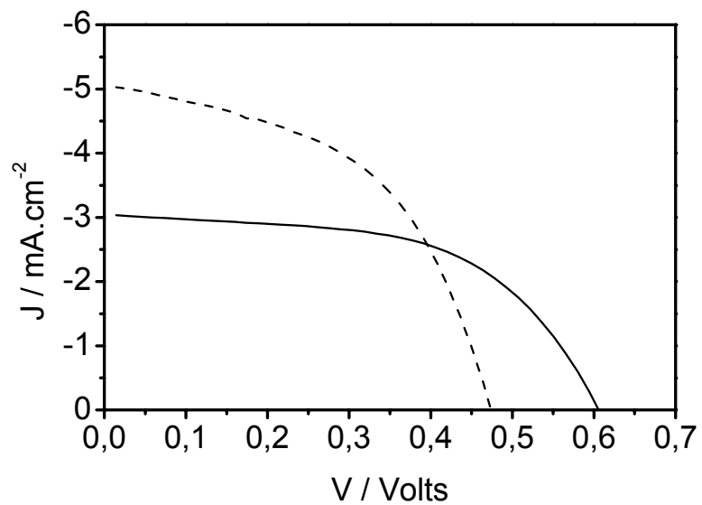
Figura 35. Curva corrente-potencial obtida com uma célula solar sensibilizada pelo extrato etanólico (—) e aquoso (---) de maria-preta.
