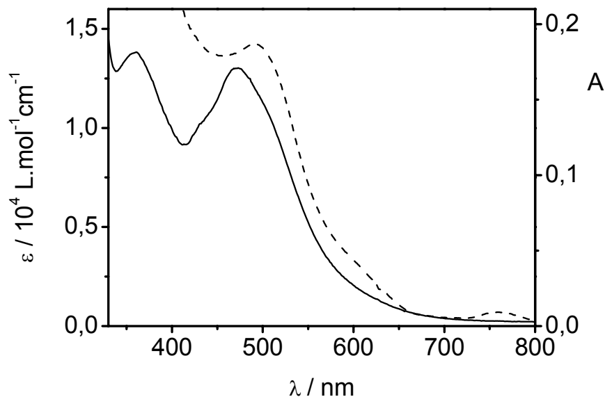
Figura 13. Espectro eletrônico do composto cis -[(H 3 BCN) 2 Ru(dcbH 2 ) 2 ] em solução metanólica (—) e após a sua adsorção à superfície do TiO 2 (---).
