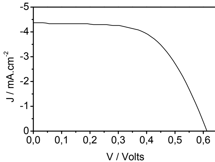
Figura 21. Curva corrente-potencial obtida com uma célula solar sensibilizada pelo corante cis-[Ru(dobH_2)_2(H_2O)_2]^{2+} .
