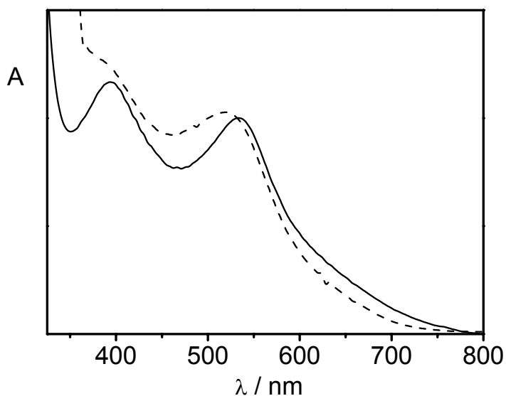
Figura 22. Espectro eletrônico do composto cis -[(SCN) 2 Ru(dobH) 2 ] em solução etanólica (—) e após adsorção à superfície do TiO 2 (---).
