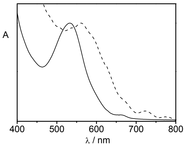
Figura 25. Espectro de absorção do extrato etanólico de jaboticaba (—) e do fotoanodo sensibilizado pelo mesmo (---).
