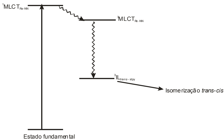
Figura 52. Diagrama simplificado dos níveis de energia para os compostos fac-[Re(CO)_3(NN)(trans-stpy)]^+ .
