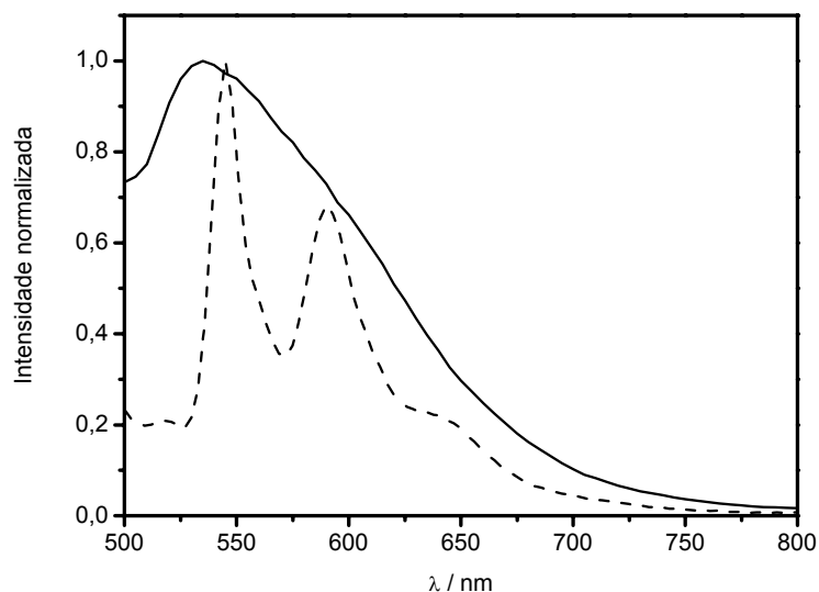
Figura 62. Espectro de emissão \text{fac-}[\text{Re}(\text{CO})_3(\text{dppz})(\text{cis-stpy})]^+ em acetonitrila (—) a 298K e em EPA a 77 K (---). ( \lambda_{\text{ex}} = 450 \text{ nm} , \nu = 5 \text{ nm}\cdot\text{s}^{-1} )
