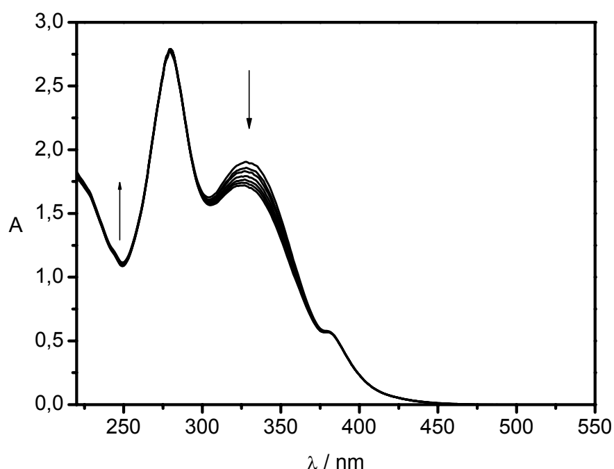
Figura 50. Variações espectrais em função do tempo de irradiação a 404 nm da solução 46,3 \mu\text{mol}\cdot\text{L}^{-1} do complexo fac-[Re(CO)_3(dppz)(trans-stpy)]^+ em acetonitrila. ( T = 300\text{K} , \Delta t = 20 \text{ s} )
