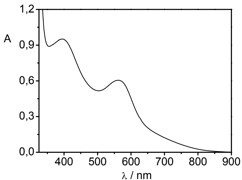
Figura 20. Espectro eletrônico do composto cis -[Ru(dobH 2 ) 2 (H 2 O) 2 ] 2+ em DMF.
