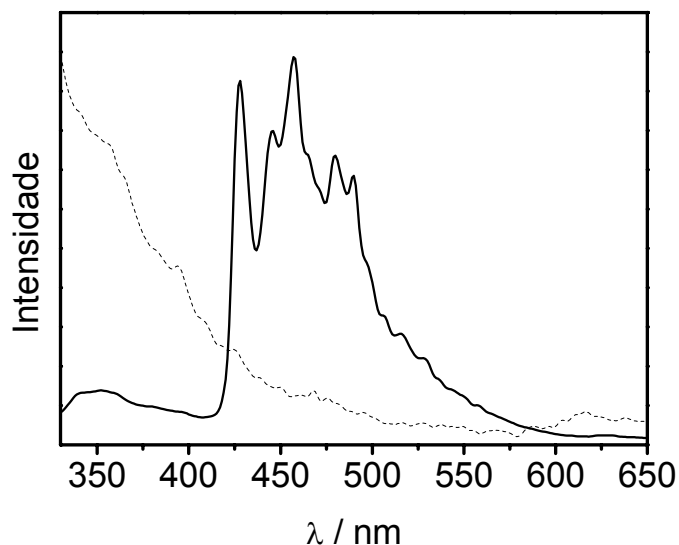
Figura 59. Espectros de emissão do ligante 2,2'-bipiridina em EPA a 77K (—) e a 298 K (---). ( \lambda_{\text{ex}} = 285 \text{ nm} , \nu = 1 \text{ nm}\cdot\text{s}^{-1} ).
