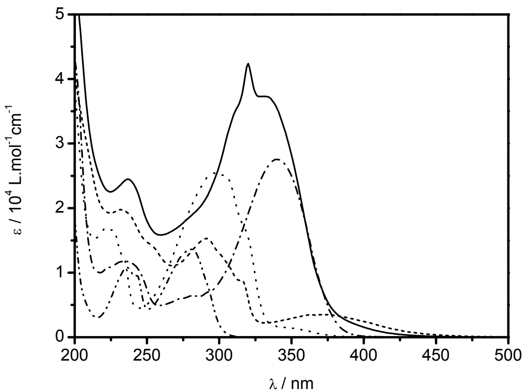
Figura 39. Espectros eletrônicos dos compostos fac\text{-[Re(CO)}_3\text{(bpy)(trans-stpy)]}^+ (—), fac\text{-[ClRe(CO)}_3\text{(bpy)]} (---), trans\text{-stpy} (.....), trans\text{-Hstpy}^+ (-.-.-) e bpy (— · —) em acetonitrila.
