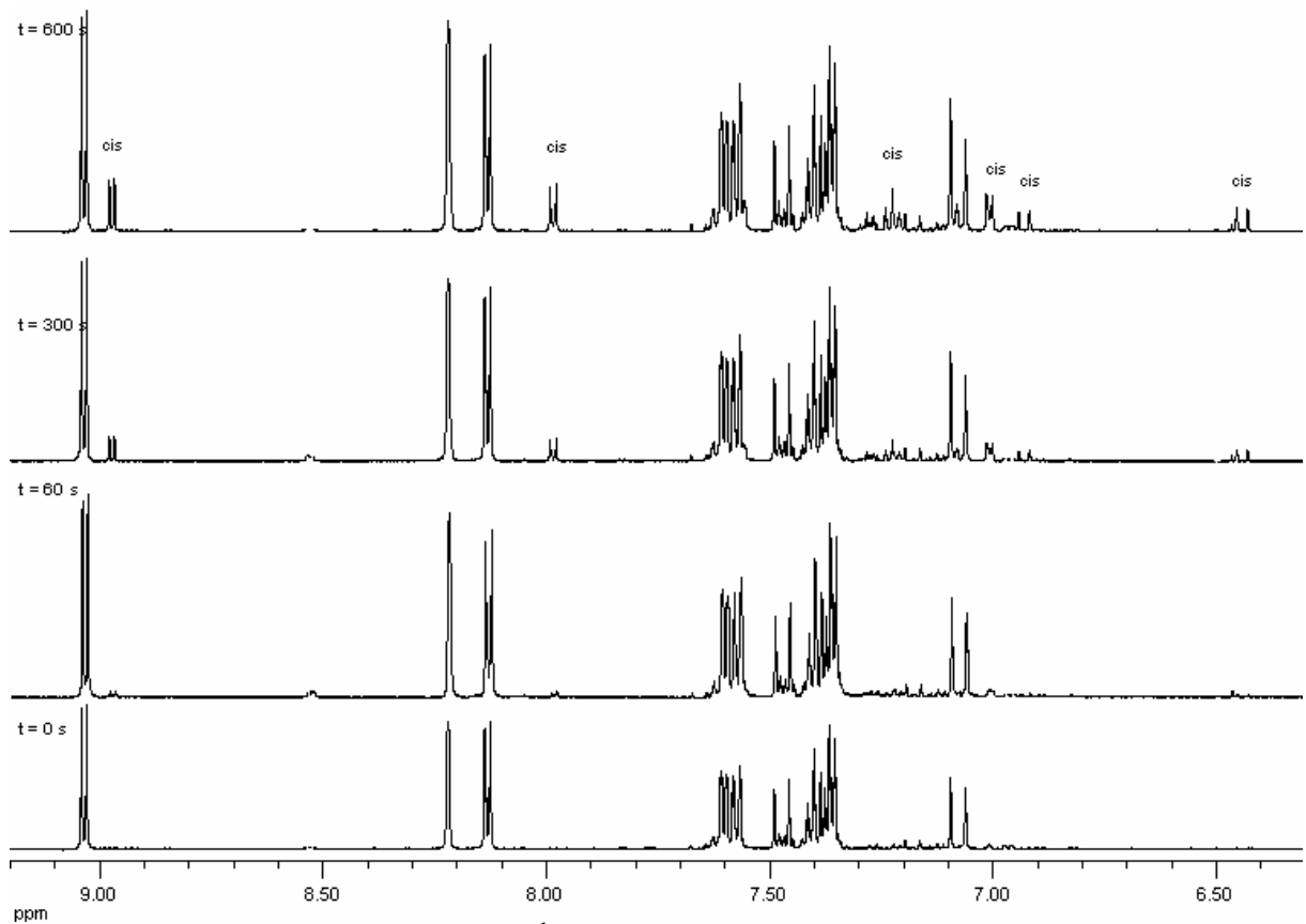
Figura 47. Variação no espectro de ^1\text{H} RMN do composto \text{fac-}[\text{Re}(\text{CO})_3(\text{Me}_2\text{bpy})(\text{trans-stpy})]^+ em \text{CD}_3\text{CN} após 60, 300 e 600 s sob irradiação em 404 nm. (500 MHz, T = 298\text{ K} )
