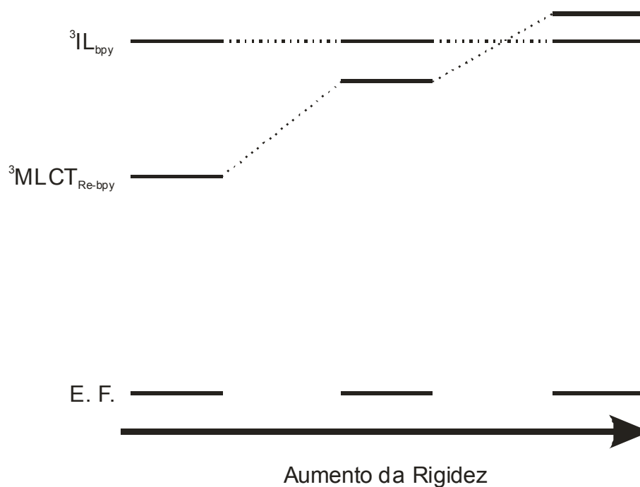
Figura 61 Diagrama simplificado dos níveis de energia do composto fac-[Re(CO)_3(bpy)(cis-stpy)]^+ . (E. F. = Estado fundamental)
