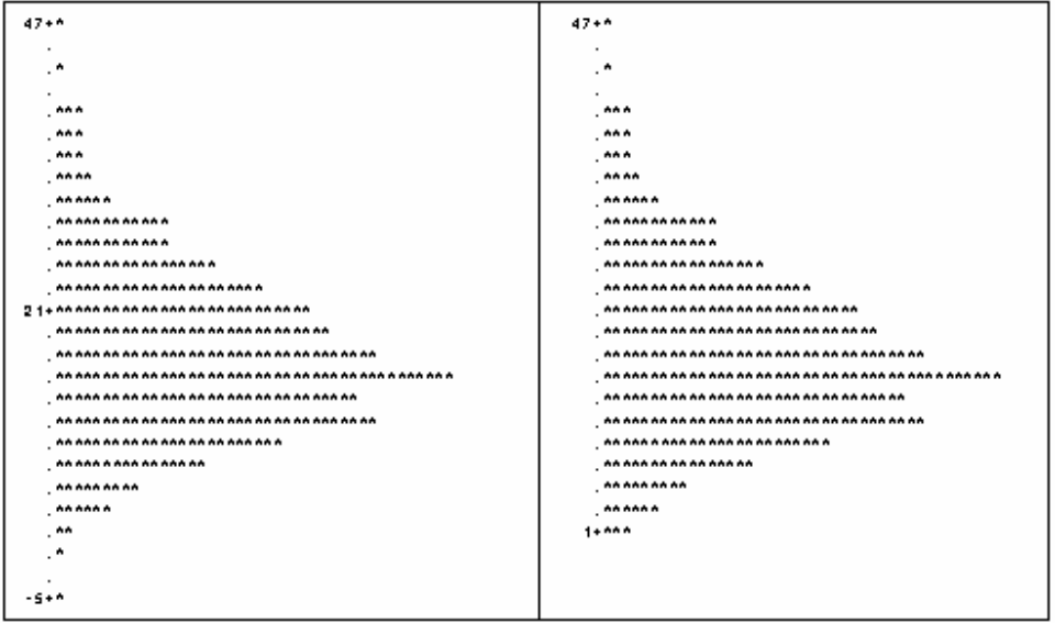
Figura 76 - Histogramas dos conjuntos de dados das estimativas pelos métodos da ANOVA (esquerda) e da MV (direita) do componente de variância relacionado aos tratamentos \sigma_i^2 = 17,1429
