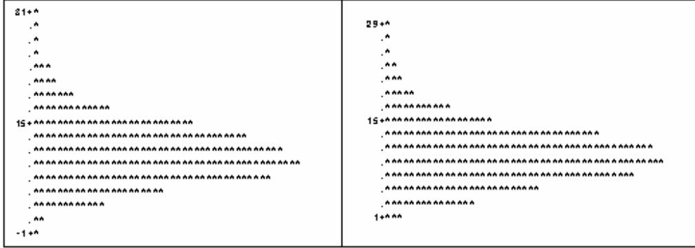
Figura 35 - Histogramas dos conjuntos de dados das estimativas pelos métodos da ANOVA (esquerda) e da MV (direita) do componente de variância relacionado aos tratamentos \sigma_t^2 = 10,6061
