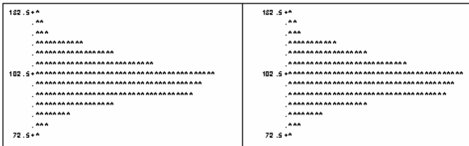
Figura 62 - Histogramas dos conjuntos de dados das estimativas pelos métodos da ANOVA (esquerda) e da MV (direita) do componente de variância relacionado ao erro experimental \sigma^2 = 100
