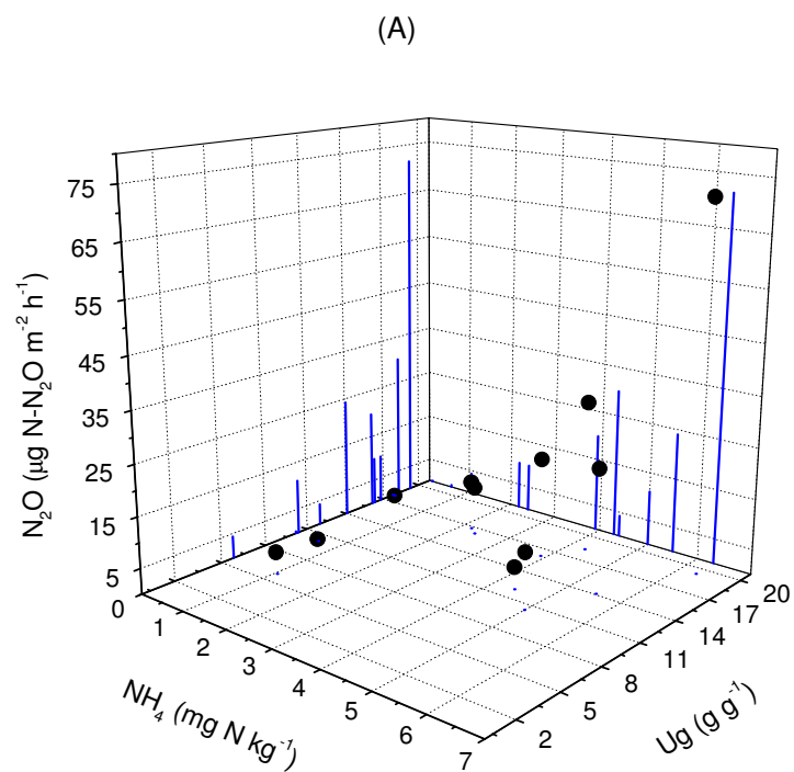
Figura 13. Relação entre as emissões de N_2O com: (A) concentração de amônio no solo ( \text{NH}_4^+ ) e umidade gravimétrica ( U_g ); e (B) concentração de amônio ( \text{NH}_4^+ ) e carbono solúvel em água ( C_s ) no sistema PD E/M 0N. Ano: 2003/2004.
