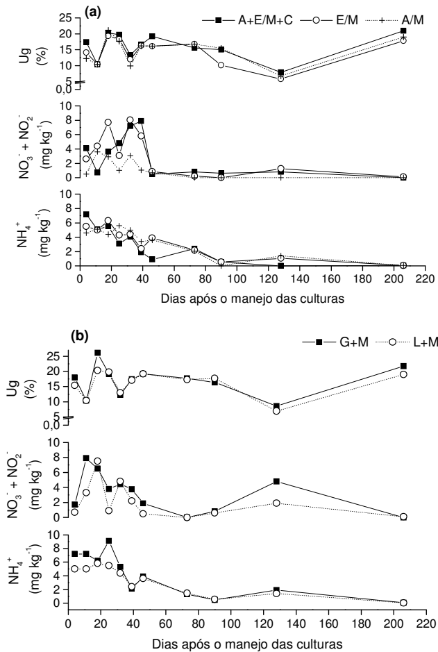
Figura 30. Umidade gravimétrica do solo (Ug), concentrações de amônio ( \text{NH}_4^+ ) e nitrato + nitrito ( \text{NO}_2^- + \text{NO}_3^- ) no solo analisadas em amostras (camada de 0 a 20 cm) coletadas dos sistemas de manejo que incluem as leguminosas de inverno em sucessão com o milho e em consórcio com a aveia (a), e nos sistemas que incluem as leguminosas de verão semeadas em consórcio com o milho (b). Ano de 2003/2004.
