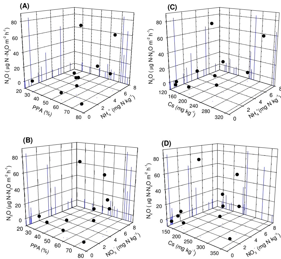
Figura 23. Relação entre emissões de N_2O com: (A) concentração de amônio ( \text{NH}_4^+ ) e porosidade preenchida por água (PPA); (B) concentração de nitrato+nitrito ( \text{NO}_3^- + \text{NO}_2^- ) e porosidade preenchida por água (PPA); (C) concentração de amônio ( \text{NH}_4^+ ) e carbono solúvel em água (Cs); e (D) concentração de nitrato + nitrito ( \text{NO}_3^- + \text{NO}_2^- ) no solo e carbono solúvel em água (Cs) no sistema A+E/M+C. Ano 2003/2004.
