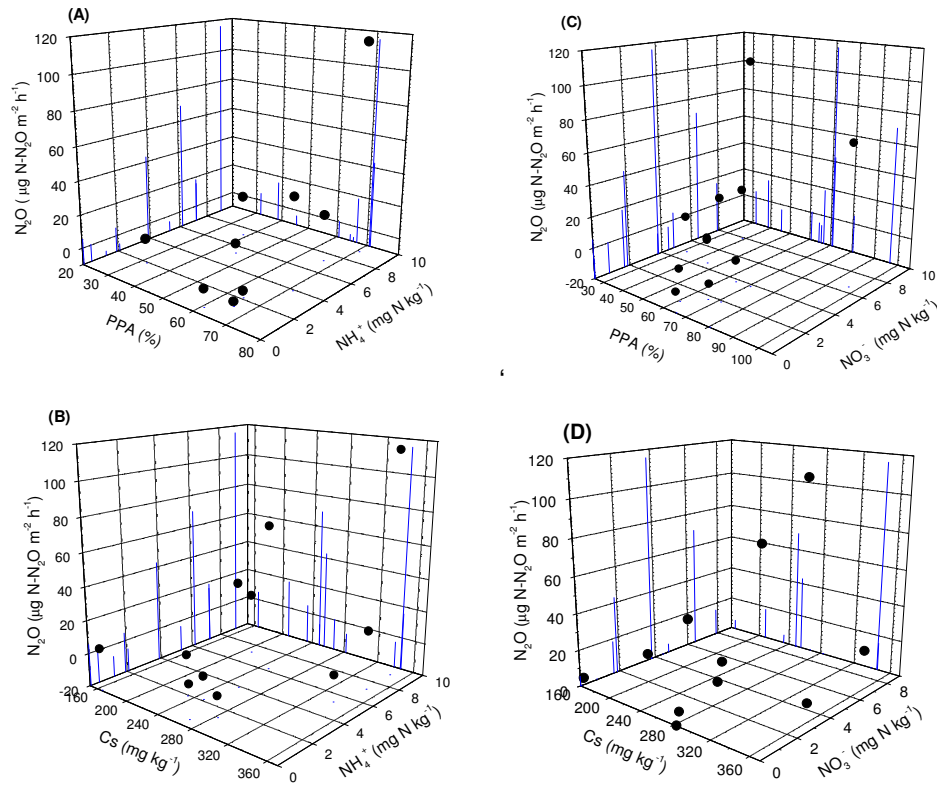
Figura 24. Relação entre emissões de N_2O com: (A) concentração de amônio ( \text{NH}_4^+ ) e porosidade preenchida por água (PPA); (B) concentração de amônio ( \text{NH}_4^+ ) no solo e carbono solúvel em água (Cs); (C) concentração de nitrato+nitrito ( \text{NO}_3^-+\text{NO}_2^- ) e PPA; e (D) concentração de nitrato+nitrito ( \text{NO}_3^-+\text{nitrito} ) no solo e carbono solúvel em água (Cs) no sistema PD G+M. Ano 2003/2004.
