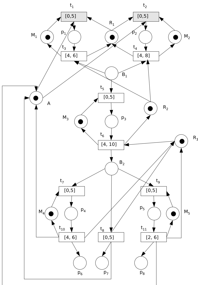
Figura 70: Rede de Petri temporal da planta
