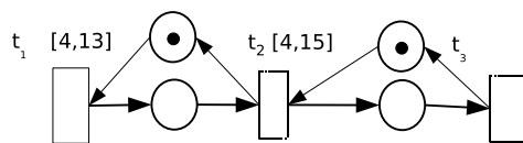
Figura 74: Rede acíclica e segura
