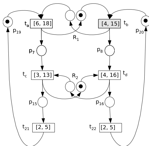
Figura 59: RPT reduzida representando as tarefas
