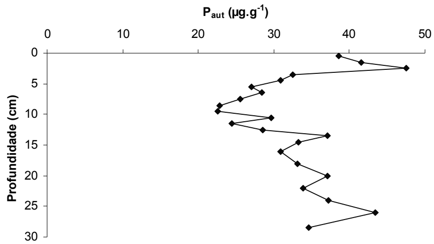
Figura 27. Distribuição das concentrações de fósforo autigênico ( P_{aut} ) ao longo do testemunho P1.
