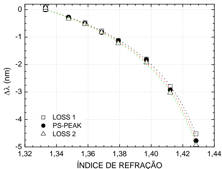
Figura 40 - Resposta em comprimento de onda da PS-LPG01 quando o índice de refração circunvizinho à rede é alterado. Os espectros usados para a obtenção dessa resposta são aqueles obtidos na configuração convencional de leitura de LPG.
