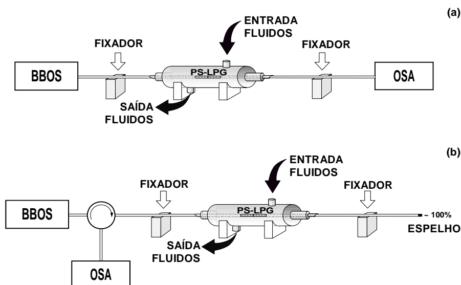
Figura 13 - Montagem experimental para medida de índice de refração usando (a) os espectros de transmissão da PS-LPG e (b) os espectros de reflexão da PS-LPG.
