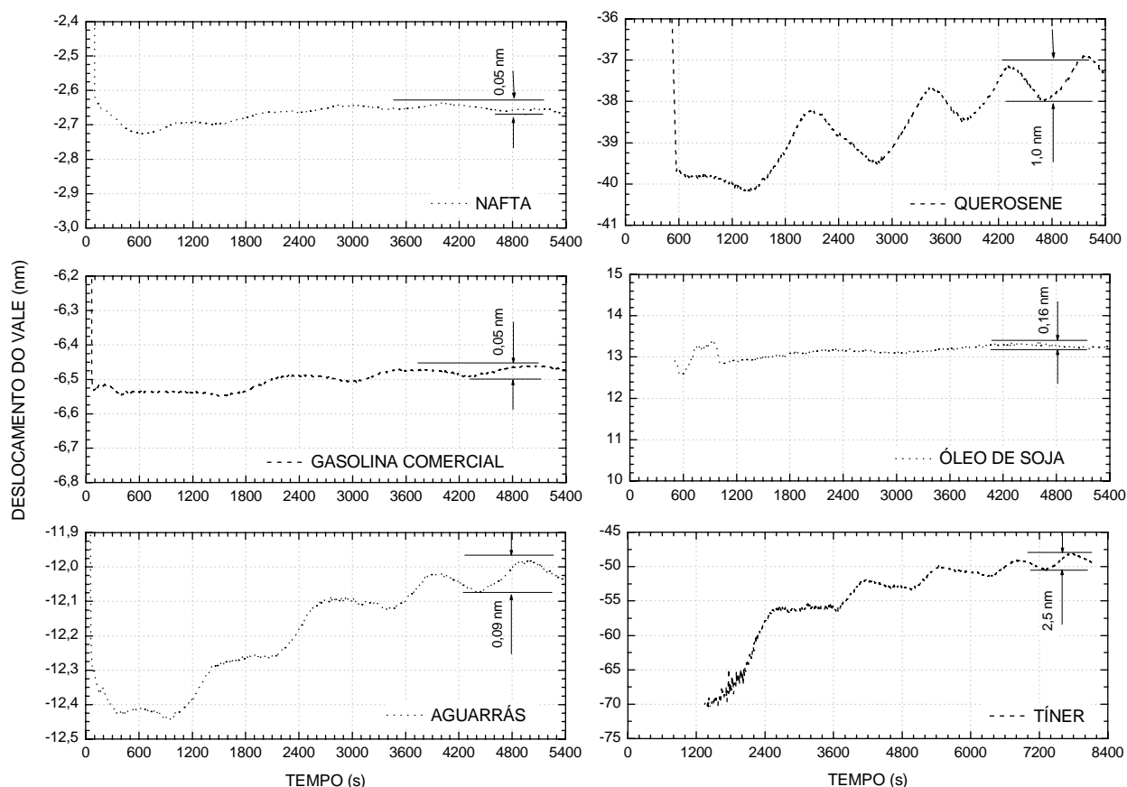
Figura 32 - Evolução temporal da LPG na presença das substâncias usadas nos experimentos de medida de índice de refração. Os deslocamentos do vale com a utilização das substâncias da coluna da esquerda são menores do que 0,10 nm, enquanto que com as substâncias da coluna da direita são maiores do que 0,16 nm.
