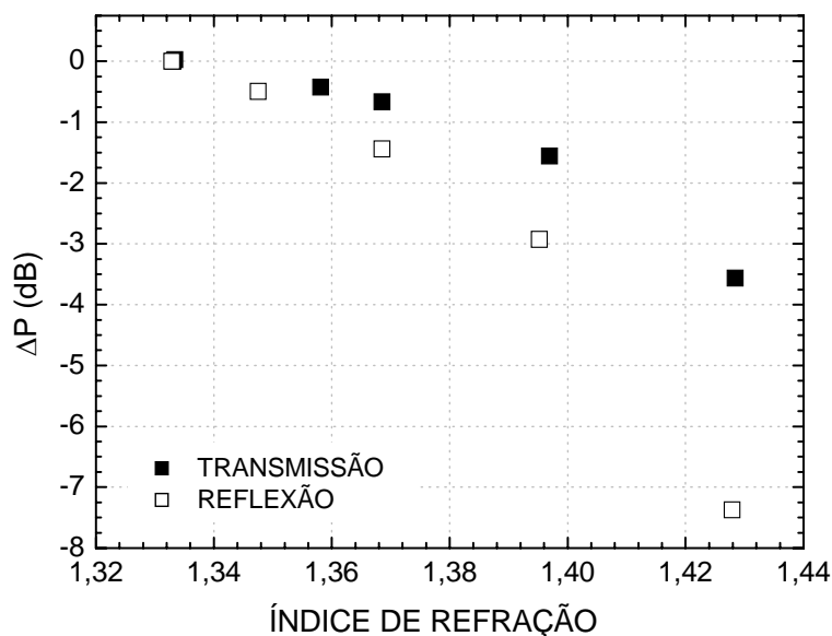
Figura 41 - Variação da potência óptica em 1552,8 nm como função da mudança do índice de refração do meio externo para as medidas de espectro na transmissão e na reflexão.
