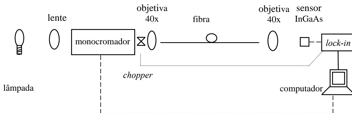
Figura 55 - Sistema de leitura de espectros no infravermelho com monocromador [180].
