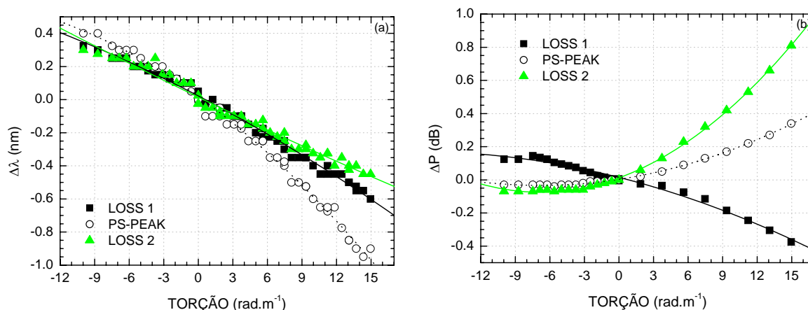
Figura 53 - Resposta da PS-LPG em (a) comprimento de onda e (b) amplitude devido à torção aplicada.
