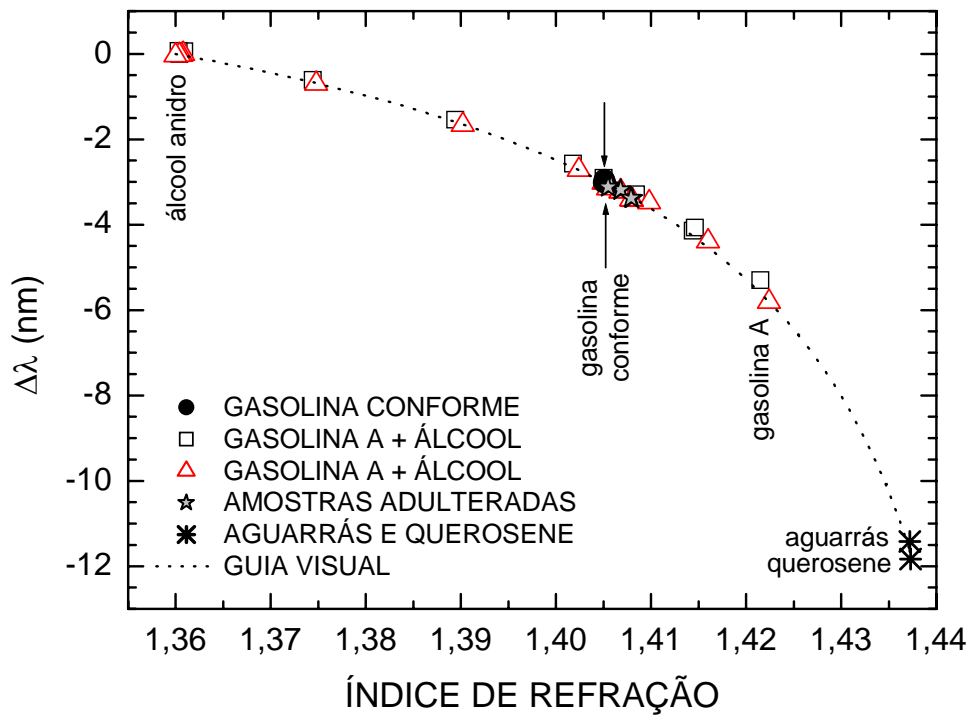
Figura 35 - Sensibilidade da LPG ao índice de refração.
