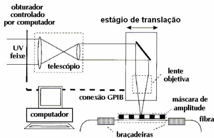
Figura 6 - Montagem experimental de fabricação de LPG, alternável entre o método ponto-a-ponto e máscara de amplitude [155].
