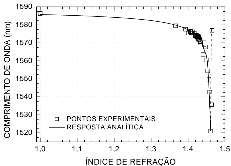
Figura 22 - Posição do vale de atenuação no espectro de transmissão de uma LPG ( \Lambda = 649 nm, 53 pontos) como função do índice de refração do meio externo a 20 °C (a linha pontilhada é um guia visual). As incertezas nos pontos medidos são menores que o tamanho do símbolo [182].
