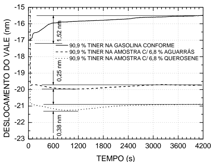
Figura 31 - Evolução temporal da LPG quando ela estava imersa em diferentes subamostras de gasolina com tiner. O deslocamento máximo do vale de atenuação é de aproximadamente 1,52 nm para a amostra de gasolina comercial contendo 90,9 % de tiner.
