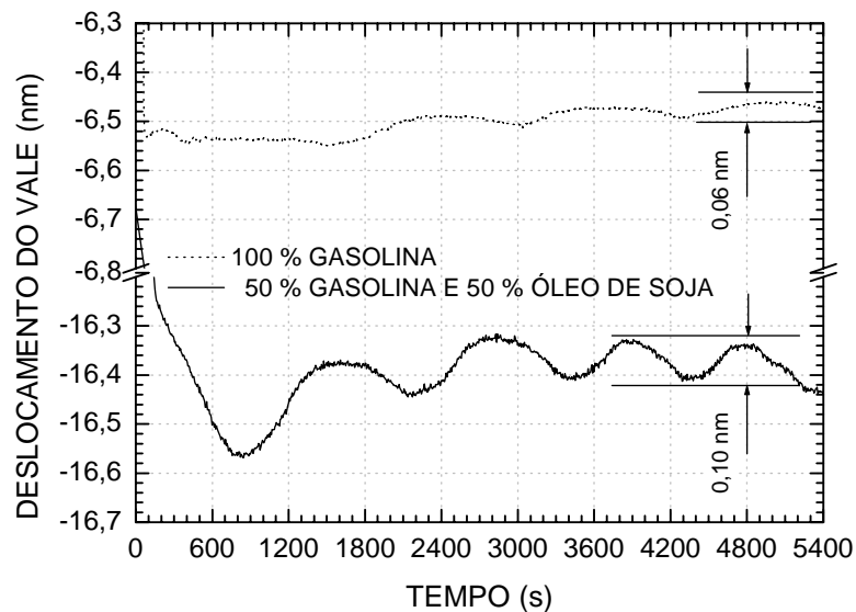
Figura 33 - Evolução temporal da LPG quando ela é imersa na gasolina comercial e numa mistura contendo 50 % de gasolina comercial e 50 % de óleo de soja.
