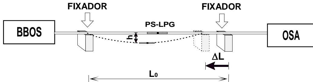
Figura 17 - Montagem experimental para medida da sensibilidade a deformação longitudinal ( \Delta L < 0 ) e curvatura da PS-LPG ( \Delta L > 0 ).
