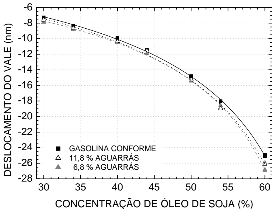
Figura 34 - Determinação da conformidade da gasolina usando como substância de referência o óleo de soja.
