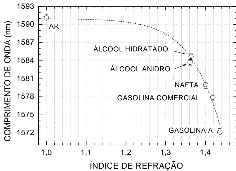
Figura 22 - Posição do vale de atenuação no espectro de transmissão de uma LPG ( \Lambda = 649 nm, 53 pontos) como função do índice de refração do meio externo a 20 °C (a linha pontilhada é um guia visual). As incertezas nos pontos medidos são menores que o tamanho do símbolo [182].
