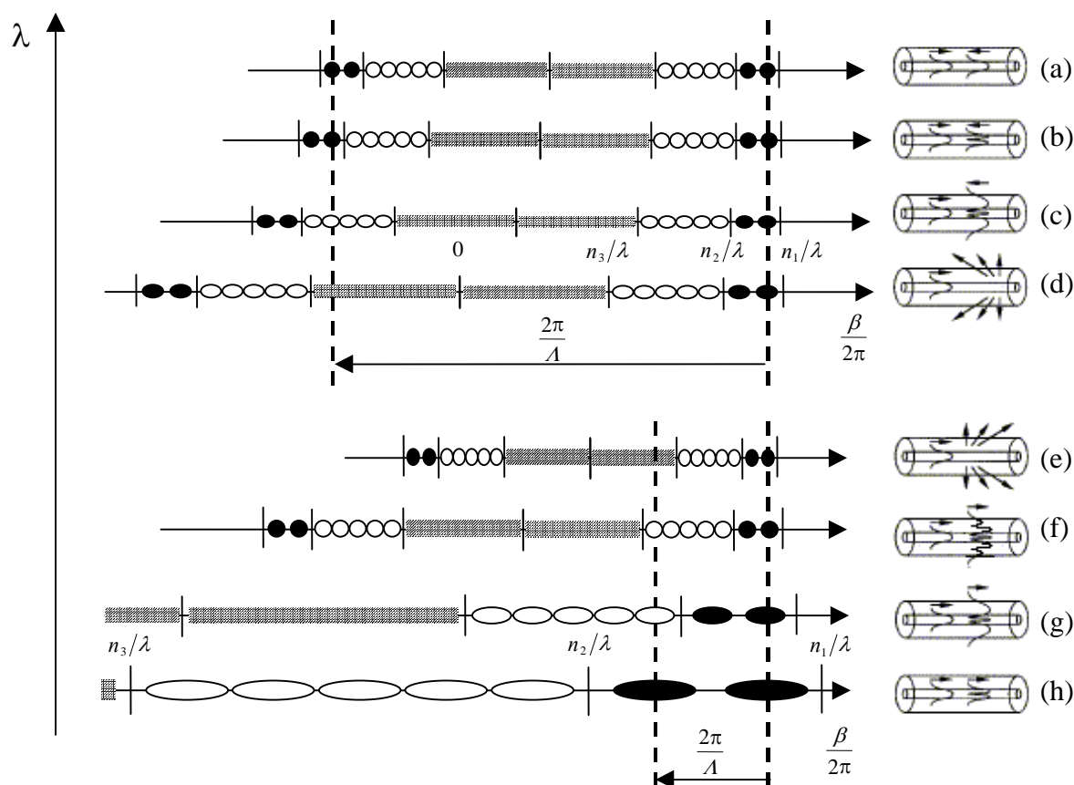
Figura 4 - Diagramas que ilustram as condições de casamento de fase necessárias para ocorrer ressonância entre dois modos por um período da rede de \Lambda . As figuras de (a)-(e) e (g)-(h) foram retiradas de [146].
