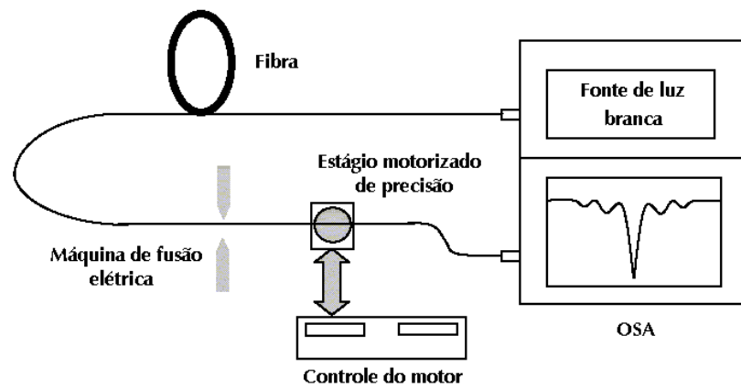
Figura 8 - Diagrama esquemático da montagem para a fabricação de redes de período longo usando descarga de arco elétrico (figura retirada da referência [39]).
