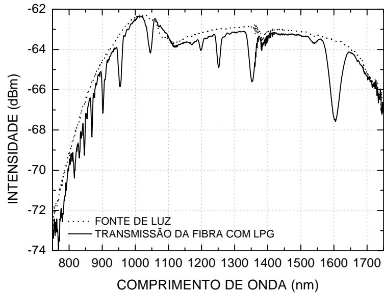
Figura 20 - Espectro de transmissão com ampla faixa espectral obtido no INESC Porto/UOSE para uma fibra óptica antes (curva pontilhada) e após a fabricação de uma LPG (curva contínua).
