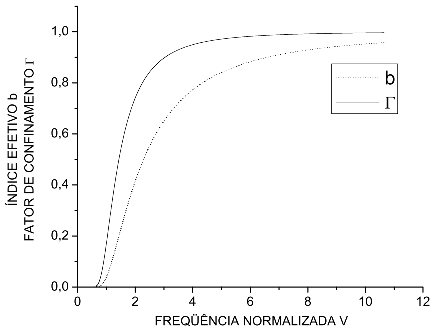
Figura 2.5: Comportamento do fator de confinamento e do índice efetivo do modo fundamental ( l = 0 ).
