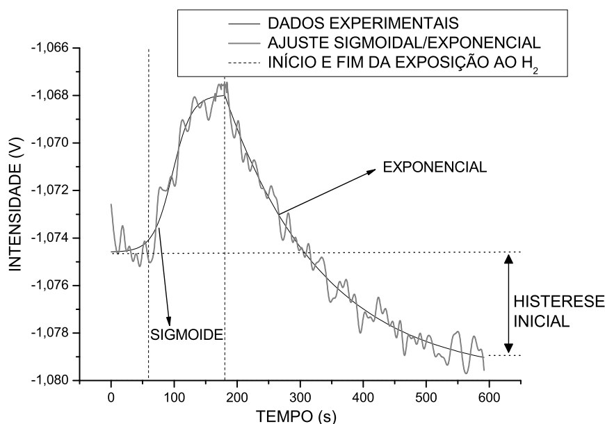
Figura 5.6: Curva obtida após expor-se o sensor a 3.5% de hidrogênio. As barras verticas tracejadas ilustram o instante de início e fim do fluxo de hidrogênio.
