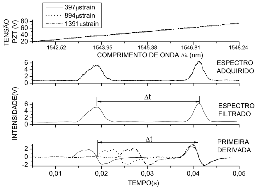
Figura 4.16: Sinais envolvidos na obtenção das curvas durante caracterização com DTG. No topo, o sinal aplicado ao PZT; no segundo gráfico, o sinal adquirido sem filtragem; no terceiro, o espectro filtrado dos sensores onde se ilustra a distância medida entre picos, \Delta t_{\text{pico}} ; no último, o sinal da primeira derivada do espectro filtrado.
