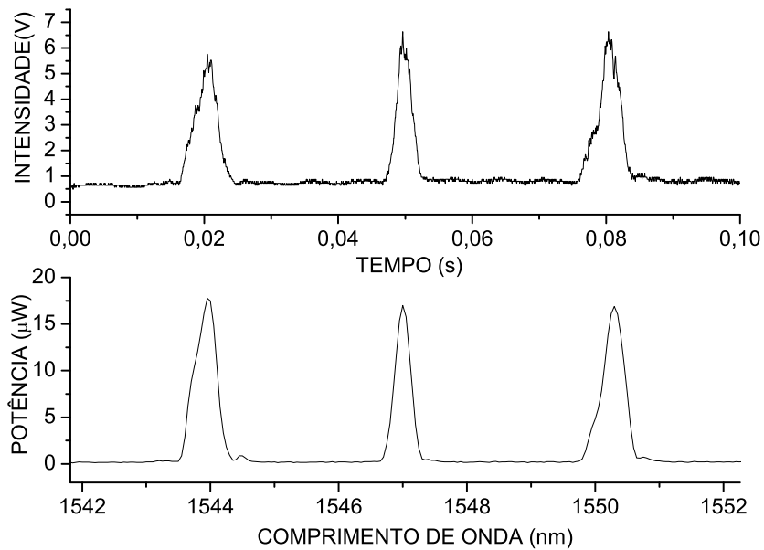
Figura 4.15: Espectros de três sensores obtidos com o laser sintonizável pela DTG (topo) e com o OSA(baixo).
