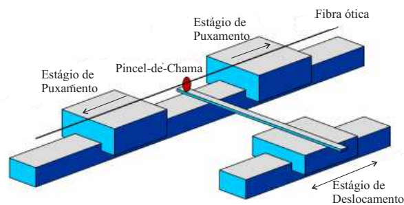
Figura 5.2: Esquema do método do pincel-de-chama em que uma chama percorre a região de estreitamento enquanto a fibra é esticada.
