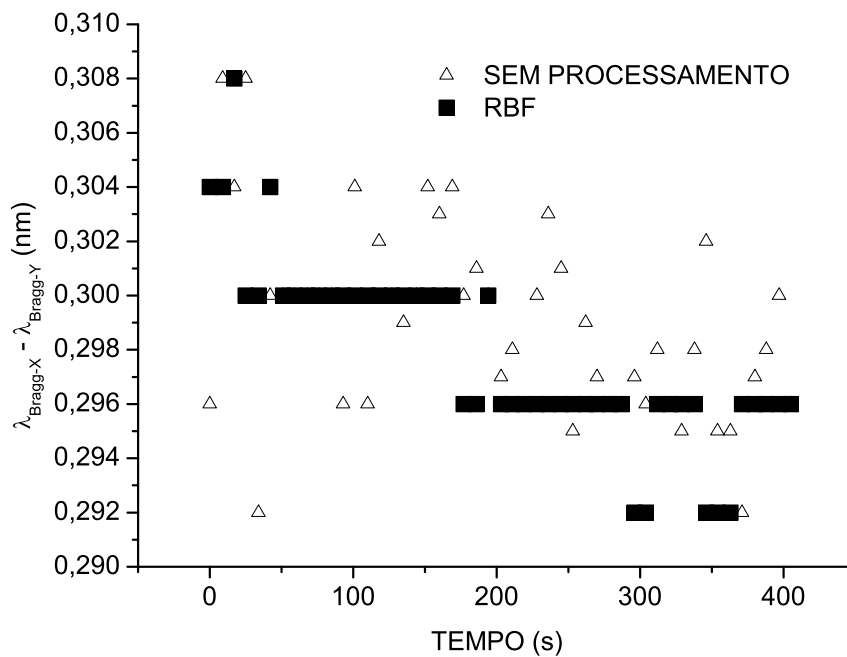
Figura 3.10: Evolução da diferença \lambda_{Bragg-X} - \lambda_{Bragg-Y} entre os picos das bandas de reflexão em um sensor a FBG em fibra ótica HIBI para monitoração da contração radial de uma resina polimérica odontológica.
