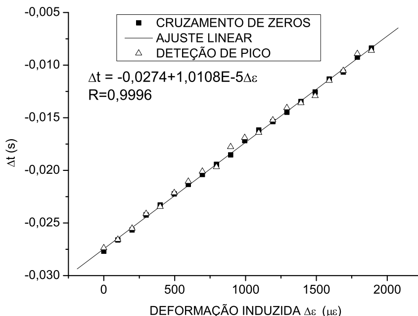
Figura 4.17: Pontos experimentais e reta de ajuste para caracterização da resposta do sistema com laser e DTG. Os pontos foram obtidos para distâncias temporais entre pontos de cruzamento de zero e picos do espectro em função da deformação aplicada a um dos sensores.
