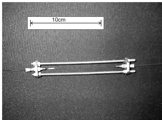
Figura 5.4: Suporte com chapas sextavadas e parafusadas para evaporação do filme fino de paládio sobre o sensor.
