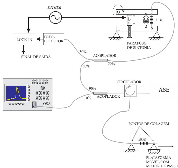
Figura 4.1: Diagrama esquemático do circuito óptico e do aparato de modulação da FBG interrogadora. Linhas cinzas grossas representam fibras ópticas; linhas pretas grossas representam circuito elétrico e linhas pretas finas representam direção de movimento.
