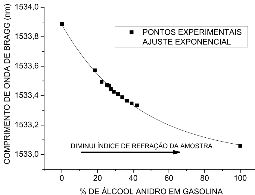
Figura 5.12: Comprimento de onda de Bragg em função da porcentagem de álcool na gasolina da amostra envolvendo o sensor com raio 6\ \mu\text{m} . A curva contínua é a aproximação por uma exponencial de primeira ordem. Os pontos foram medidos para gasolina pura, álcool puro e para concentrações entre 20% e 45%.
