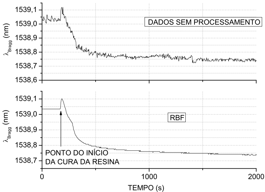
Figura 3.11: Comparação entre as curvas sem processamento e com processamento por meio de rede neural RBF na deformação durante a polimerização em resina odontológica medida com sensor a FBG.
