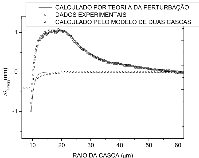
Figura 5.10: Curvas mostrando o comportamento da variação do comprimento de onda de Bragg da FBG com casca corroída em função do raio da casca, para os casos experimental, simulado com teoria da perturbação e com a solução da equação de dispersão para o modelo de duas cascas.
