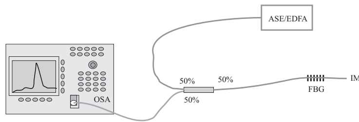
Figura 3.1: Diagrama representando esquema para monitoração do espectro de reflexão de uma FBG. Uma fonte de banda larga (ASE/EDFA) ilumina a FBG, cujo sinal refletido é adquirido por um analisador de espectros óticos (OSA). Linhas cinzas representam fibras óticas.
