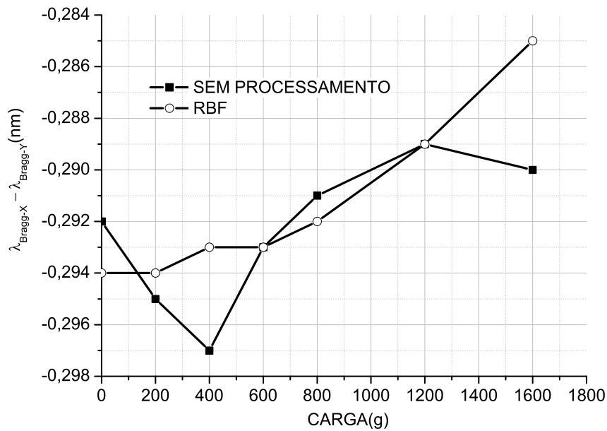
Figura 3.12: Medidas da diferença entre os comprimentos de onda de Bragg para as duas bandas em um sensor a FBG em fibra HIBI instalado em um maxilar metálico quando aplicadas as forças ortodônticas.
