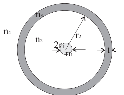
Figura 5.3: Seção transversal de um sensor em taper com raio de núcleo r_1 e índice n_1 , raio de casca r_2 e índice n_2 , envolvido por um filme metálico de índice n_3 e espessura t , num ambiente de índice de refração n_4 .
