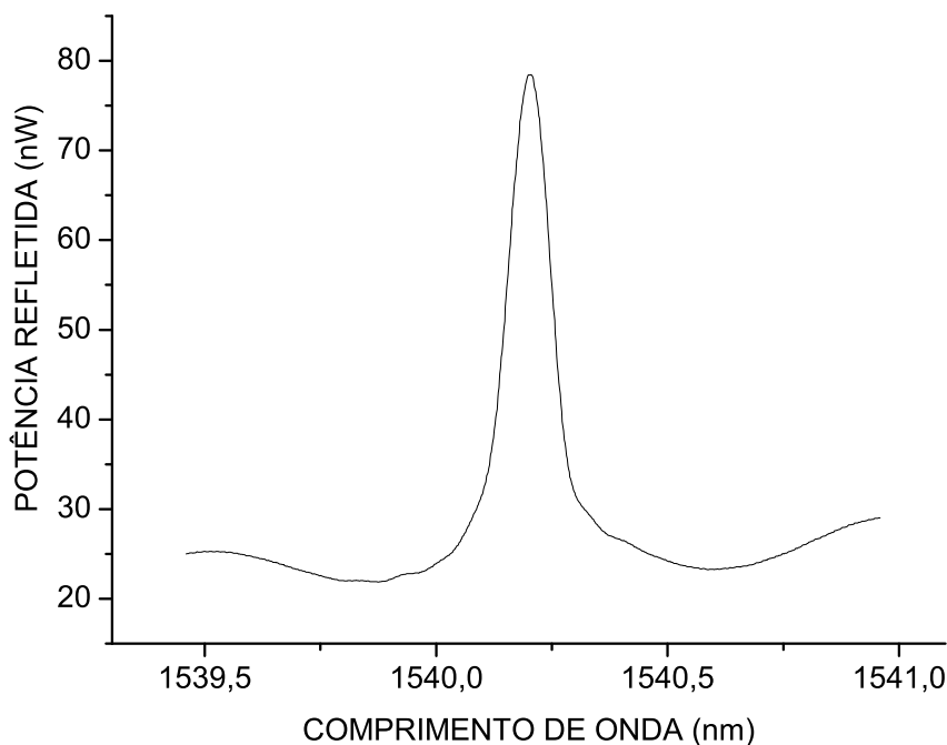
Figura 4.13: Espectro da DTG sintonizável utilizada no laser.
