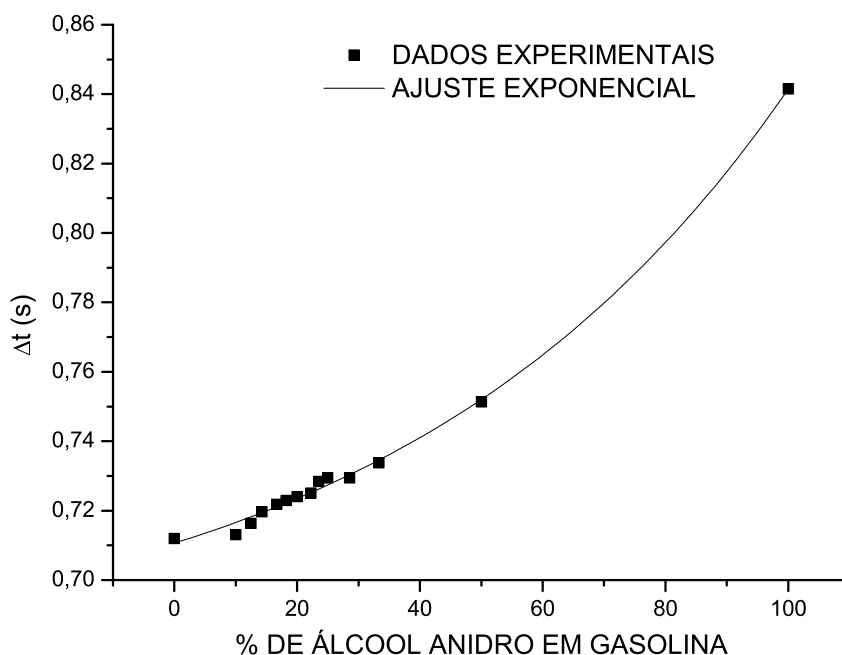
Figura 5.13: Diferença temporal entre os pontos de cruzamento de zero em função da porcentagem de álcool na gasolina da amostra envolvendo o sensor com raio 10\ \mu\text{m} . A curva contínua é a aproximação por uma exponencial de primeira ordem. Os pontos foram medidos para gasolina pura, álcool puro e para concentrações entre 10% e 50% de álcool em gasolina.
