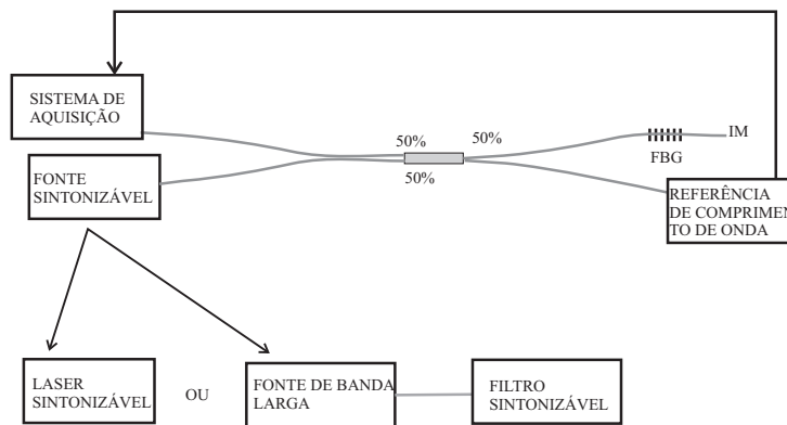
Figura 3.2: Diagrama representando esquema para monitoração do espectro de reflexão de uma FBG com uma fonte sintonizável, que pode ser um laser sintonizável ou fonte de banda larga seguida de um filtro sintonizável. Linhas cinzas representam fibras óticas. (IM=gel casador de índice)
