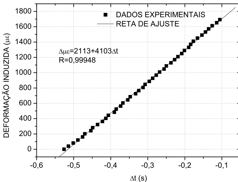
Figura 4.8: Curva de resposta da deformação em função do intervalo temporal caracterizando a sensibilidade do sistema.
