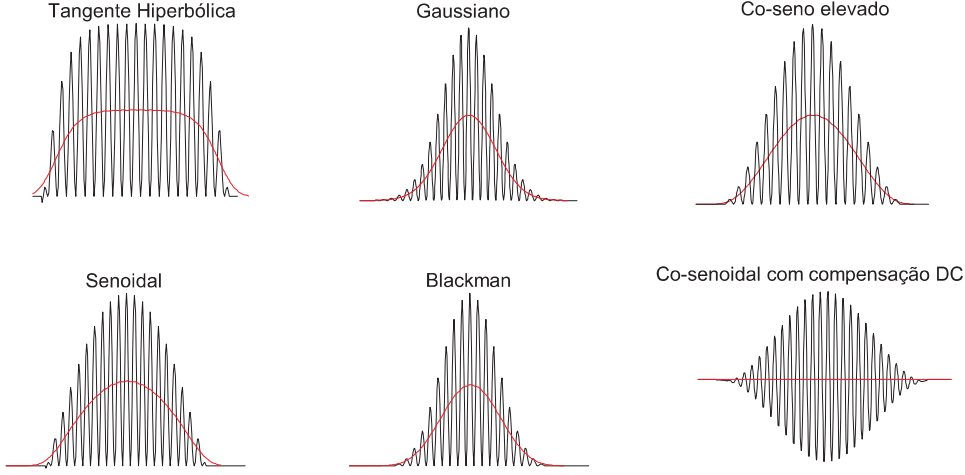
Figura 2.2: Perfis de modulação de índice do núcleo para uma FBG típica. A linha vermelha ilustra o comportamento do valor médio da perturbação. Da esquerda para direita, na primeira linha, os perfis tangente hiperbólica, gaussiano e co-seno elevado; na segunda linha, os perfis senoidal, Blackman e co-senoidal com compensação DC, neste caso o valor médio da perturbação é nulo.
