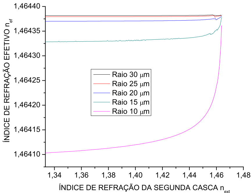
Figura 5.11: Variação do índice de refração efetivo do modo de propagação fundamental em função do índice do ambiente do sensor (segunda casca). As curvas foram calculadas resolvendo a equação de dispersão para o modelo de duas cascas.
