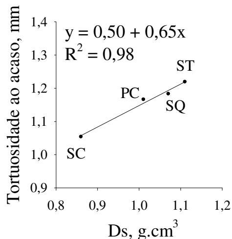
Figura 14. Relação entre a tortuosidade ao acaso da superfície do solo e a densidade do solo, D_s , da camada de 0,5 - 3,0 cm de um Nitossolo Háplico alumínico, submetidos à escarificação mecânica (média de duas repetições).
