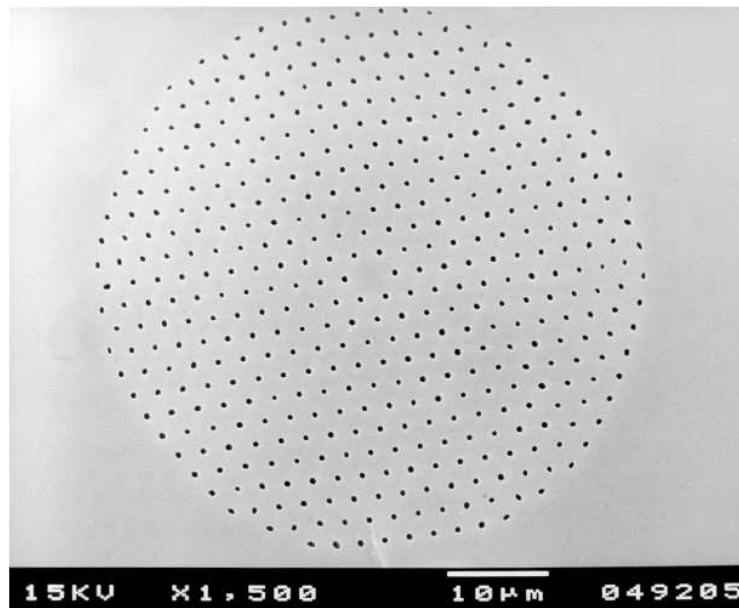
Figura 2.1: Micrografia da fibra PCF de 11 anéis de W. H. Reeves. et al. com perfil de dispersão ultra aplainado. \Lambda = 2.47\mu\text{m} e um d médio de 0.57\mu\text{m} .
