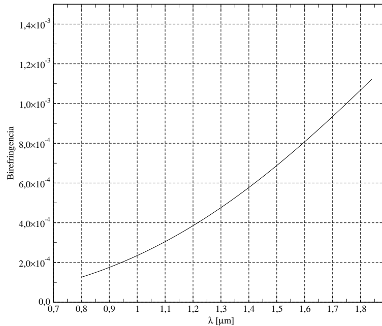
Figura 6.32: Birefringência calculada para a fibra PCF.
