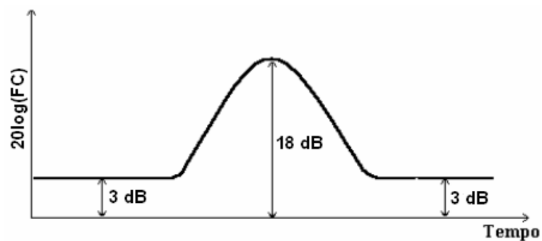
Figura 2.4. Comportamento do Fator de Crista no tempo
