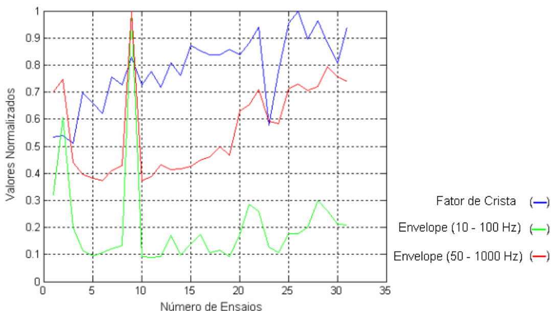
Figura 6.25. Curvas dos valores normalizados dos Parâmetros indicados de 4, 5 e 6.
