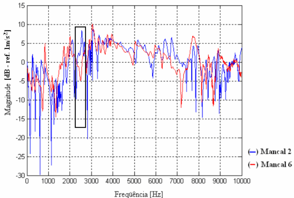
Figura 5.16. Magnitudes das FRF(s) dos mancais 2 e 6
