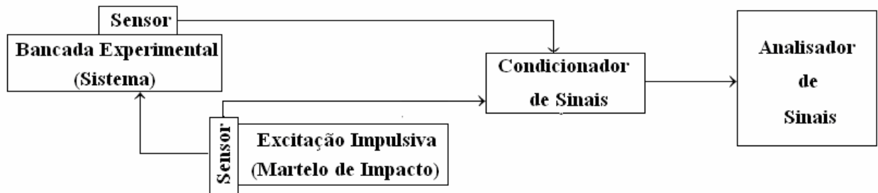
Figura 5.15. Cadeia de Instrumentação para determinação das FRF(s) do sistema
