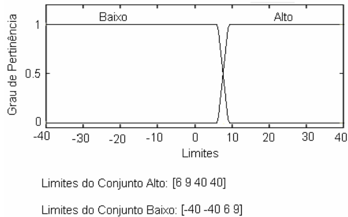
Figura 6.13. Funções de pertinência trapezoidais para o parâmetro de entrada RMS_1 , para o mancal 6
