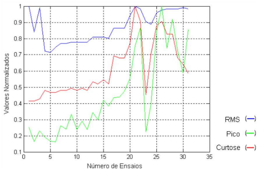
Figura 6.24. Curvas dos valores normalizados dos Parâmetros indicados de 1, 2 e 3.
