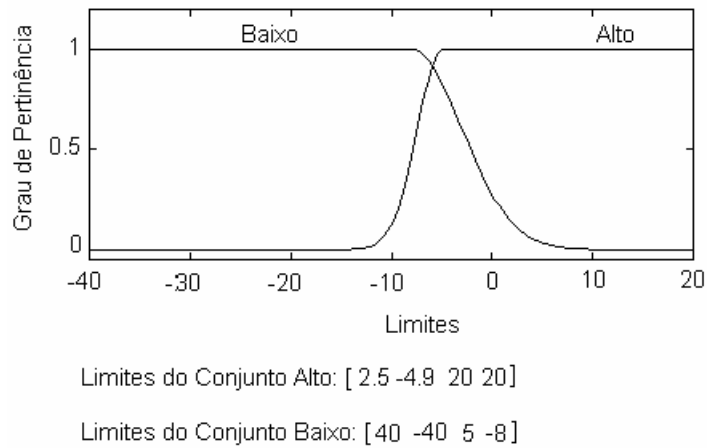
Figura 6.7. Funções de pertinência gaussianas de dois lados para o parâmetro de entrada RMS 18 , para o mancal 2
