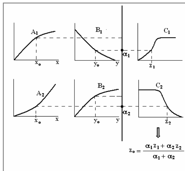
Figura 4.14. Modelo de raciocínio de Tsukamoto
