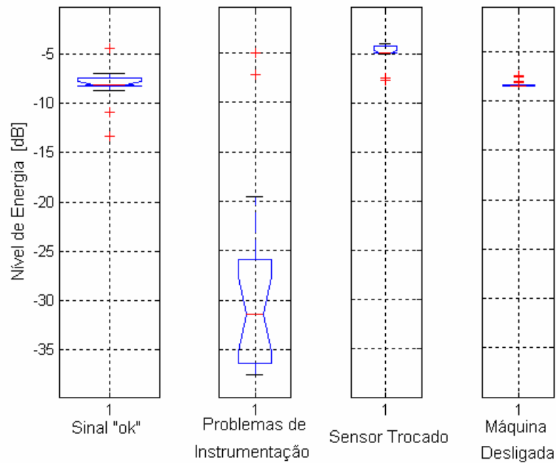
Figura 6.15. Gráficos “Boxplot” do RMS_{18} para as quatro categorias de sinal, do mancal 6
