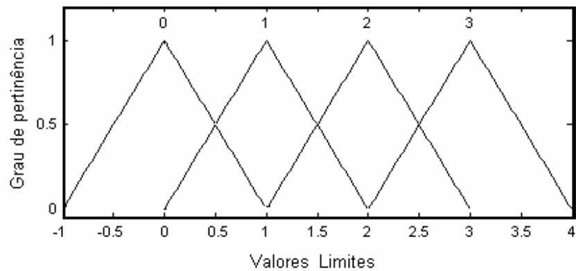
Figura 5.22. Funções de pertinência triangulares para as saídas do sistema de inferência
