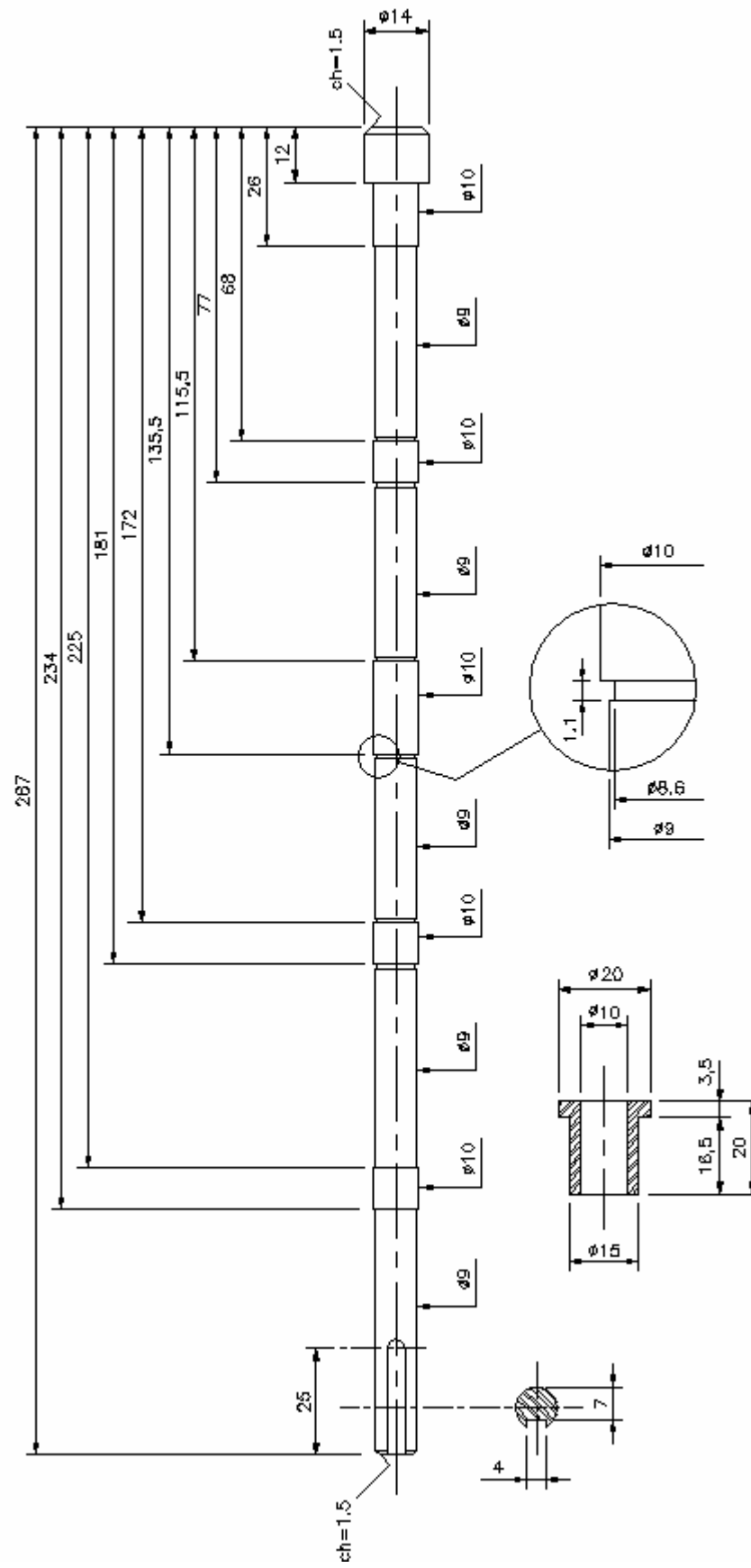
Figura 5.3. Dimensões do Eixo
