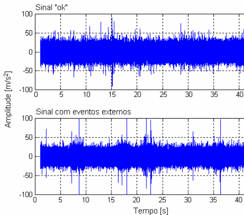
Figura 6.1. Amplitudes de aceleração no tempo, de um sinal considerado “ok” e de um sinal com eventos aleatórios aplicados à bancada experimental.
