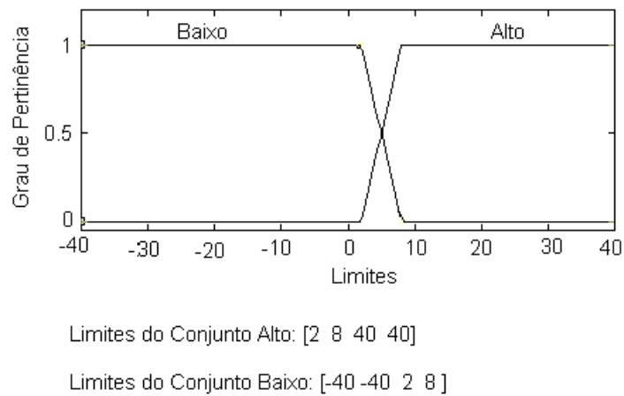
Figura 6.3. Funções de pertinência trapezoidais para o parâmetro de entrada RMS_1 , para o mancal 2
