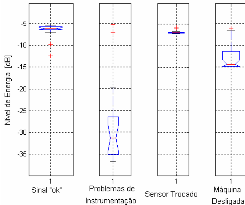
Figura 6.18. Gráficos “Boxplot” do RMS_{19} para as quatro categorias de sinal, do mancal 6
