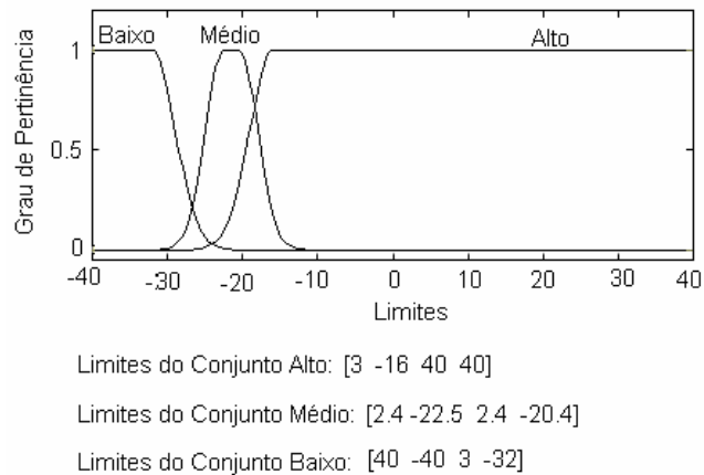
Figura 6.11. Funções de pertinência gaussianas de dois lados para o parâmetro de entrada RMS_{21} , para o mancal 2
