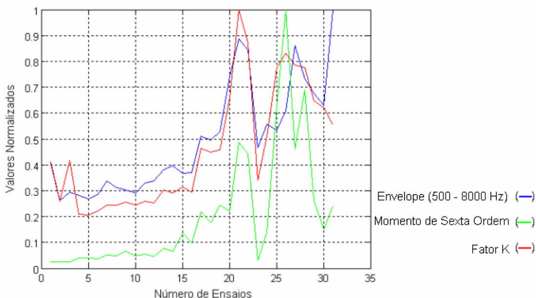
Figura 6.26. Curvas dos valores normalizados dos Parâmetros iniciados de 7, 8 e 9.
