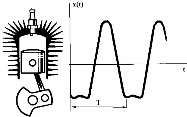
Figura 2.6. Curva de aceleração de um pistão de motor de combustão interna.
