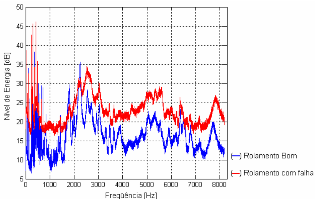
Figura 6.23. Espectros dos sinais para o rolamento bom e após a falha
