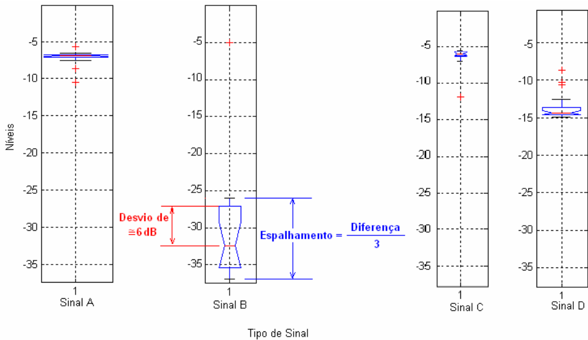
Figura 5.25. Exemplo de Gráficos “Boxplot” para determinação dos limites da função gaussiana.
