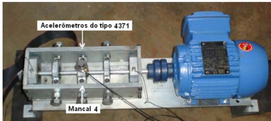
Figura 5.11. Acelerômetro tipo 4371, fixado no mancal 4
