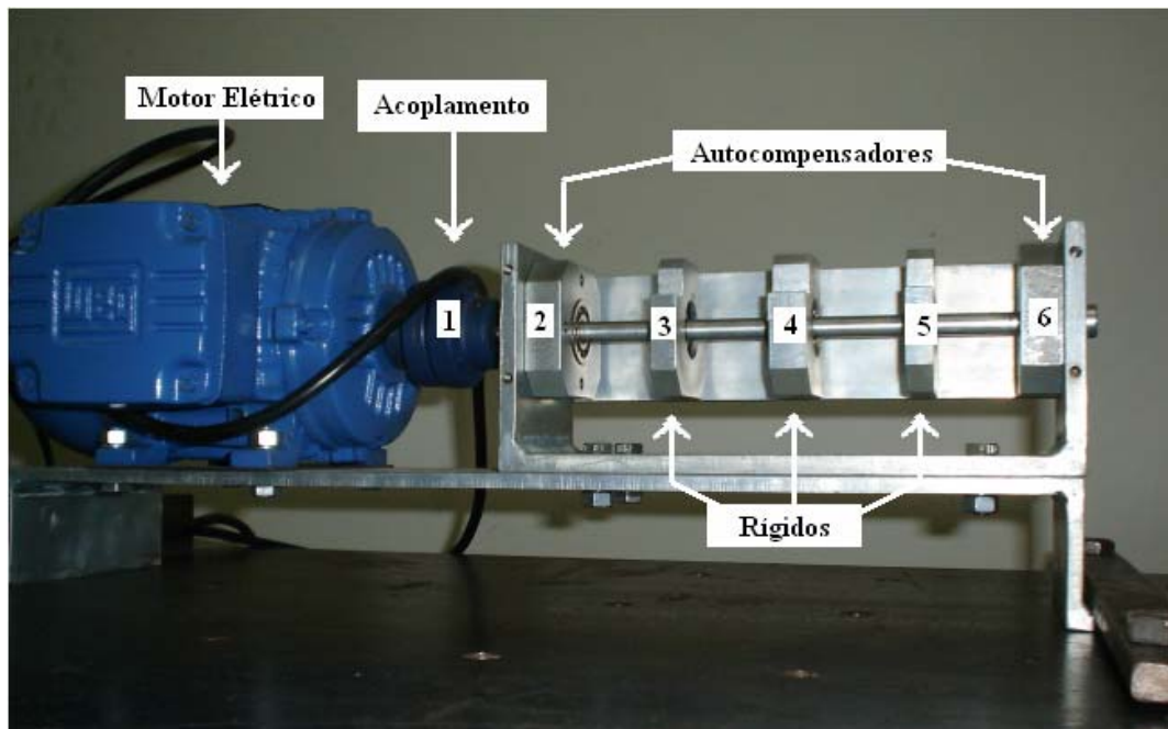
Figura 5.2. Bancada Experimental.
