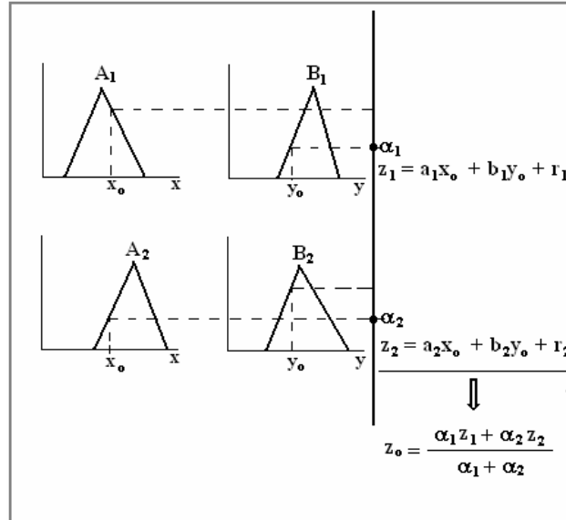
Figura 4.13. Modelo de raciocínio de Sugeno
