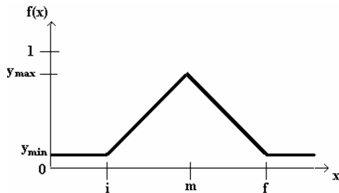
Figura 4.1. Função de Pertinência Triangular
