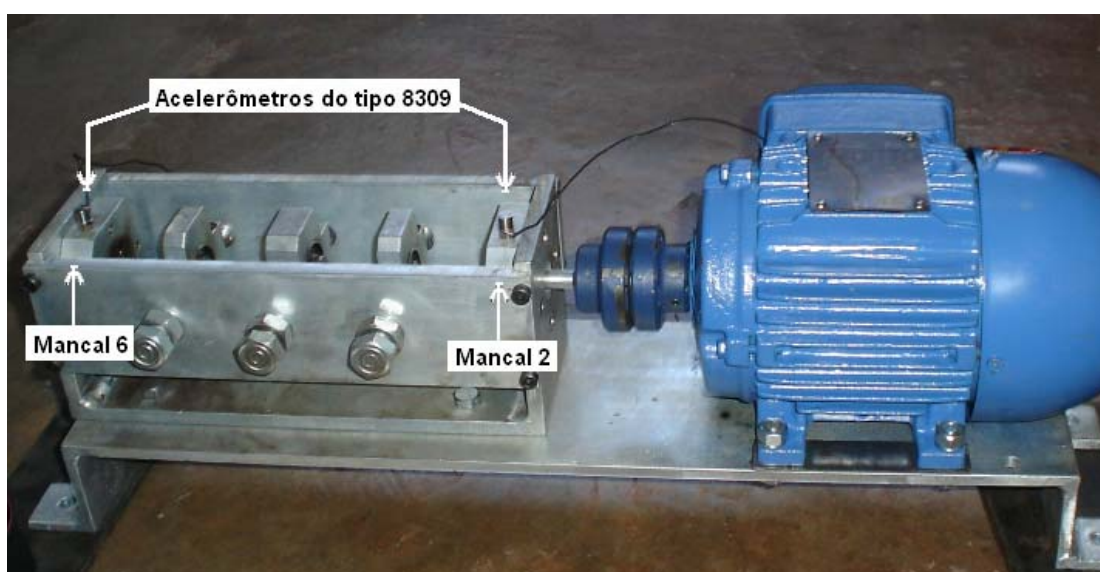
Figura 5.9. Acelerômetros tipo 8309, fixados nos mancais 2 e 6.
