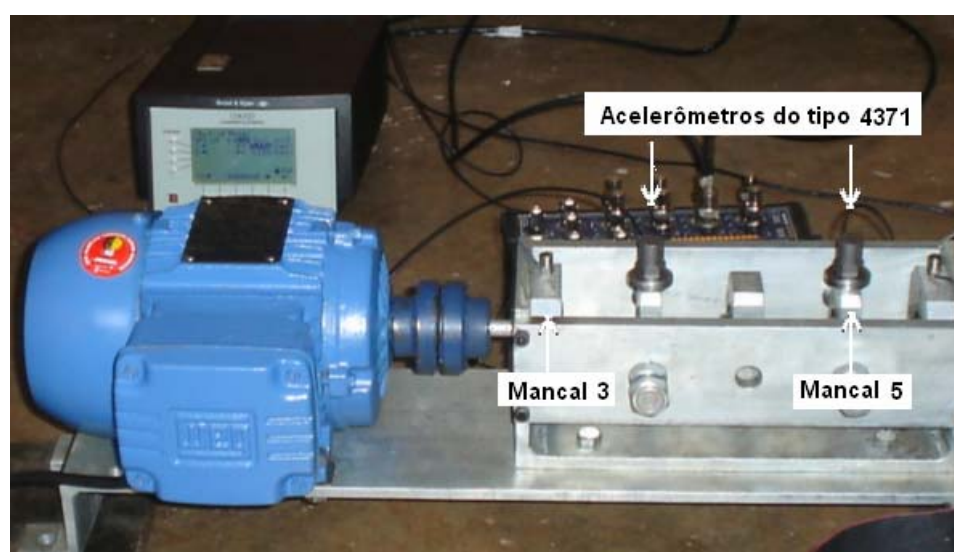
Figura 5.10. Acelerômetros tipo 4371, fixados nos mancais 3 e 5.
