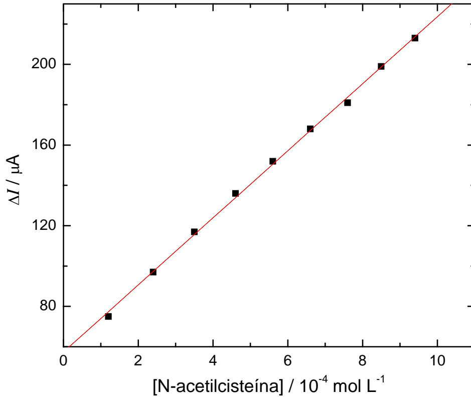
FIGURA 4.34. Curva analítica obtida para N-acetilcisteína empregando-se um EPCM com hexacianoferrato (III) de cobre (II) em solução tampão acetato 0,2 \text{ mol L}^{-1} (pH 6,0), a 25 \text{ }^\circ\text{C} .
