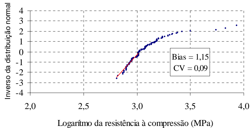
Figura 3.11 – Papel de probabilidade lognormal - f_{ck} = 18 MPa .
