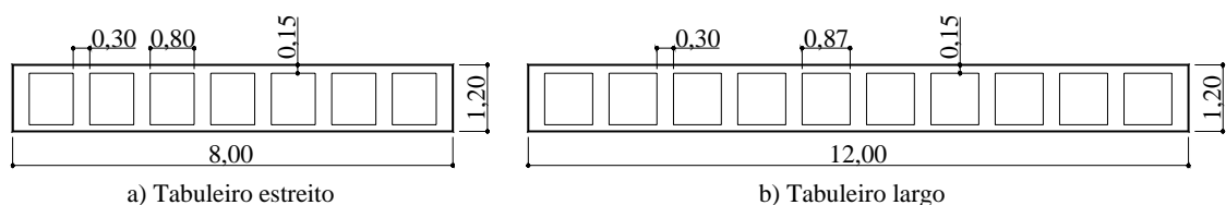
Figura 3.3 – Dimensões das lajes para dimensionamento.
