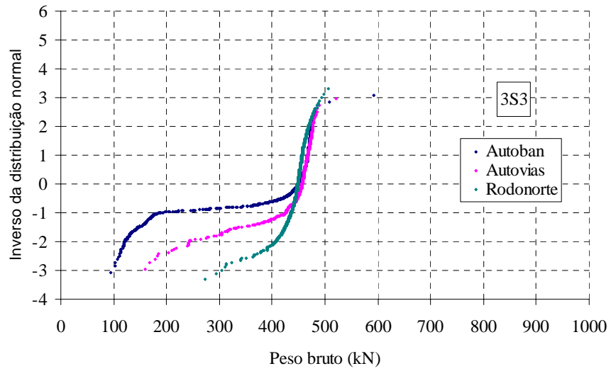
Figura A5 – Distribuições de pesos brutos – caminhão 3S3.
