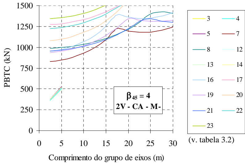
Figura 6.7 – PBTC - VIGA T – 2 VIGAS - Momento fletor negativo.
