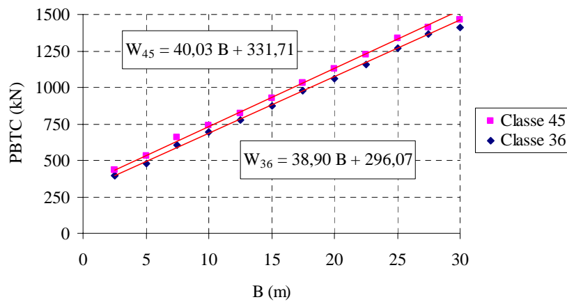
Figura D2 – ECPLs para o estado limite último – veículo isolado.
