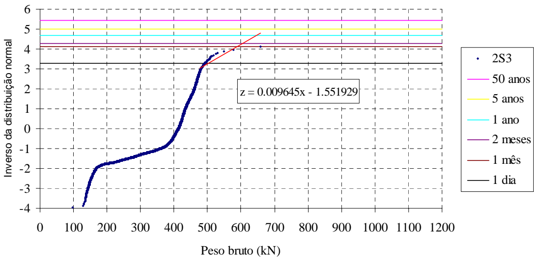
Figura 4.19 – Extrapolação para o caminhão 2S3 longo.
