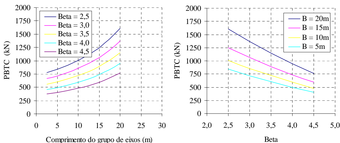
Figura 6.3 – PBTC para a ponte de 2 vigas SA TE V10 TR2 (concreto armado, classe 45).
