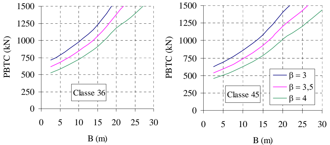
Figura 6.24 – Limites inferiores das curvas W x B – VIGA T – 5 VIGAS (com transversinas).
