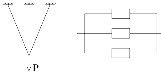
Figura 2.9 – Exemplo de um sistema em paralelo.
