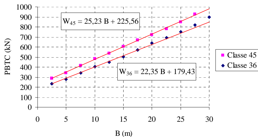
Figura C3 – ECPLs para o estado limite último.
