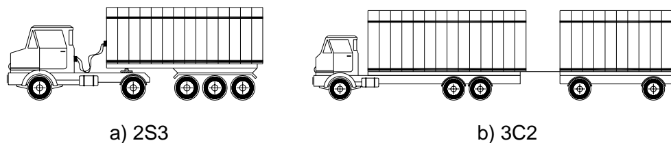
Figura 4.1 – Ilustração da nomenclatura dos caminhões.
