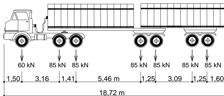
Figura 4.13 – Bitrem para 570 kN.
