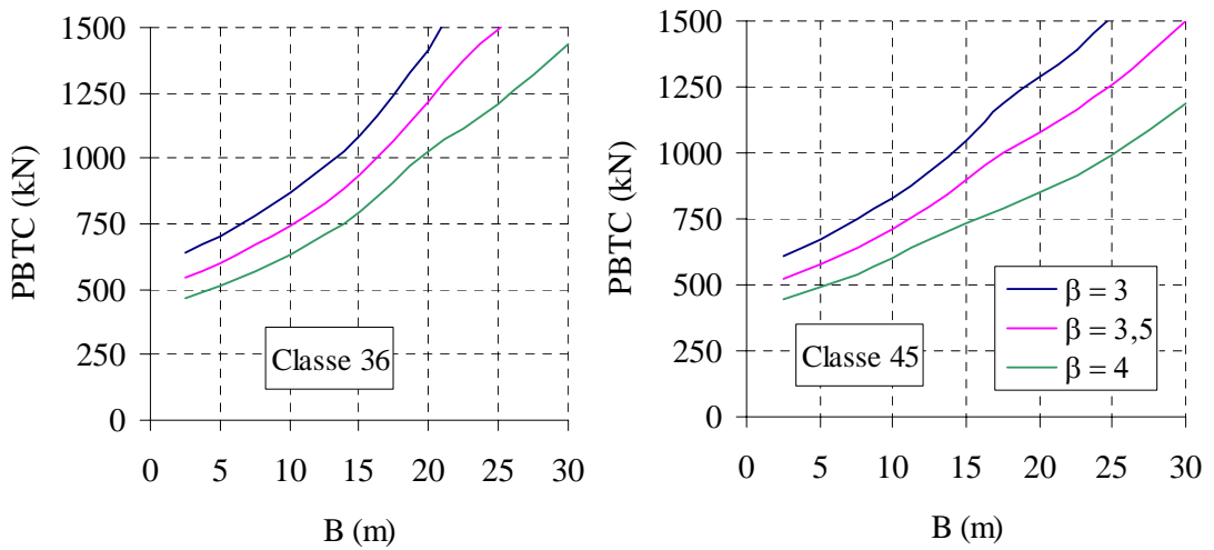
Figura 6.25 – Limites inferiores das curvas W x B – VIGA T – 5 VIGAS (sem transversinas).
