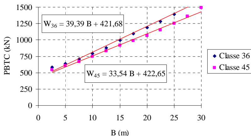
Figura D4 – ECPLs para o estado limite de serviço – veículo isolado.
