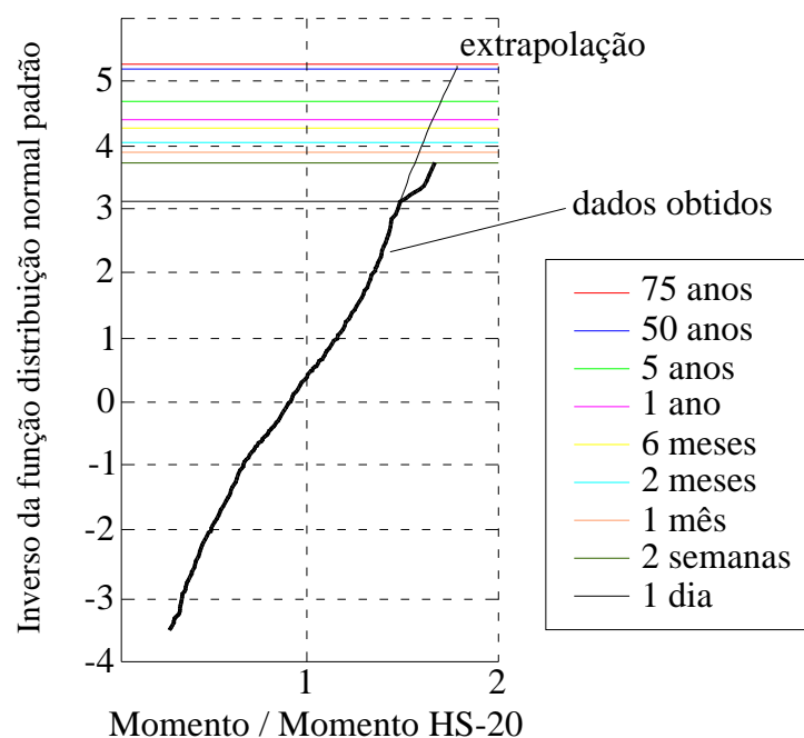
Figura 2.14 – Extrapolação para momento fletor negativo para vão de 9 metros. (NOWAK, 1999)
