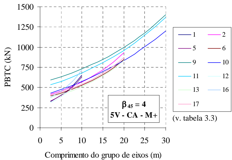
Figura 6.8 – PBTC - VIGA T – 5 VIGAS - Momento fletor positivo.
