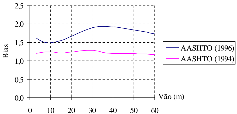
Figura 2.19 – Bias para força cortante, 75 anos de vida útil. (NOWAK, 1999)
