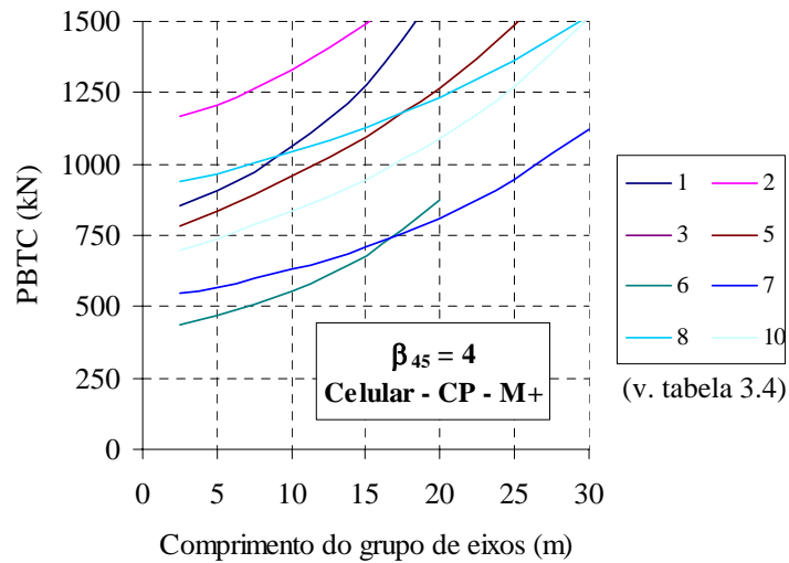
Figura 6.14 – PBTC – SEÇÃO CELULAR – ELU - Concreto protendido.
