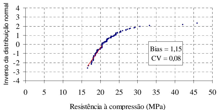
Figura 3.10 – Papel de probabilidade normal - f_{ck} = 18 MPa .
