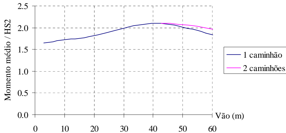
Figura 2.16 – Média dos máximos momentos fletores em 75 anos devido a um ou dois caminhões em uma faixa de tráfego. (NOWAK, 1999)
