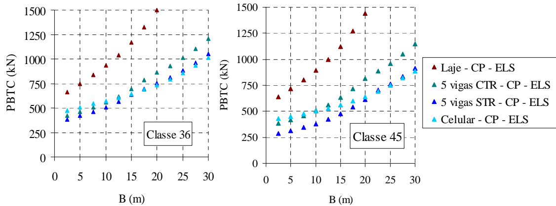
Figura C4 – Casos críticos para o estado limite de serviço.
