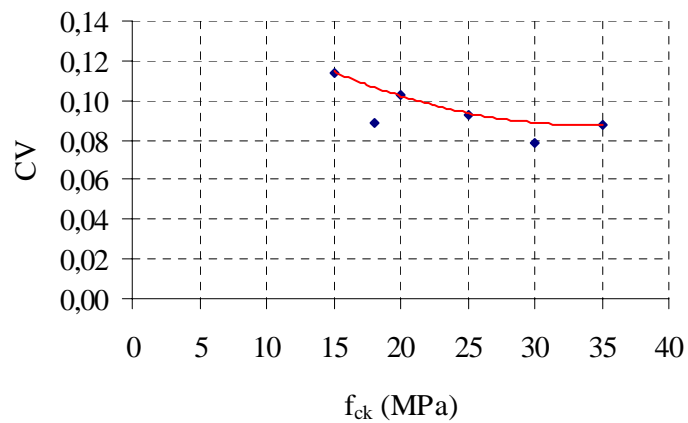
Figura 3.20 – Coeficiente de variação recomendado para a resistência à compressão do concreto.
