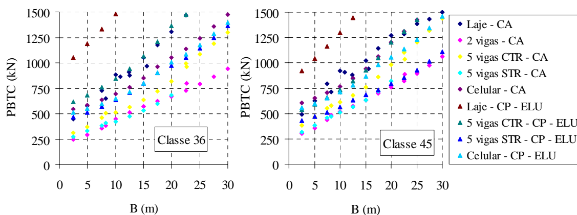
Figura C2 – Casos críticos para o estado limite último
