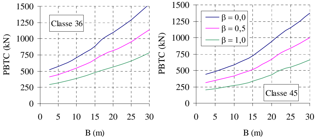
Figura 6.29 – Limites inferiores das curvas W x B – VIGA T – 5 VIGAS (sem transversinas).
