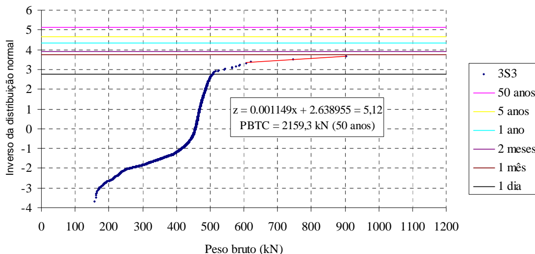
Figura 4.16 – Extrapolação segundo Nowak (1999) para o caminhão 3S3.
