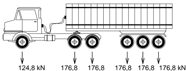
Figura 4.24 – Caminhão 3S3 curto.
