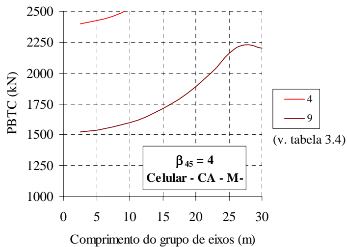
Figura 6.11 – PBTC - SEÇÃO CELULAR - Momento fletor negativo.
