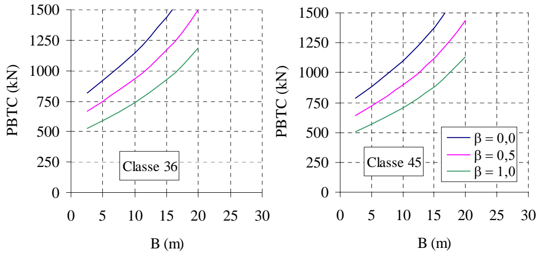
Figura 6.27 – Limites inferiores das curvas W x B – LAJE.
