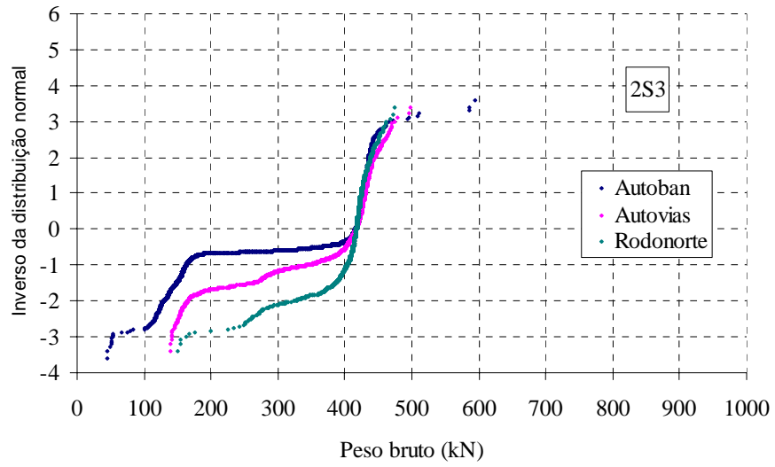
Figura A4 – Distribuições de pesos brutos – caminhão 2S3.
