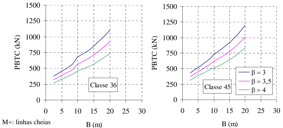
Figura 6.21 – Limites inferiores das curvas W x B – VIGA T – 5 VIGAS (sem transversinas).
