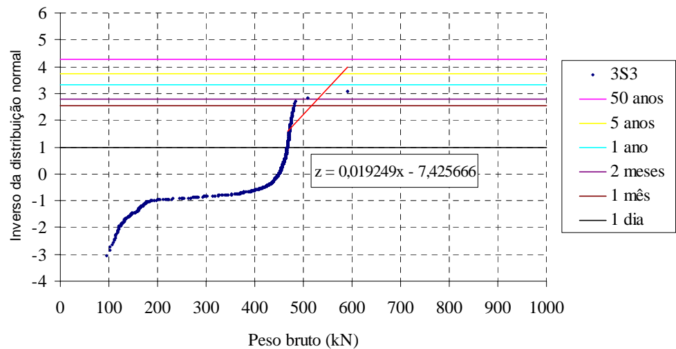
Figura A9 – Extrapolação de pesos brutos – 3S3.
