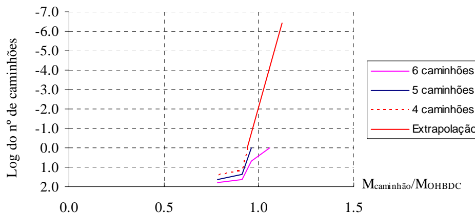
Figura 2.13 – Extrapolação para vida útil de 50 anos. (NOWAK e ZHOU, 1985)
