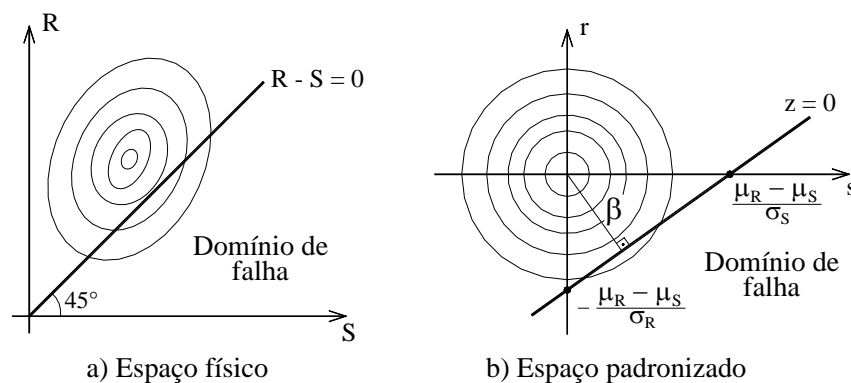
Figura 2.3 – Definição do índice de confiabilidade.
