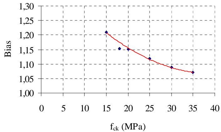
Figura 3.19 – Bias recomendada para a resistência à compressão do concreto.
