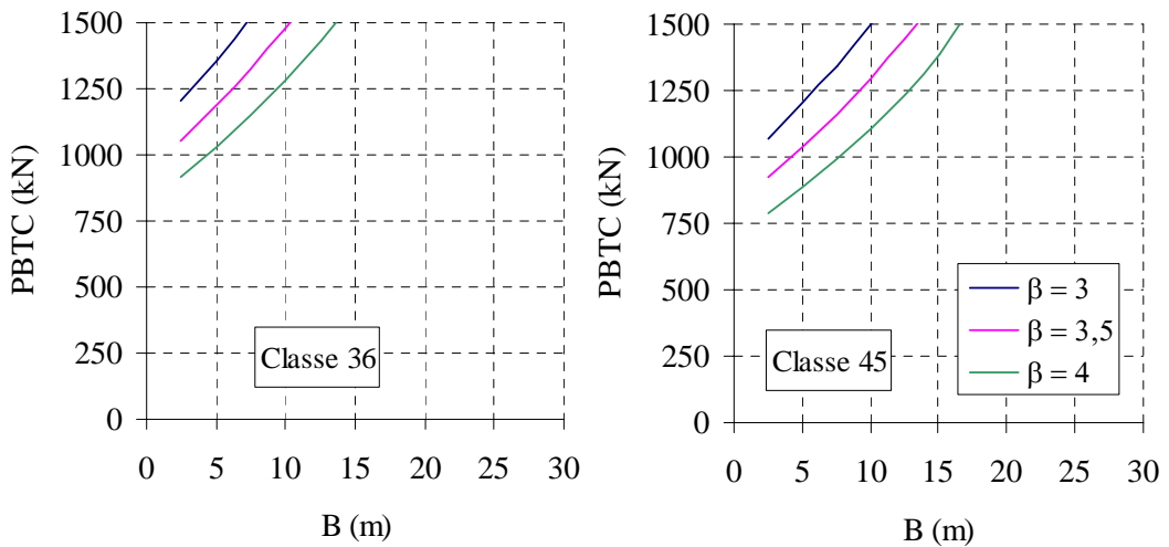
Figura 6.23 – Limites inferiores das curvas W x B – LAJE.
