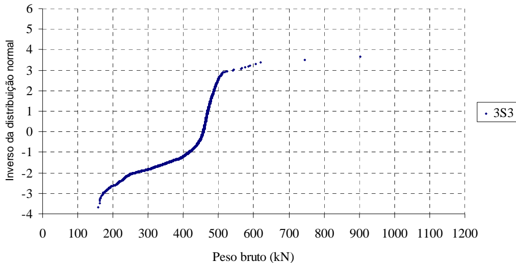
Figura 4.14 – Distribuição de peso bruto para o caminhão 3S3.
