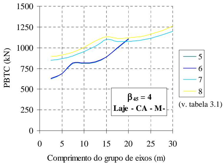
Figura 6.5 – PBTC – LAJE - Momento fletor negativo.
