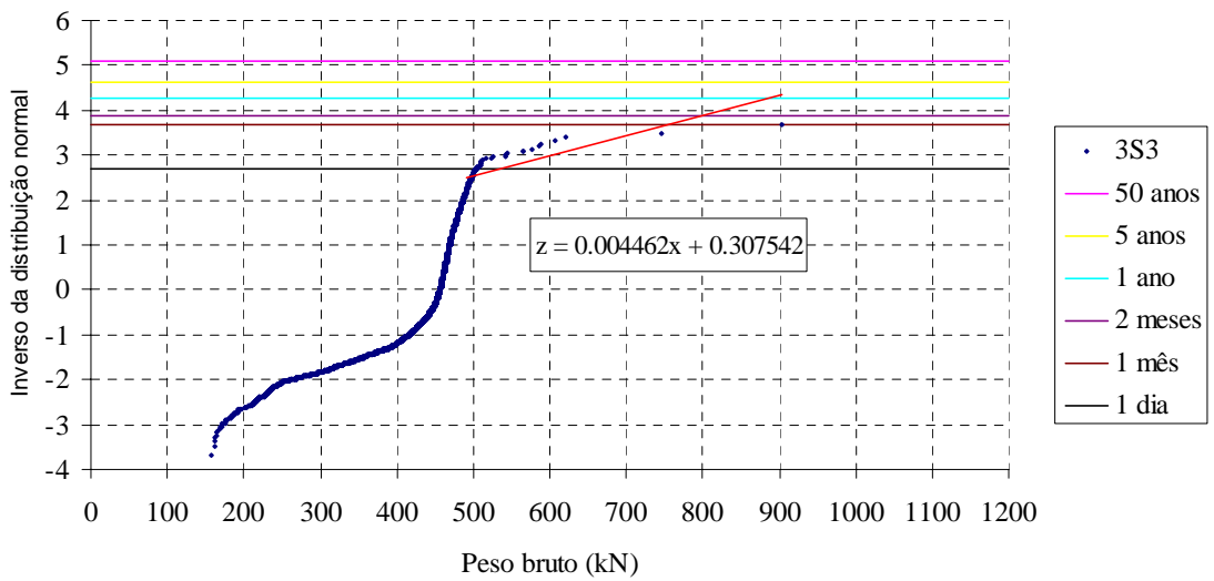
Figura 4.21– Extrapolação para o caminhão 3S3 longo.
