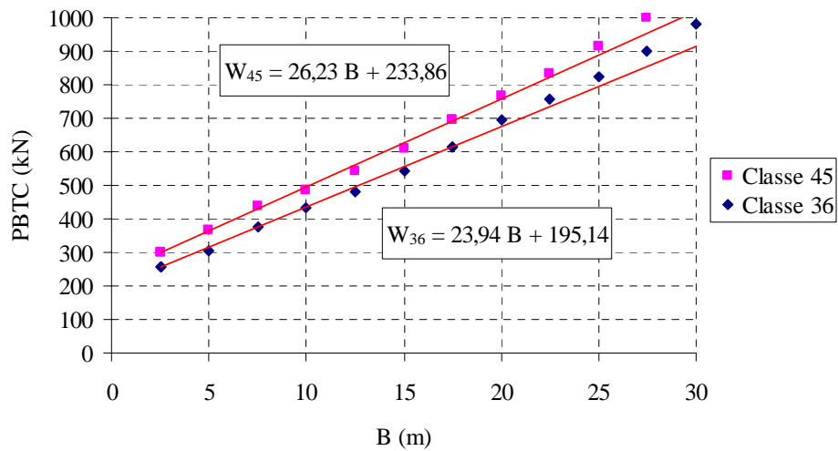
Figura 6.32 – ECPLs para o estado limite último.
