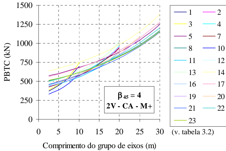
Figura 6.6 – PBTC - VIGA T – 2 VIGAS - Momento fletor positivo.
