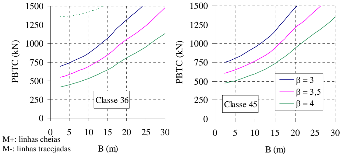
Figura 6.22 – Limites inferiores das curvas W x B – VIGA T – SEÇÃO CELULAR.
