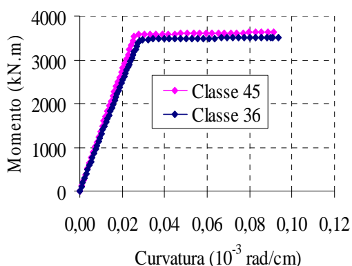
Figura 3.7 – Relação momento-curvatura para a ponte de 5 vigas, ordem 2 (SA TE V20 TR2).
