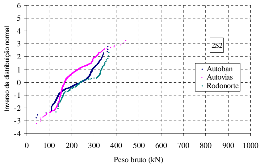
Figura A6 – Distribuições de pesos brutos – caminhão 2S2.
