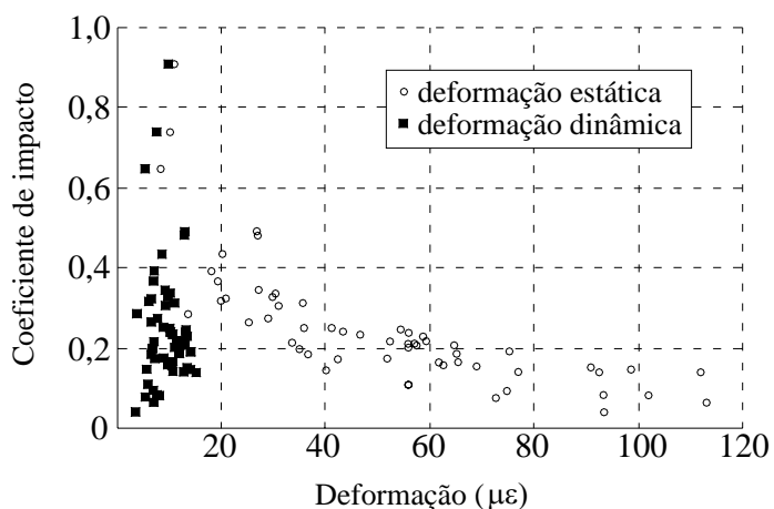
Figura 2.21 – Coeficiente de impacto em função das deformações. (NOWAK, 2004)
