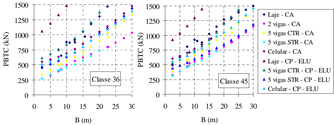
Figura 6.31 – Casos críticos para o estado limite último.
