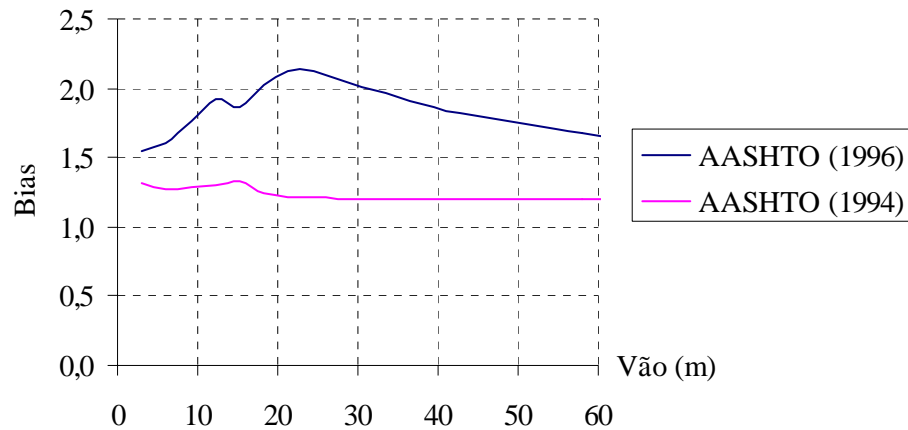
Figura 2.20 – BIAS para momento fletor negativo, 75 anos de vida útil. (NOWAK, 1999)
