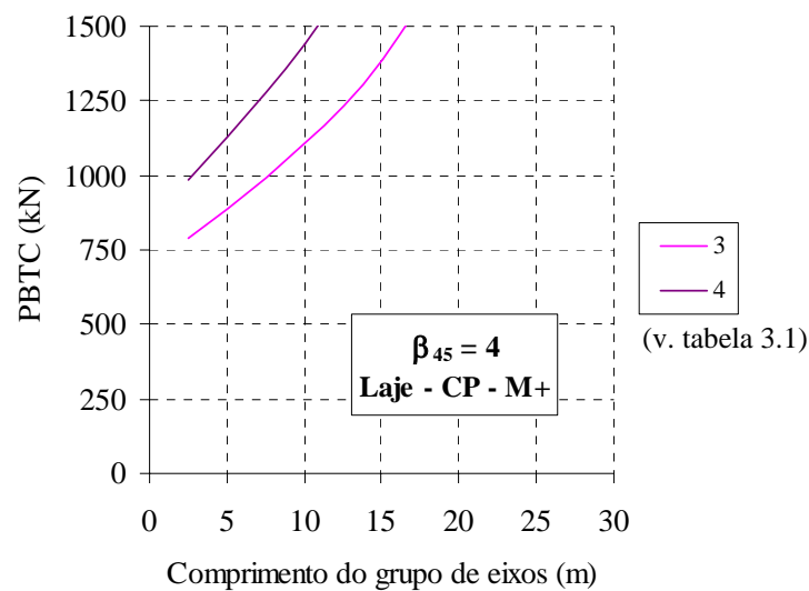
Figura 6.12 – PBTC - LAJE – ELU - Concreto protendido.
