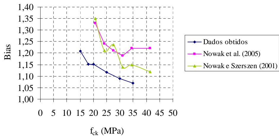
Figura 3.17 – Bias para a resistência à compressão do concreto.
