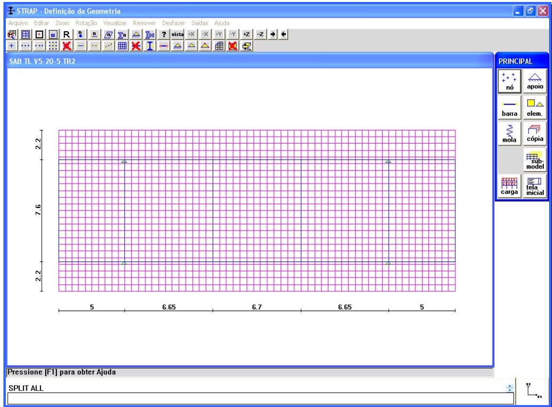
Figura 3.1 – Discretização do tabuleiro de uma ponte.
