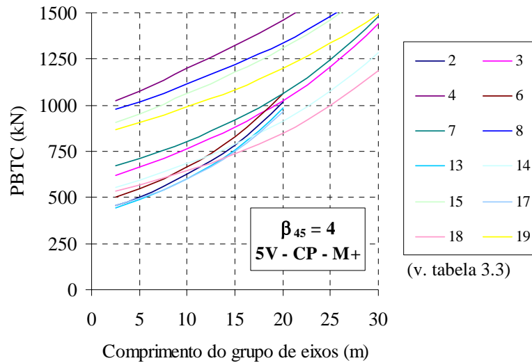
Figura 6.13 – PBTC – VIGA T – 5 VIGAS – ELU - Concreto protendido.
