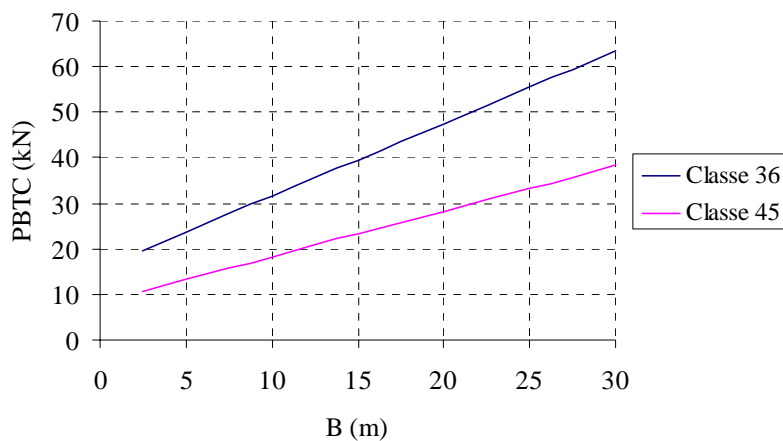
Figura C6 – Redução no PBTC devido à inclusão de um terceiro veículo - ELU.
