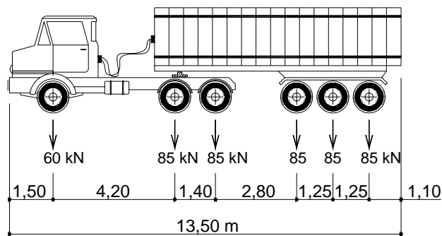
Figura 4.10 – Caminhão 3S3 curto para 450 kN.
