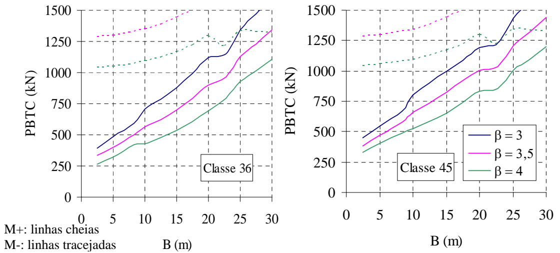
Figura 6.20 – Limites inferiores das curvas W x B – VIGA T – 5 VIGAS (com transversinas).
