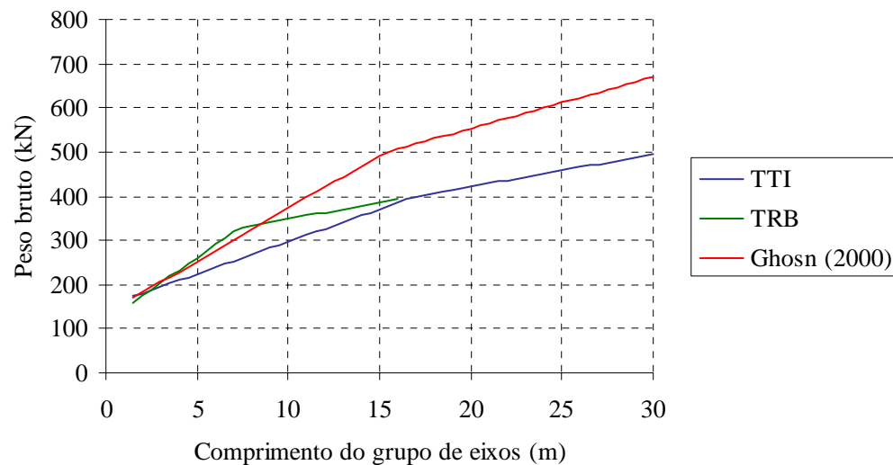
Figura 2.2 – Comparação entre a TTI formula , o TRB e a equação de Ghosn (2000).
