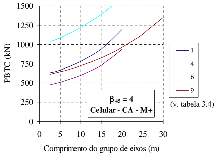
Figura 6.10 – PBTC - SEÇÃO CELULAR - Momento fletor positivo.
