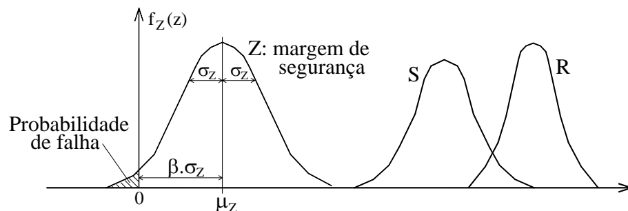
Figura 2.4 – Probabilidade de falha e margem de segurança.
