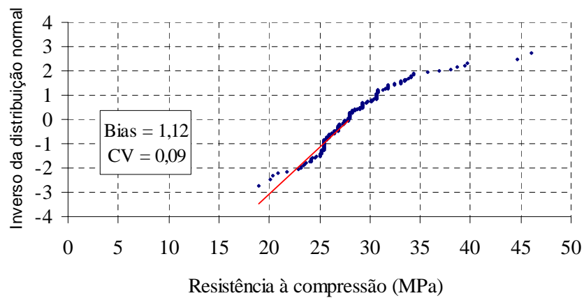
Figura 3.14 – Papel de probabilidade normal - f_{ck} = 25 MPa .
