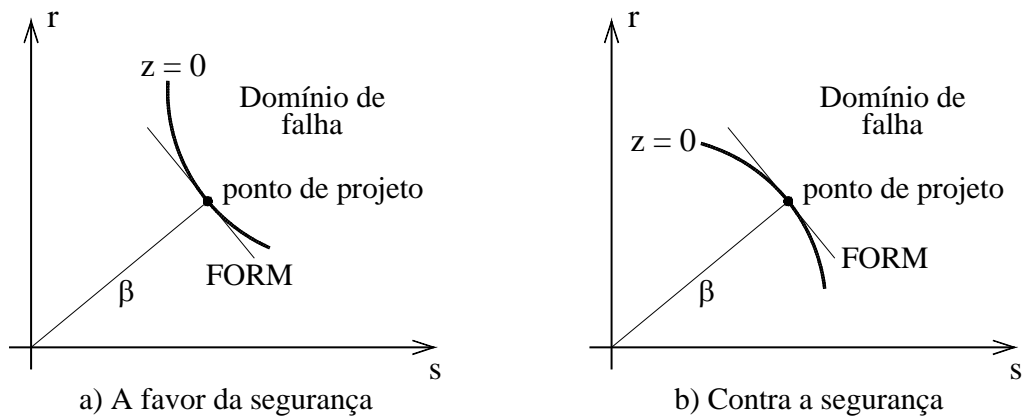
Figura 2.6 – Aproximação FORM para funções não-lineares de estado limite.
