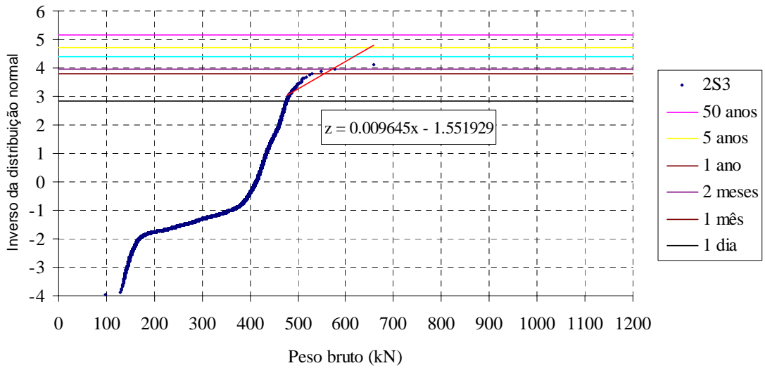
Figura 4.18 – Extrapolação para o caminhão 2S3 curto.
