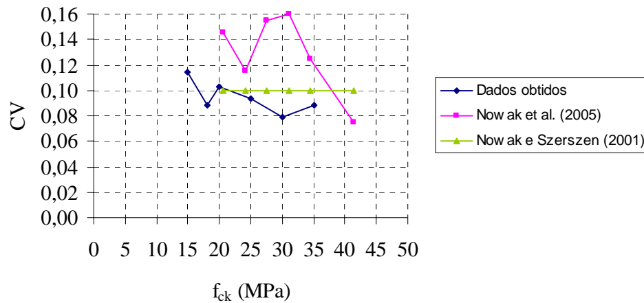
Figura 3.18 – Coeficiente de variação para a resistência à compressão do concreto.
