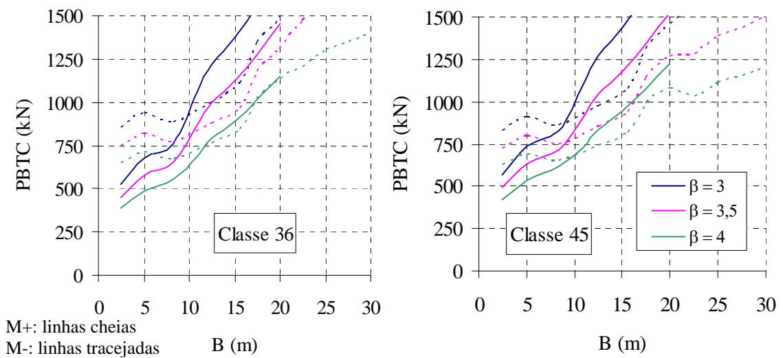
Figura 6.18 – Limites inferiores das curvas W x B – LAJE.
