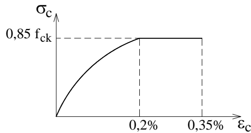
Figura 3.5 – Relação tensão x deformação do concreto à compressão.
