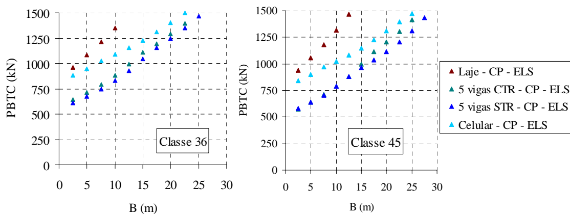
Figura D3 – Casos críticos para o estado limite de serviço – veículo isolado.
