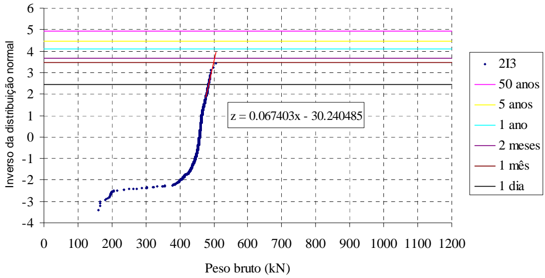
Figura 4.17 – Extrapolação para o caminhão 2I3.
