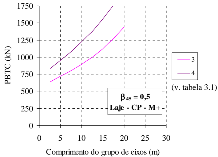
Figura 6.15 – PBTC – LAJE – ELS - Concreto protendido.
