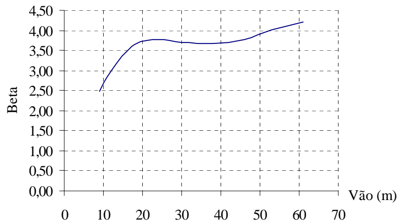
Figura 2.11 – Índices de confiabilidade obtidos a partir do método das tensões admissíveis da AASHTO (1996).
