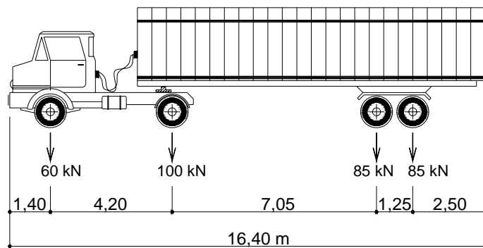
Figura 4.12 – Caminhão 2S2 para 330 kN.
