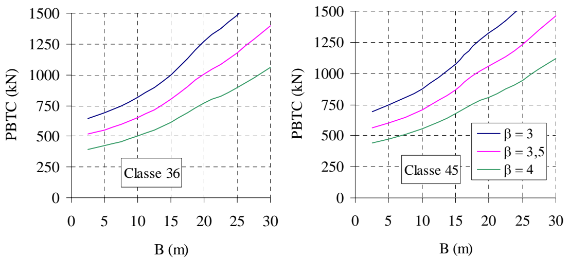
Figura 6.26 – Limites inferiores das curvas W x B – VIGA T – SEÇÃO CELULAR.
