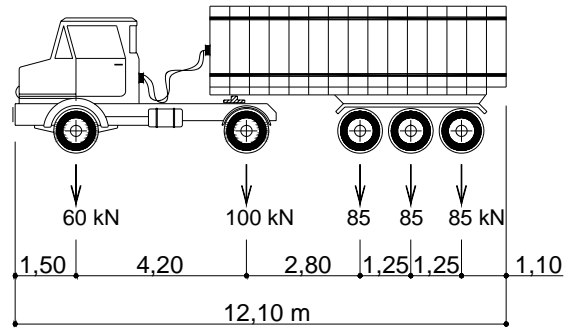
Figura 4.8 – Caminhão 2S3 curto para 415 kN.
