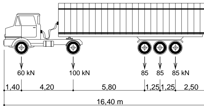
Figura 4.9 – Caminhão 2S3 longo para 415 kN.
