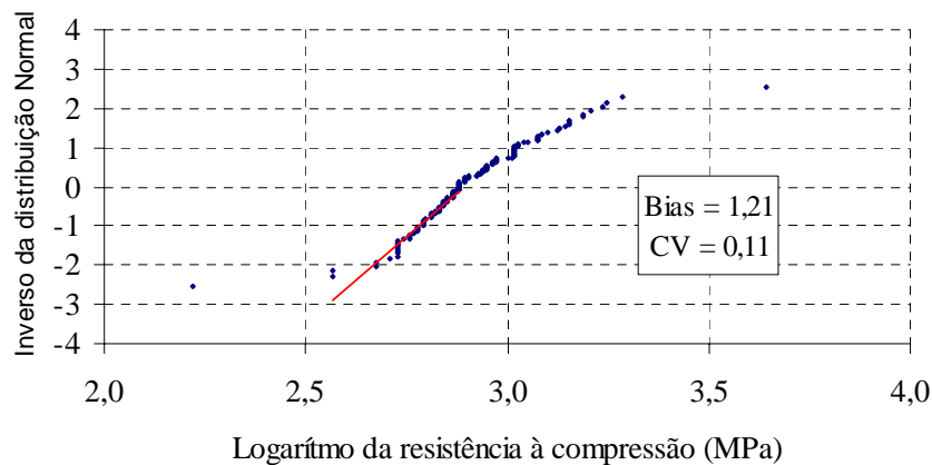
Figura 3.9 – Papel de probabilidade lognormal - f_{ck} = 15 MPa .
