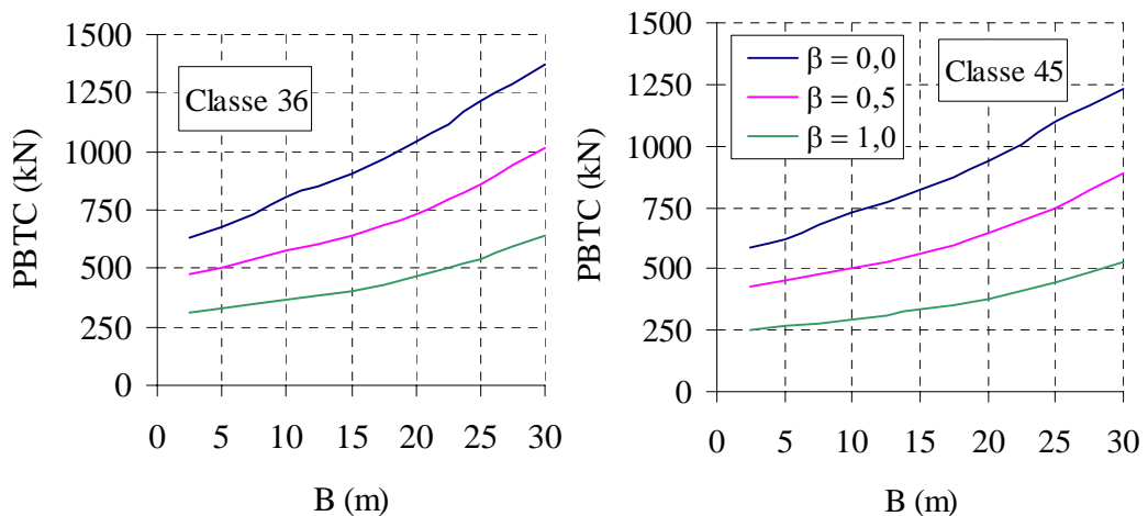
Figura 6.30 – Limites inferiores das curvas W x B – VIGA T – SEÇÃO CELULAR.
