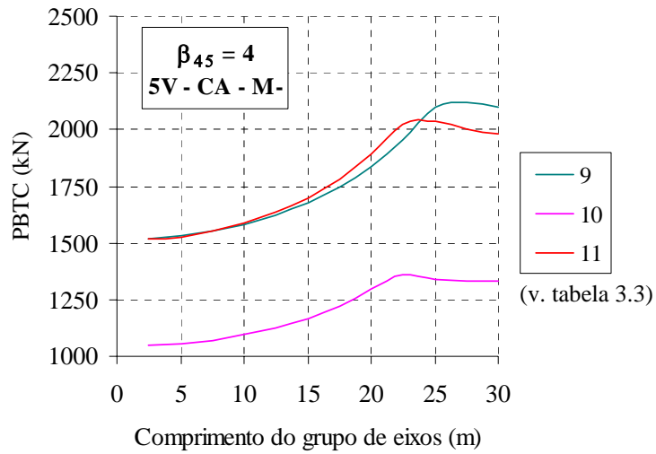
Figura 6.9 – PBTC - VIGA T – 5 VIGAS - Momento fletor negativo.
