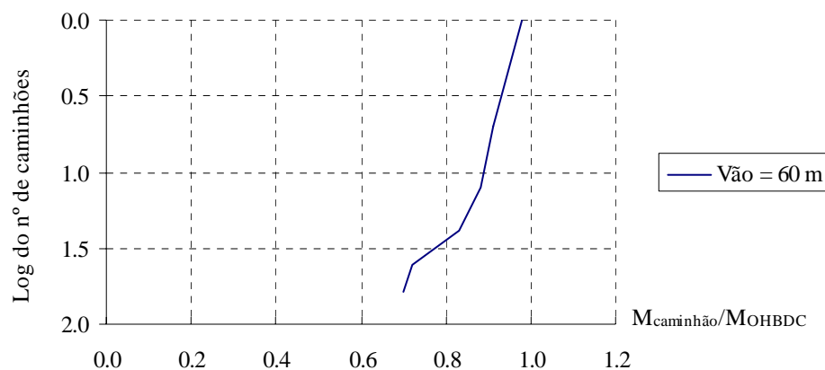
Figura 2.12 – Cauda superior da distribuição de momentos fletores. (NOWAK e ZHOU, 1985)
