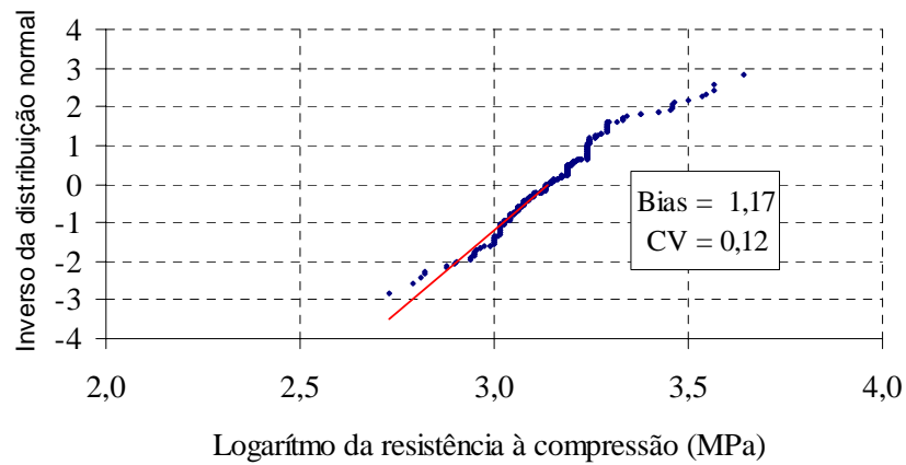
Figura 3.13 – Papel de probabilidade lognormal - f_{ck} = 20 MPa .
