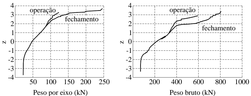
Figura 4.26 – Resultados do weigh-in-motion durante o fechamento e a operação de uma balança fixa. (NOWAK, 2004)
