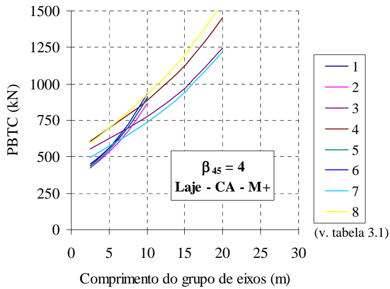
Figura 6.4 – PBTC – LAJE - Momento fletor positivo.
