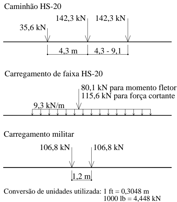
Figura 2.10 – Carregamento HS-20 da AASHTO (1996).
