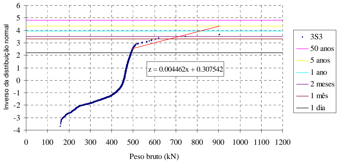
Figura 4.20 – Extrapolação para o caminhão 3S3 curto.
