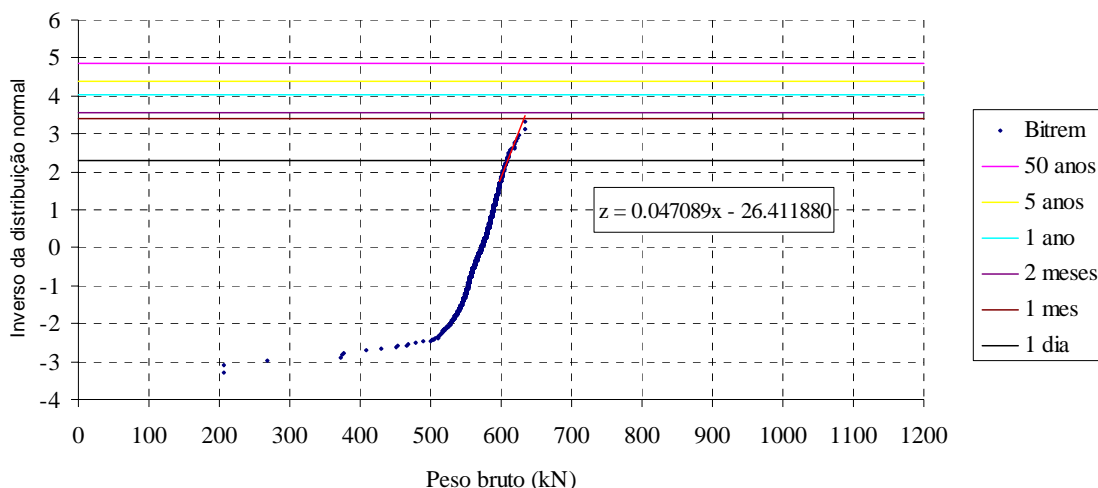
Figura 4.23 – Extrapolação para o bitrem.
