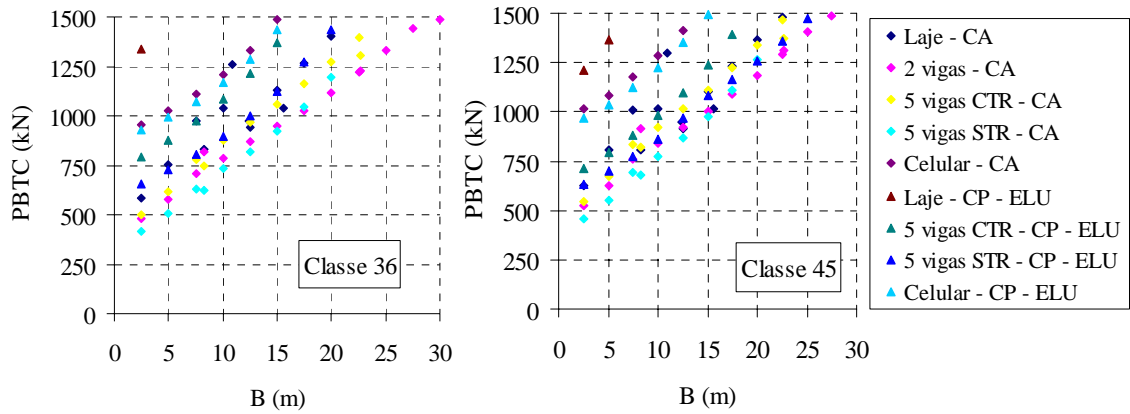
Figura D1 – Casos críticos para o estado limite último – veículo isolado.
