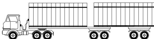
Figura 4.4 – Bitrem com comprimento de até 19,80m e PBTC de até 570 kN.
