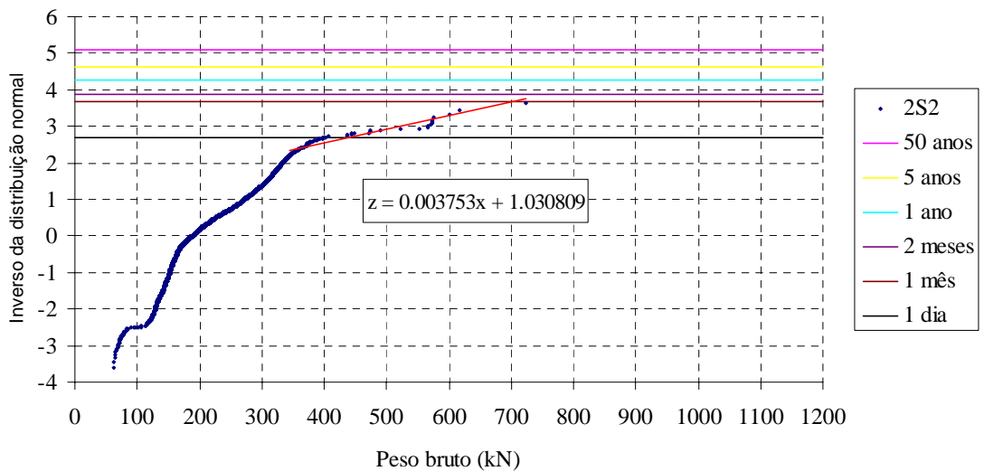
Figura 4.22 – Extrapolação para o caminhão 2S2.
