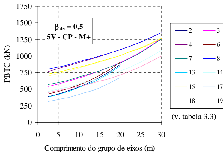
Figura 6.16 – PBTC – VIGA T – 5 VIGAS – ELS - Concreto protendido.
