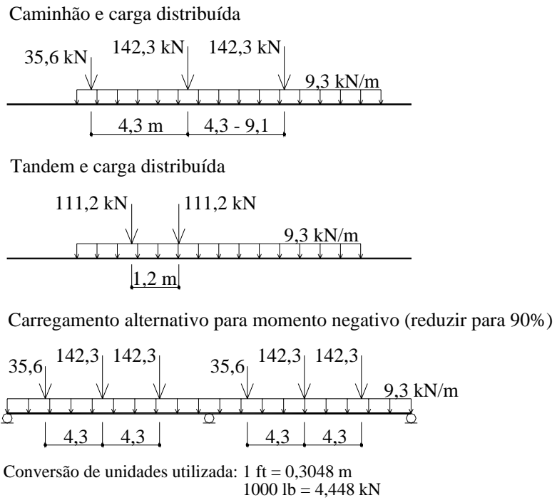
Figura 2.17 – Carga móvel de projeto na AASHTO LRFD. (NOWAK, 1999)
