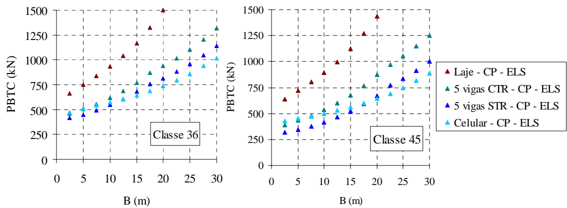
Figura 6.33 – Casos críticos para o estado limite de serviço.
