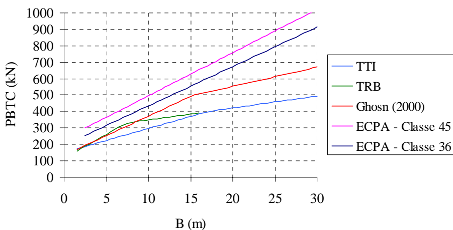
Figura 6.35 – Comparação entre equações para o ELU.
