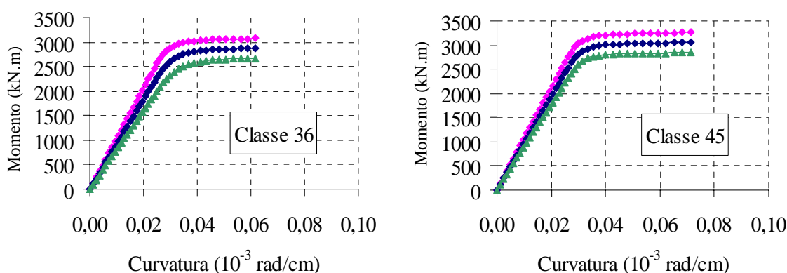
Figura 3.22 – Relações momento-curvatura para a ponte de 2 vigas, ordem 1 (SA TE V10 TR2).
