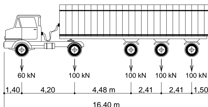
Figura 4.7 – Caminhão 213 para 450 kN.
