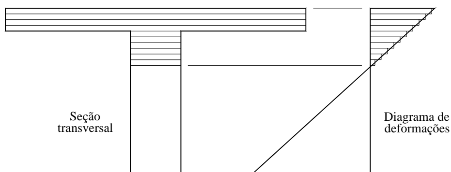
Figura 3.4 – Seção transversal dividida em fatias na zona comprimida.
