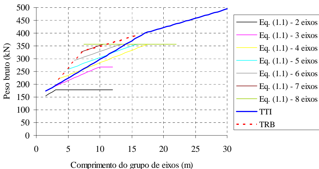
Figura 2.1 – Comparação entre a bridge formula oficial (para vários N ), a TTI formula e a equação do TRB.
