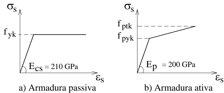
Figura 3.6 - Relações tensão x deformação das armaduras ativa e passiva.
