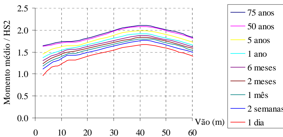
Figura 2.15 – Média dos máximos momentos fletores para vãos únicos devido a um caminhão isolado. (NOWAK, 1999)
