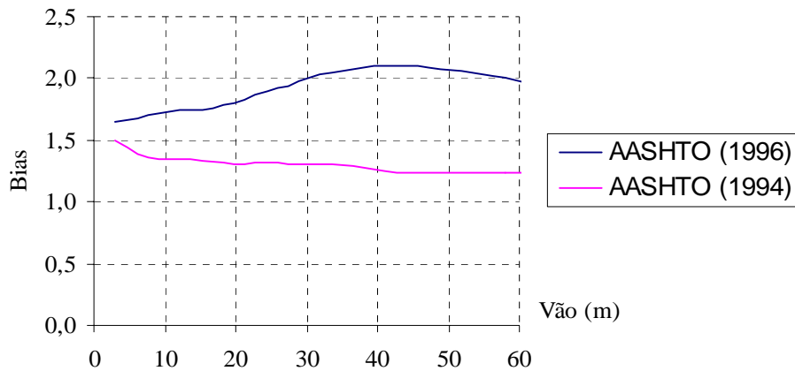
Figura 2.18 – Bias para momento fletor positivo, 75 anos de vida útil. (NOWAK, 1999)
