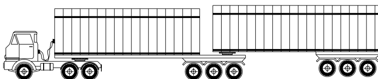
Figura 4.3 – Bitrenção com comprimento de até 30m e PBTC de até 740 kN.
