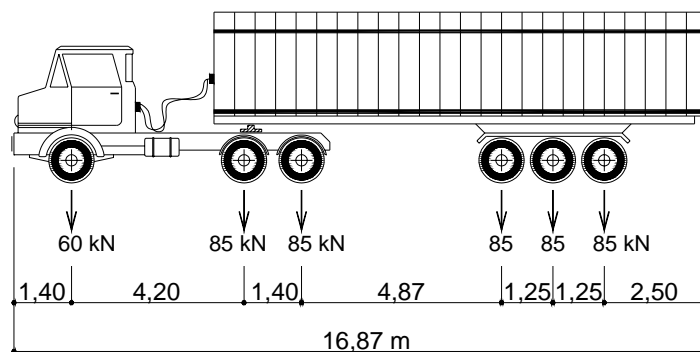
Figura 4.11 – Caminhão 3S3 longo para 450 kN.
