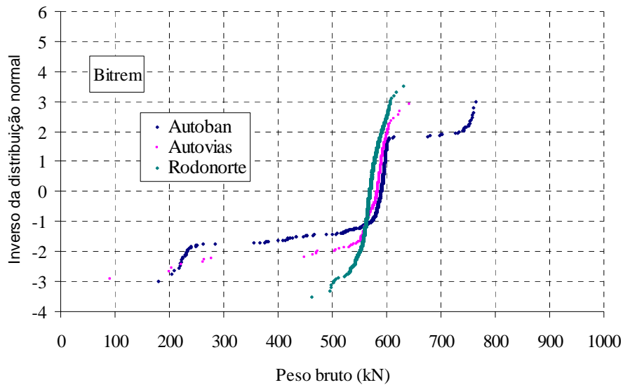
Figura A7 – Distribuições de pesos brutos – bitrem.
