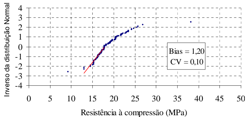
Figura 3.8 – Papel de probabilidade normal - f_{ck} = 15 MPa .
