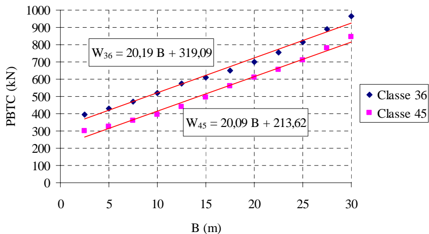
Figura 6.34 – ECPLs para o estado limite de serviço.
