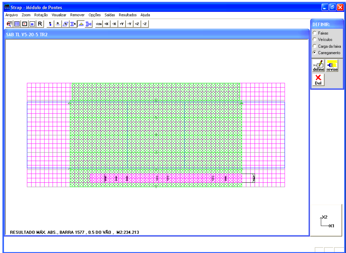
Figura 3.2 – Carregamento crítico para momento máximo na longarina.
