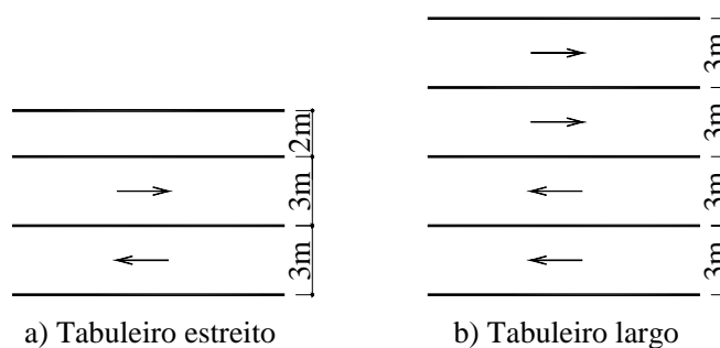
Figura 4.25 – Sentido do tráfego e disposição das faixas.
