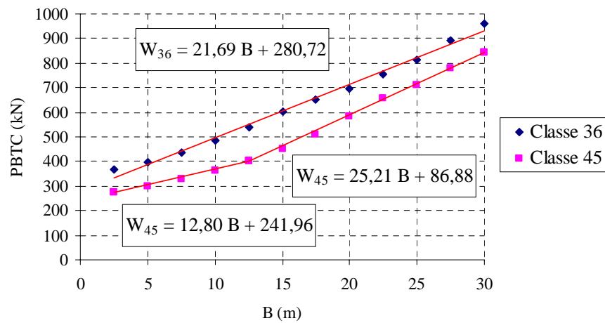
Figura C5 – ECPLs para o estado limite de serviço.
