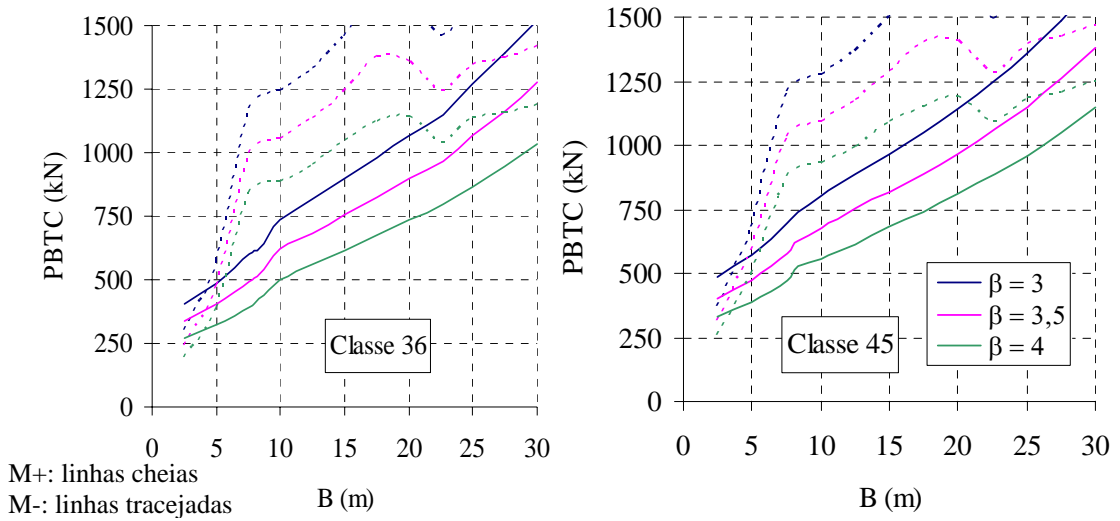
Figura 6.19 – Limites inferiores das curvas W x B – VIGA T – 2 VIGAS.
