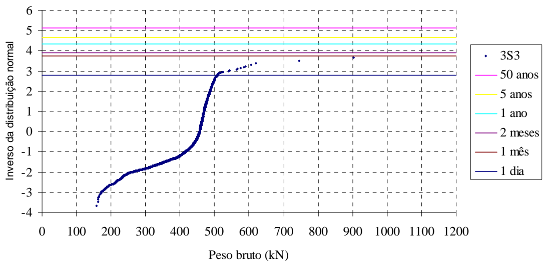
Figura 4.15 – Extrapolação para diversos períodos (3S3).
