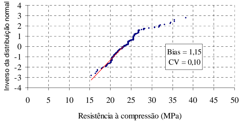
Figura 3.12 – Papel de probabilidade normal - f_{ck} = 20 MPa .
