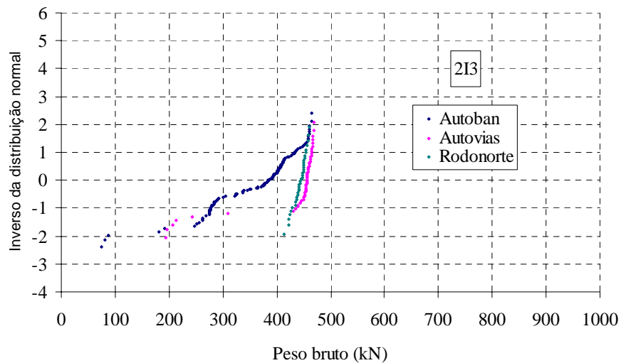
Figura A3 – Distribuições de pesos brutos – caminhão 2I3.
