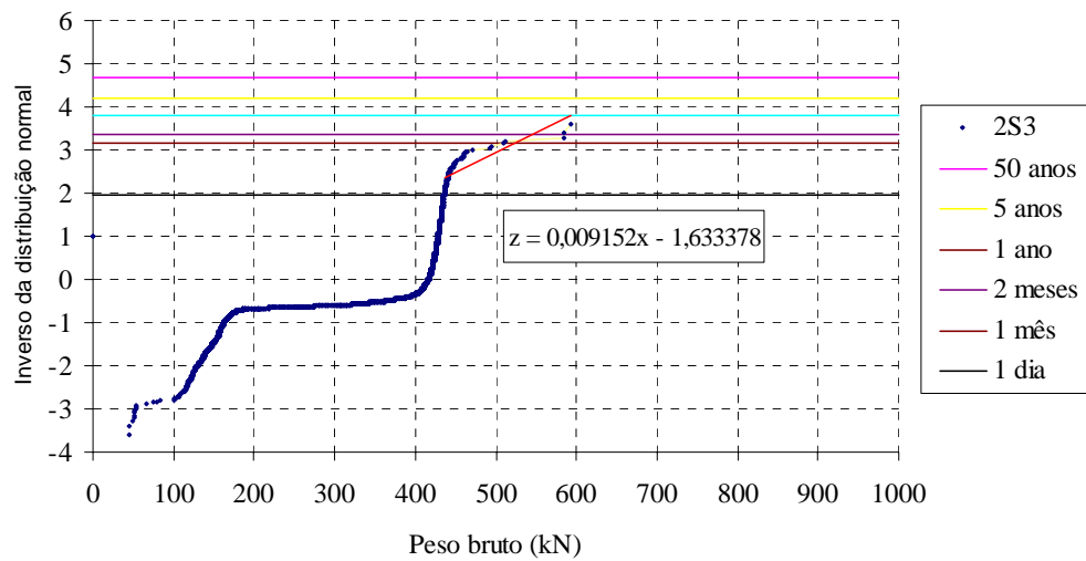
Figura A8 – Extrapolação de pesos brutos – 2S3.
