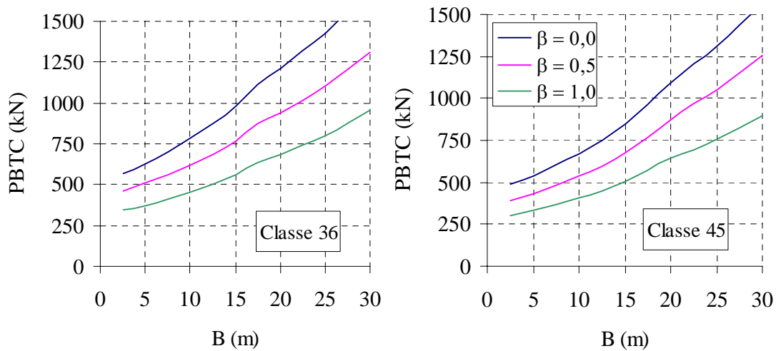
Figura 6.28 – Limites inferiores das curvas W x B – VIGA T – 5 VIGAS (com transversinas).
