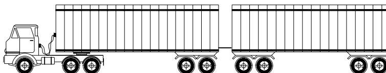
Figura 4.2 – Rodotrem com comprimento de até 30m e PBTC de até 740 kN.
