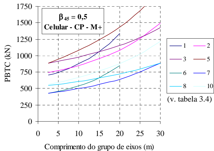
Figura 6.17 – PBTC – SEÇÃO CELULAR – ELS - Concreto protendido.
