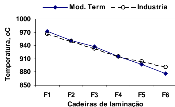
Fig.4.35 – Resultados da temperatura fornecida pela industria e a temperatura obtida pelo modelo termomicroestrutural.
