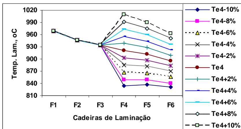
Figura G.24 – Resultados da temperatura de laminação, obtidos pelo modelo para aço carbono manganês 3, devido a variações provocadas na temperatura de entrada do material na cadeira F4, tabela D3.4.
