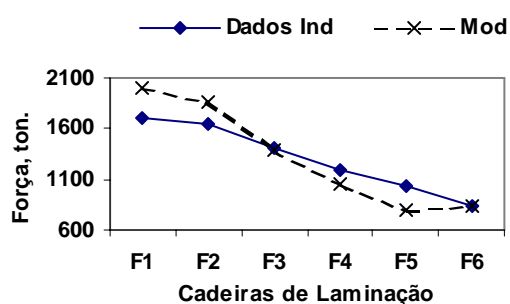
Fig.4.13 – Resultados de força de laminação fornecido pela industria e obtidos pelo modelo microestrutural com a correção para a equação de Misaka.
