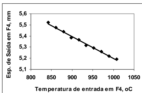
Figura G.20 – Resultados de espessura de saída (mm) obtidos pelo modelo termomicroestrutural para aço carbono manganês 3, devido a variações na temperatura de entrada do em F4, tabela D3.1.
