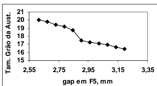
Figura H.8 – Resultados de tamanho de grão ( \mu\text{m} ) obtidos pelo modelo termomicroestrutural para aço carbono manganês 3, devido a variações provocadas no gap da cadeira F5, tabela E3.1.
