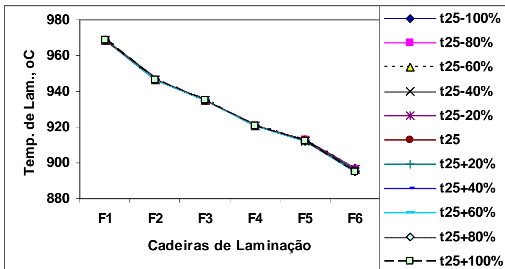
Figura H.38 – Resultados da temperatura de laminação, obtidos pelo modelo termomicroestrutural para aço carbono manganês 3, devido a variações provocadas tensão a frente na tira em F5, tabela E5.4
