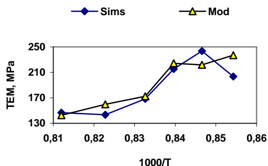
Fig.4.6 – Resultados da TEM obtidas pelo modelo de Sims e pelo modelo com a correção para a equação de Misaka.
