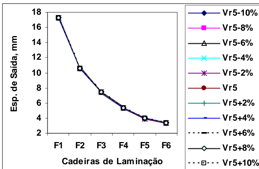
Figura H.49 – Resultados da espessura de saída do material, obtidos pelo modelo termomicroestrutural para aço carbono manganês 3, devido a variações provocadas na velocidade do cilindro em F5, tabela E6.5.
