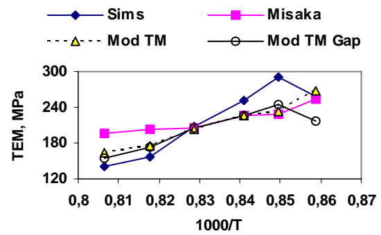
Fig.4.41 – Resultados da TEM obtidas pelo modelo de Sims e os obtidos pelo modelo termomicroestrutural utilizando h1 e h2 (Mod TM) e utilizando o gap (Mod TMGap).
