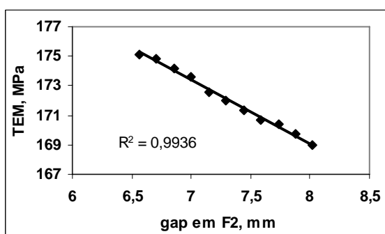
Figura 5.56 – Resultados das tensões de escoamento média(TEM), obtidos pelo modelo termomicroestrutural para aço carbono manganês 3, devido a variações provocadas no gap da cadeira F2, tabela B2.1.
