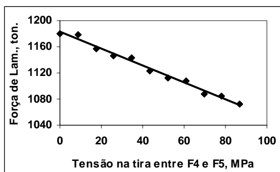
Figura G.36 – Resultados de carga de laminação (ton.) obtidas pelo modelo termomicroestrutural para aço carbono manganês 3, devido a variações na tensão a frente da tira em F4, tabela D5.1
