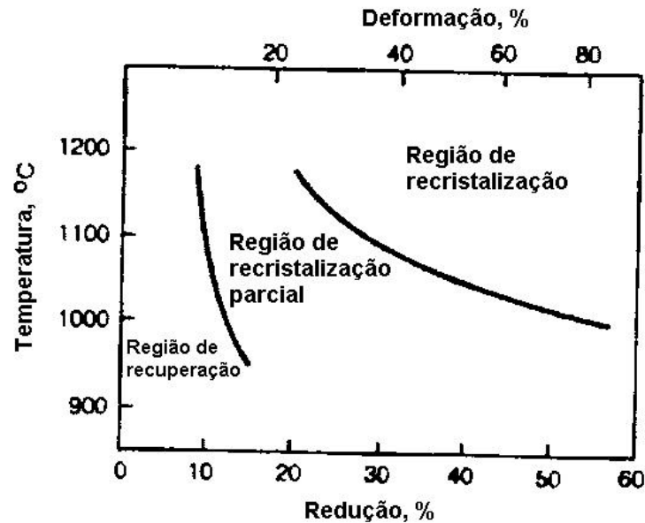
Fig.1.14 - Efeito da quantidade de redução e temperatura de laminação sobre o comportamento da restauração: o aço ao níbio foi aquecido para 1150° C a qual deu um tamanho de grão de aproximadamente 180 \mu\text{m} e laminado em um passe [9].
