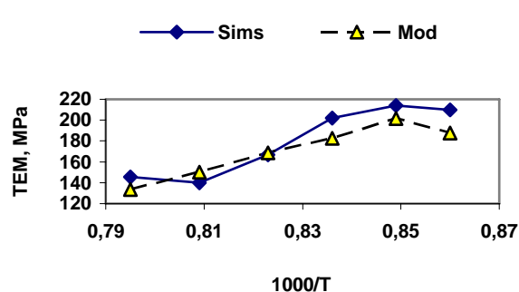
Fig.4.10 – Resultados da TEM obtidas pelo modelo de Sims e pelo modelo com a correção para a equação de Misaka.
