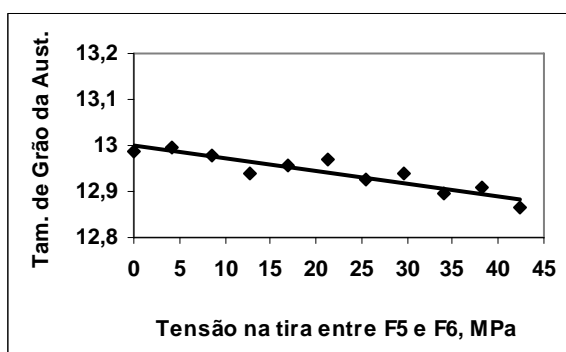
Figura I.28 – Resultados de tamanho de grão ( \mu\text{m} ) obtidos pelo modelo para aço carbono manganês 3, devido a variações provocadas tensão a ré da tira da cadeira F6, tabela F4.1.
