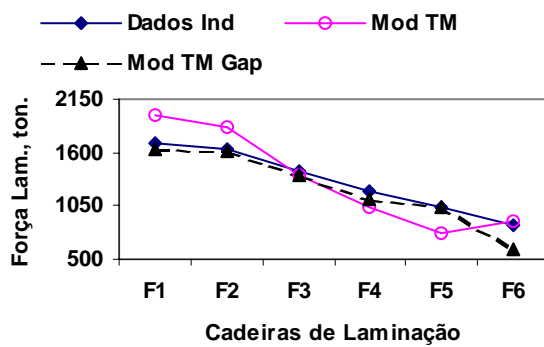
Fig.4.40 – Resultados de força de laminação fornecida pela industria e os obtidos pelo modelo termomicroestrutural utilizando h1 e h2 (Mod TM) e utilizando o gap (Mod TMGap).
