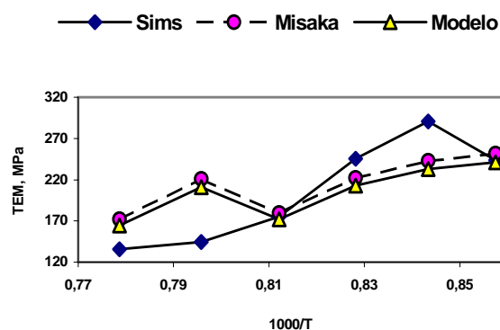
Fig.4.24 – Resultados da TEM obtidas pelo modelo de Sims, pela equação de Misaka com correções e pelo modelo microestrutural.
