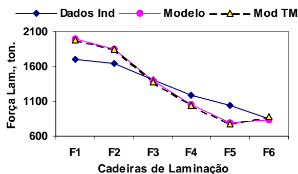
Fig.4.34 – Resultados de força de laminação fornecida pela industria e obtidos pelo modelo com correção pela equação de Misaka (Mod) e pelo modelo termomicroestrutural (Mod TM) também com as correções.
