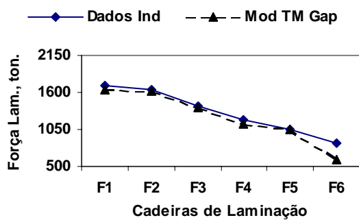
Fig.4.42 – Resultados de força de laminação fornecida pela industria e os obtidos pelo modelo termomicroestrutural utilizando o gap (Mod TMGap).
