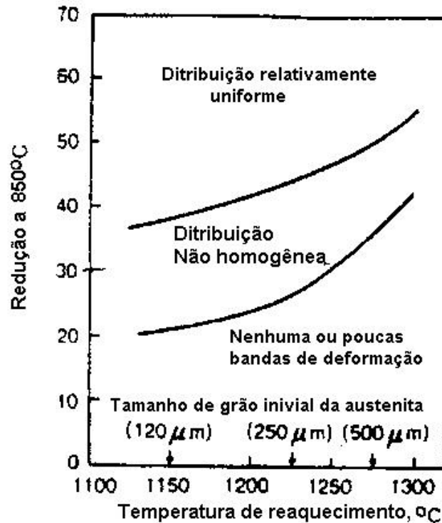
Fig.1.9 - Efeito da quantidade de redução sobre a formação das bandas de deformação
