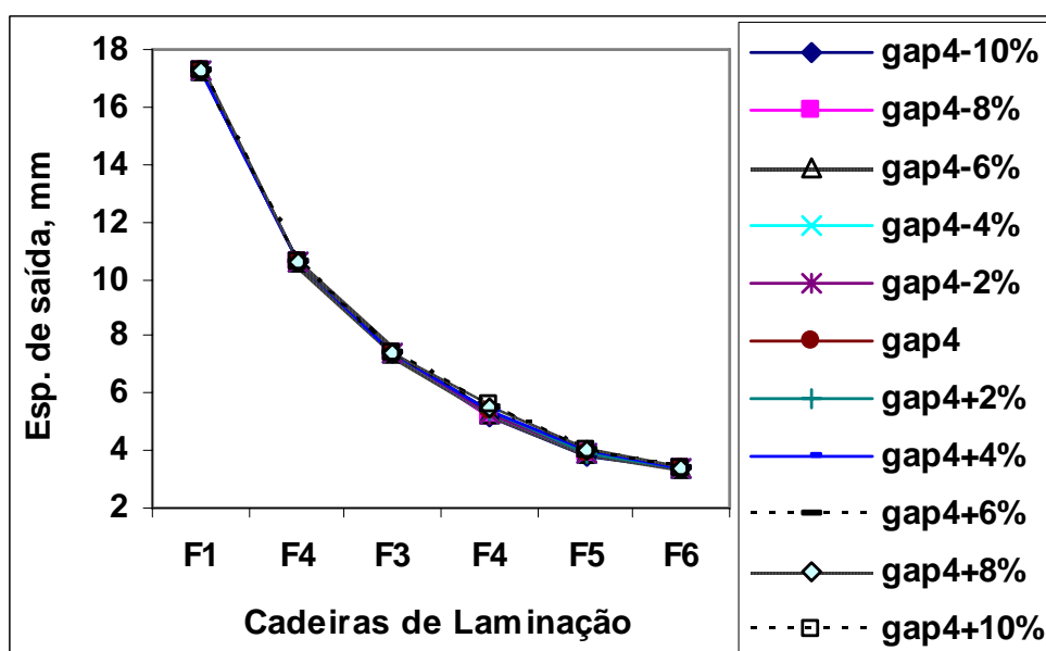
Figura G.15 – Resultados da espessura de saída do material, obtidos pelo modelo para aço carbono manganês 3, devido a variações provocadas no gap em F4, tabela D3.5.
