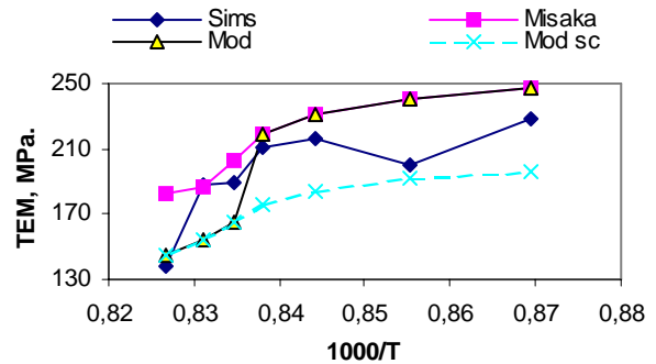
Fig.4.20 – Resultados da TEM obtidas pelo modelo de Sims, pela equação de Misaka com correções e pelo modelo com a correção para a equação de Misaka(Mod) e sem a correção (Mod sc).
