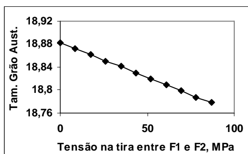
Figura 5.78 – Resultados de tamanho de grão ( \mu\text{m} ) obtidos pelo modelo para aço carbono manganês 3, devido a variações provocadas tensão a ré da tira da cadeira F2, tabela B4.1.
