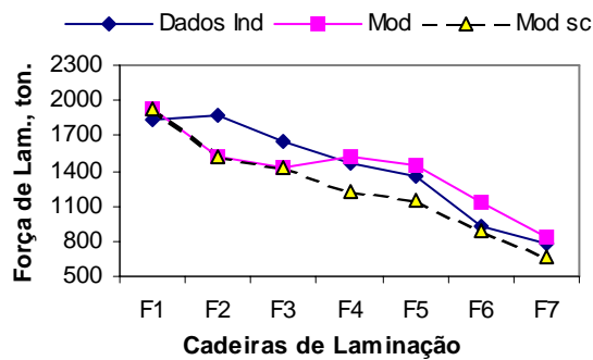
Fig.4.19 – Resultados de força de laminação fornecido pela industria e obtidos pelo modelo microestrutural com a correção para a equação de Misaka(Mod) e sem a correção (Mod sc).
