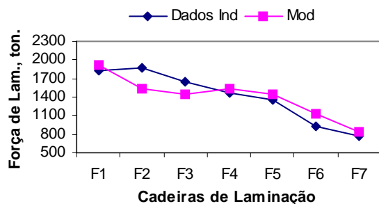
Fig.4.21 – Resultados de força de laminação fornecido pela industria e obtidos pelo modelo microestrutural com a correção para a equação de Misaka(Mod).
