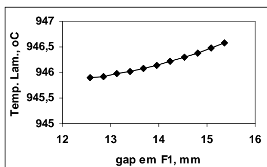
Figura 5.52 – Resultados de temperatura de laminação em F2, obtidos pelo modelo termomicroestrutural para aço carbono manganês 3, devido a variações no gap em F1, tabela B1.1.
