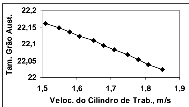
Figura 5.43 – Resultados de tamanho de grão ( \mu\text{m} ) obtidos pelo modelo para aço carbono manganês 3, devido a variações na velocidade do cilindro da cadeira F1, tabela A5.1.
