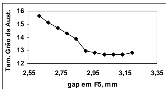
Figura I.3 – Resultados de tamanho de grão ( \mu\text{m} ) em F6 obtidos pelo modelo termomicroestrutural para aço carbono manganês 3, devido a variações no gap em F5, tabela F1.1.
