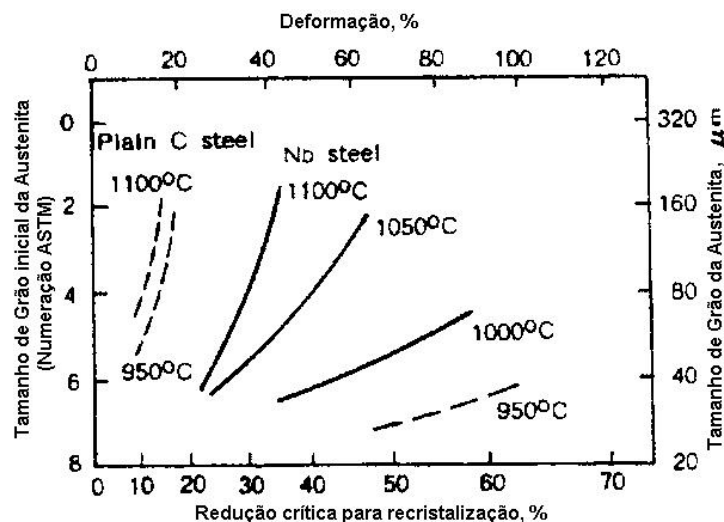
Fig.1.12 - Efeito da temperatura de deformação e do tamanho de grão sobre a quantidade crítica de redução necessária para a completa recristalização no aço carbono e ao nióbio.
