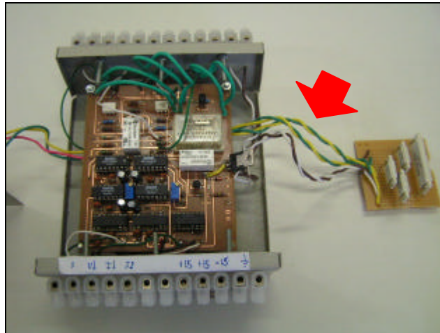
Figura 4.23 – Foto do sistema de medição com fios em paralelo com resistores do divisor
