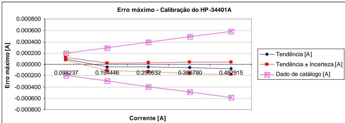
Figura C.63 – Gráfico de erro máximo na medição de corrente CC do multímetro HP-34401A, faixa de 0.1 a 0.5 A
