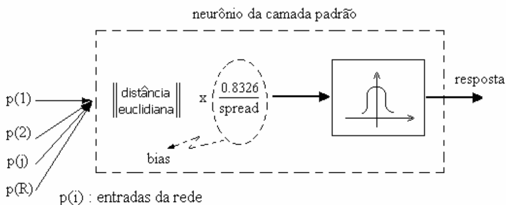
Figura 3.3 – Neurônio da camada padrão [25].
