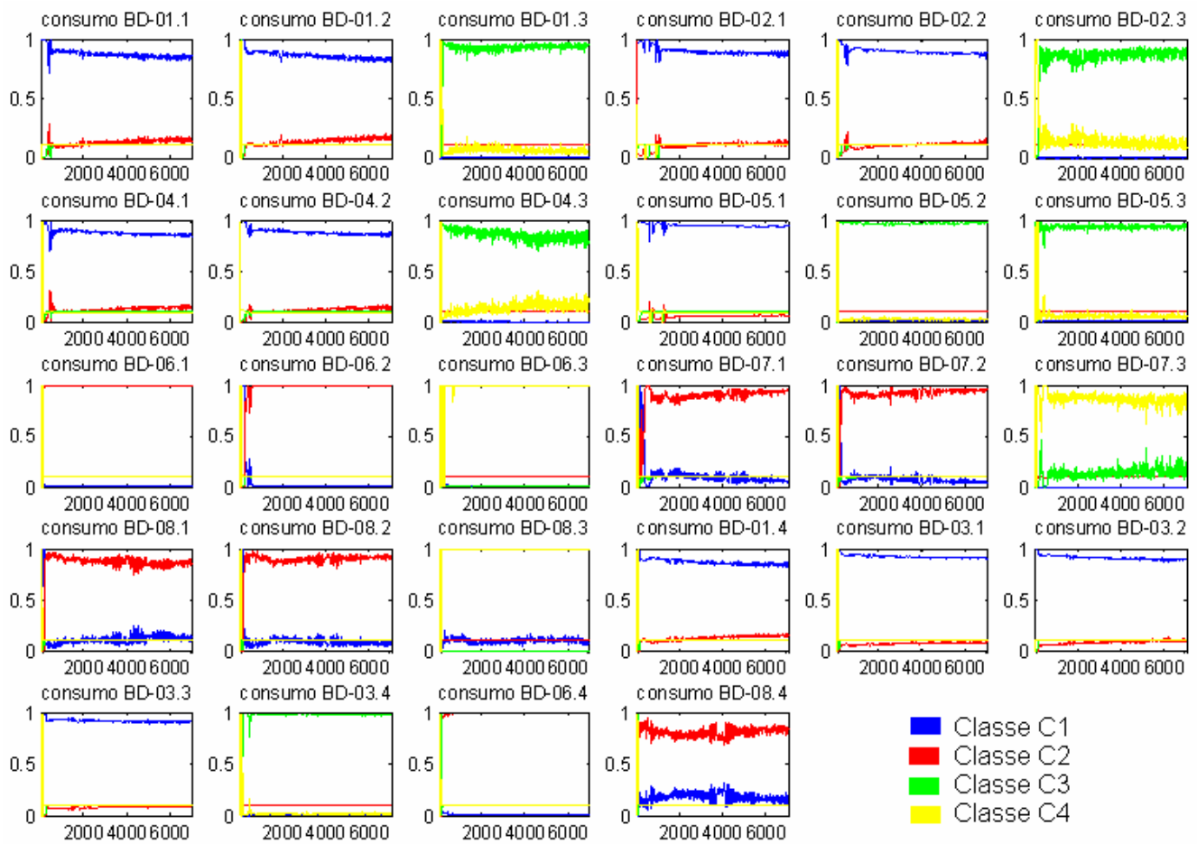
Figura 6.16 – Saídas da RNA de consumo para todos os ensaios.
