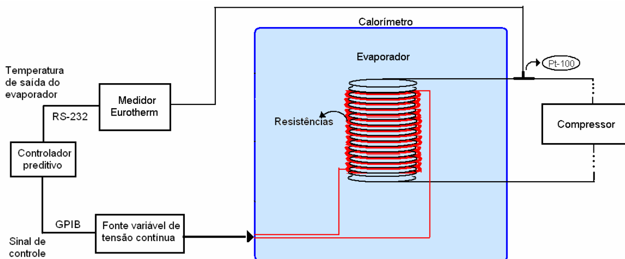
Figura 4.5 – Situação atual do controle de temperatura de saída do evaporador.
