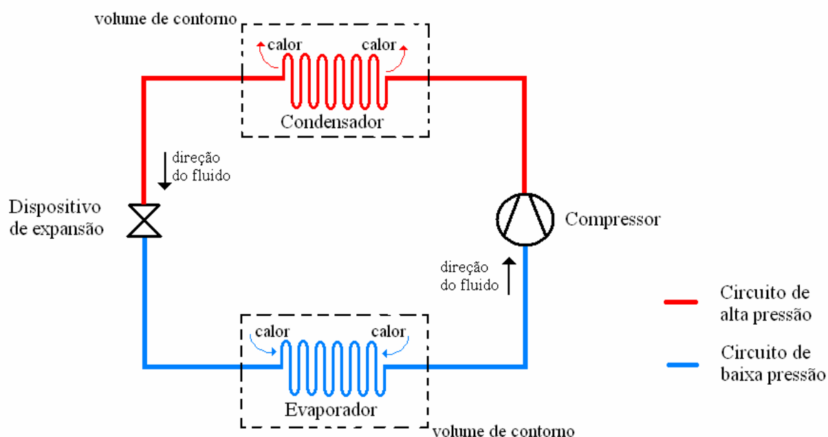
Figura 2.2 - Circuito básico de refrigeração.
