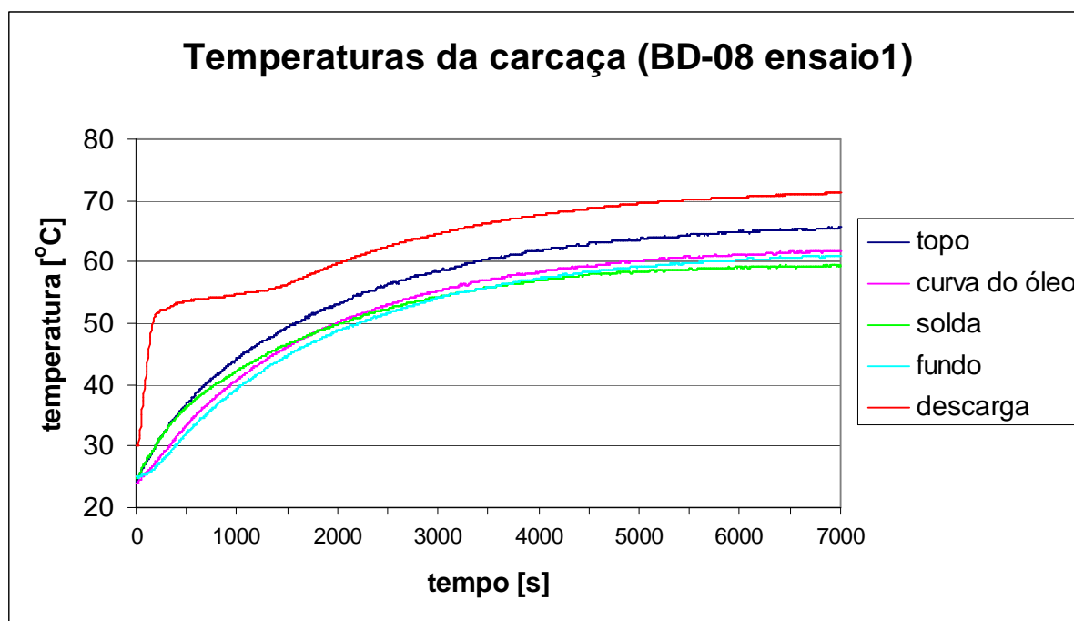
Figura 5.2 - Gráfico das temperaturas da carcaça (BD-08).
