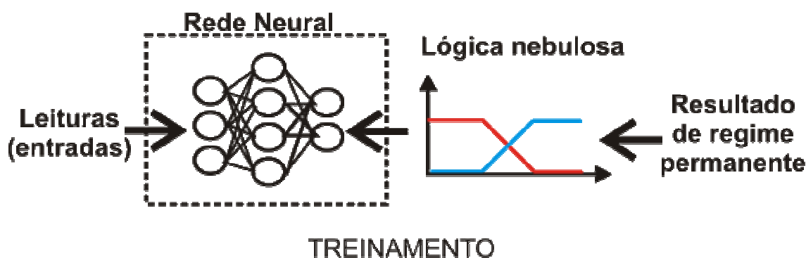
Figura 5.10 – Uso de lógica nebulosa durante o treinamento da rede.
