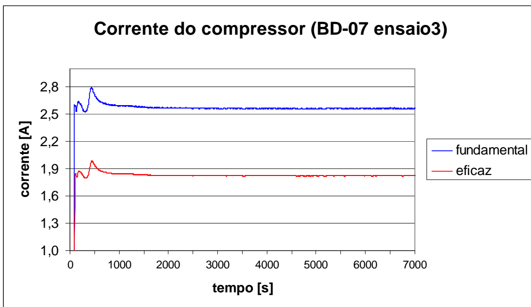
Figura 5.5 – Gráfico da corrente que circula pelo compressor.
