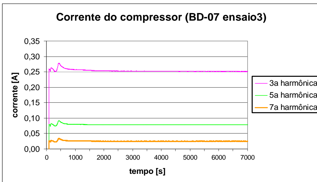
Figura 5.6 – Harmônicas de corrente BD-07 ensaio 3.
