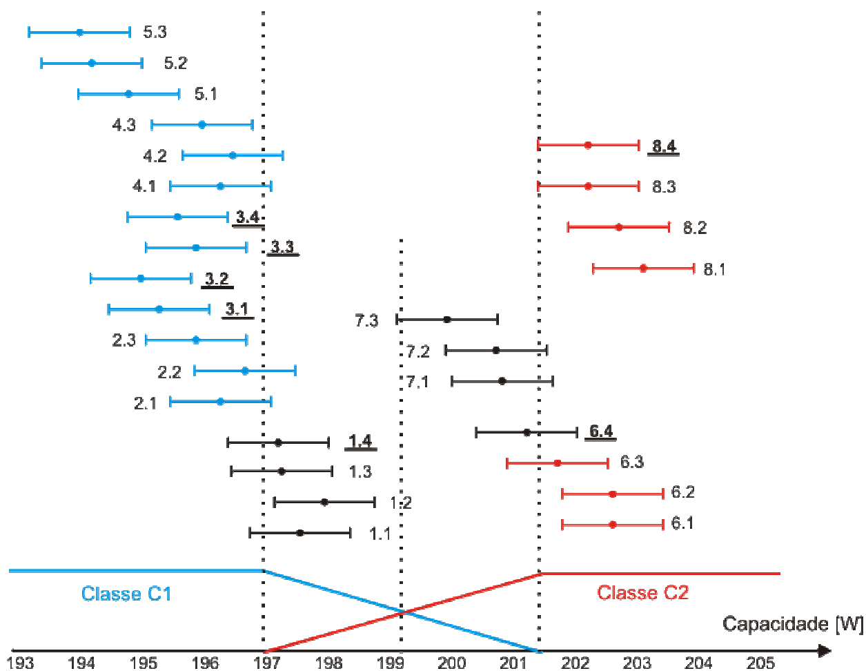
Figura 6.5 – Classificação dos resultados de capacidade de refrigeração.
