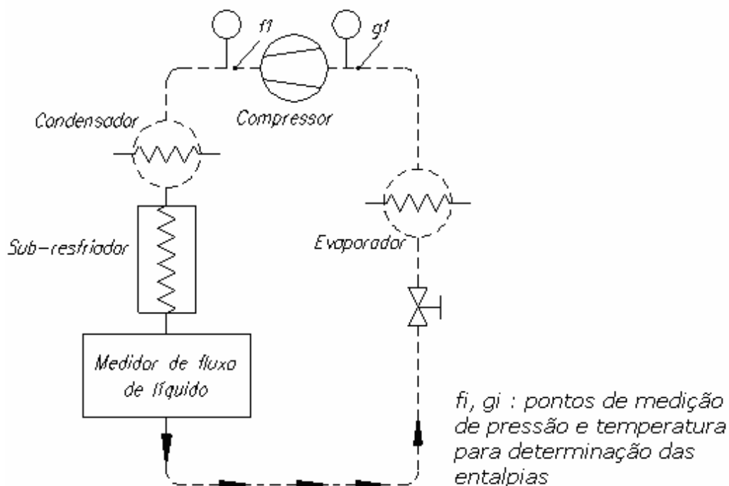
Figura 2.6 – Diagrama do circuito (método F) [4].
