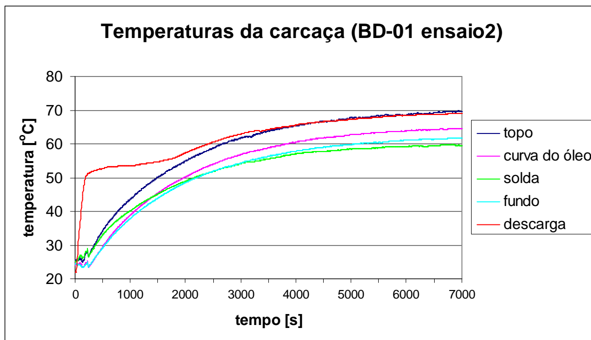
Figura 5.1 – Gráfico das temperaturas da carcaça (BD-01).
