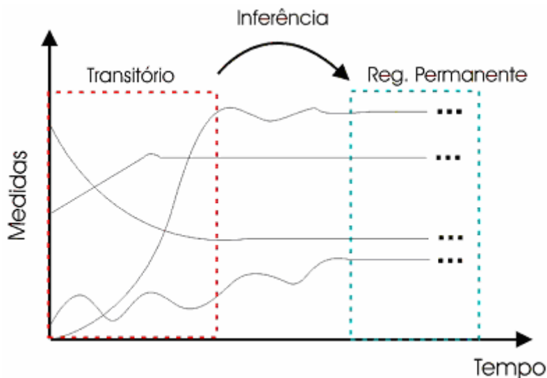
Figura 1.1 - Regime transitório e permanente.
