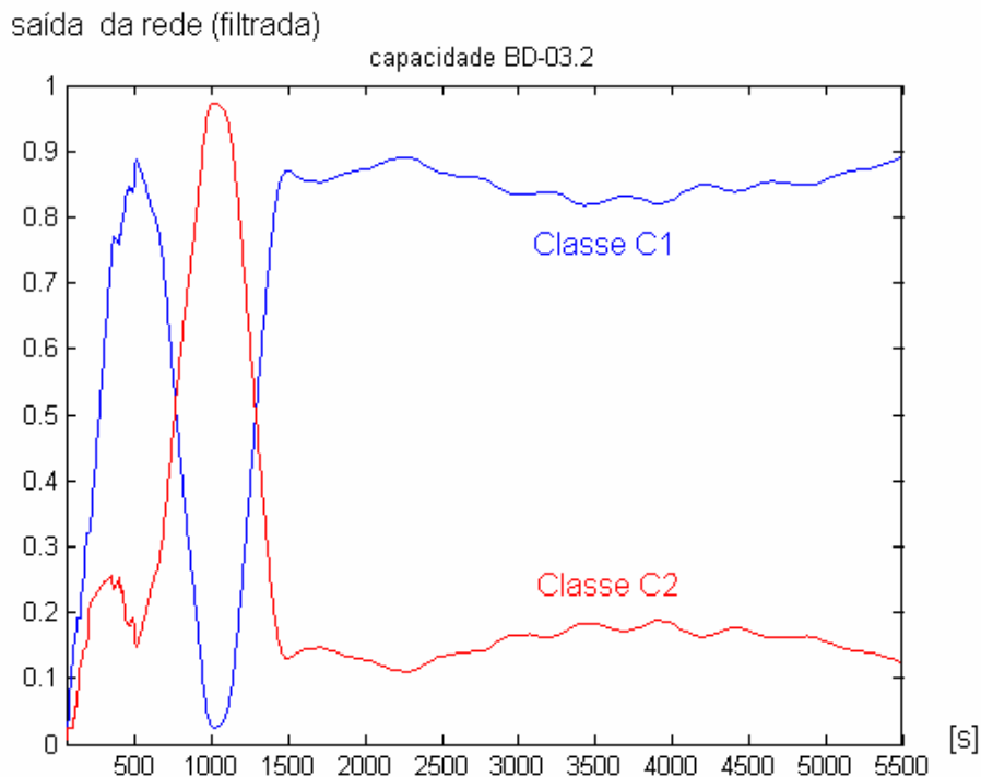
Figura 6.8 - Saída filtrada da RNA de capacidade para o ensaio BD-03.2.
