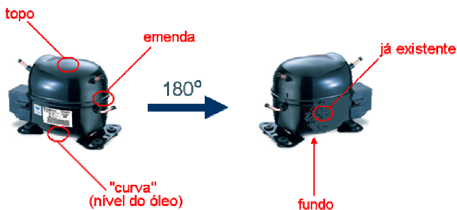
Figura 4.1 – Pontos para medição de temperatura da carcaça.
