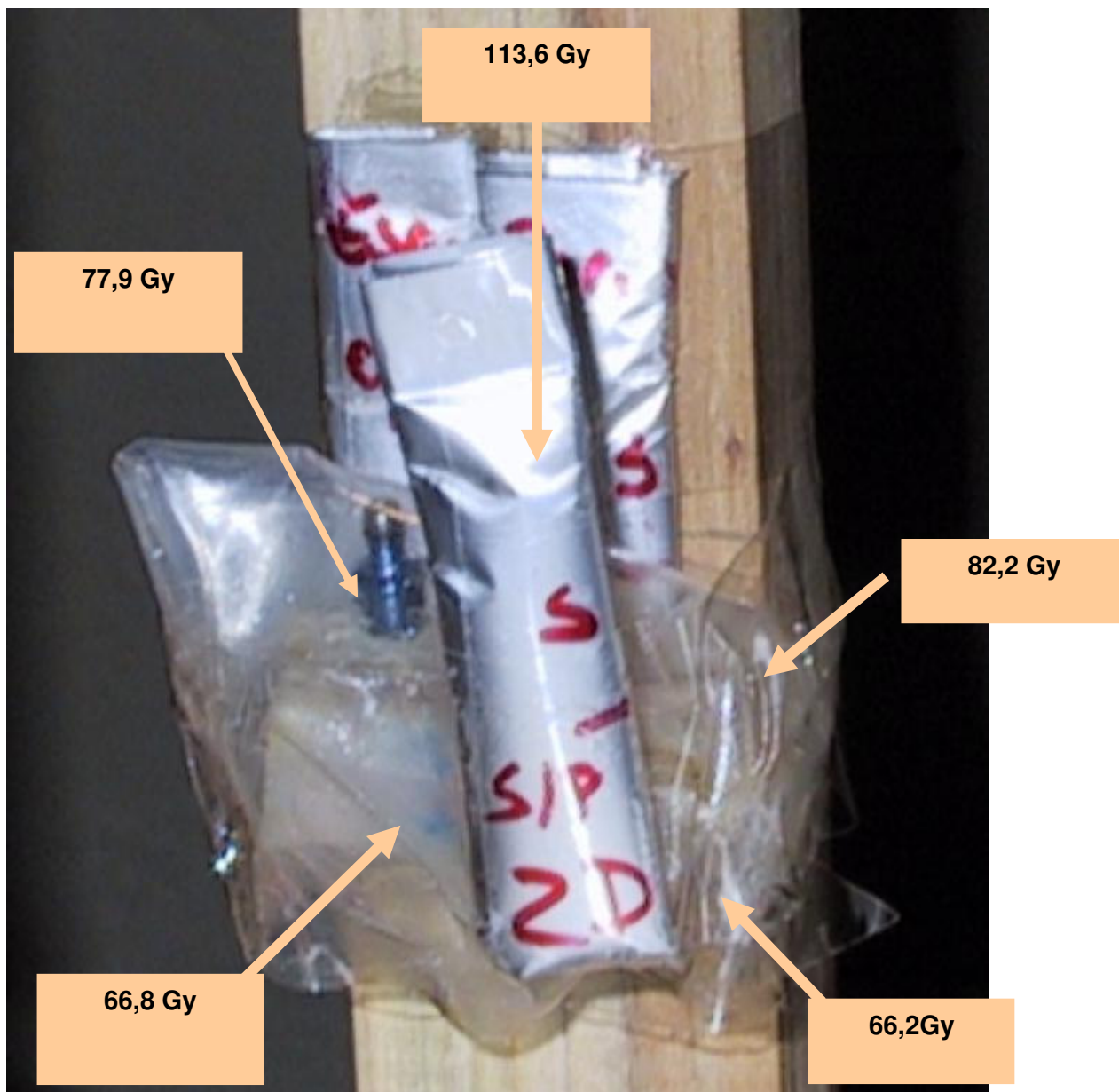
Figura 18 – Valores obtidos após irradiação do implante com radiação gama (100Gy), amostra 2
