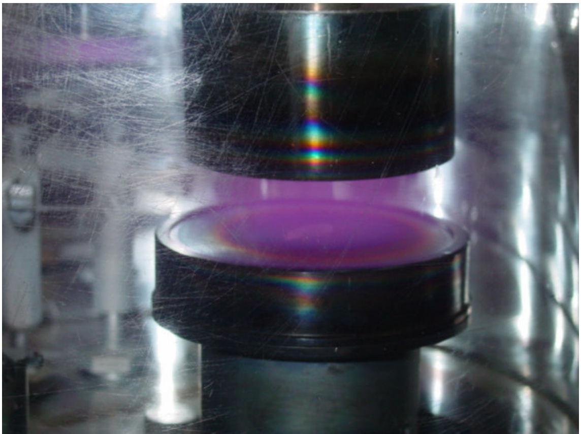
Figura 11 - Equipamento de Imersão a Plasma
