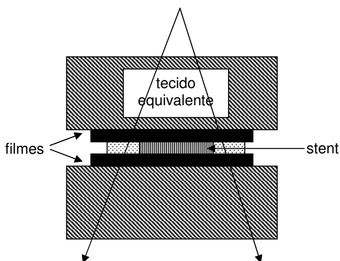
Figura 7 – Conjunto experimental desenvolvido por Gez et al. (1997)
