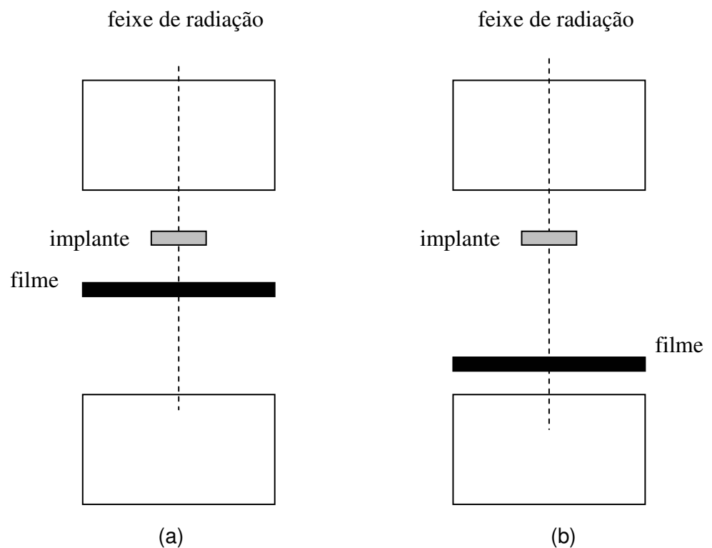
Figura 6 - Conjunto de modelos usados por Niroomand-Rad et al. (1995) para determinar: (a) dose (b) redução da dose
