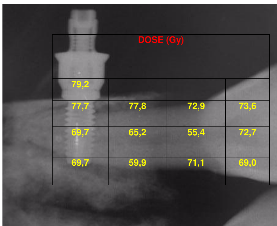
Figura 22 – Valores obtidos para implante de titânio com revestimento (50µm), amostra 6
