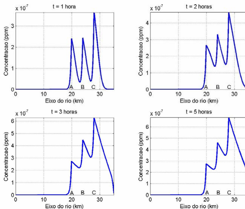
Figura 10 - Simulação do cenário 2: Distribuição da concentração de esgoto ao longo do rio, para quatro instantes de tempo (estação seca).
