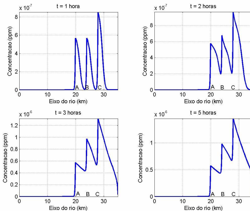
Figura 8 - Simulação do cenário 1: Distribuição da concentração de esgoto ao longo do rio, para quatro instantes de tempo (estação seca).
