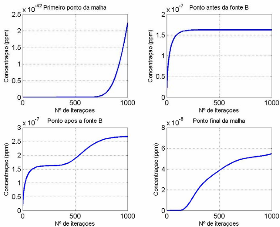
Figura 13 - Simulação do cenário 4: Processo evolutivo da concentração de esgoto, ao longo do tempo, para quatro nós distintos (estação chuvosa).
