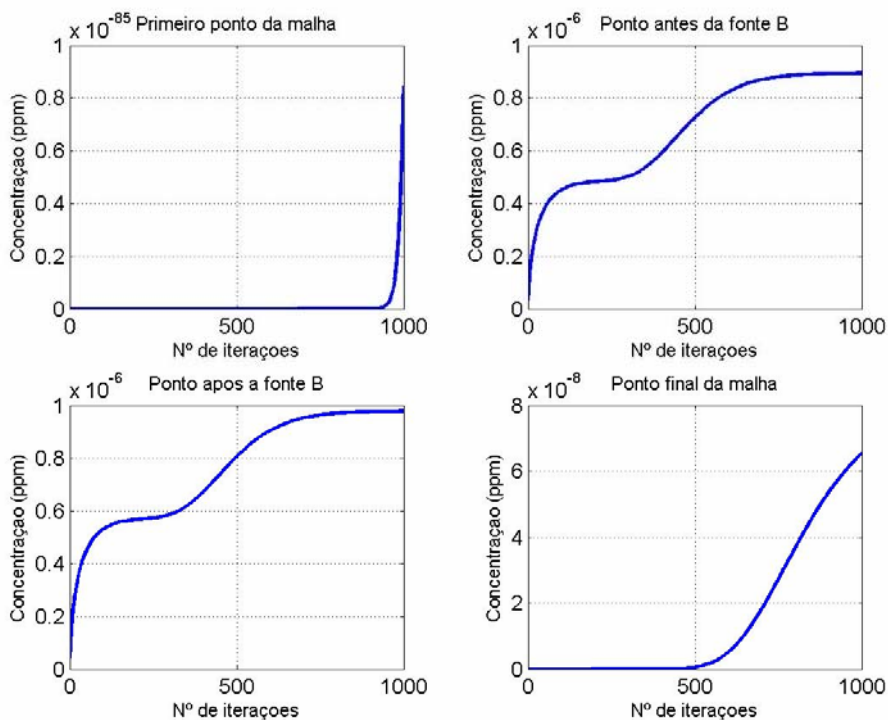
Figura 7 - Simulação do cenário 1: Processo evolutivo da concentração de esgoto, ao longo do tempo, para quatro nós distintos (estação seca).
