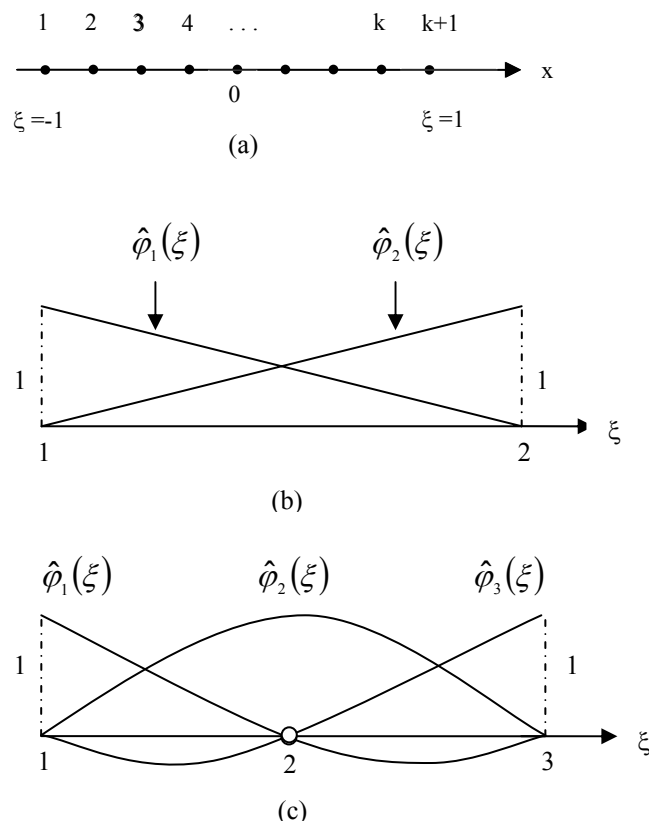
Figura 4 - (a) O elemento principal \hat{\Omega} com k+1 nós; (b) Forma linear correspondente para k = 1 e (c) Um elemento com três nós e a função quadrática por partes ( k = 2 ).
