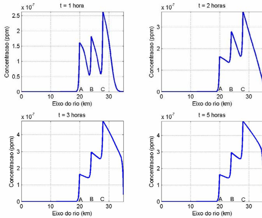
Figura 14 - Simulação do cenário 4: Distribuição da concentração de esgoto ao longo do rio, para quatro instantes de tempo (estação chuvosa).
