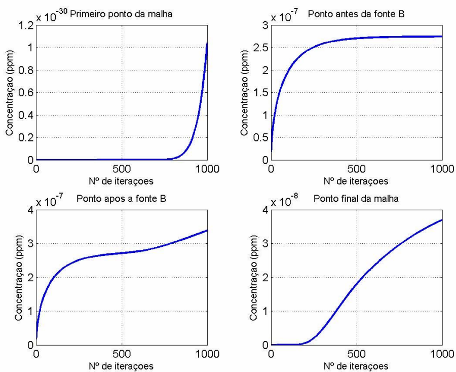
Figura 9 - Simulação do cenário 2: Processo evolutivo da concentração de esgoto, ao longo do tempo, para quatro nós distintos (estação seca).
