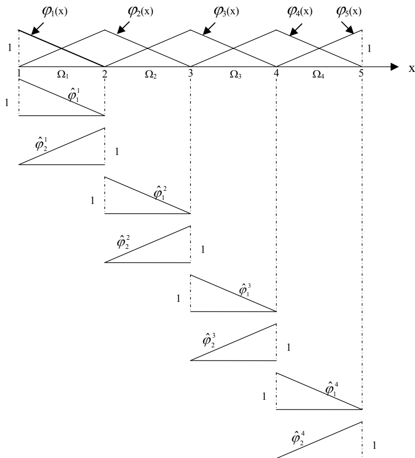
Figura 5 - Funções locais lineares por partes \varphi_1(x) para uma malha gerada por funções lineares com 4 elementos, \hat{\varphi}_1^e(x) , \hat{\varphi}_2^e(x) definida sobre cada elemento.
