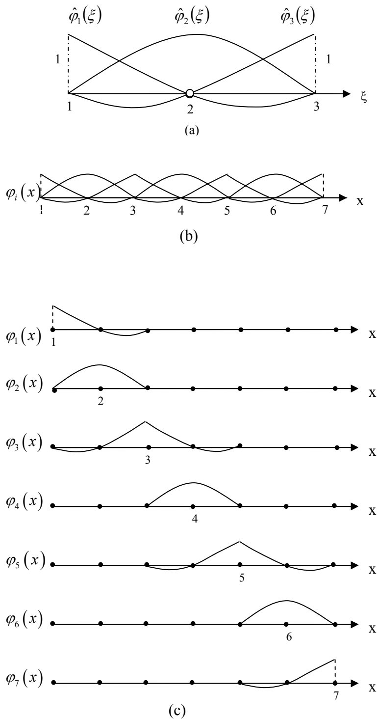
Figura 6 - (a) Função quadrática com três nós; (b) Uma malha composta de três funções locais quadráticas e (c) A função global gerada por esses elementos.
