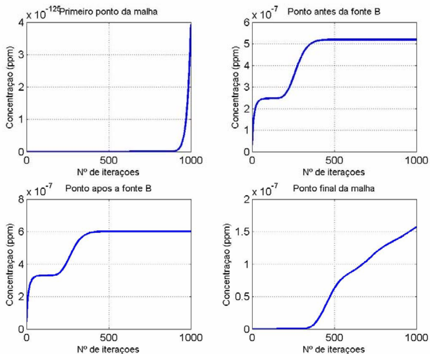
Figura 11 - Simulação do cenário 3: Processo evolutivo da concentração de esgoto, ao longo do tempo, para quatro nós distintos (estação chuvosa).
