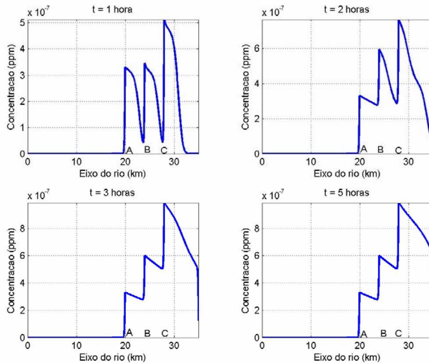
Figura 12 - Simulação do cenário 3: Distribuição da concentração de esgoto ao longo do rio, para quatro instantes de tempo (estação chuvosa).
