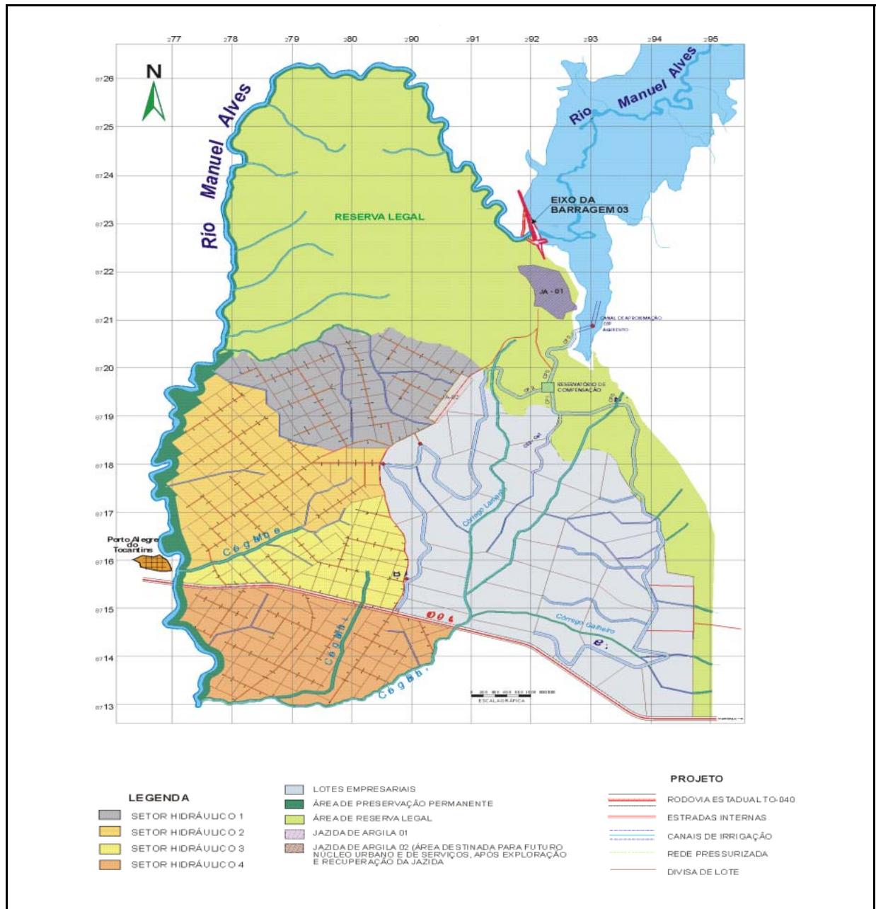
Figura 5. Concepção básica do Projeto de Irrigação Manuel Alves, Dianópolis – TO (ACL, 2002)
