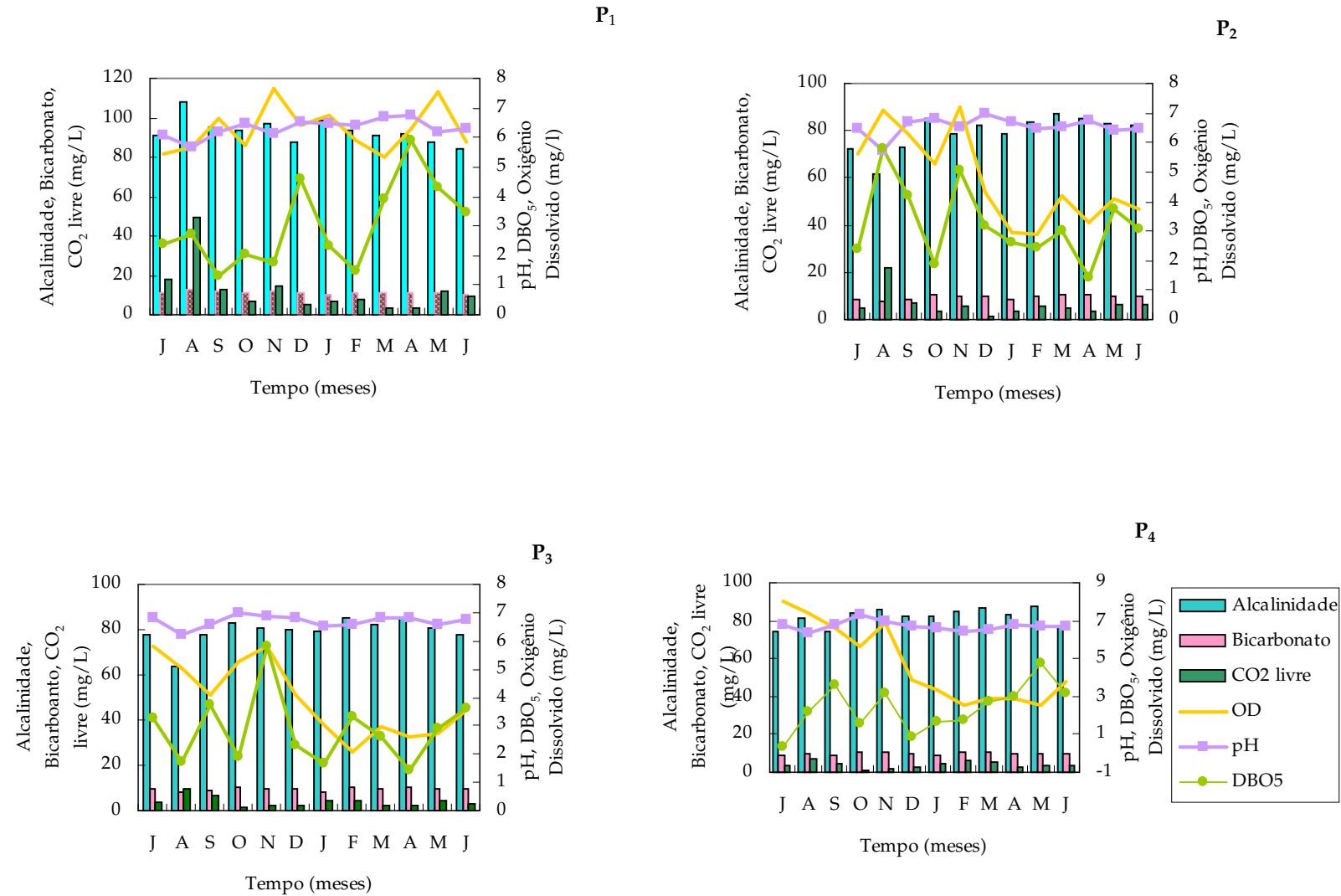
Figura 2. Variação da alcalinidade, bicarbonato, CO 2 livre, oxigênio dissolvido (OD), pH e demanda bioquímica de oxigênio (DBO 5 ) durante o período de estudo nos quatro pontos amostrados (P 1 = entrada de água, P 2 = entrada de água proveniente da carcinocultura, P 3 = retirada de água para irrigação e P 4 = saída de água para outro viveiro).
