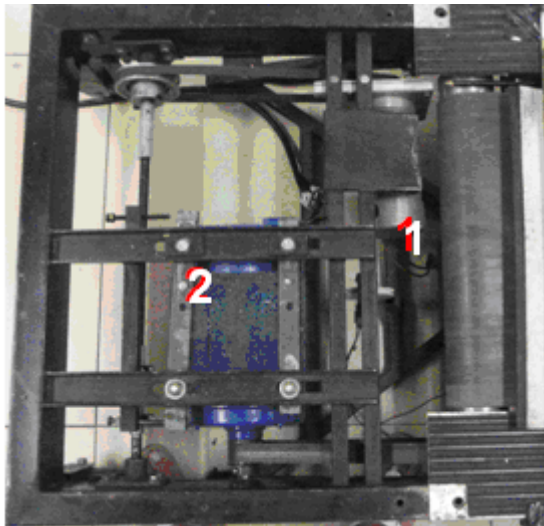
Figura 32: Ilustração dos Motores (1: inclinação; 2: velocidade)
