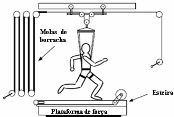
Figura 11: Simulador de gravidade reduzida com tração vertical. Fonte: Donelan & Kram (2000).
