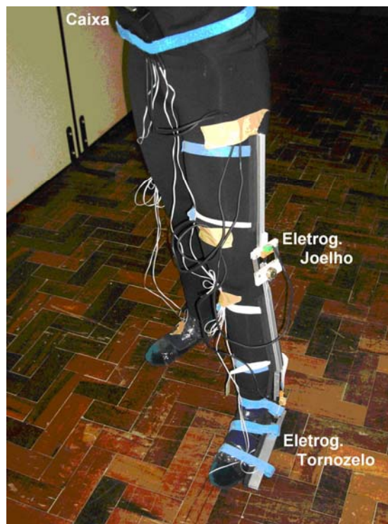
Figura 51: Instrumentação do indivíduo com os eletrogoniômetros e footswitches (sob os pés).
