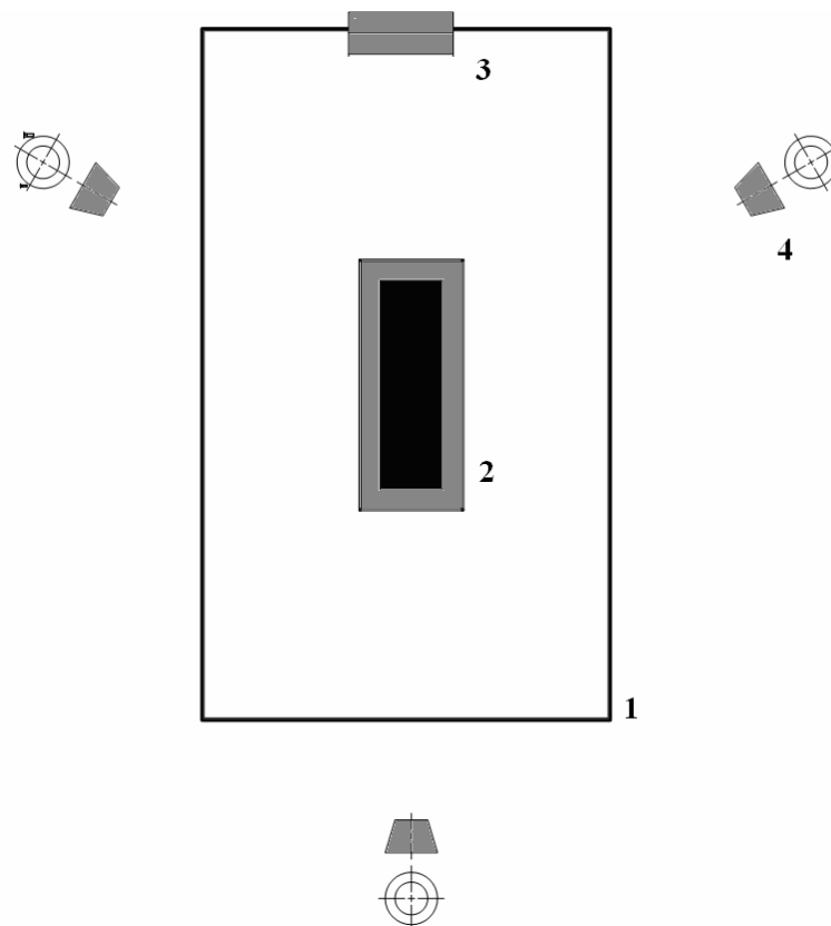
Figura 47: Técnica de videografia com 3 câmeras e sem iluminação, onde 1: SSC; 2: esteira; 3: sistema de contrapesos; e 4: as filmadoras.
