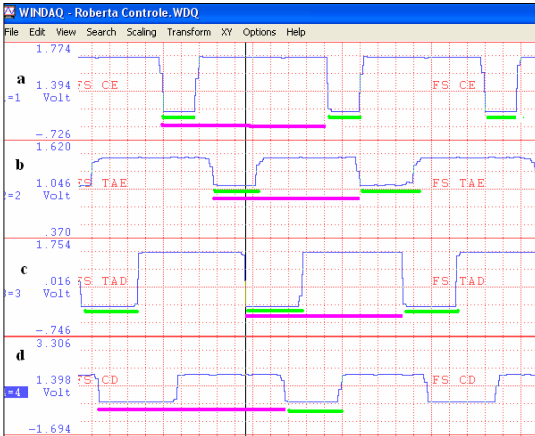
Figura 57: Tempo de Passada (linha rosa) e Tempo de Contato (linha verde). Em “a” calcâneo esquerdo, em “b” terço-anterior esquerdo, “c” terço-anterior direito e “d” calcâneo direito.
