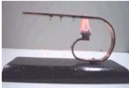
Figura 29 – Experimento: Barra Metálica
