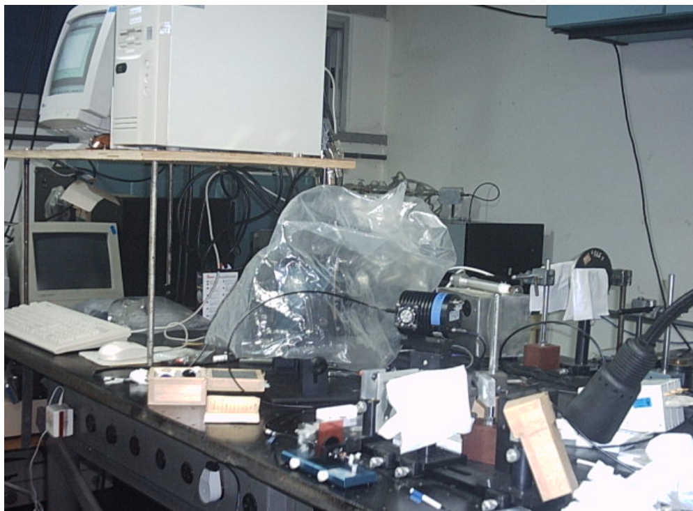
FIGURA 14a - ESPECTROMETRIA NO LABORATÓRIO DE LASER – IF/UFRGS
