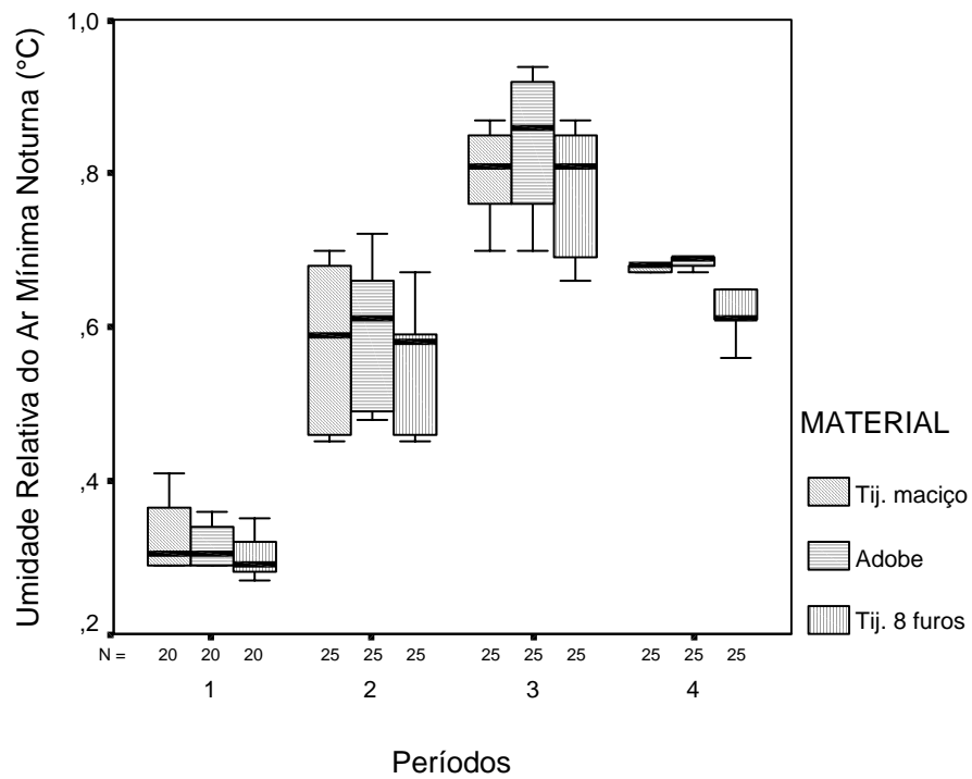
FIGURA 21 - Umidade relativa do ar mínima noturna x Períodos das coletas
