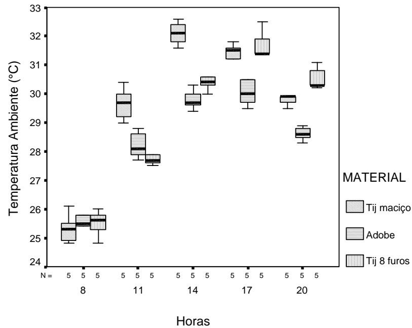
FIGURA 30 - Temperatura ambiente x Horários das coletas do período 1
