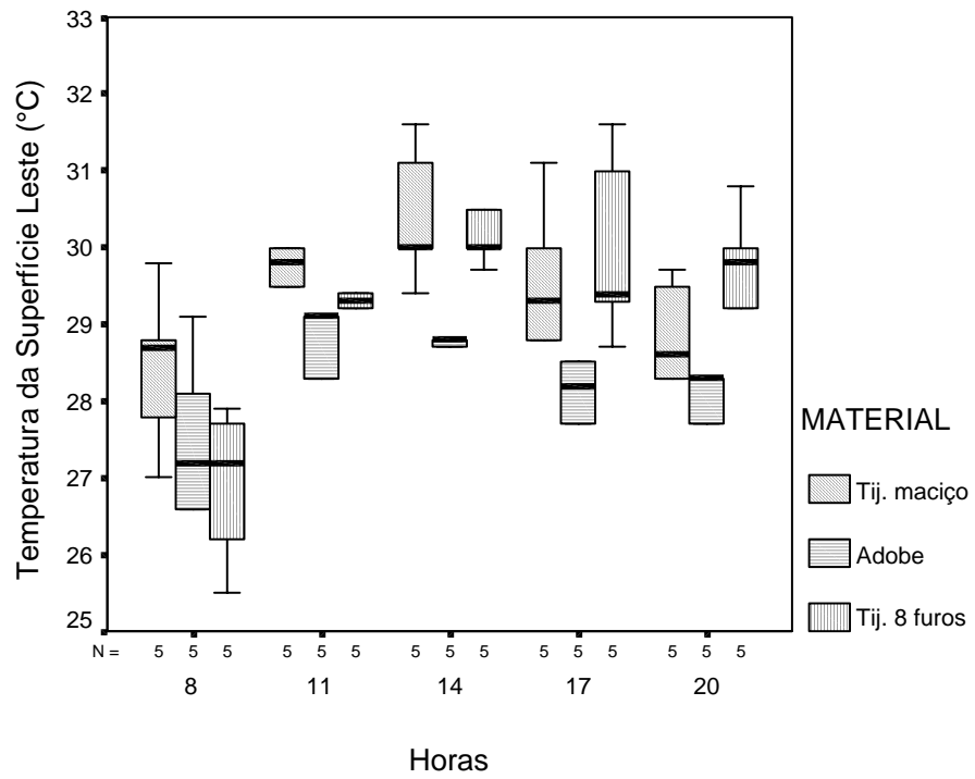
FIGURA 46 - Temperatura da superfície leste x Horários das coletas do período 4
