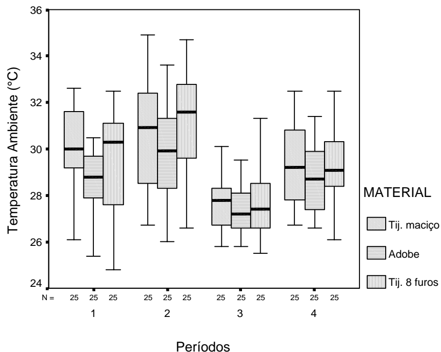
FIGURA 10 - Temperatura ambiente x Períodos das coletas
