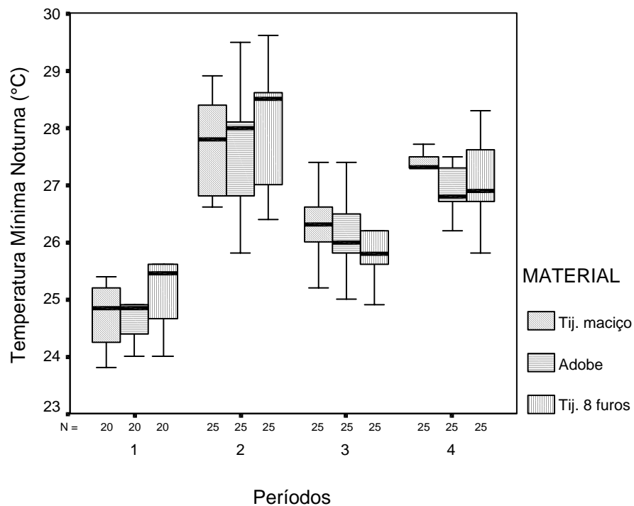
FIGURA 17 - Temperatura ambiente mínima noturna x Períodos das coletas
