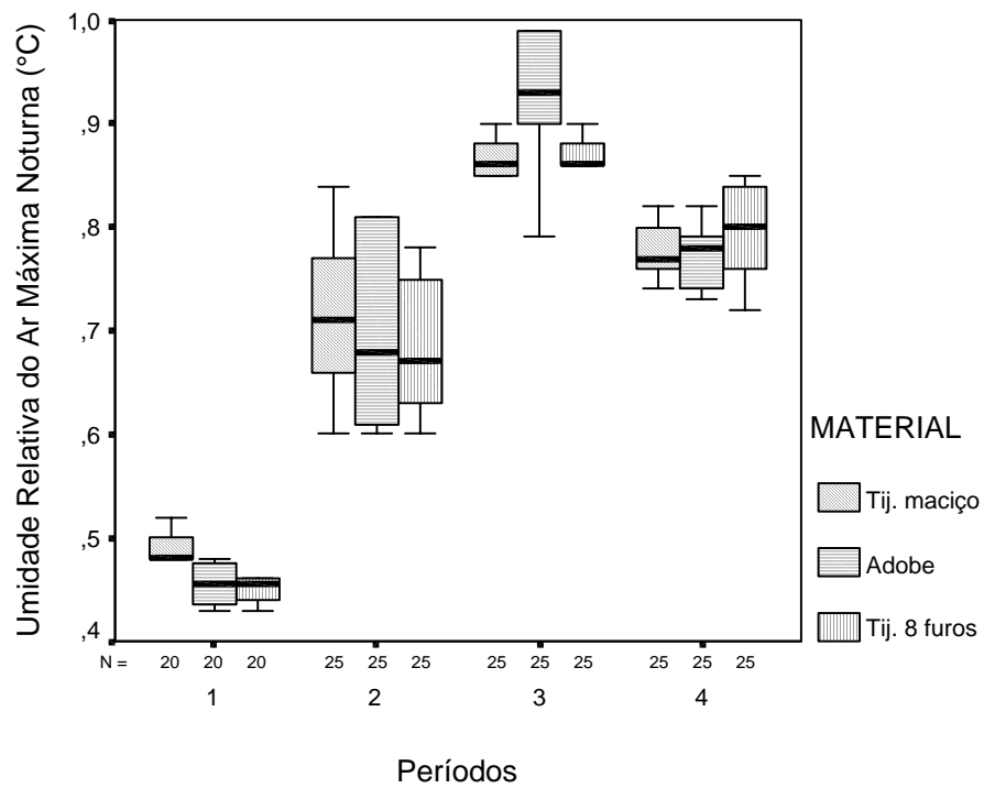
FIGURA 19 - Umidade relativa do ar máxima noturna x Períodos das coletas
