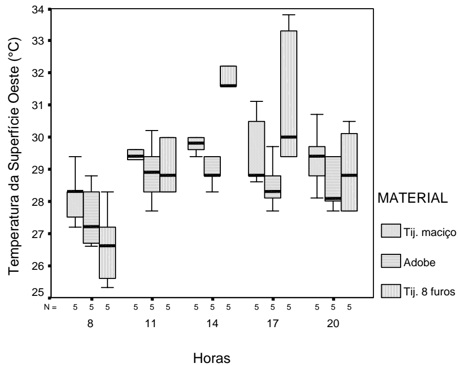
FIGURA 45 - Temperatura da superfície oeste x Horários das coletas do período 4
