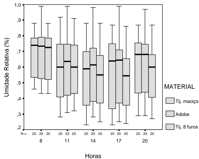
FIGURA 27 - Umidade relativa do ar x Horários das coletas
